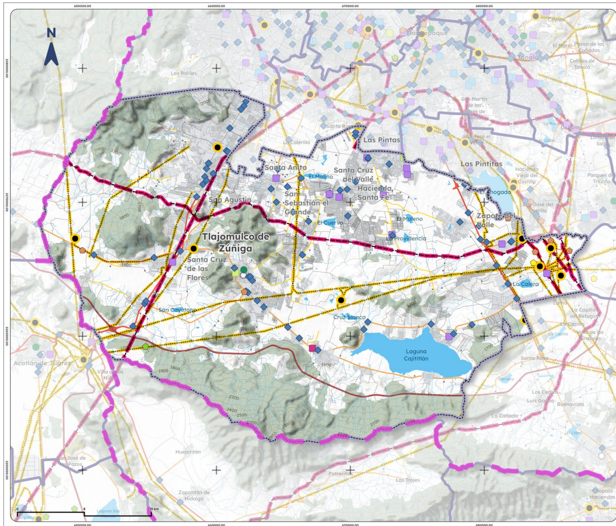
Mapa 22. Infraestructura energética de Tlajomulco de Zúñiga, 2025
