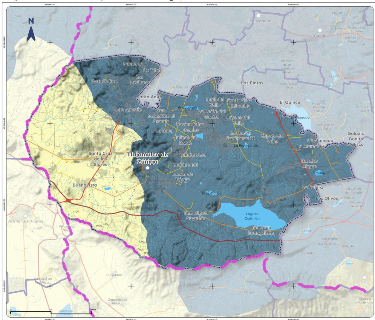
Mapa 6. Cuencas de Tlajomulco de Zúñiga, 2023
