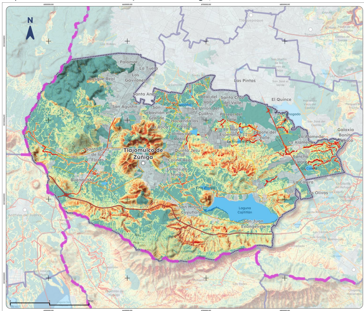
Mapa 17. Erosión efectiva de Tlajomulco de Zúñiga, 2025
