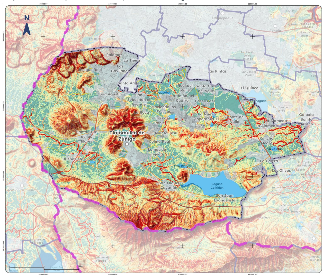
Mapa 16. Erosión potencial de Tlajomulco de Zúñiga, 2025
