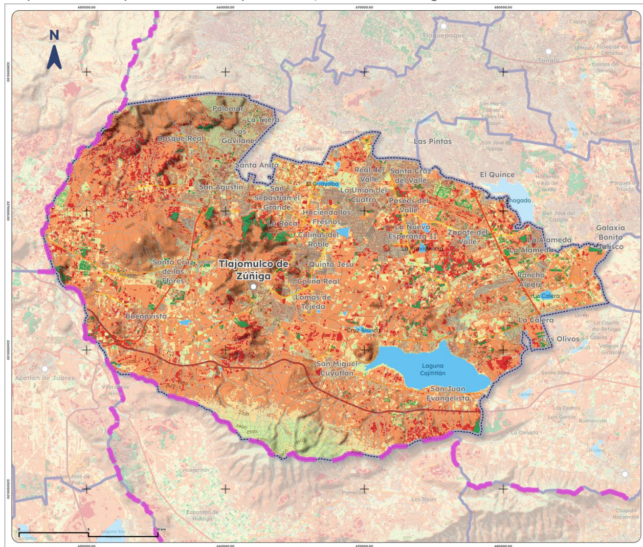
Mapa 15. Índice promedio de sequía de Tlajomulco de Zúñiga, 2025
