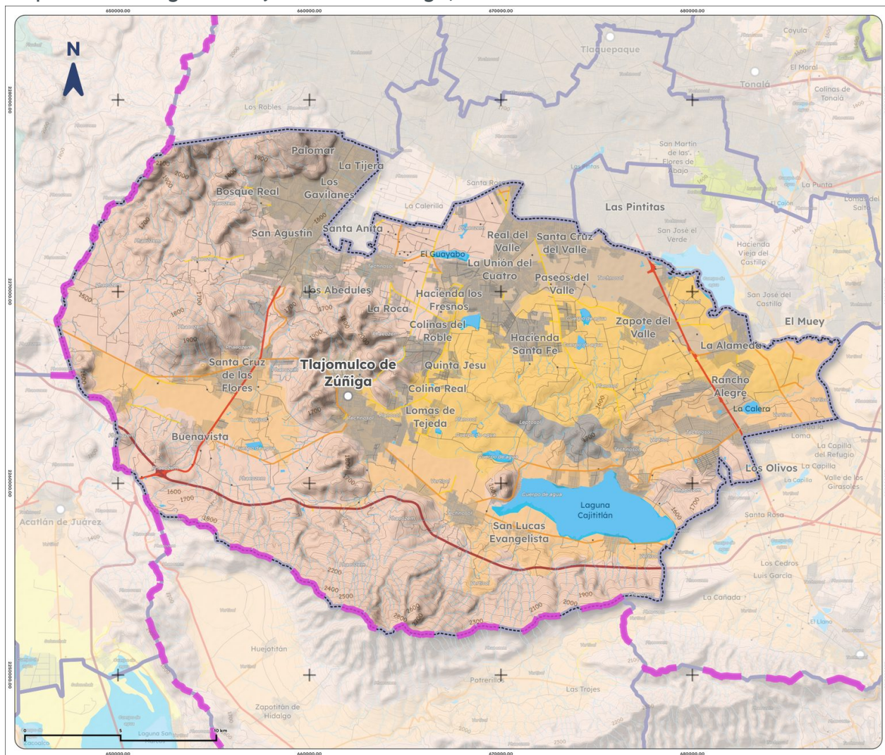
Mapa 4. Edafología de Tlajomulco de Zúñiga, 2025
