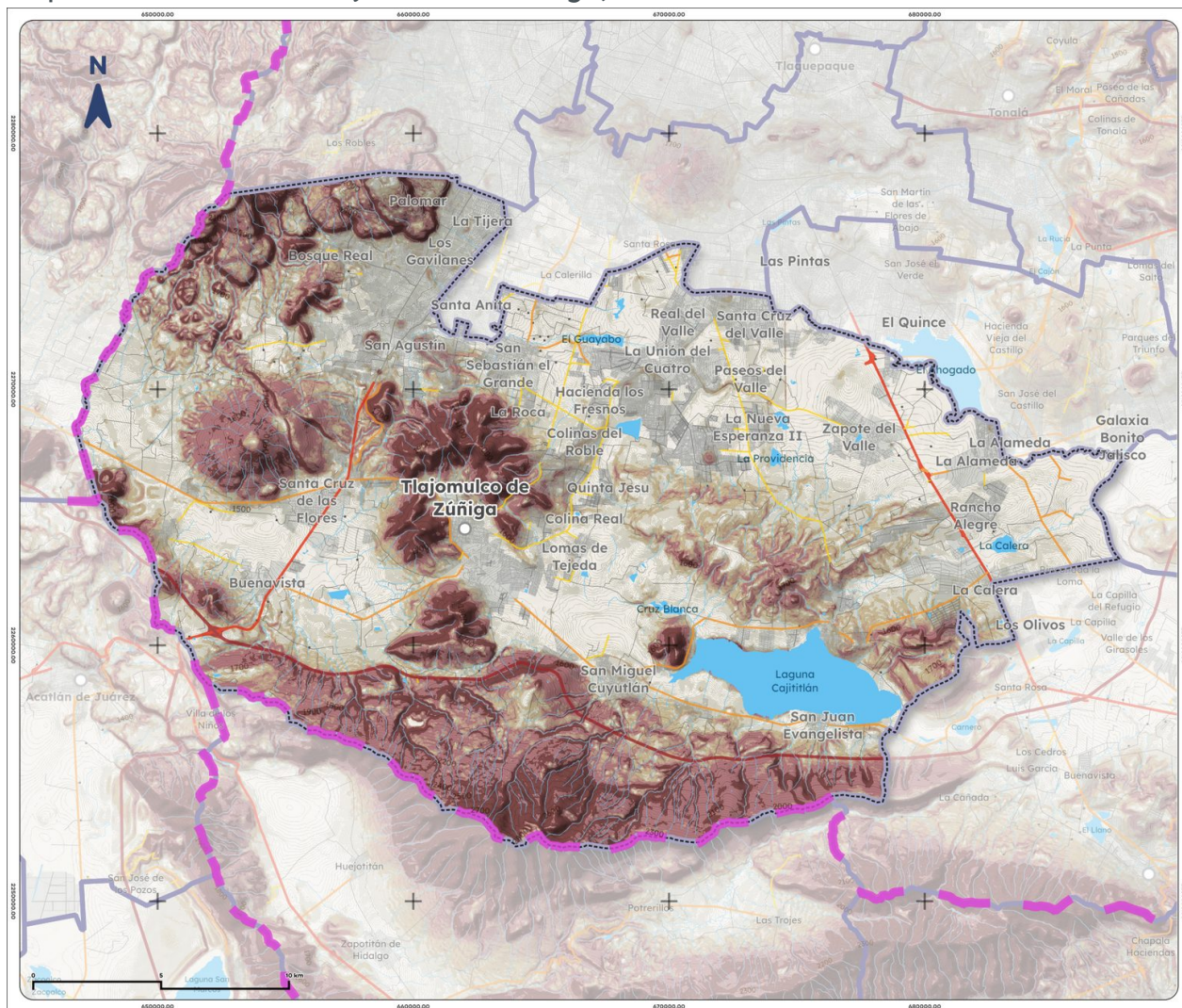
Mapa 5. Pendientes de Tlajomulco de Zúñiga, 2025
