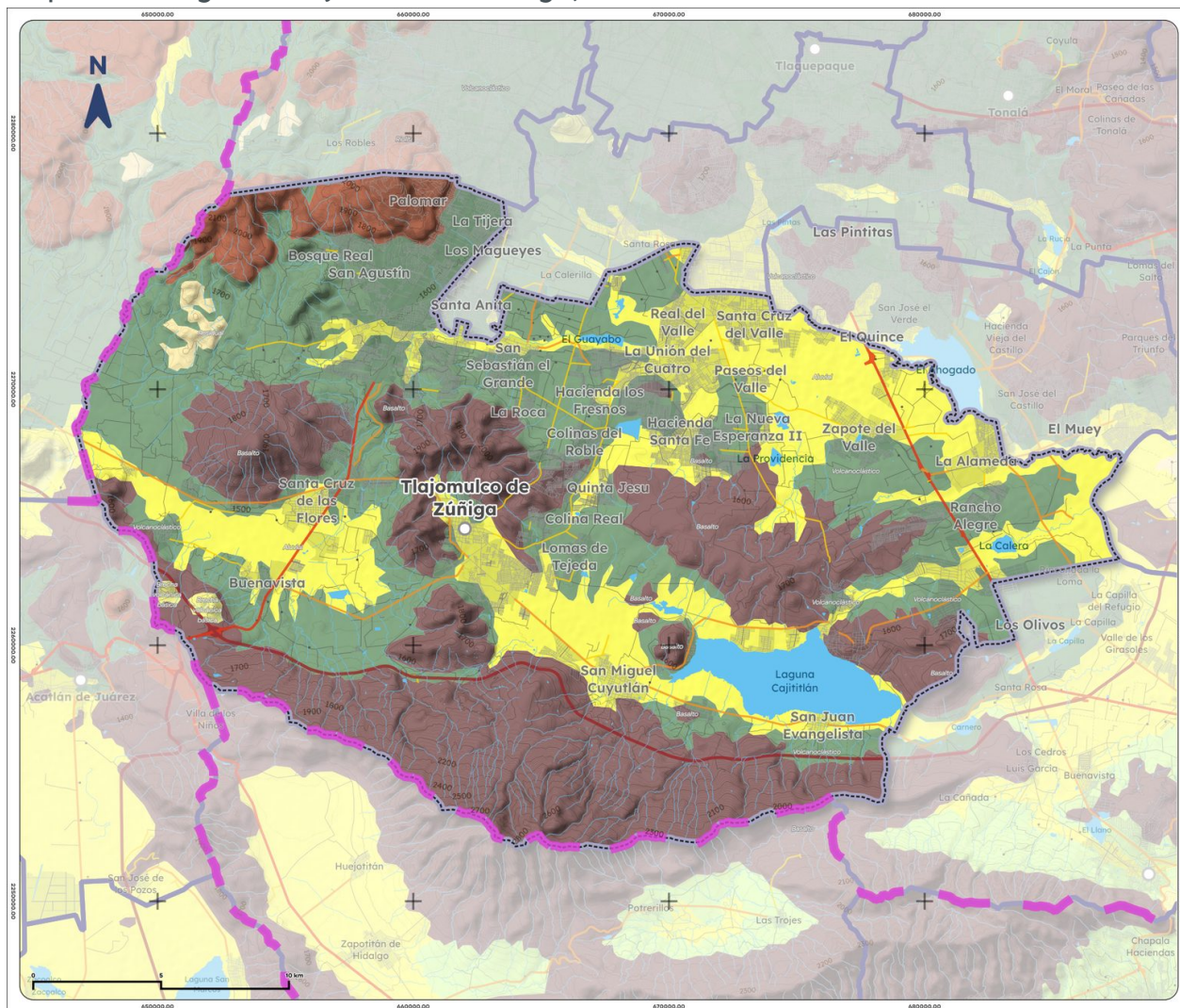
Mapa 3. Geología de Tlajomulco de Zúñiga, 1988
