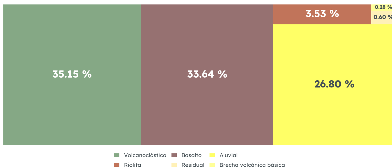
Geología de Tlajomulco de Zúñiga, 1988
