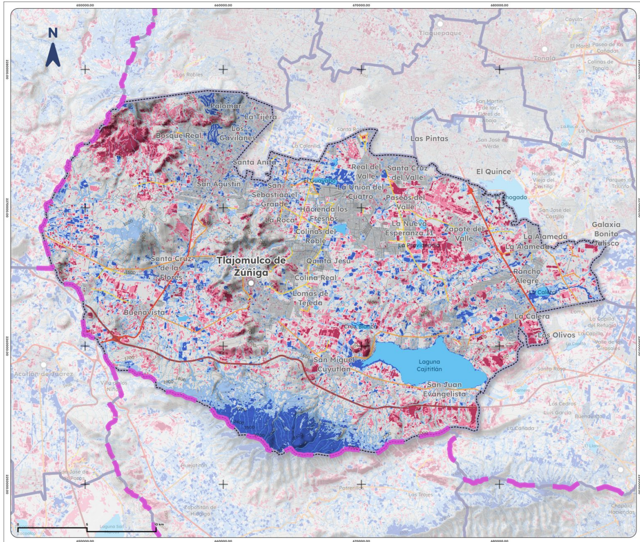
Mapa 13. NDWI promedio de Tlajomulco de Zúñiga, 2025
