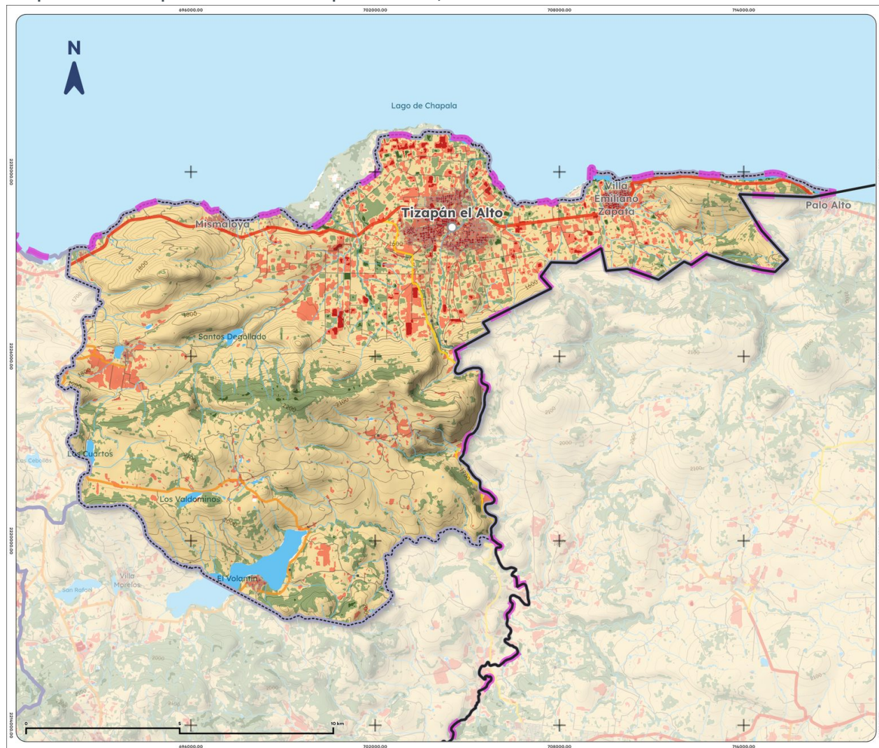
Mapa 12. NDVI promedio de Tizapán el Alto, 2025
