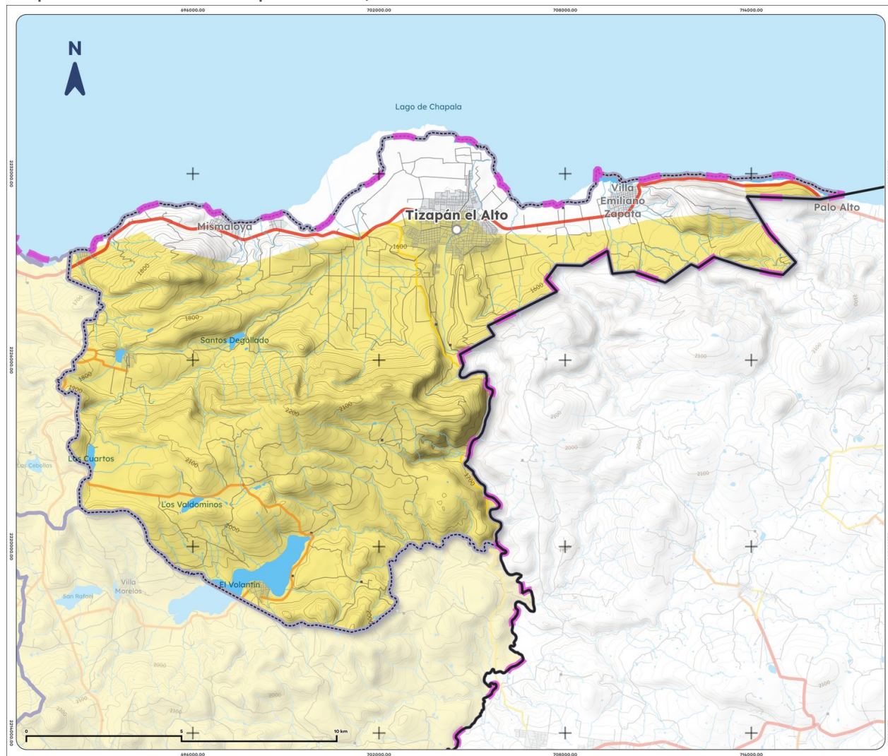
Mapa 7. Acuíferos de Tizapán el Alto, 2023
