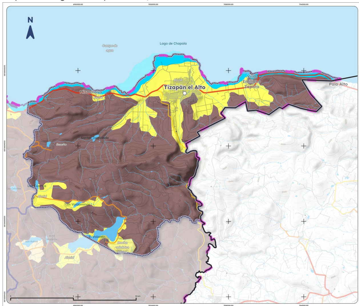
Mapa 3. Geología de Tizapán el Alto, 1988
