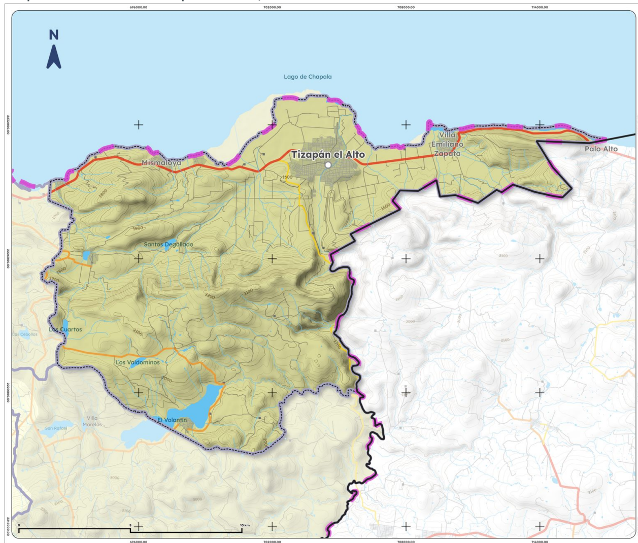
Mapa 6. Cuencas de Tizapán el Alto, 2023
