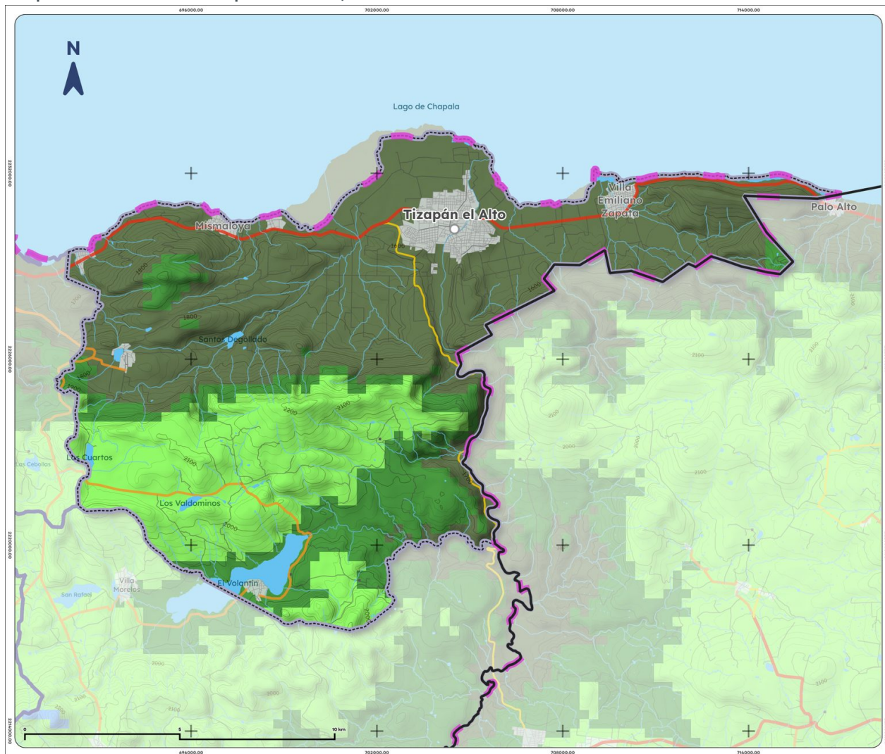
Mapa 10. Clima de Tizapán el Alto, 1995-2025
