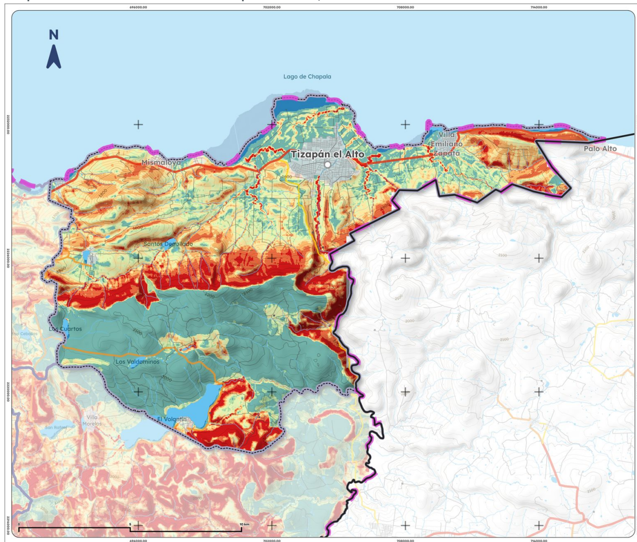
Mapa 17. Erosión efectiva de Tizapán el Alto, 2025
