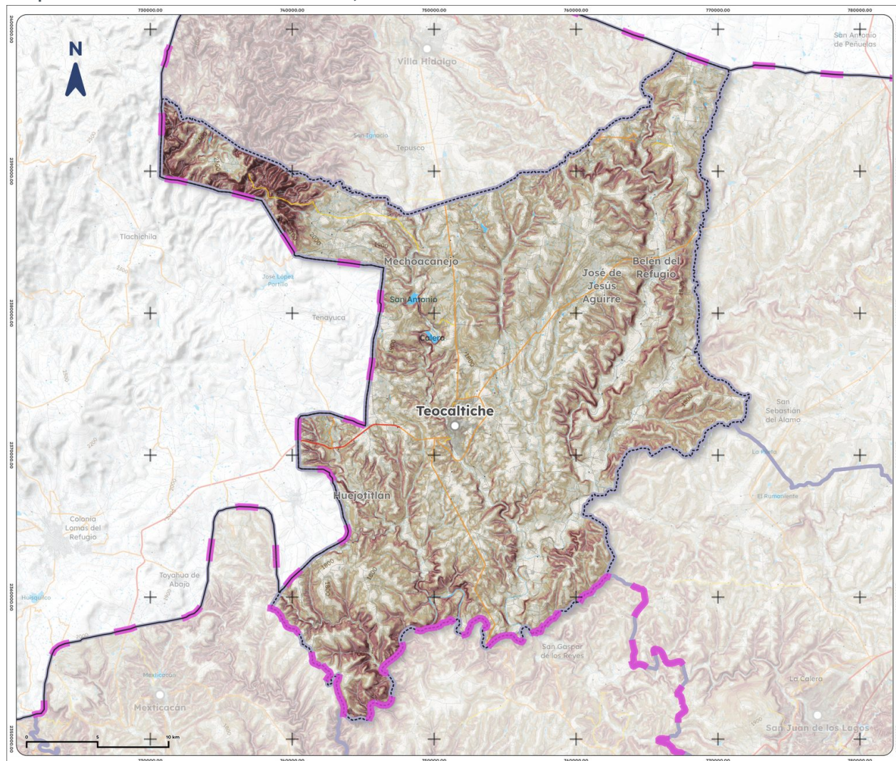
Mapa 5. Pendientes de Teocaltiche, 2025
