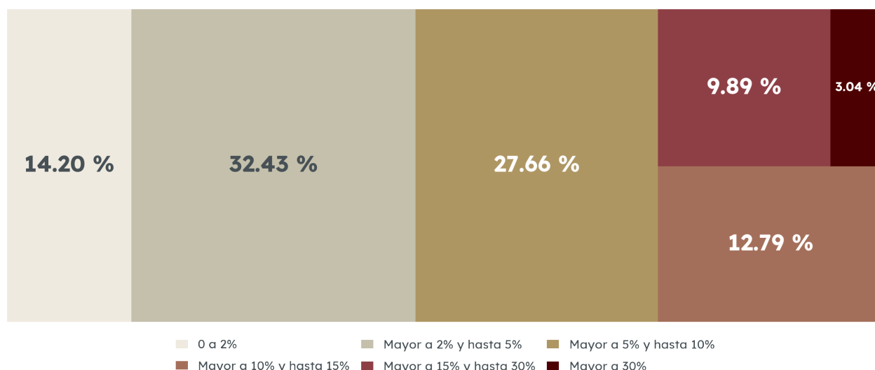
Topografía y pendientes de Teocaltiche, 2025
