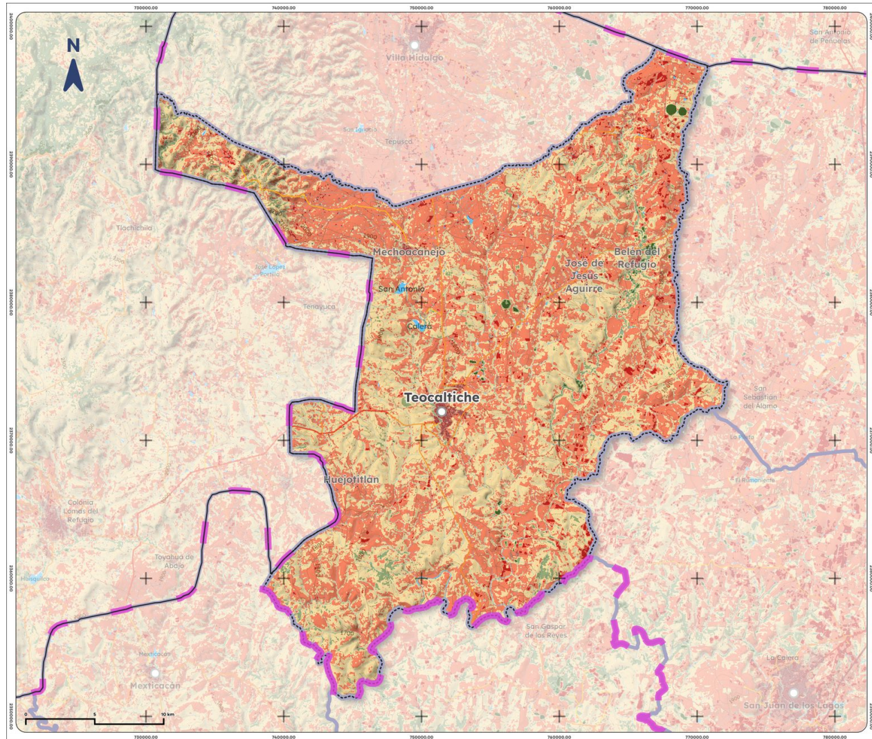
Mapa 12. NDVI promedio de Teocaltiche, 2025
