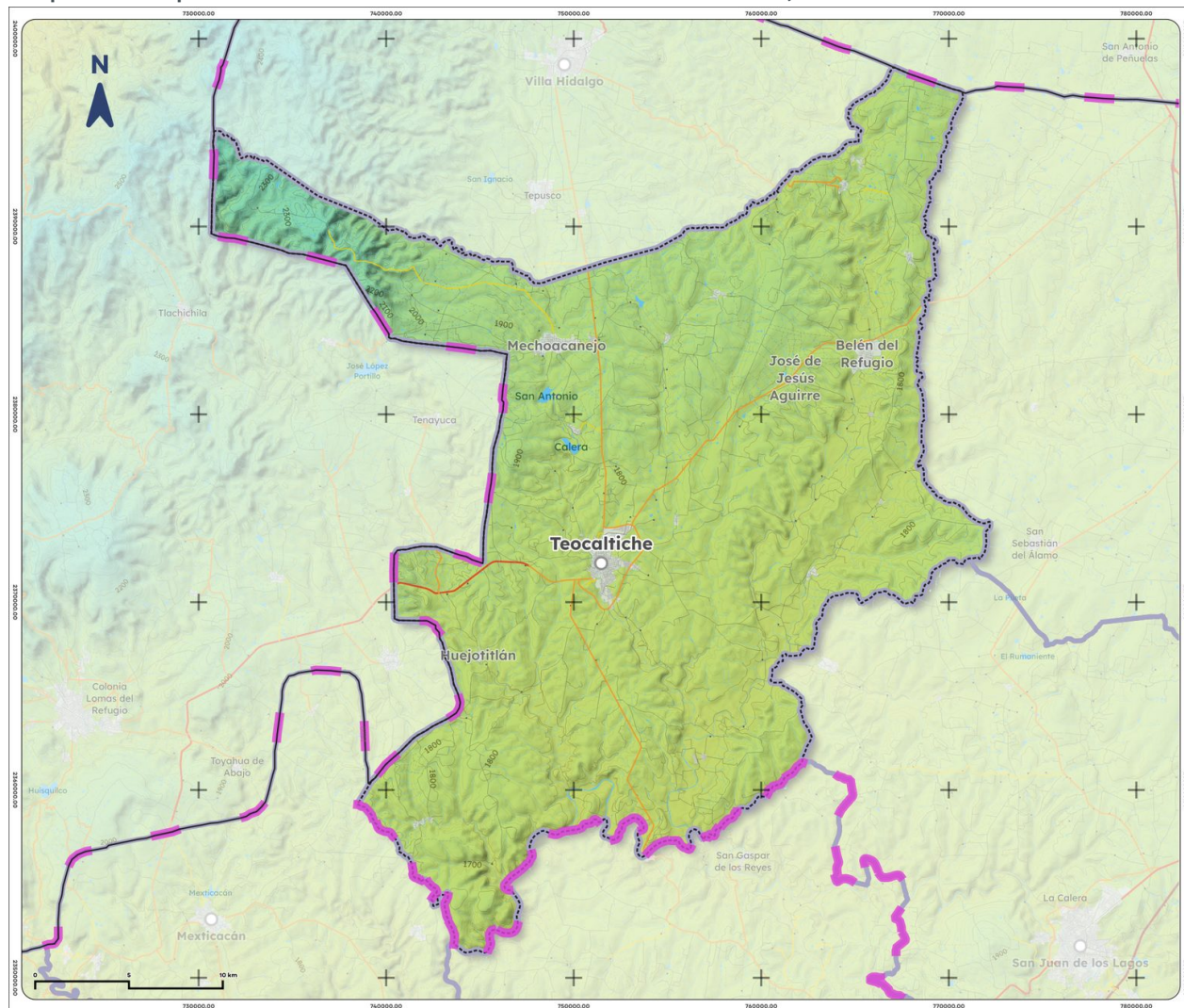
Mapa 8. Temperatura media anual histórica de Teocaltiche, 1995-2025
