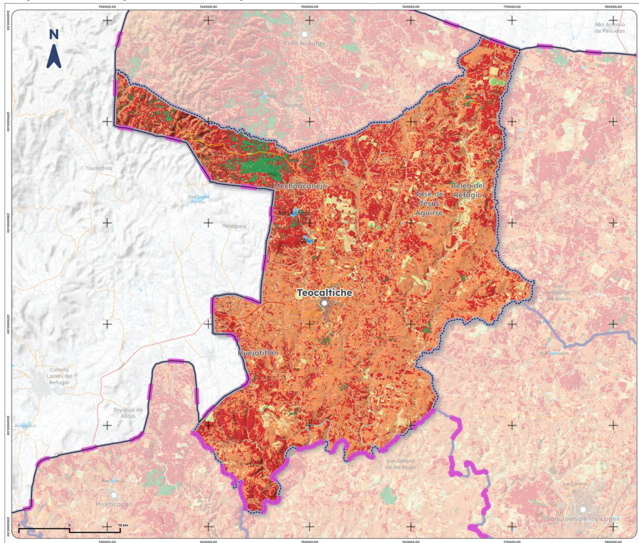
Mapa 15. Índice promedio de sequía de Teocaltiche, 2025
