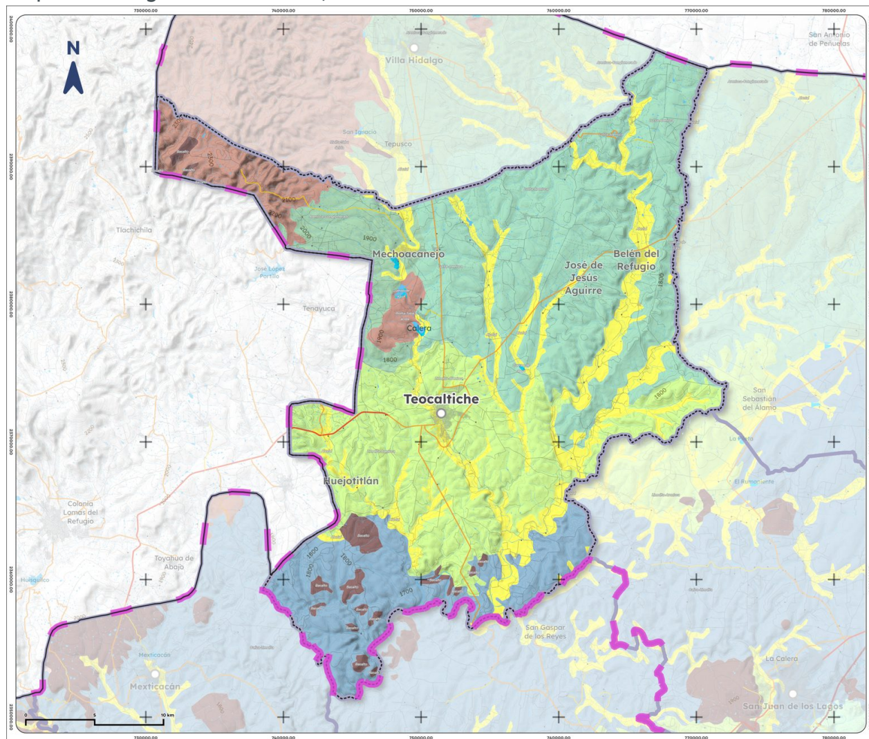
Mapa 3. Geología de Teocaltiche, 1988
