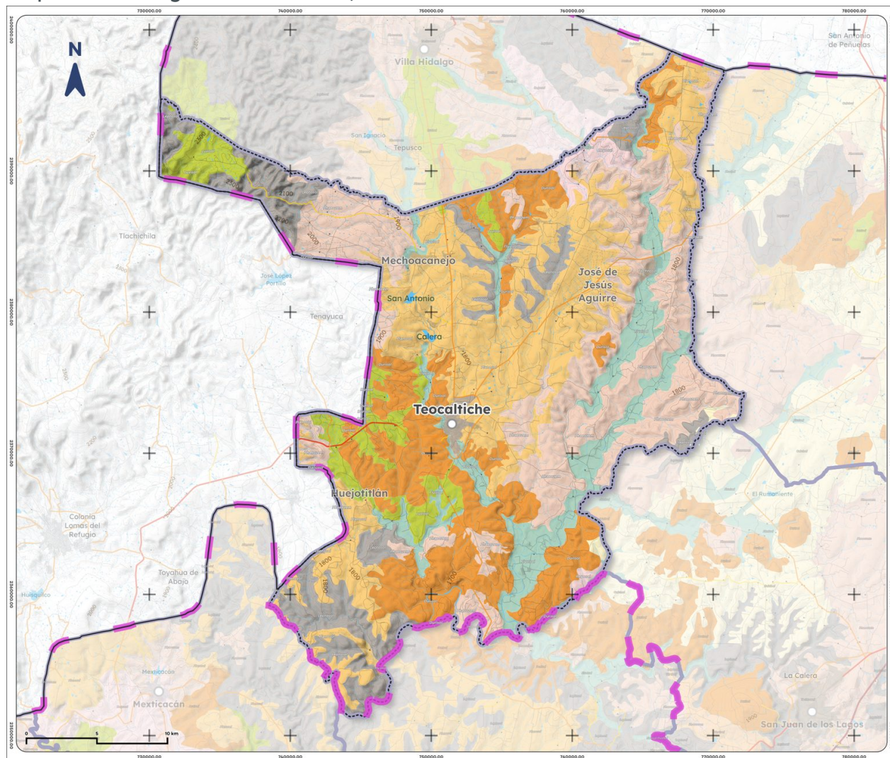
Mapa 4. Edafología de Teocaltiche, 2025
