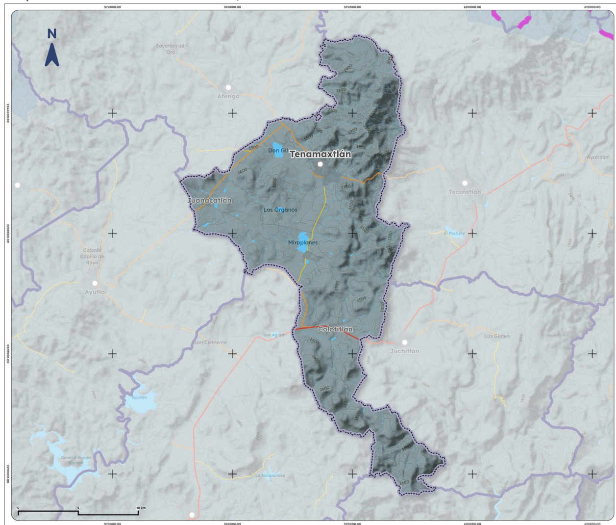
Mapa 6. Cuencas de Tenamaxtlán, 2023
