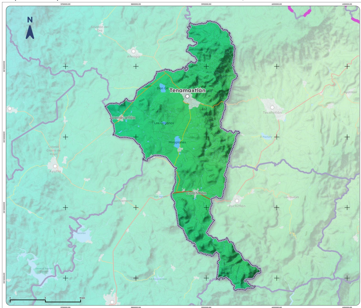
Mapa 9. Precipitación histórica acumulada de Tenamaxtlán, 1995-2025
