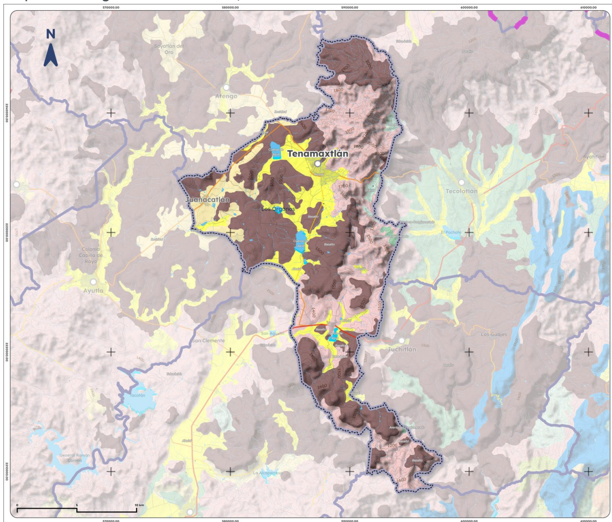
Mapa 3. Geología de Tenamaxtlán, 1988
