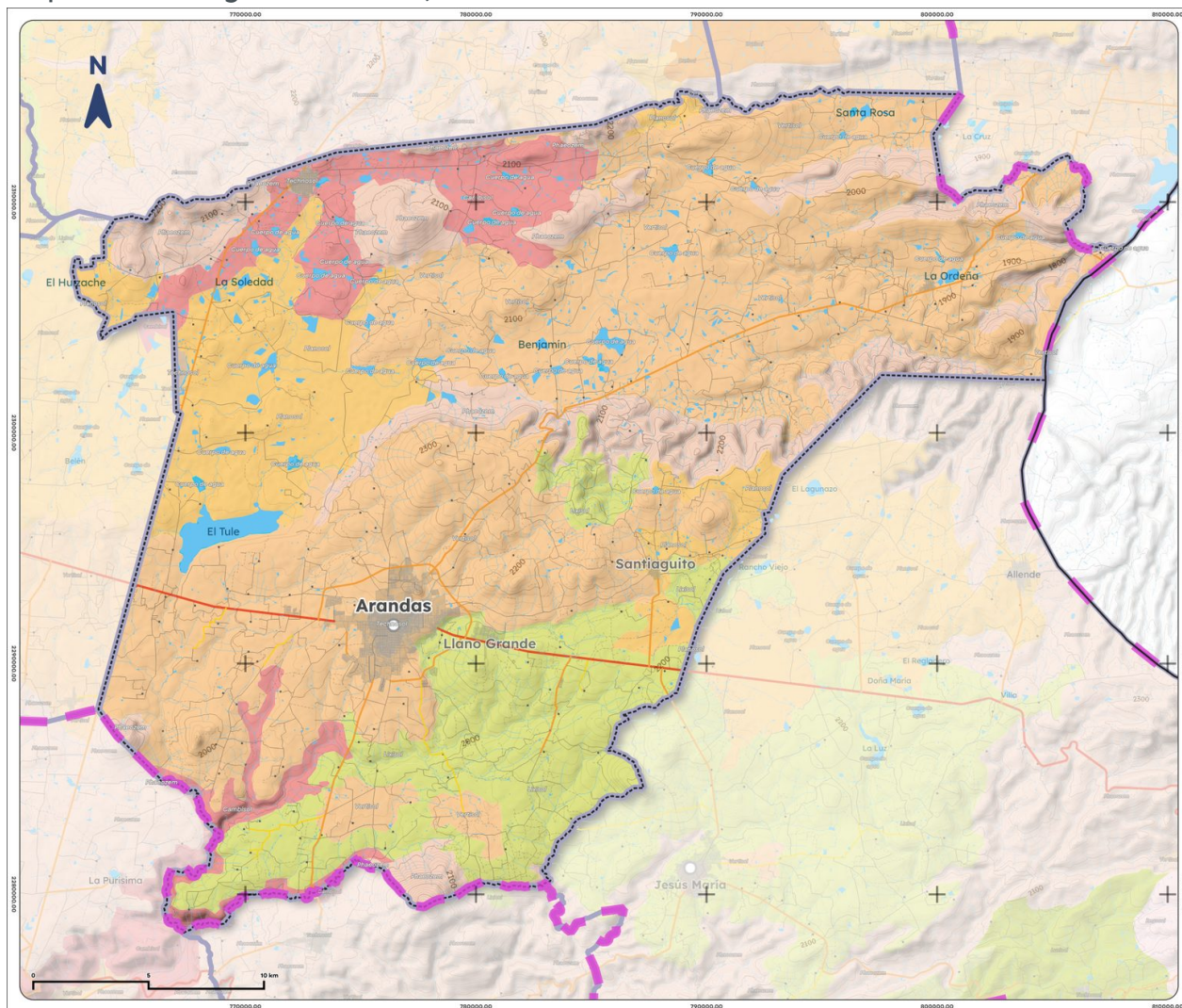
Mapa 4. Edafología de Arandas, 2025
