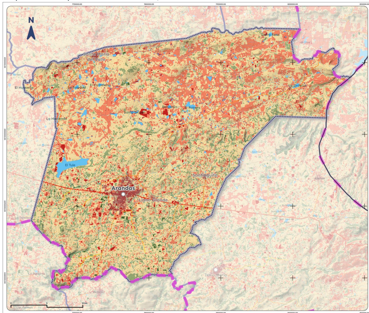
Mapa 12. NDVI promedio de Arandas, 2025
