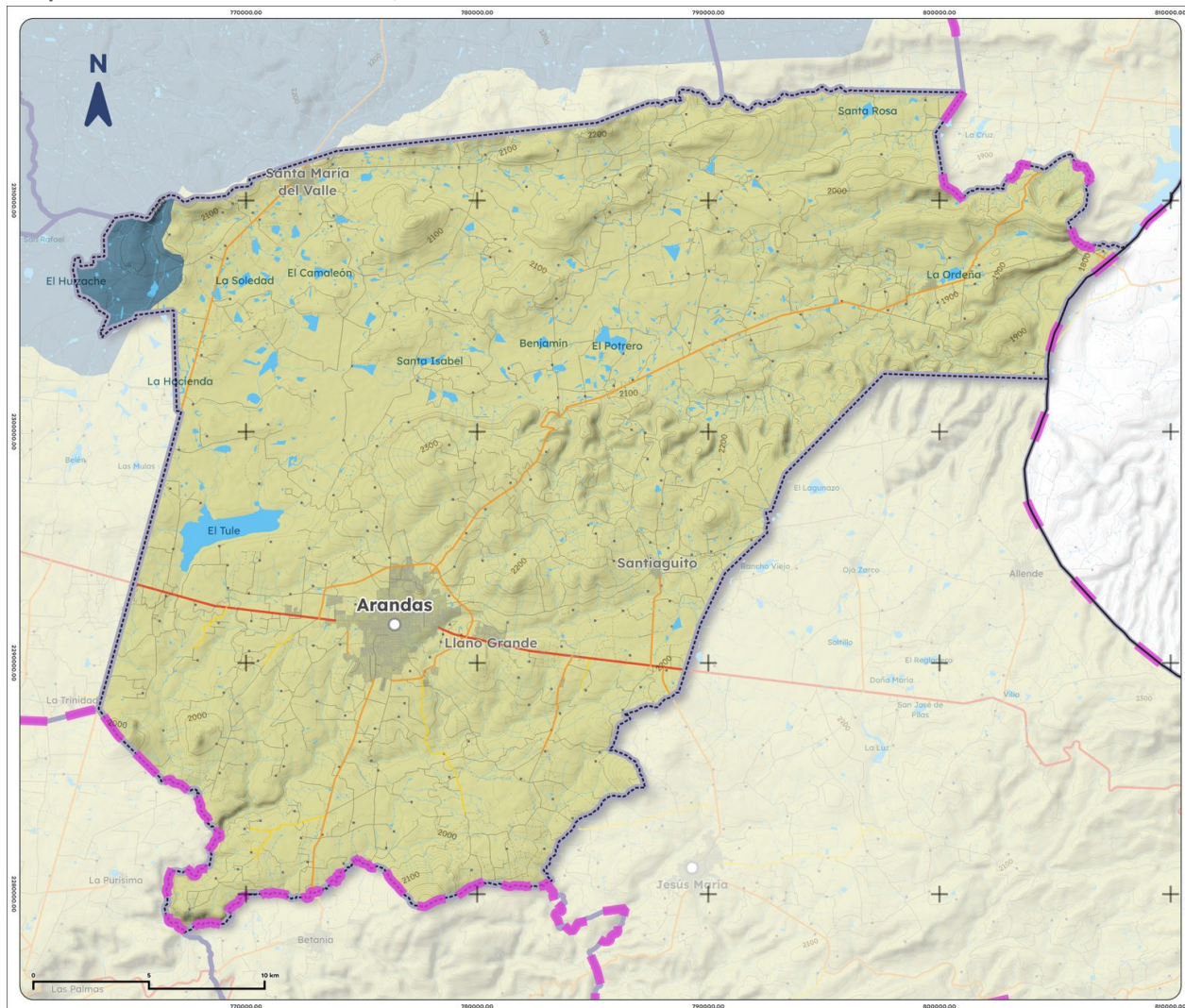
Mapa 6. Cuencas de Arandas, 2023
