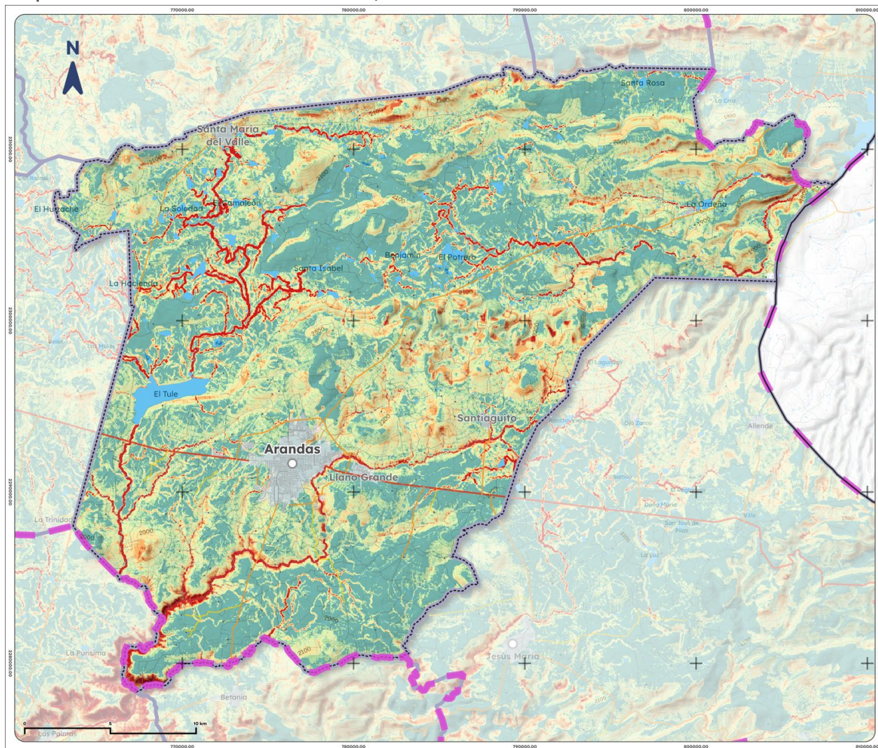
Mapa 17. Erosión efectiva de Arandas, 2025
