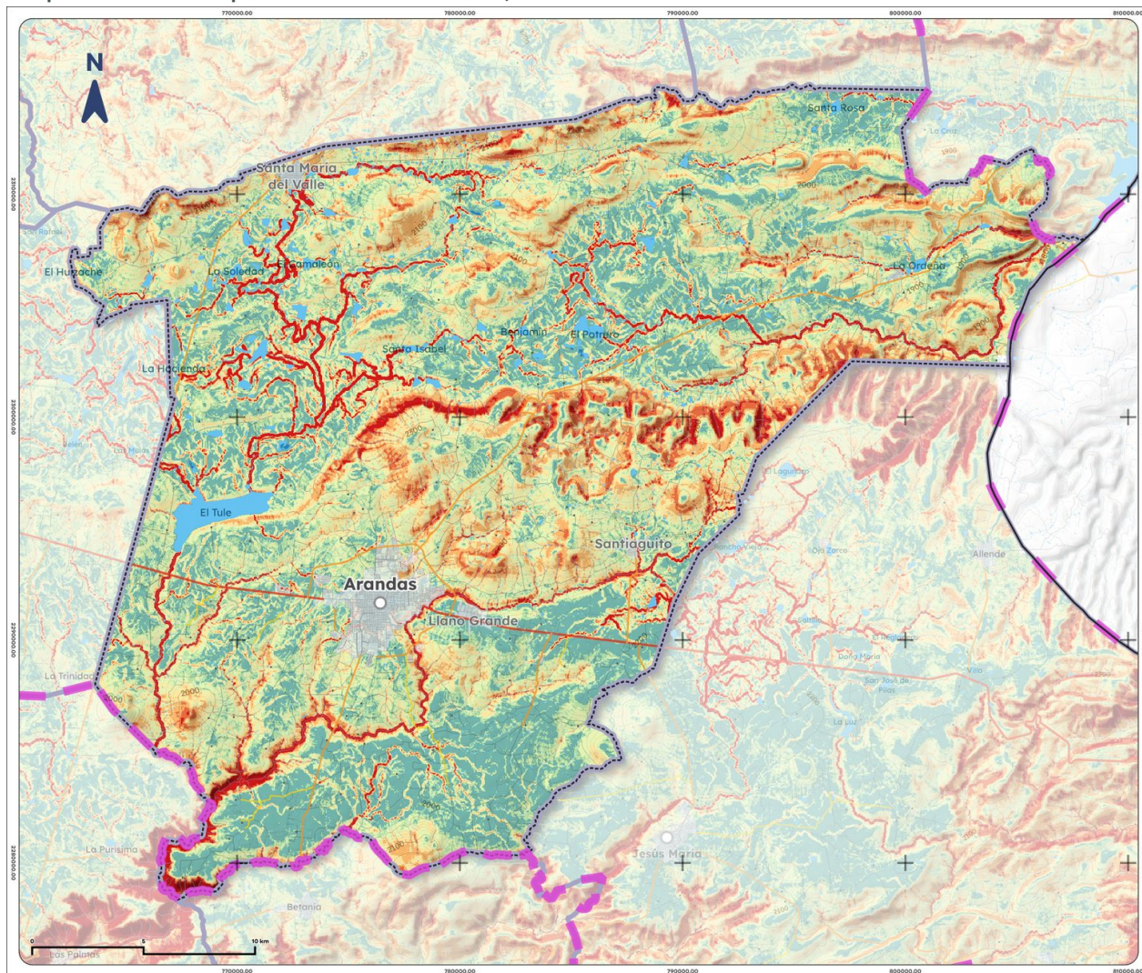
Mapa 16. Erosión potencial de Arandas, 2025
