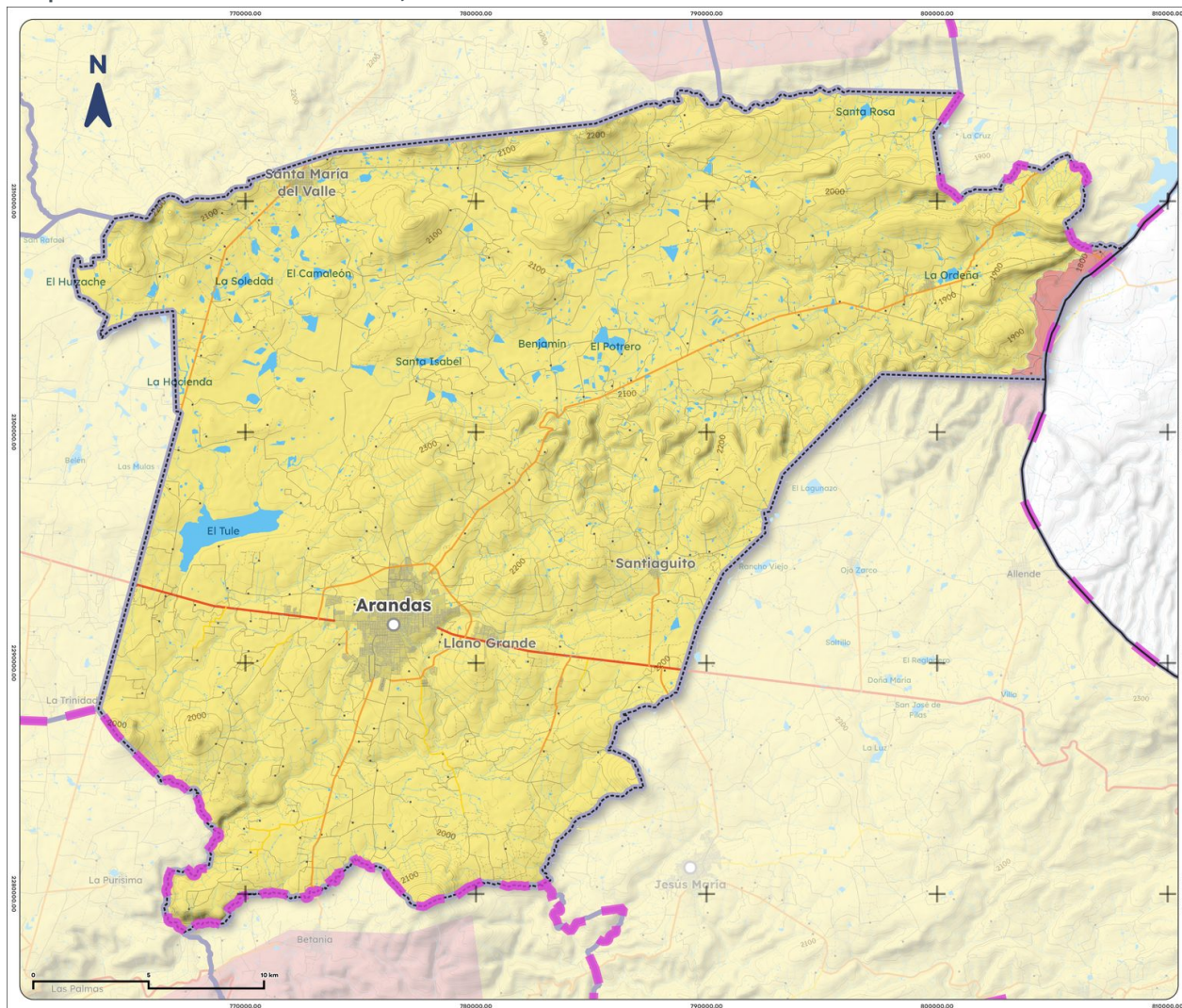
Mapa 7. Acuíferos de Arandas, 2023
