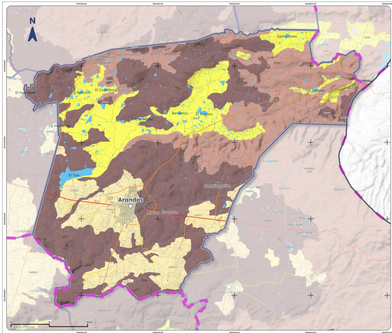
Mapa 3. Geología de Arandas, 1988
