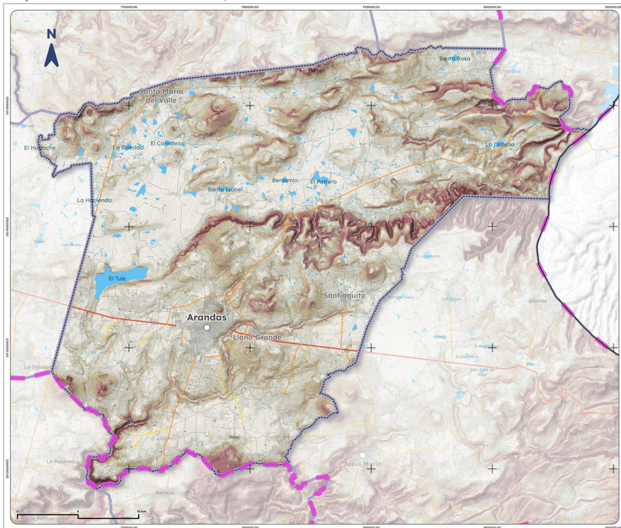
Mapa 5. Pendientes de Arandas, 2025
