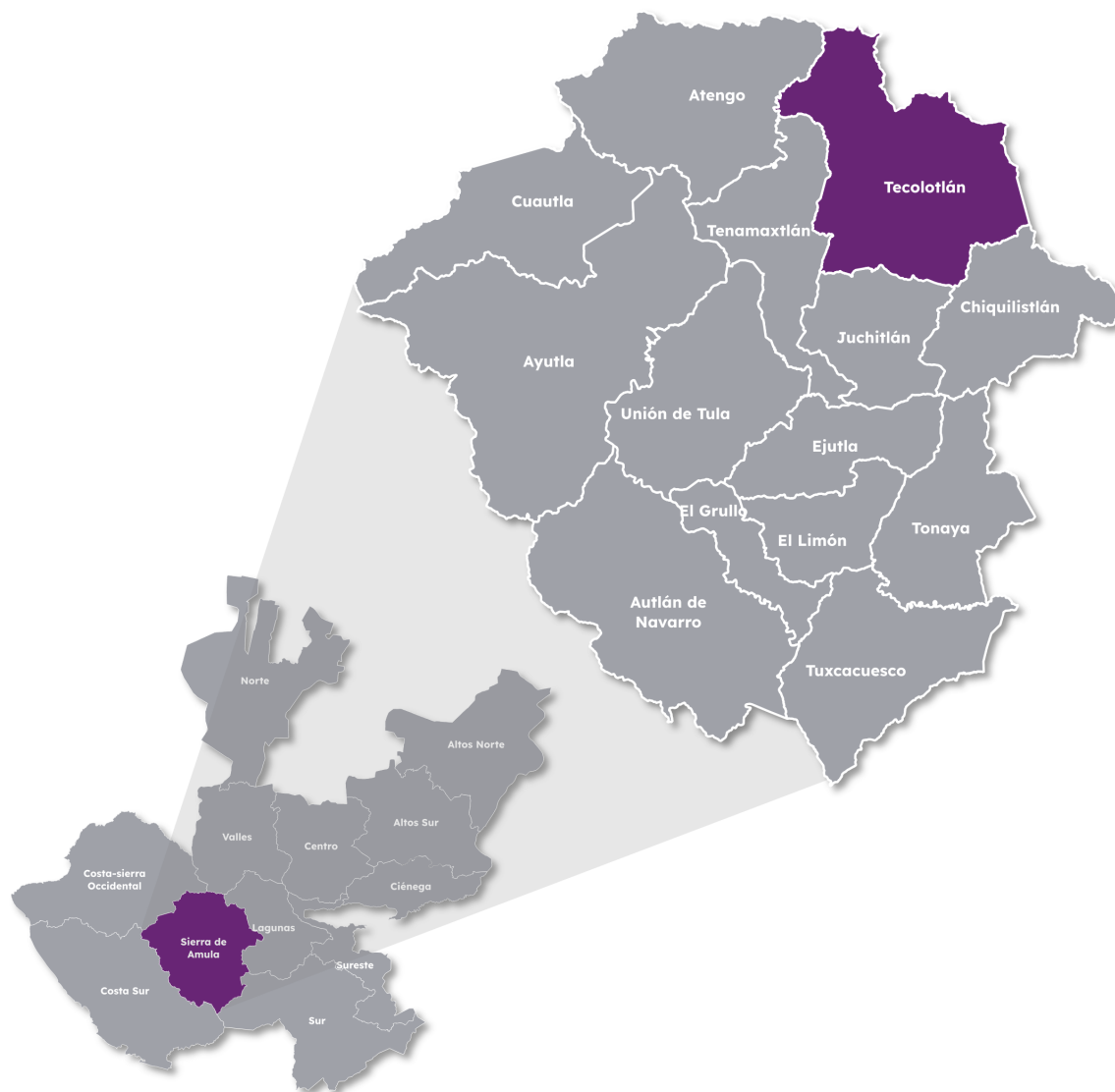
Mapa 1. Localización geográfica de Tecolotlán, Jalisco
