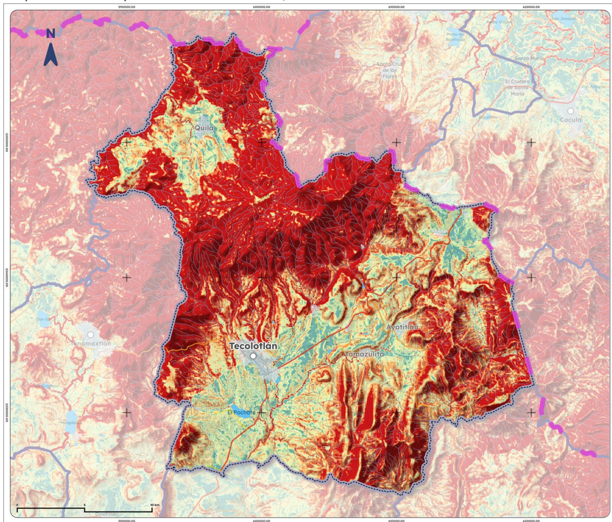
Mapa 16. Erosión potencial de Tecolotlán, 2025
