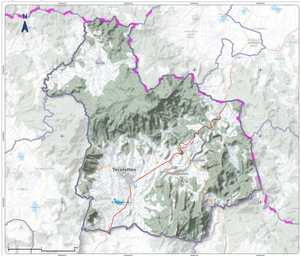
Mapa 2. Mapa base de Tecolotlán, 2025
