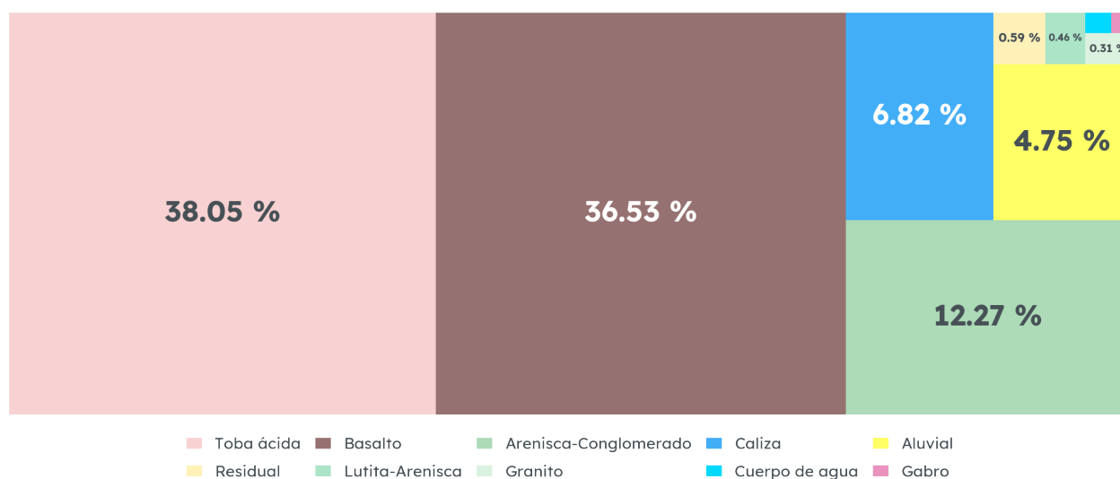
Geología de Tecolotlán, 1988
