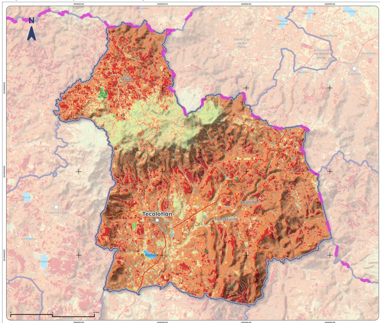
Mapa 15. Índice promedio de sequía de Tecolotlán, 2025
