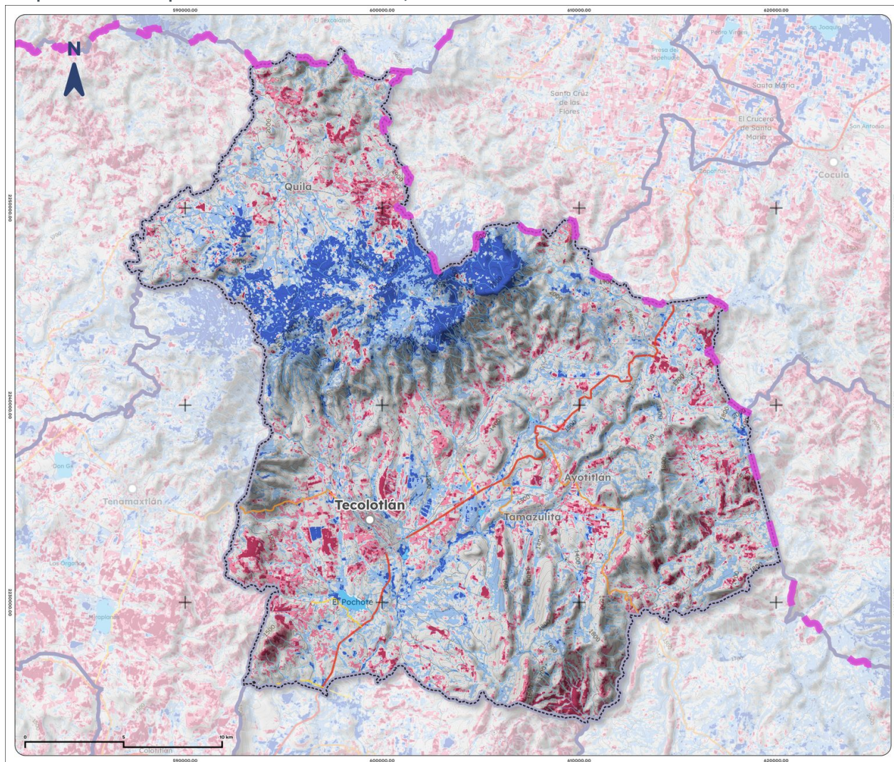
Mapa 13. NDWI promedio de Tecolotlán, 2025
