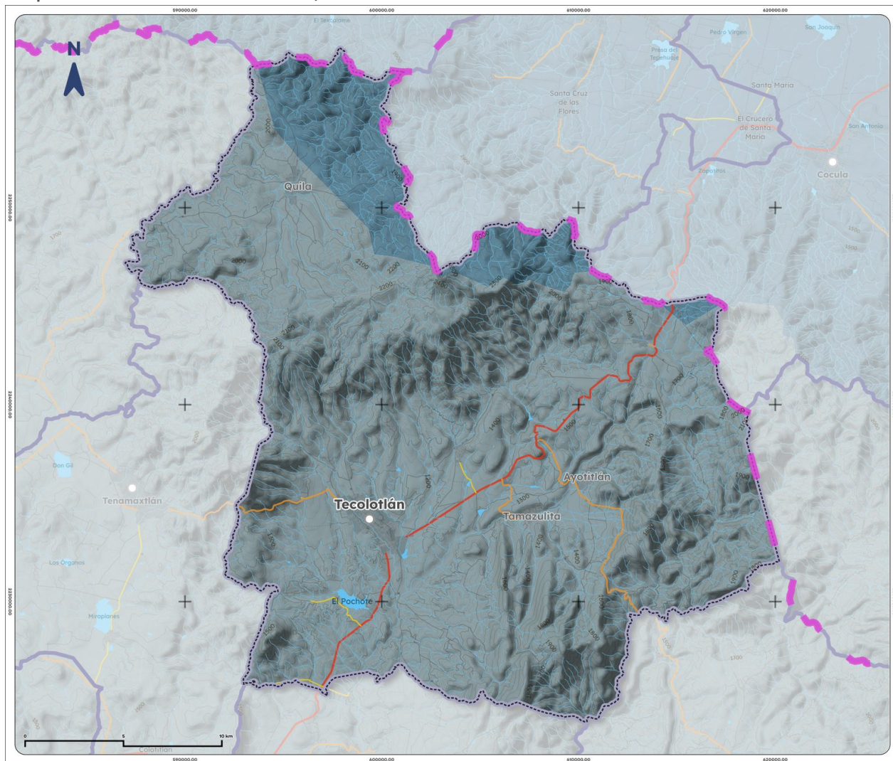
Mapa 6. Cuencas de Tecolotlán, 2023
