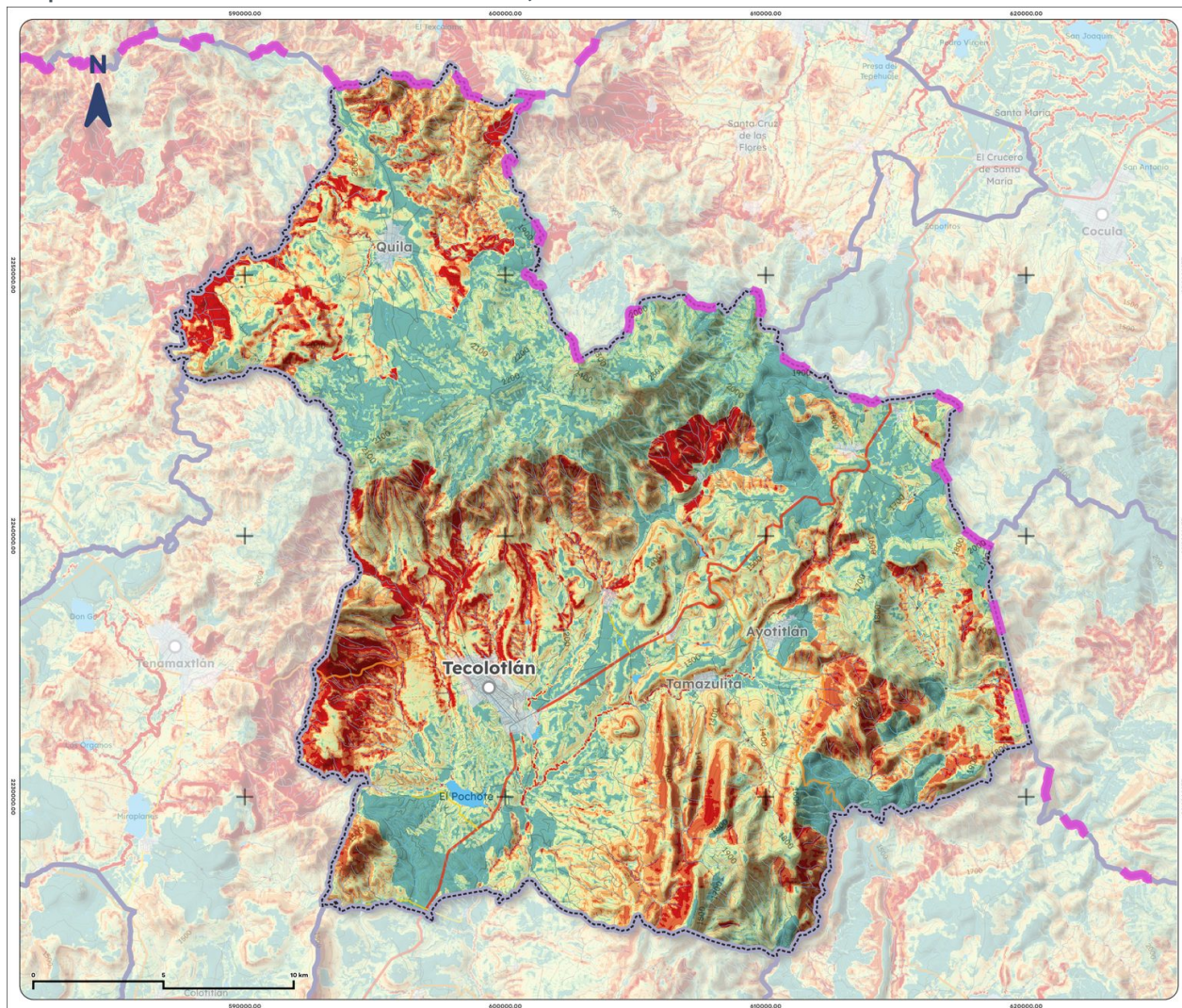
Mapa 17. Erosión efectiva de Tecolotlán, 2025
