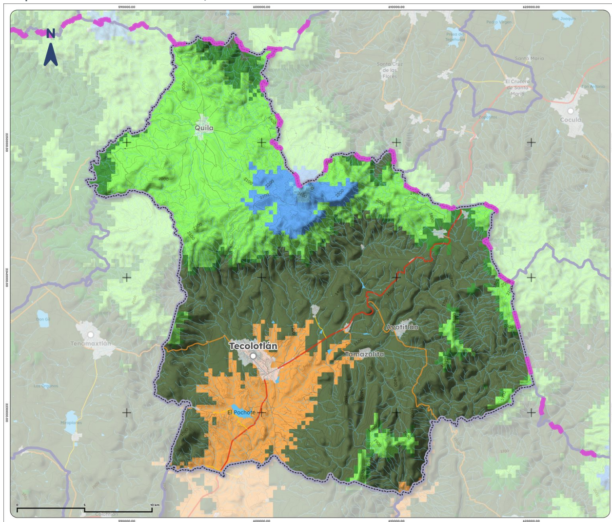
Mapa 10. Clima de Tecolotlán, 1995-2025
