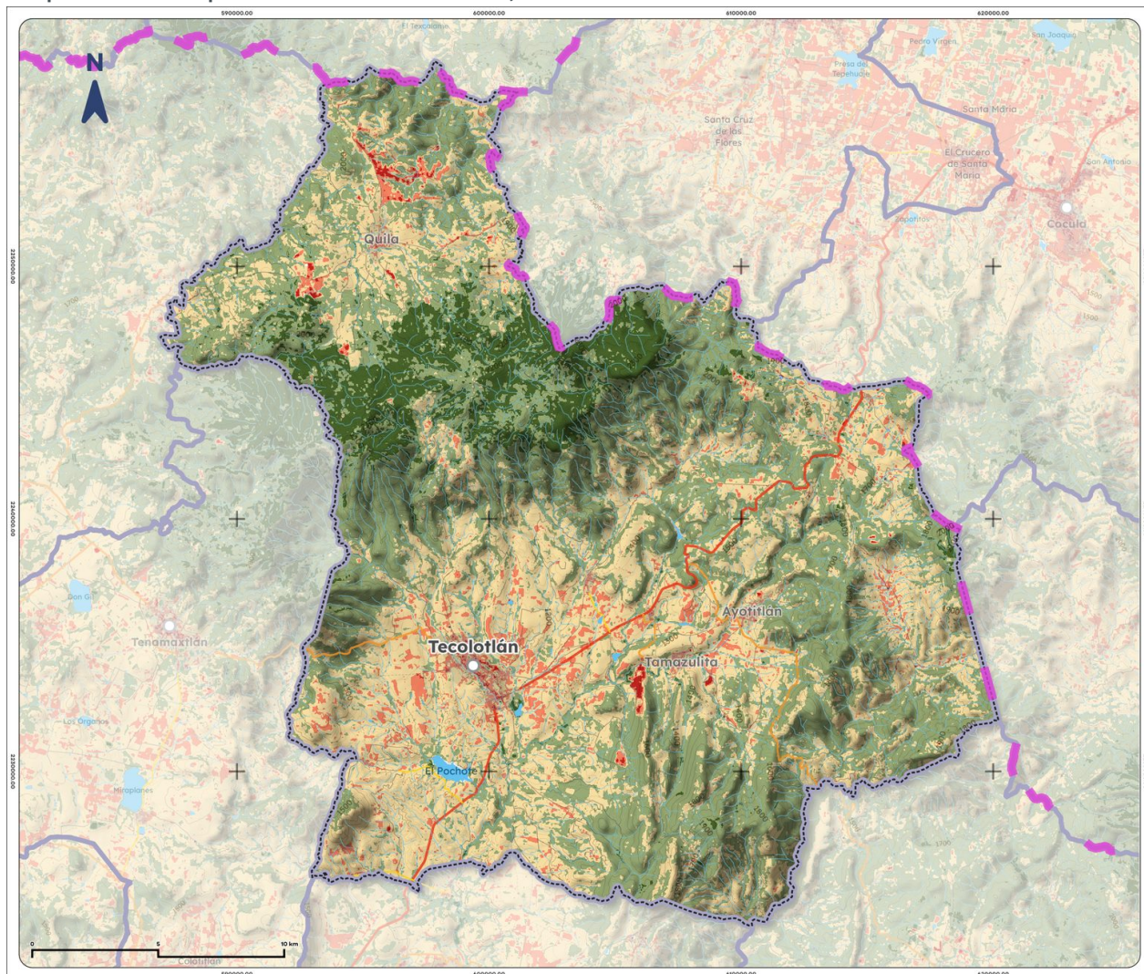
Mapa 12. NDVI promedio de Tecolotlán, 2025
