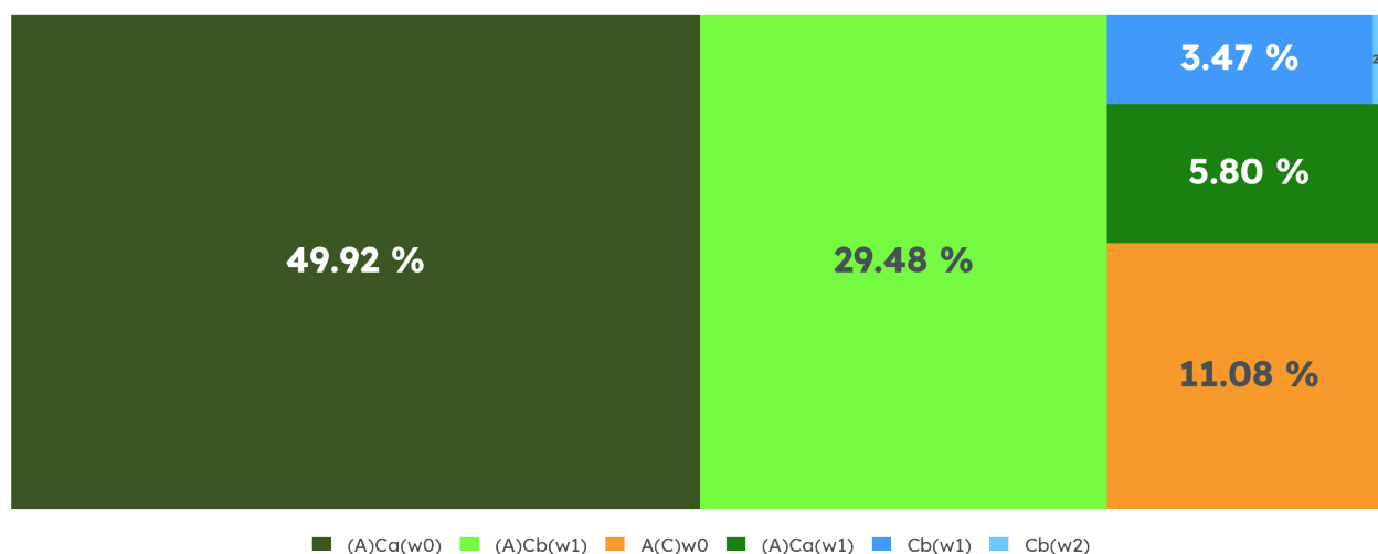
Clima de Tecolotlán, 1995-2025
