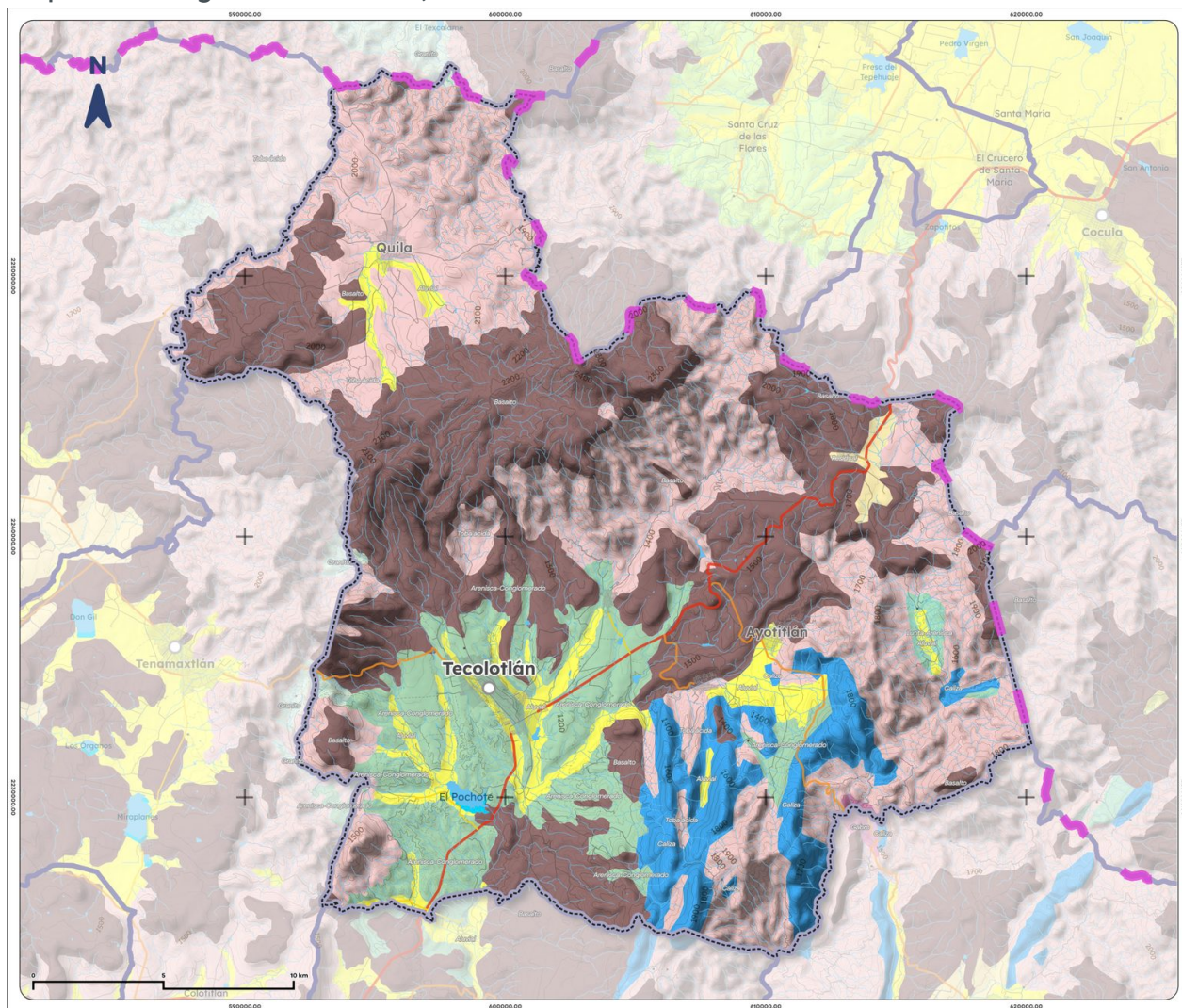
Mapa 3. Geología de Tecolotlán, 1988
