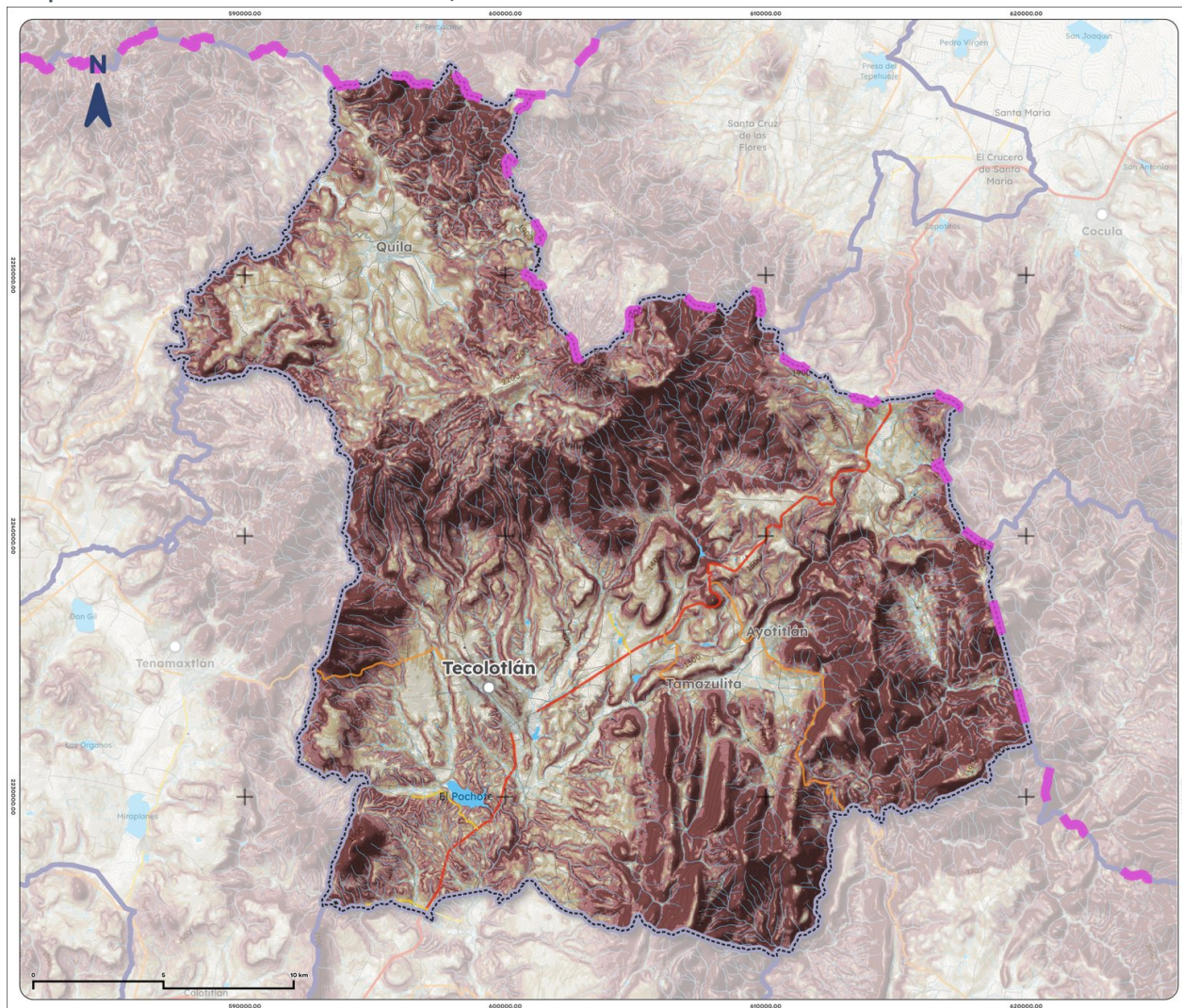
Mapa 5. Pendientes de Tecolotlán, 2025
