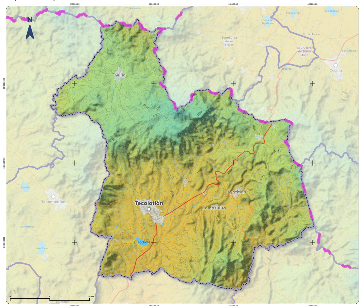
Mapa 8. Temperatura media anual histórica de Tecolotlán, 1995-2025
