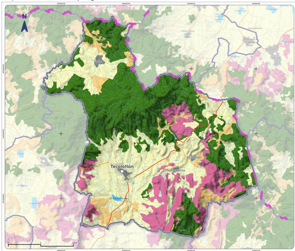
Mapa 11. Uso de suelo y vegetación de Tecolotlán, 2018
