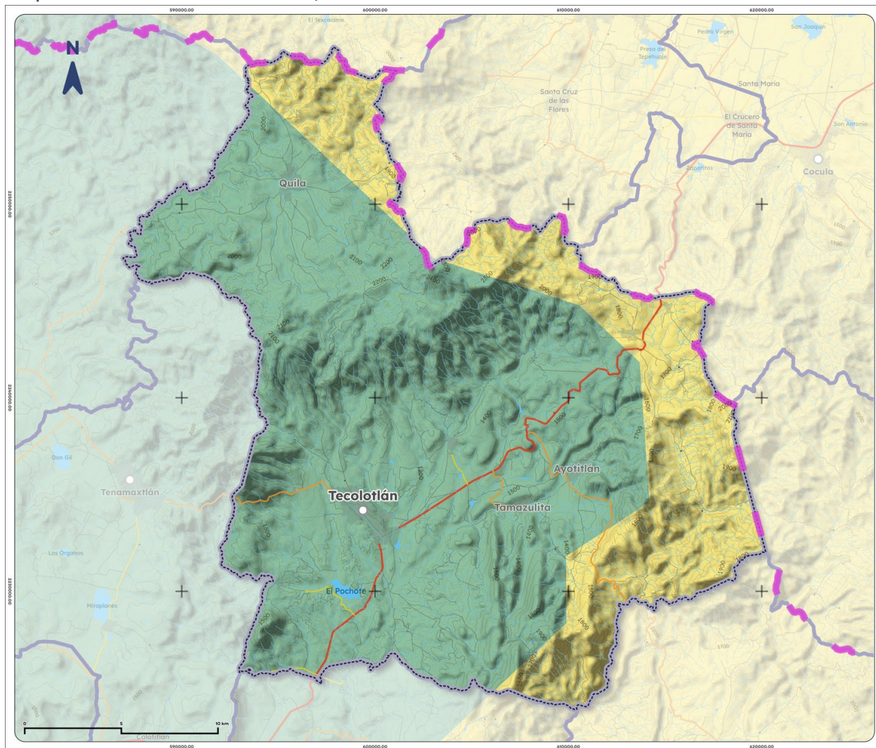
Mapa 7. Acuíferos de Tecolotlán, 2023
