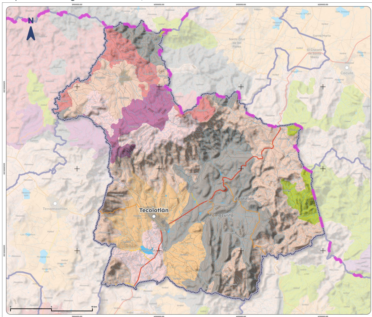
Mapa 4. Edafología de Tecolotlán, 2025
