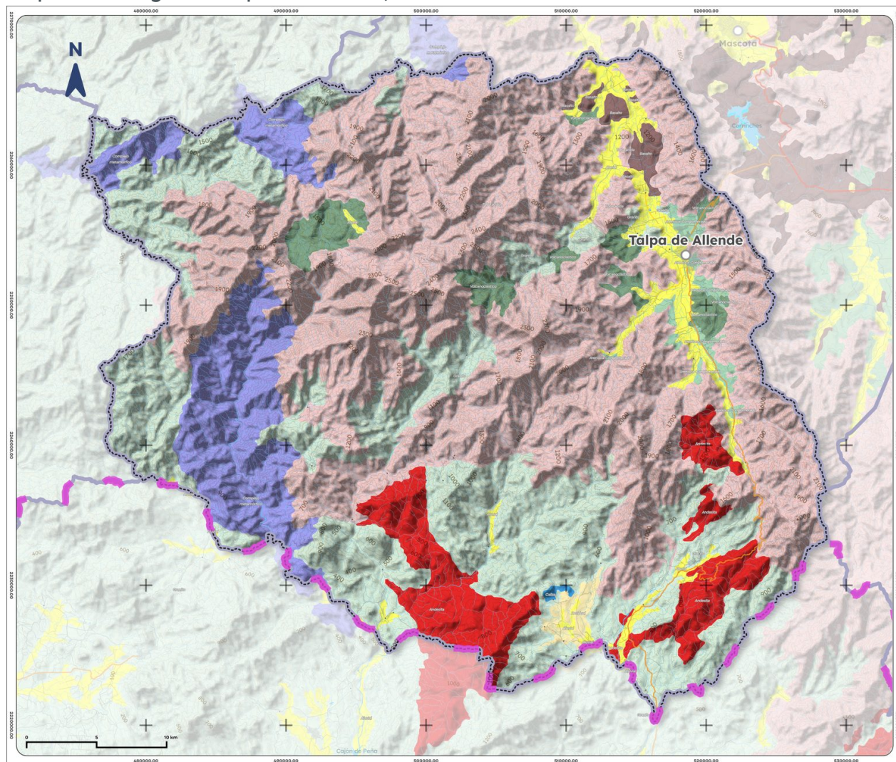
Mapa 3. Geología de Talpa de Allende, 1988
