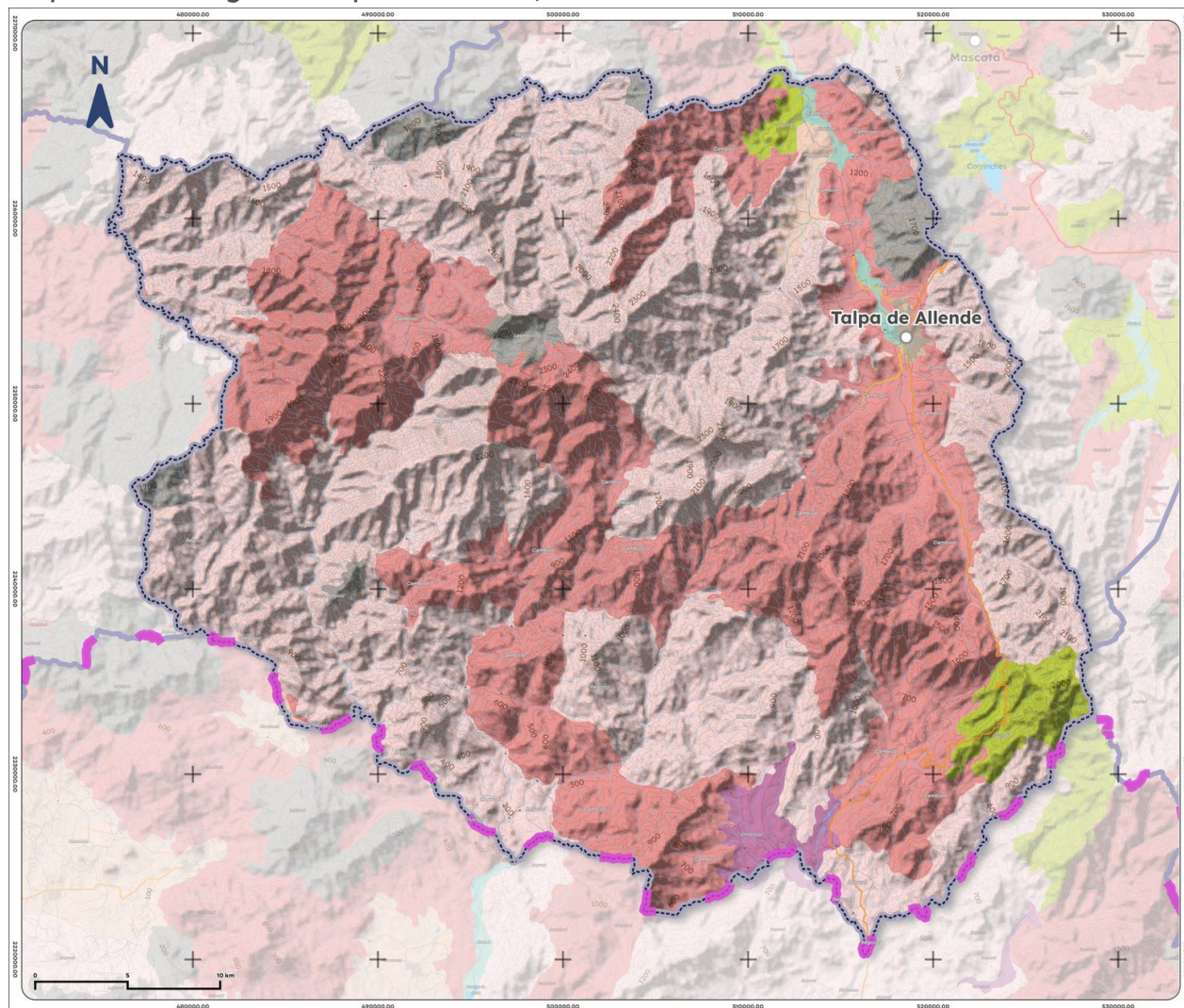
Mapa 4. Edafología de Talpa de Allende, 2025
