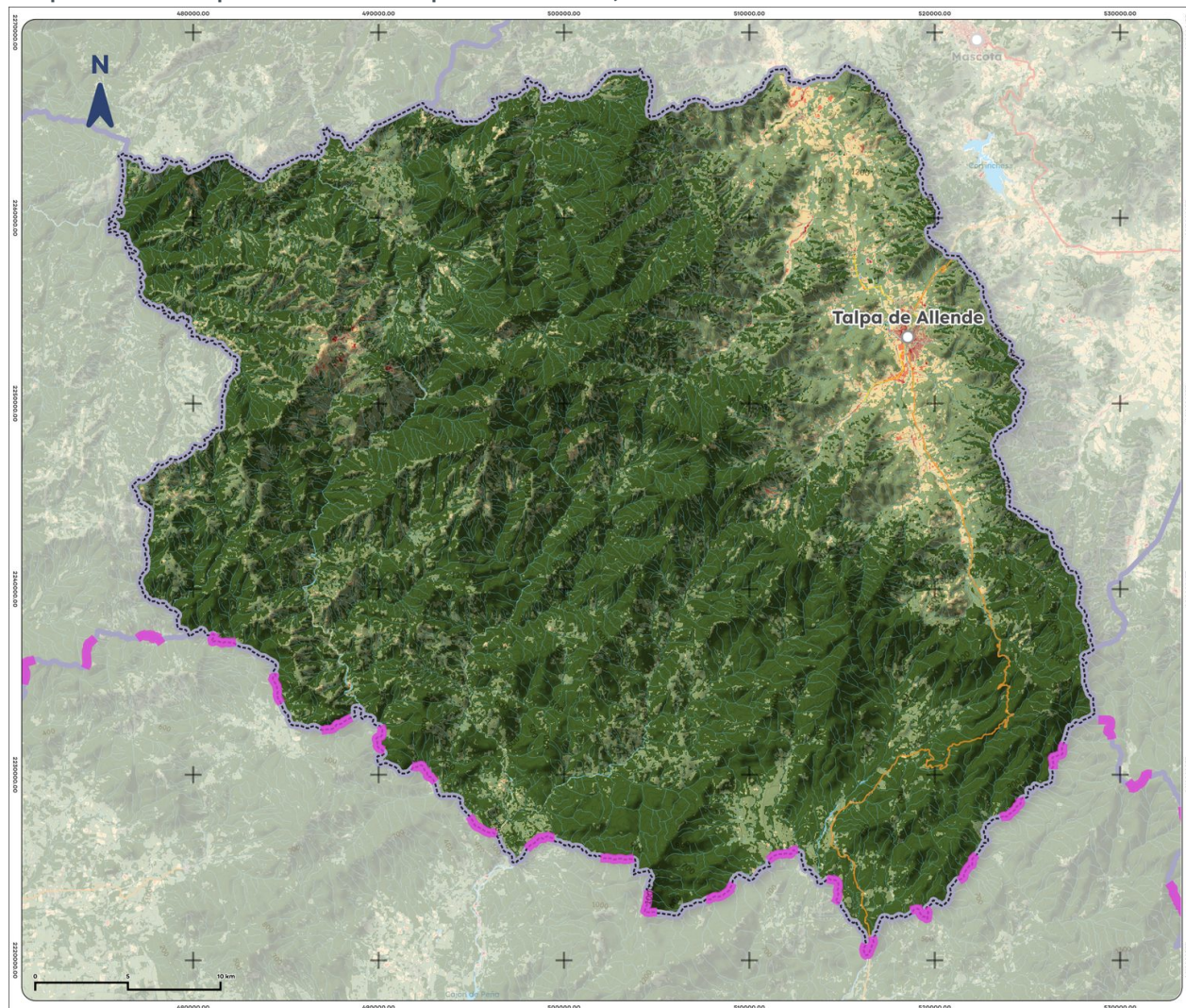
Mapa 12. NDVI promedio de Talpa de Allende, 2025
