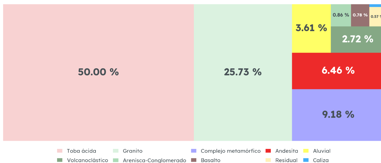
Geología de Talpa de Allende, 1988
