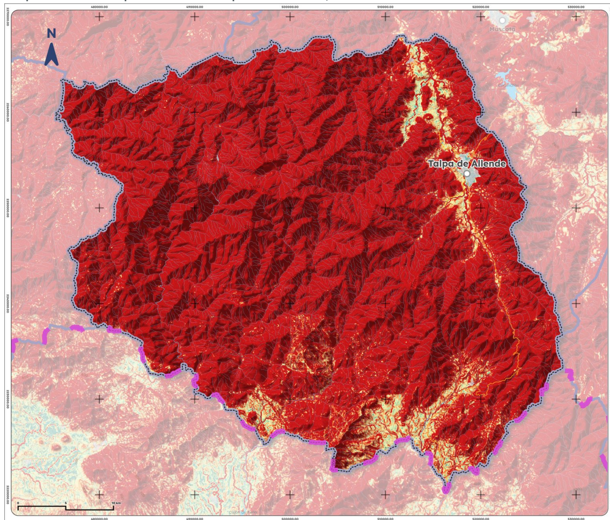
Mapa 16. Erosión potencial de Talpa de Allende, 2025
