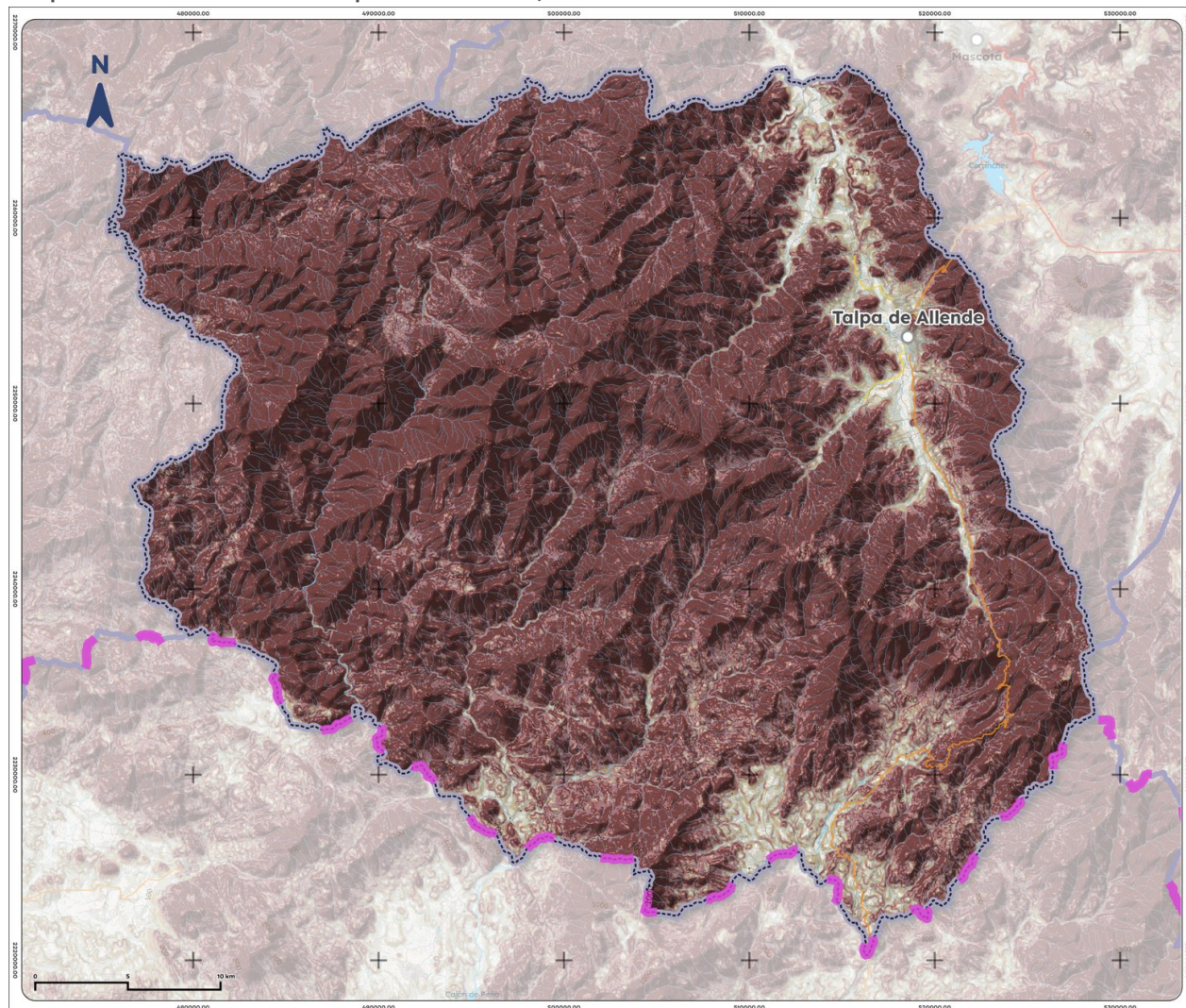
Mapa 5. Pendientes de Talpa de Allende, 2025
