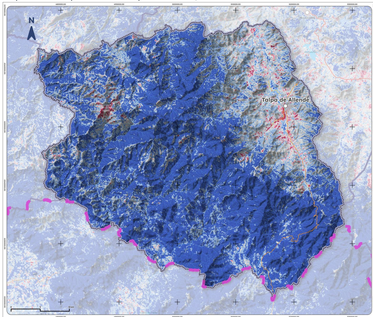
Mapa 13. NDWI promedio de Talpa de Allende, 2025
