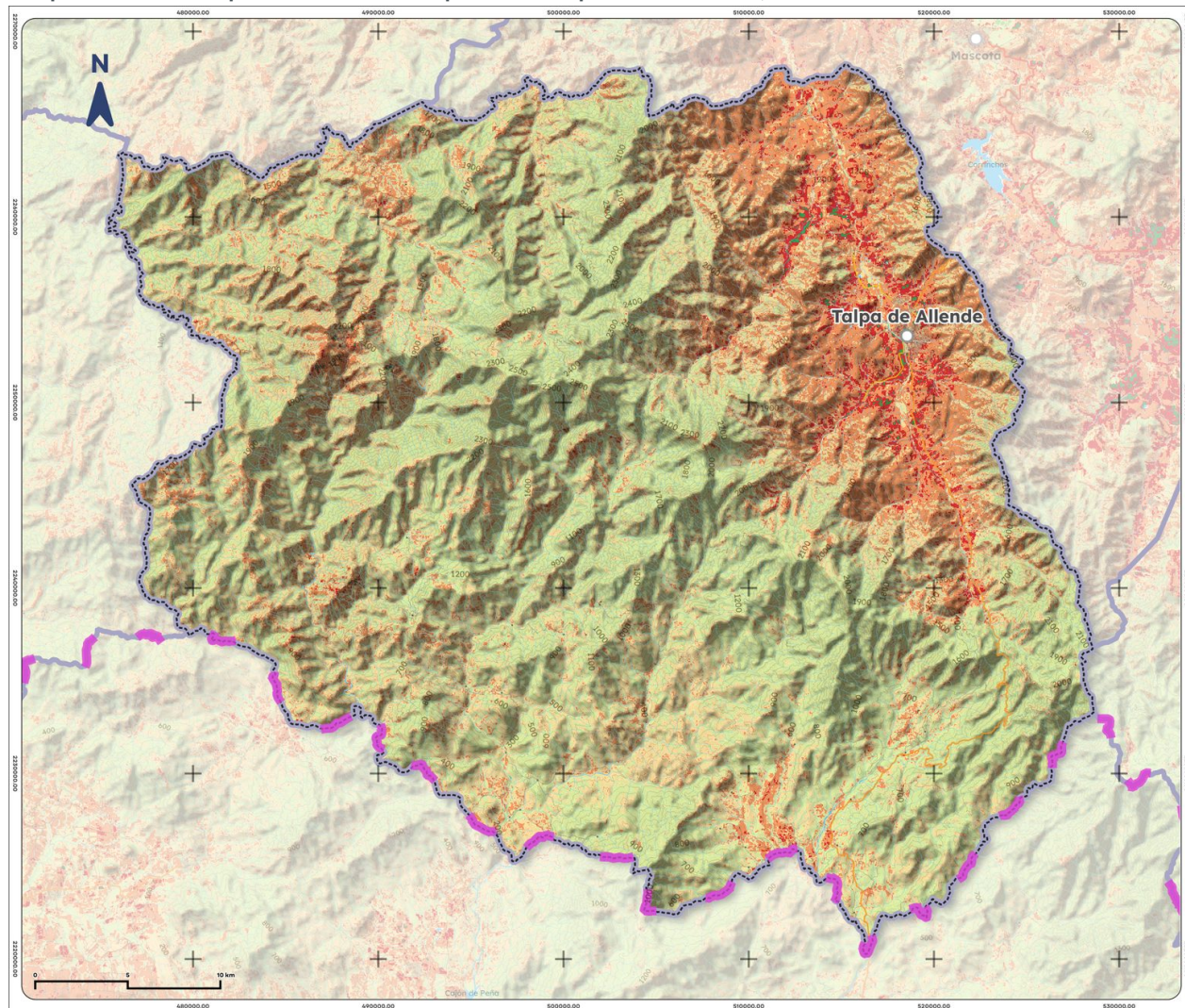
Mapa 15. Índice promedio de sequía de Talpa de Allende, 2025
