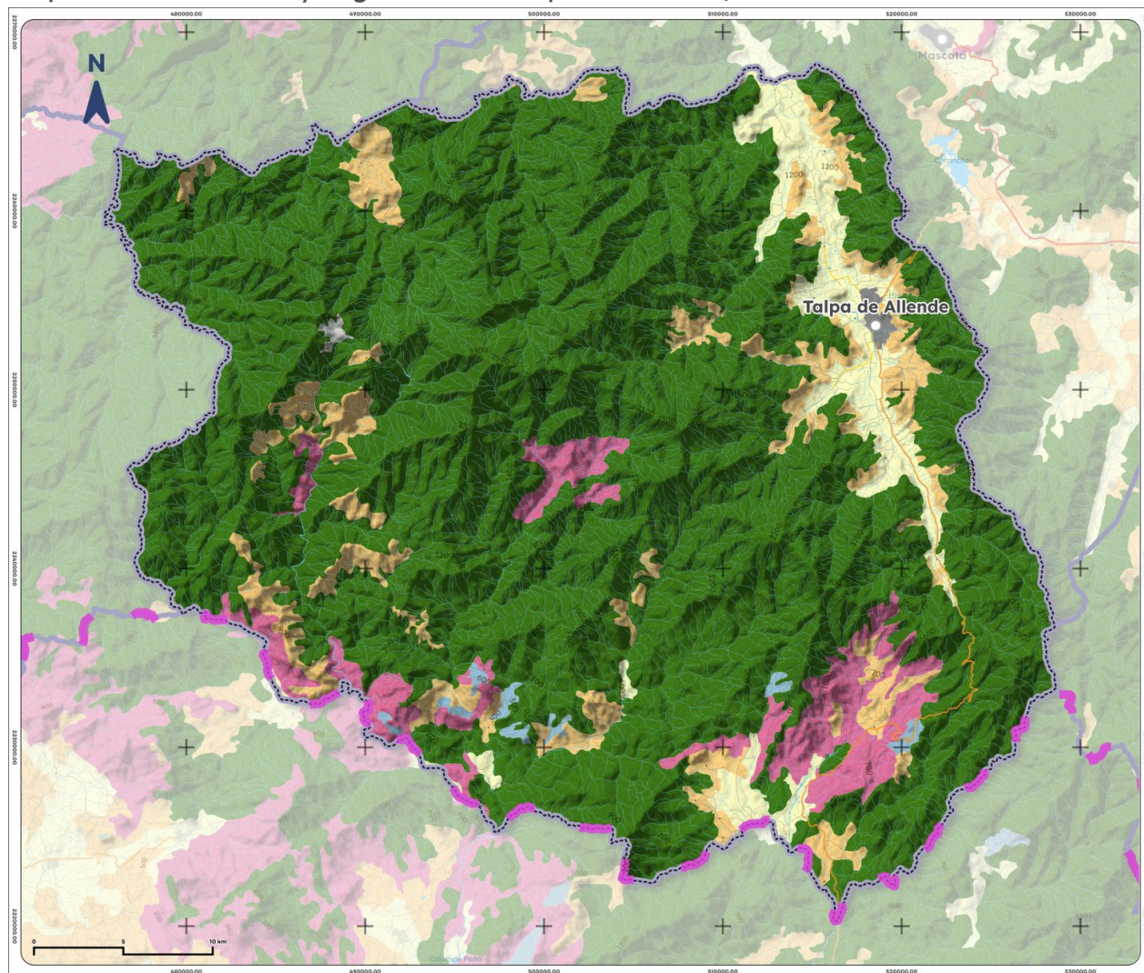
Mapa 11. Uso de suelo y vegetación de Talpa de Allende, 2018
