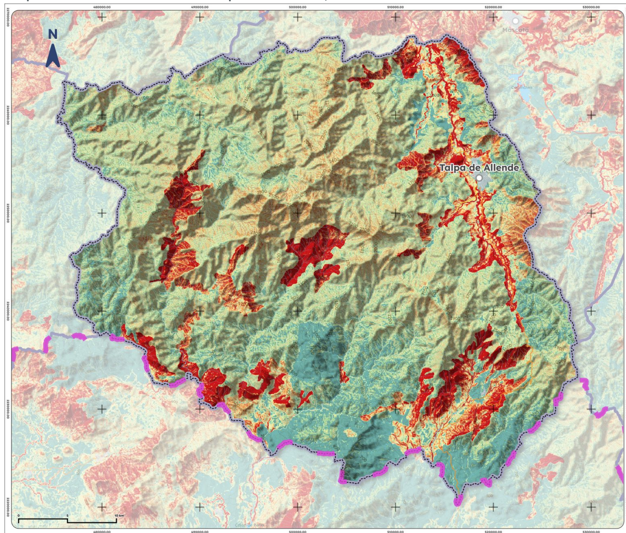
Mapa 17. Erosión efectiva de Talpa de Allende, 2025
