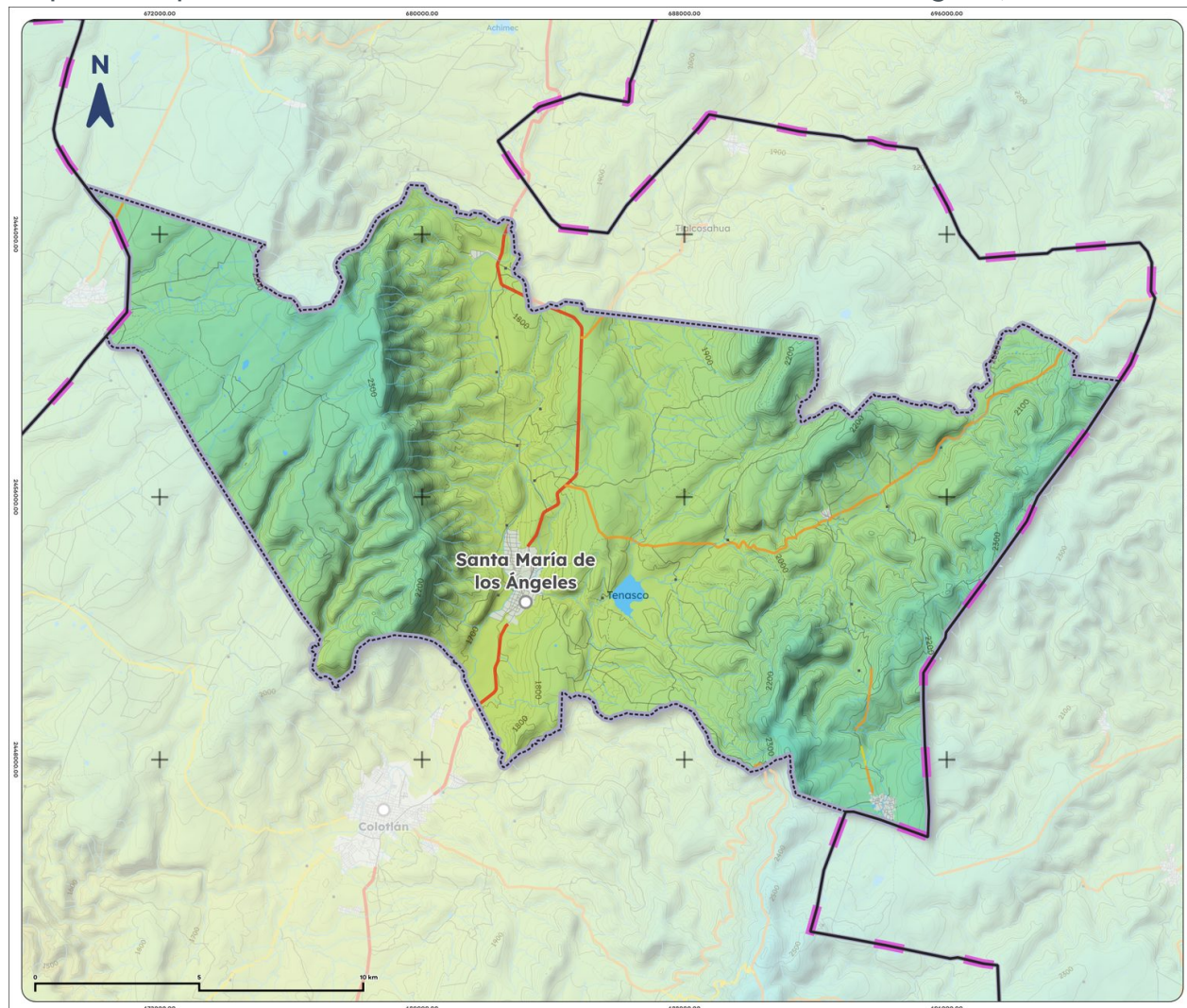
Mapa 8. Temperatura media anual histórica de Santa María de los Ángeles, 1995-2025
