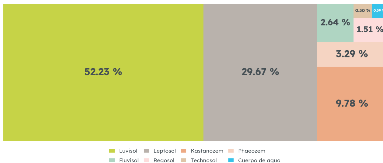
Edafología de Santa María de los Ángeles, 2025
