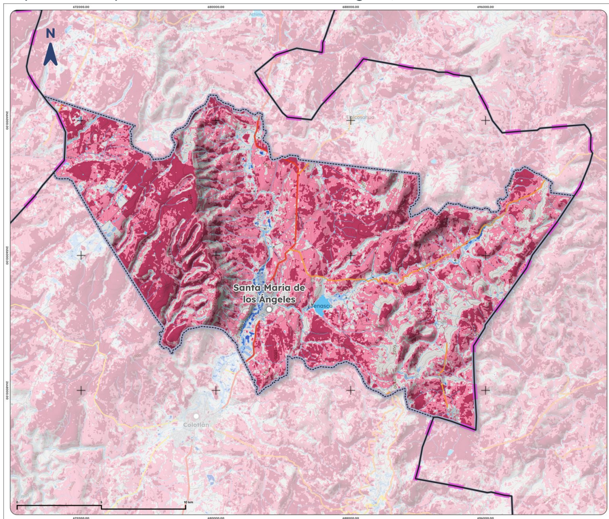
Mapa 13. NDWI promedio de Santa María de los Ángeles, 2025
