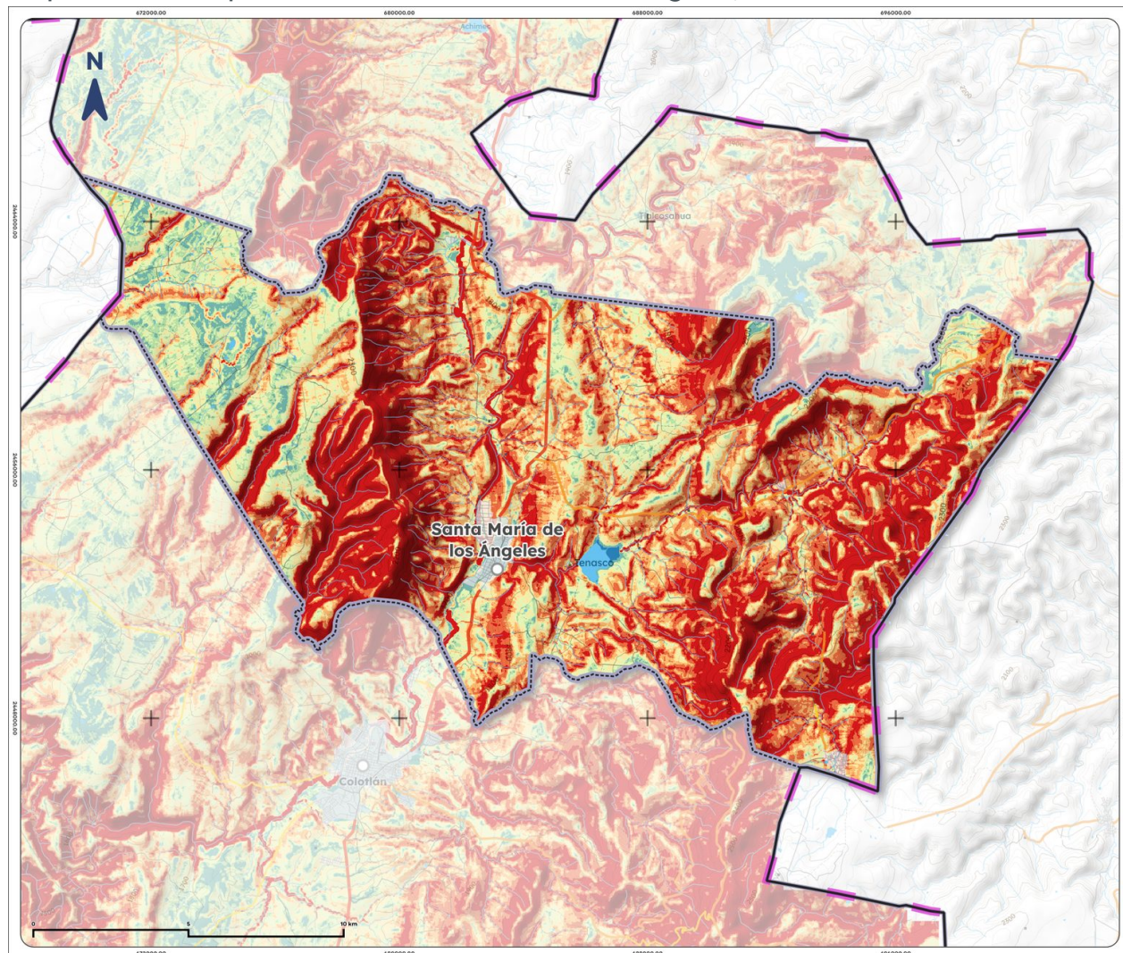
Mapa 16. Erosión potencial de Santa María de los Ángeles, 2025
