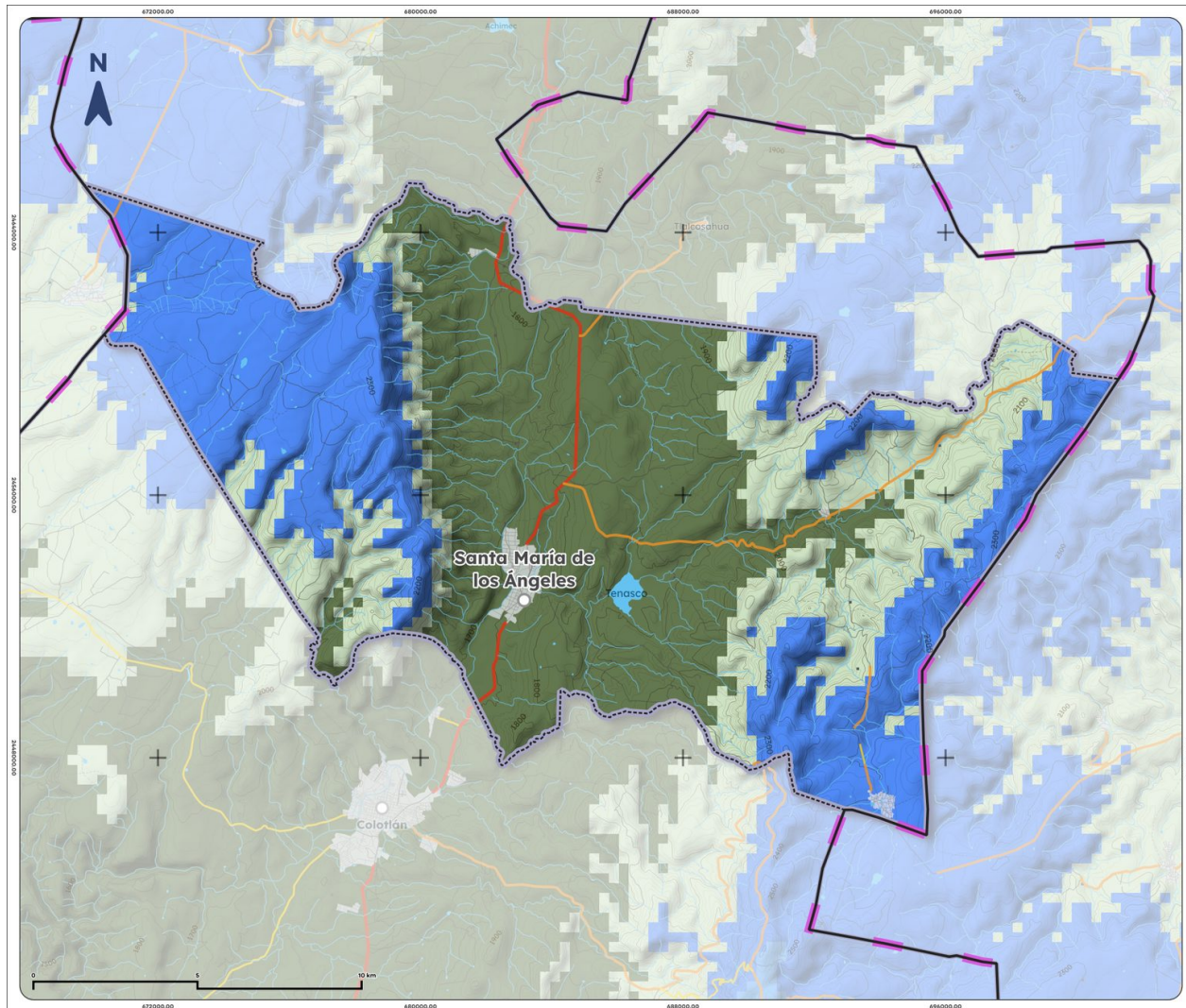
Mapa 10. Clima de Santa María de los Ángeles, 1995-2025
