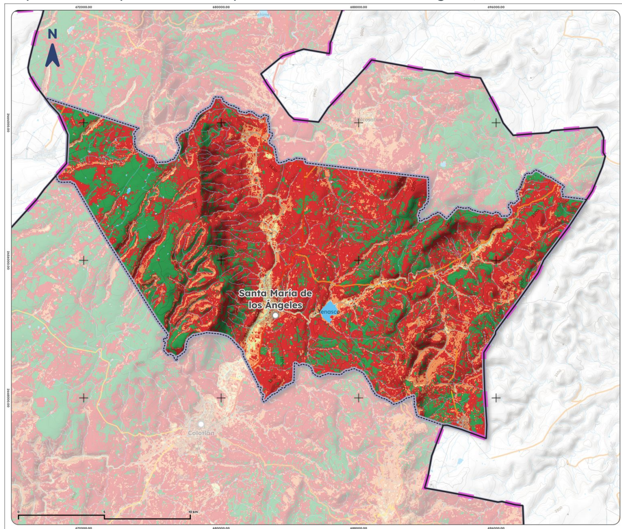
Mapa 15. Índice promedio de sequía de Santa María de los Ángeles, 2025
