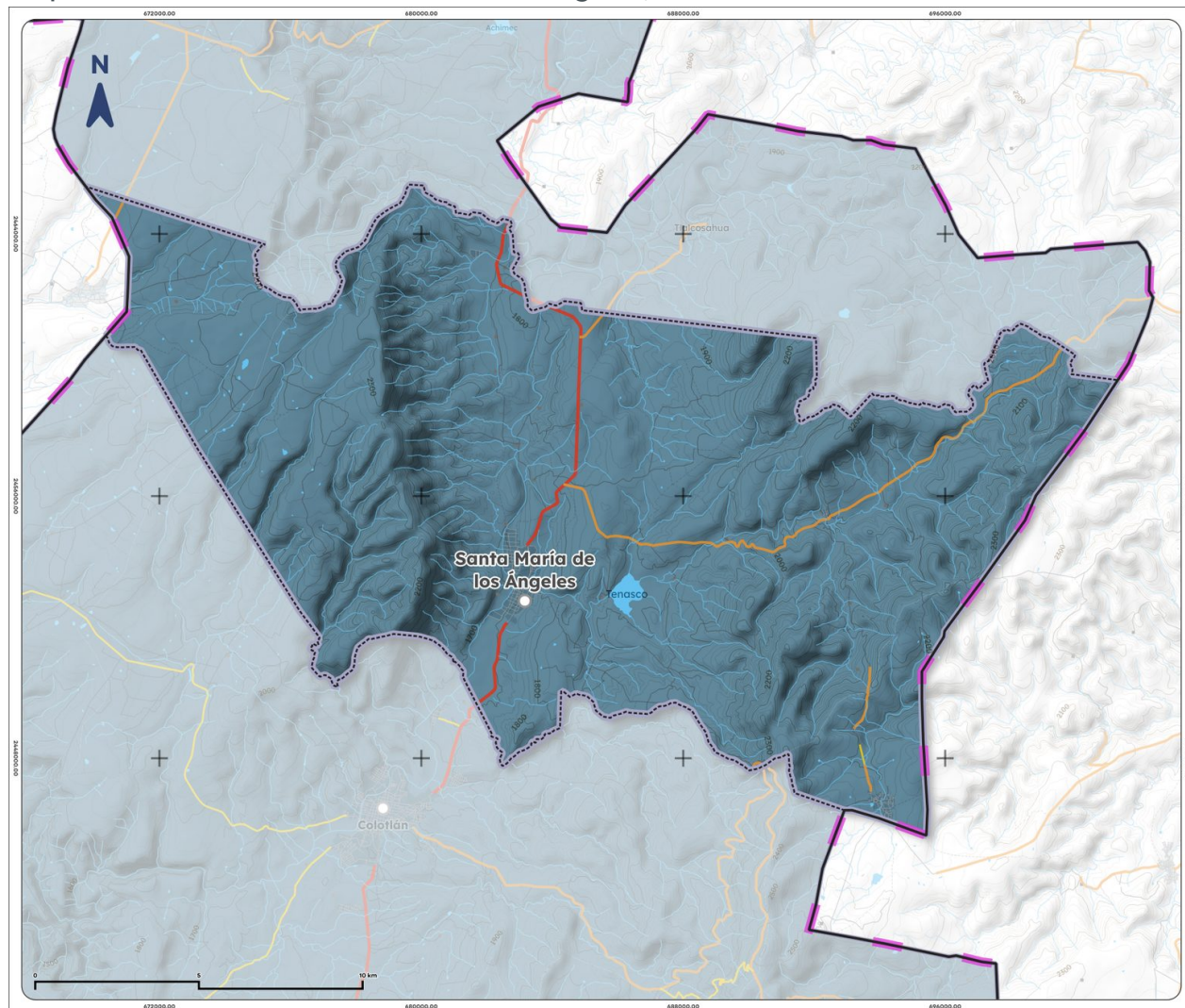
Mapa 6. Cuencas de Santa María de los Ángeles, 2023
