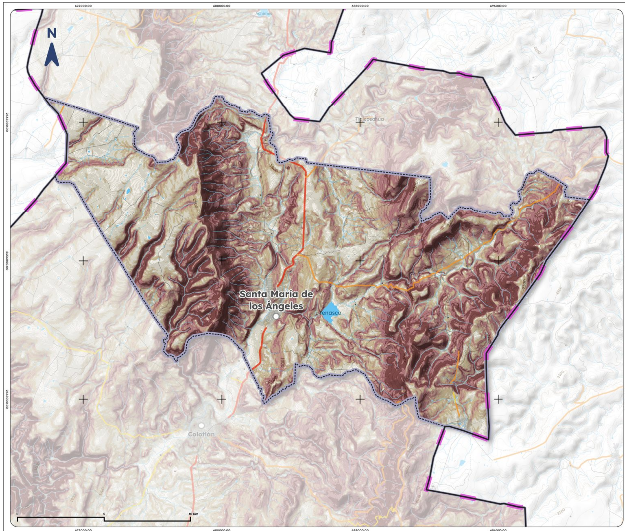
Mapa 5. Pendientes de Santa María de los Ángeles, 2025
