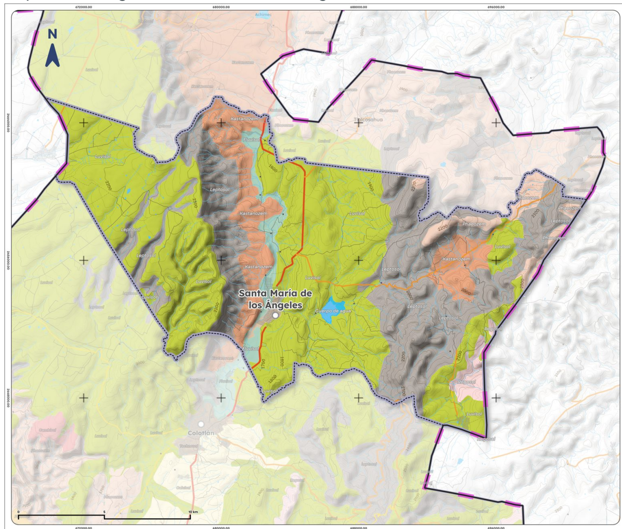
Mapa 4. Edafología de Santa María de los Ángeles, 2025
