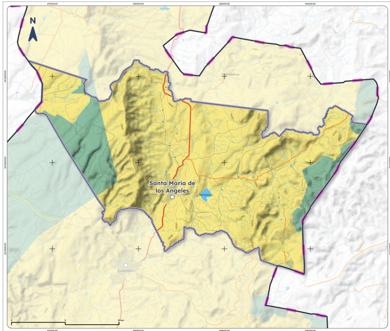
Mapa 7. Acuíferos de Santa María de los Ángeles, 2023
