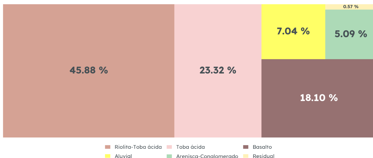
Geología de Santa María de los Ángeles, 1988
