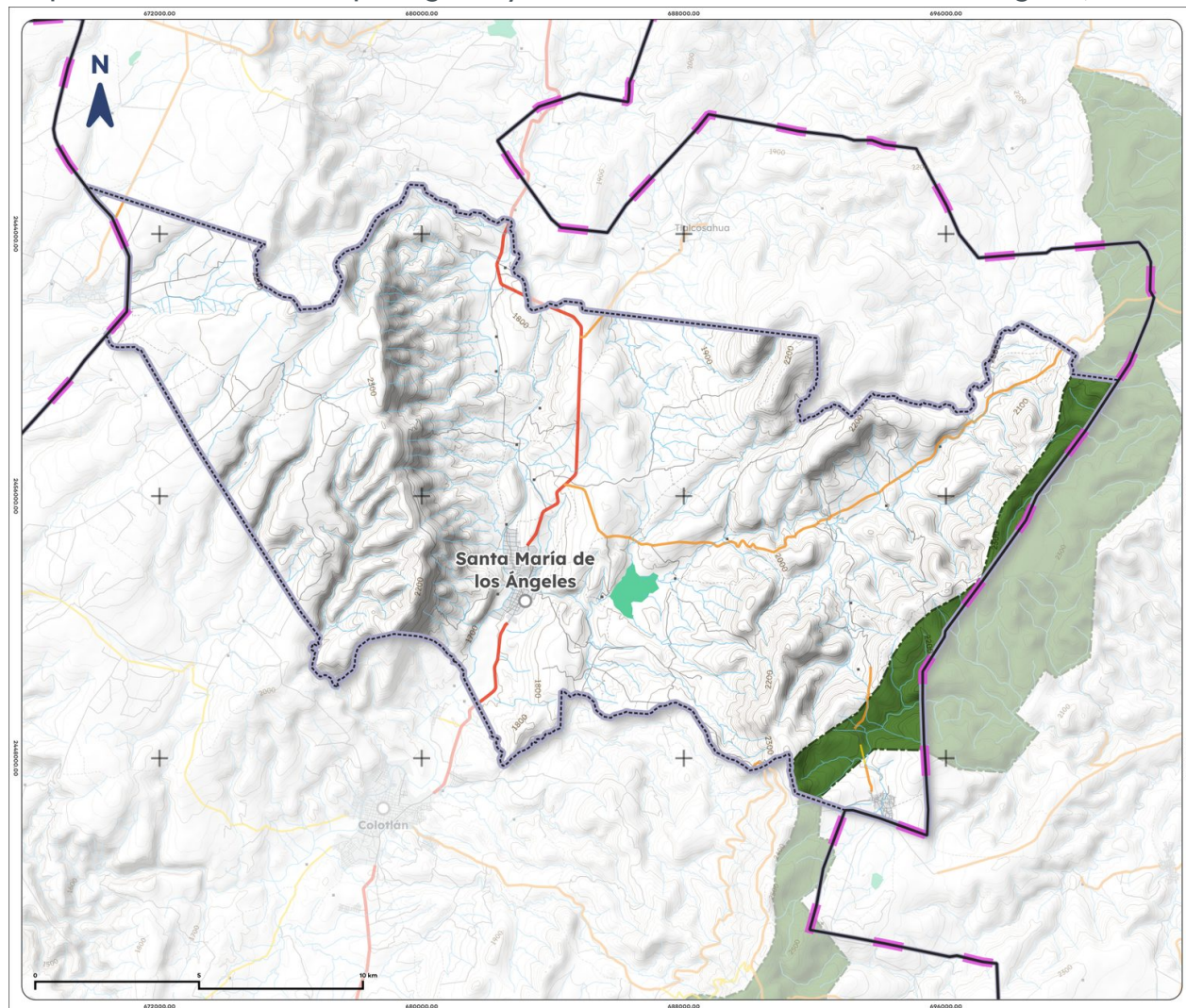
Mapa 14. Áreas naturales protegidas y humedales de Santa María de los Ángeles, 2025
