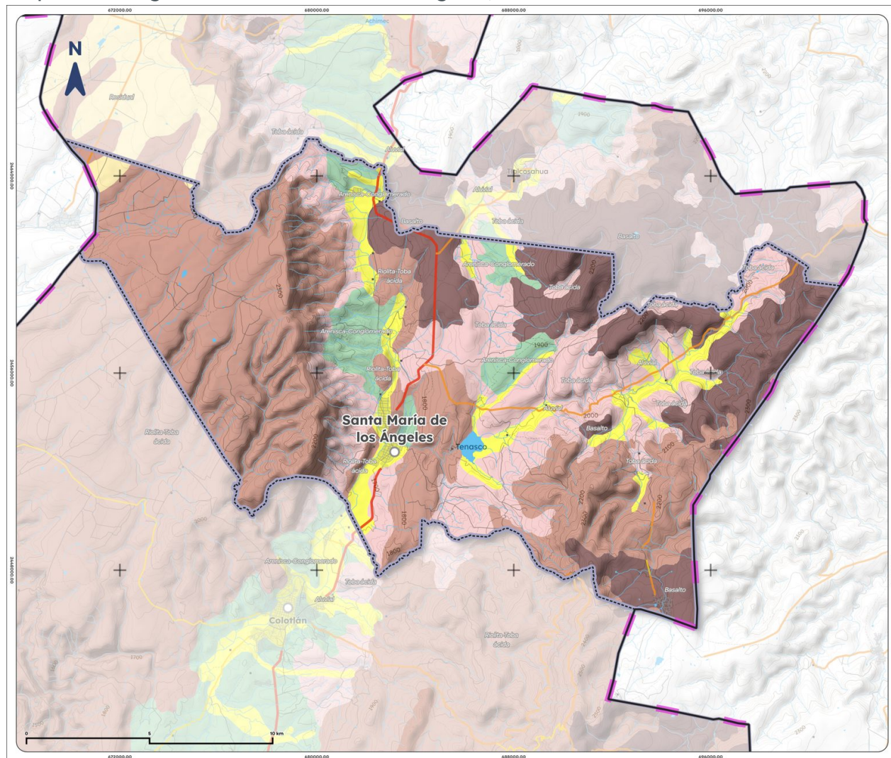
Mapa 3. Geología de Santa María de los Ángeles, 1988
