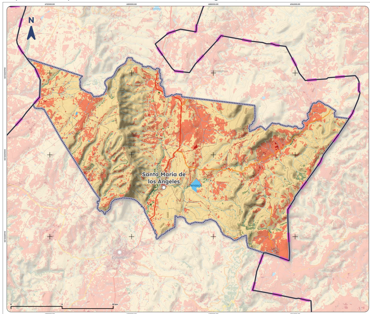
Mapa 12. NDVI promedio de Santa María de los Ángeles, 2025
