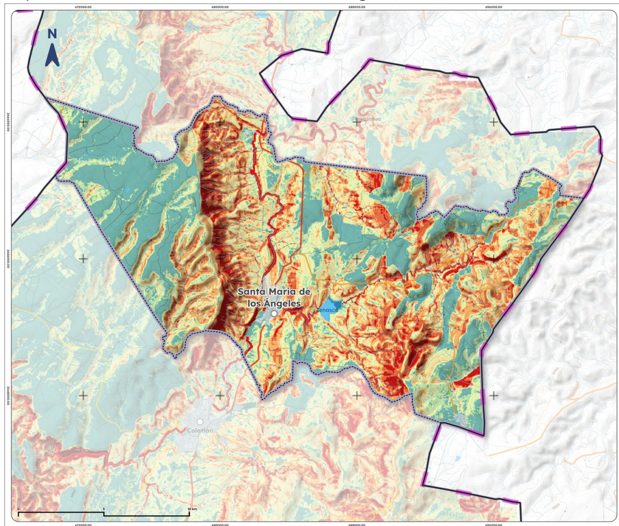
Mapa 17. Erosión efectiva de Santa María de los Ángeles, 2025
