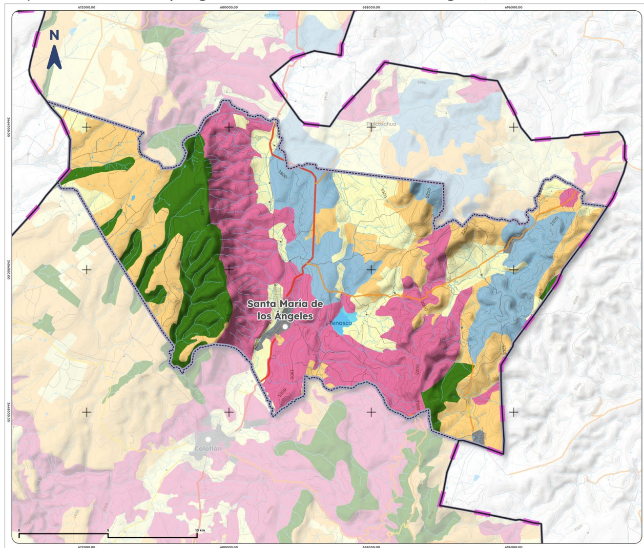
Mapa 11. Uso de suelo y vegetación de Santa María de los Ángeles, 2018
