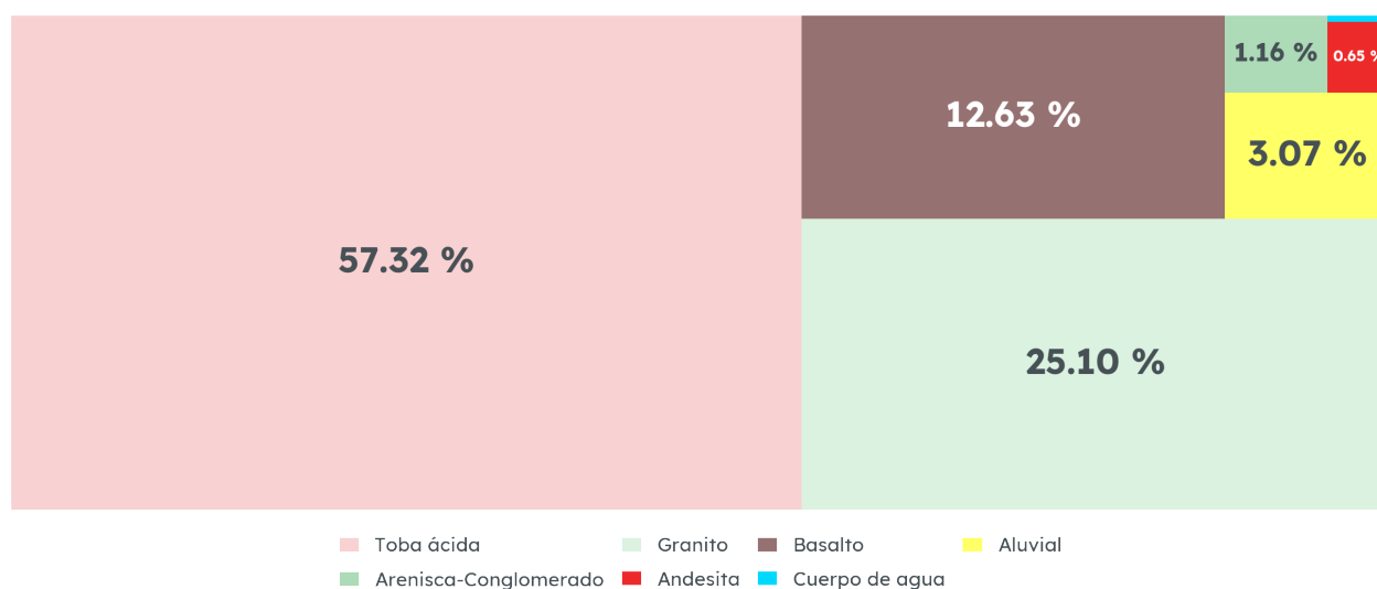
Geología de San Sebastián del Oeste, 1988
