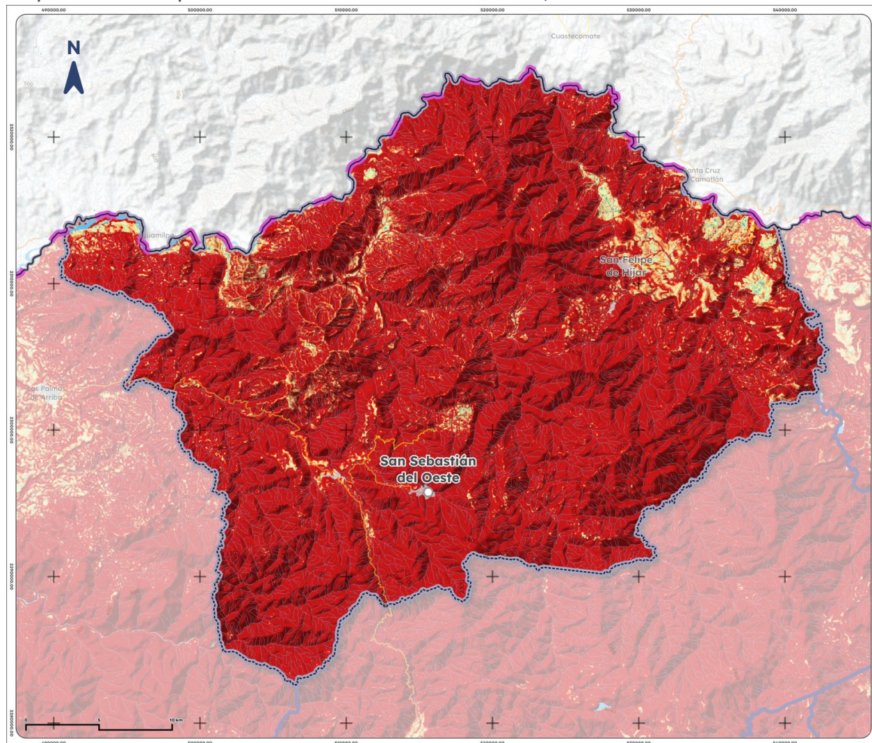
Mapa 16. Erosión potencial de San Sebastián del Oeste, 2025
