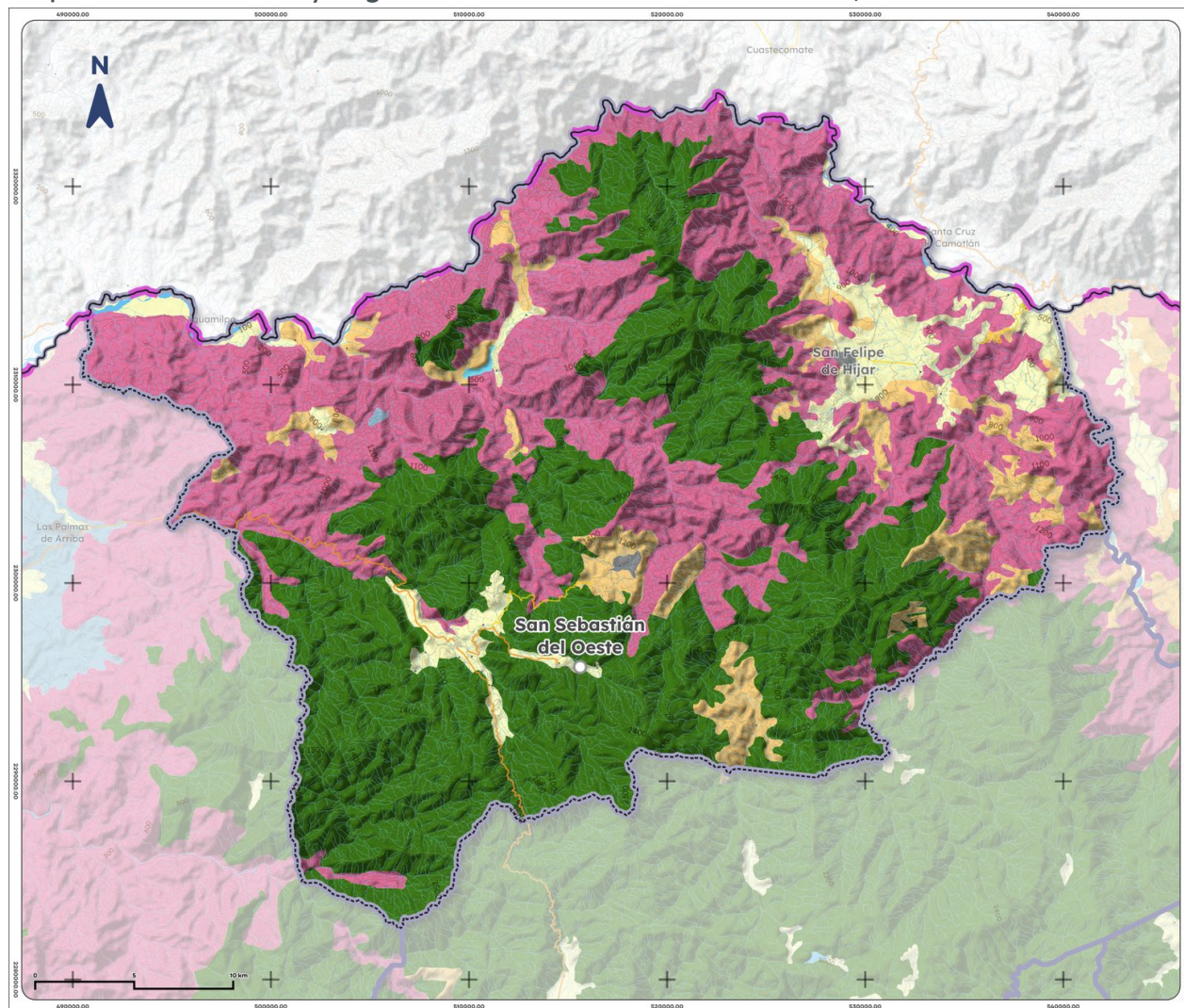
Mapa 11. Uso de suelo y vegetación de San Sebastián del Oeste, 2018
