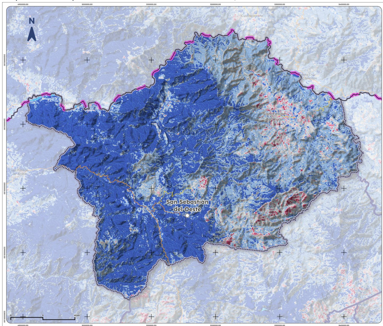
Mapa 13. NDWI promedio de San Sebastián del Oeste, 2025
