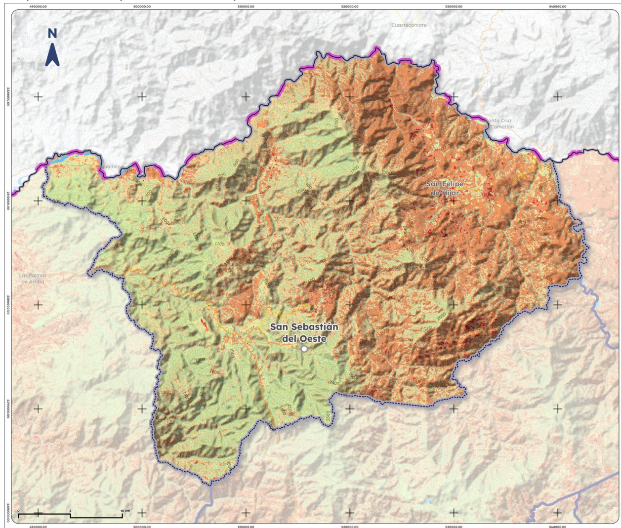
Mapa 15. Índice promedio de sequía de San Sebastián del Oeste, 2025
