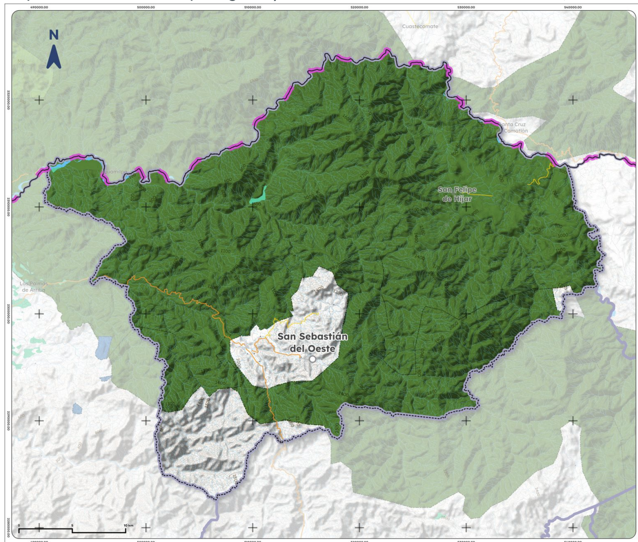
Mapa 14. Áreas naturales protegidas y humedales de San Sebastián del Oeste, 2025
