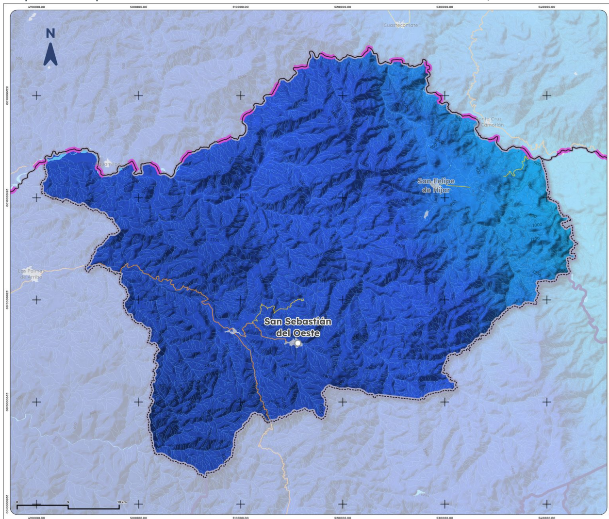
Mapa 9. Precipitación histórica acumulada de San Sebastián del Oeste, 1995-2025
