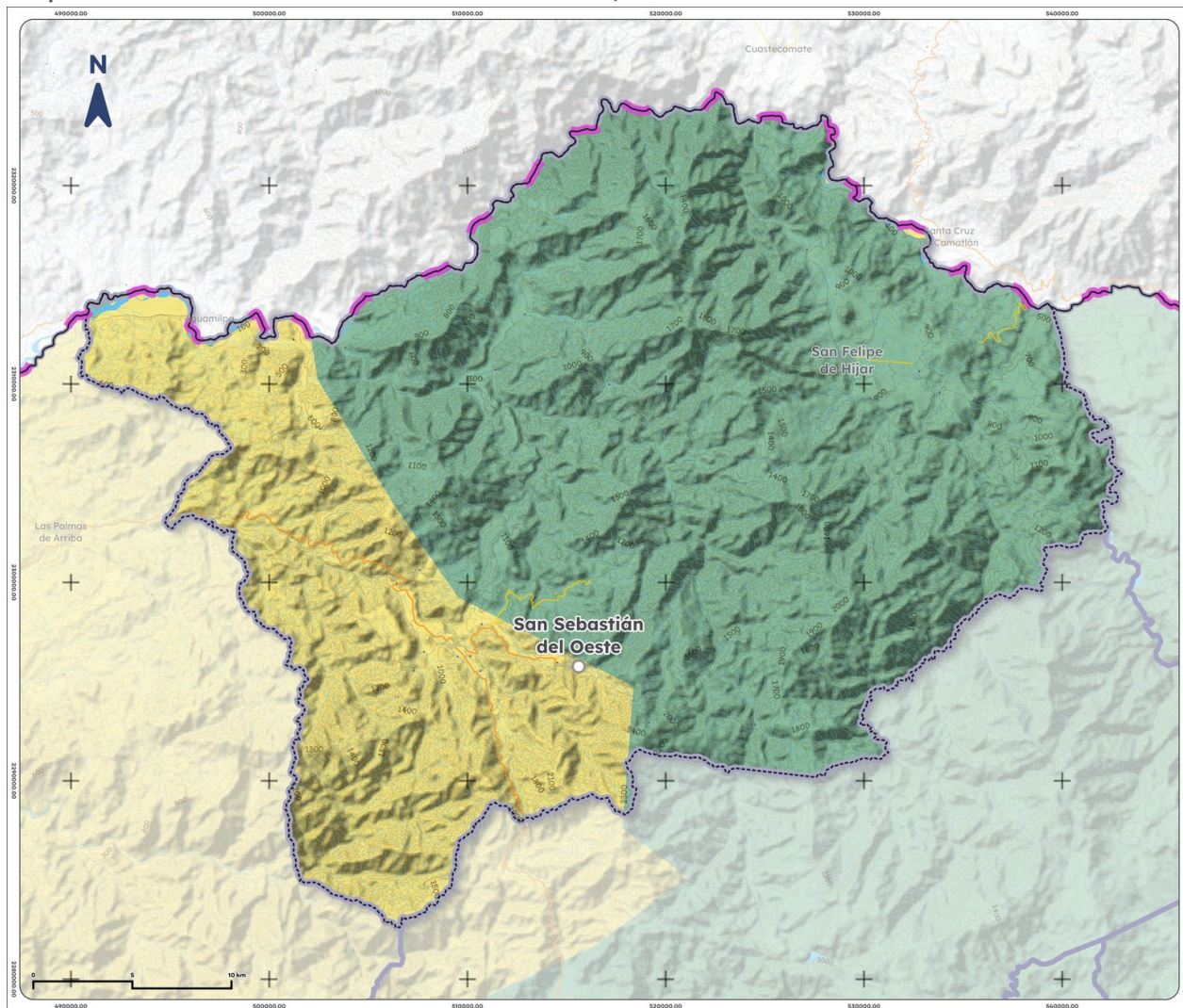
Mapa 7. Acuíferos de San Sebastián del Oeste, 2023
