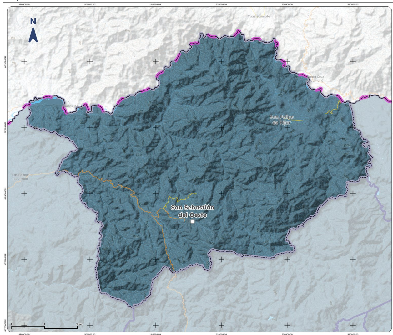
Mapa 6. Cuencas de San Sebastián del Oeste, 2023
