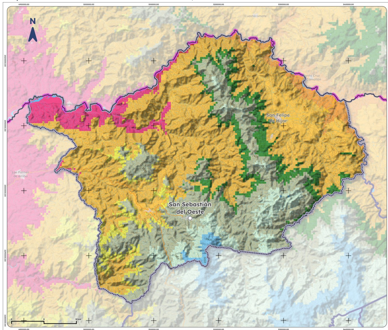
Mapa 10. Clima de San Sebastián del Oeste, 1995-2025
