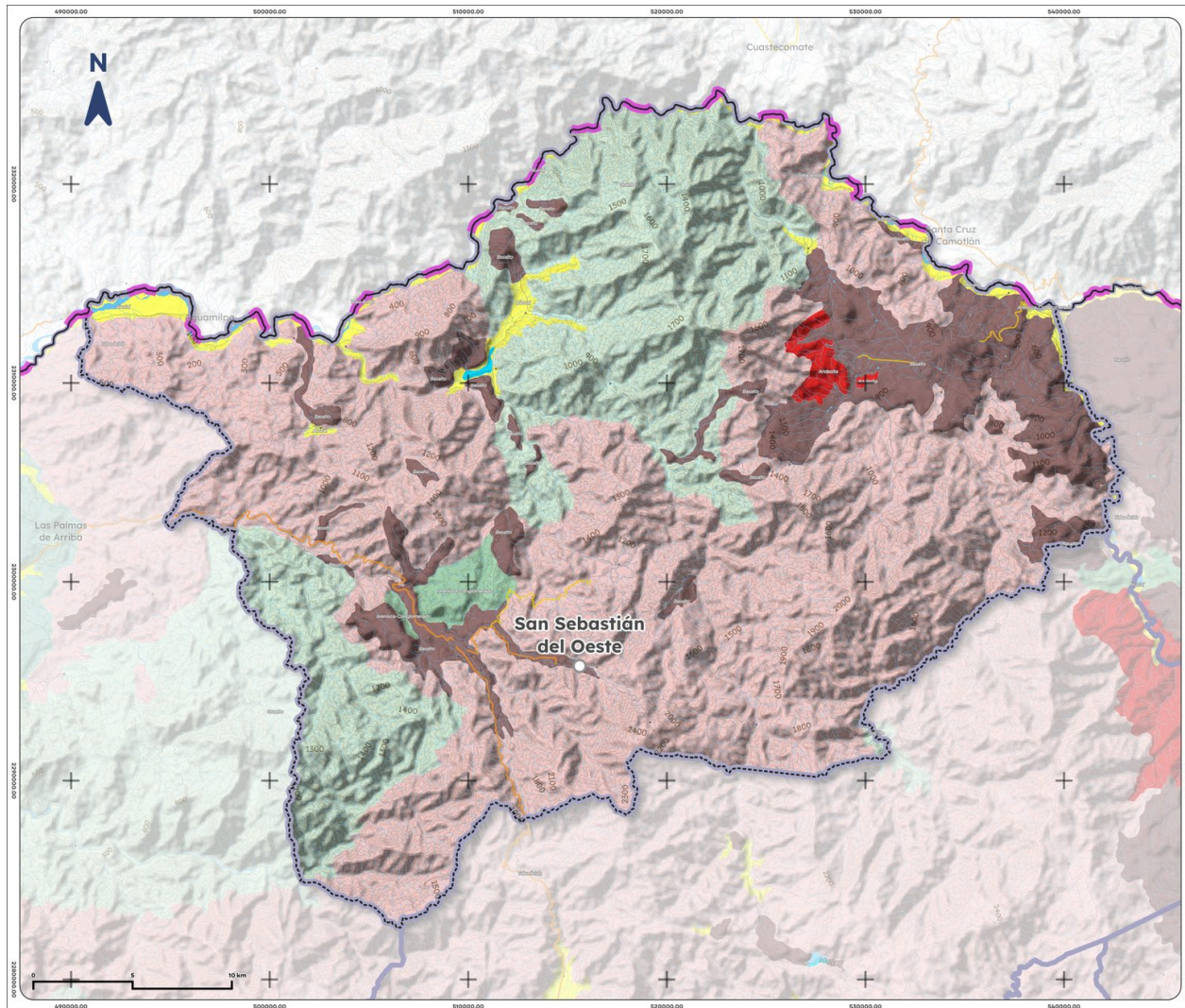
Mapa 3. Geología de San Sebastián del Oeste, 1988
