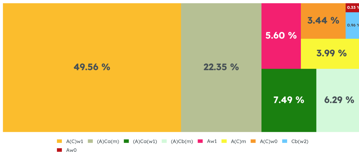
Clima de San Sebastián del Oeste, 1995-2025
