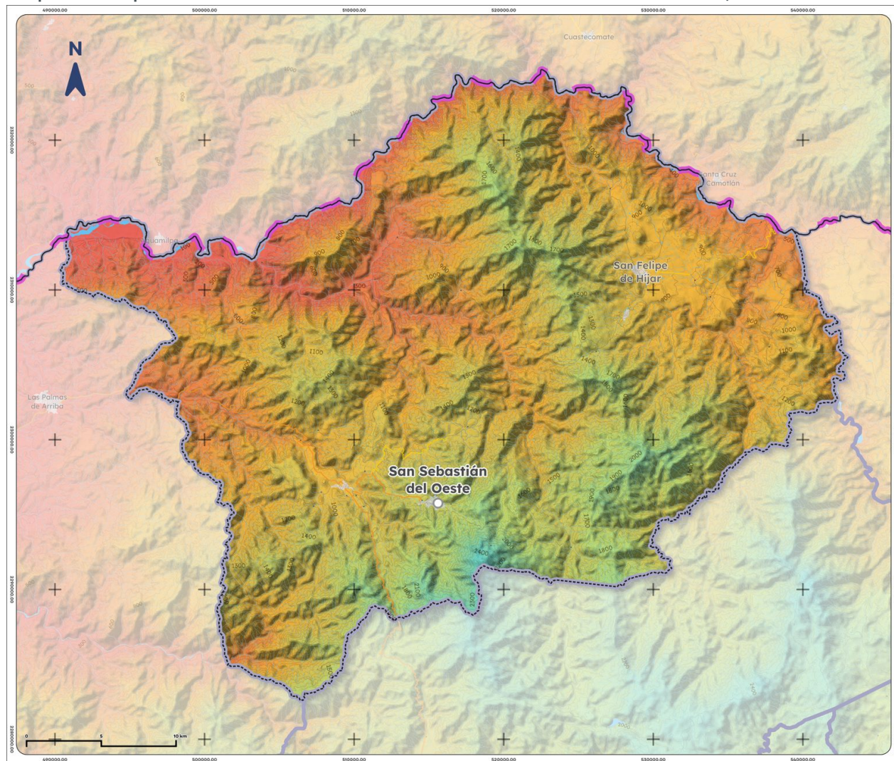
Mapa 8. Temperatura media anual histórica de San Sebastián del Oeste, 1995-2025
