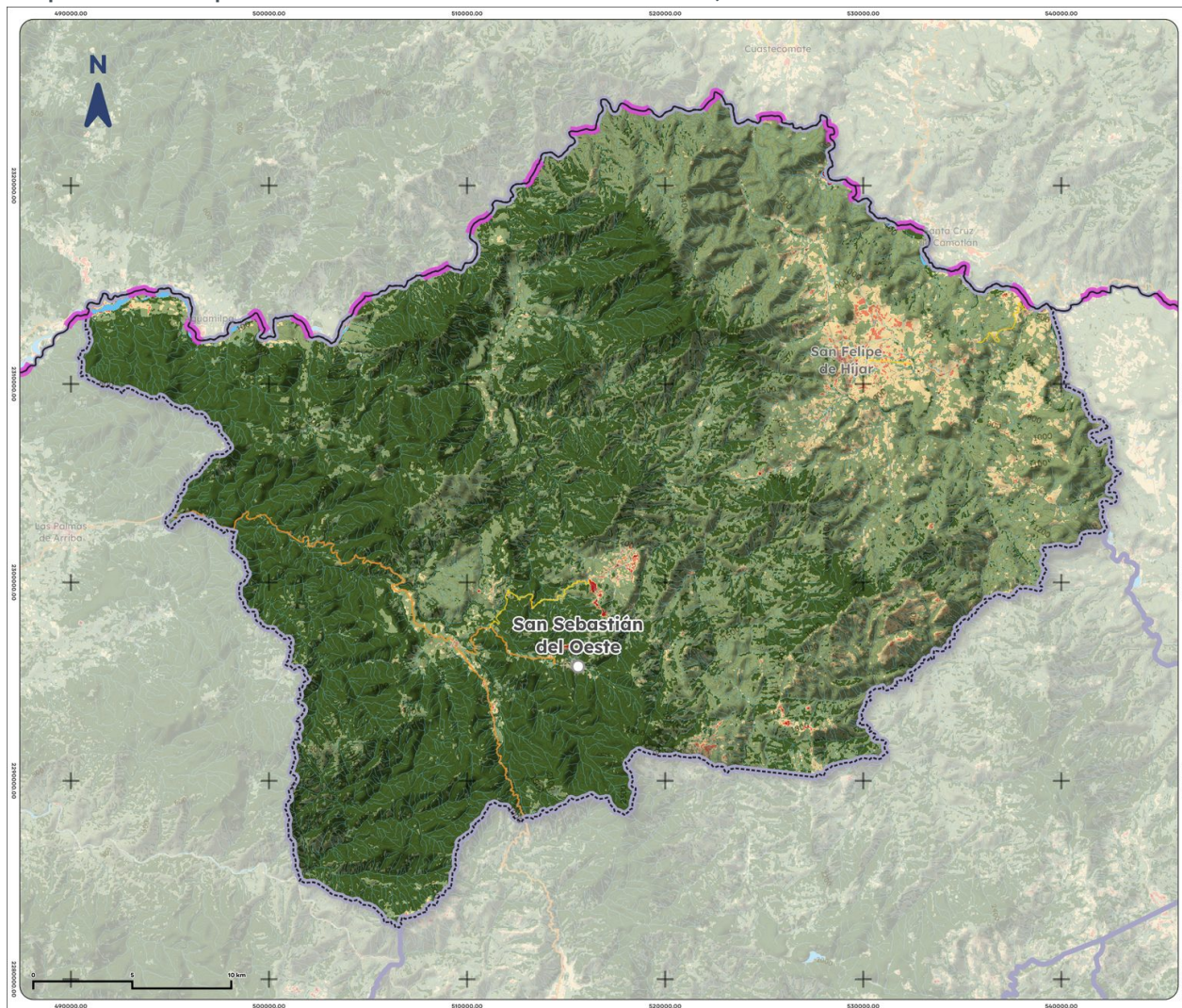
Mapa 12. NDVI promedio de San Sebastián del Oeste, 2025
