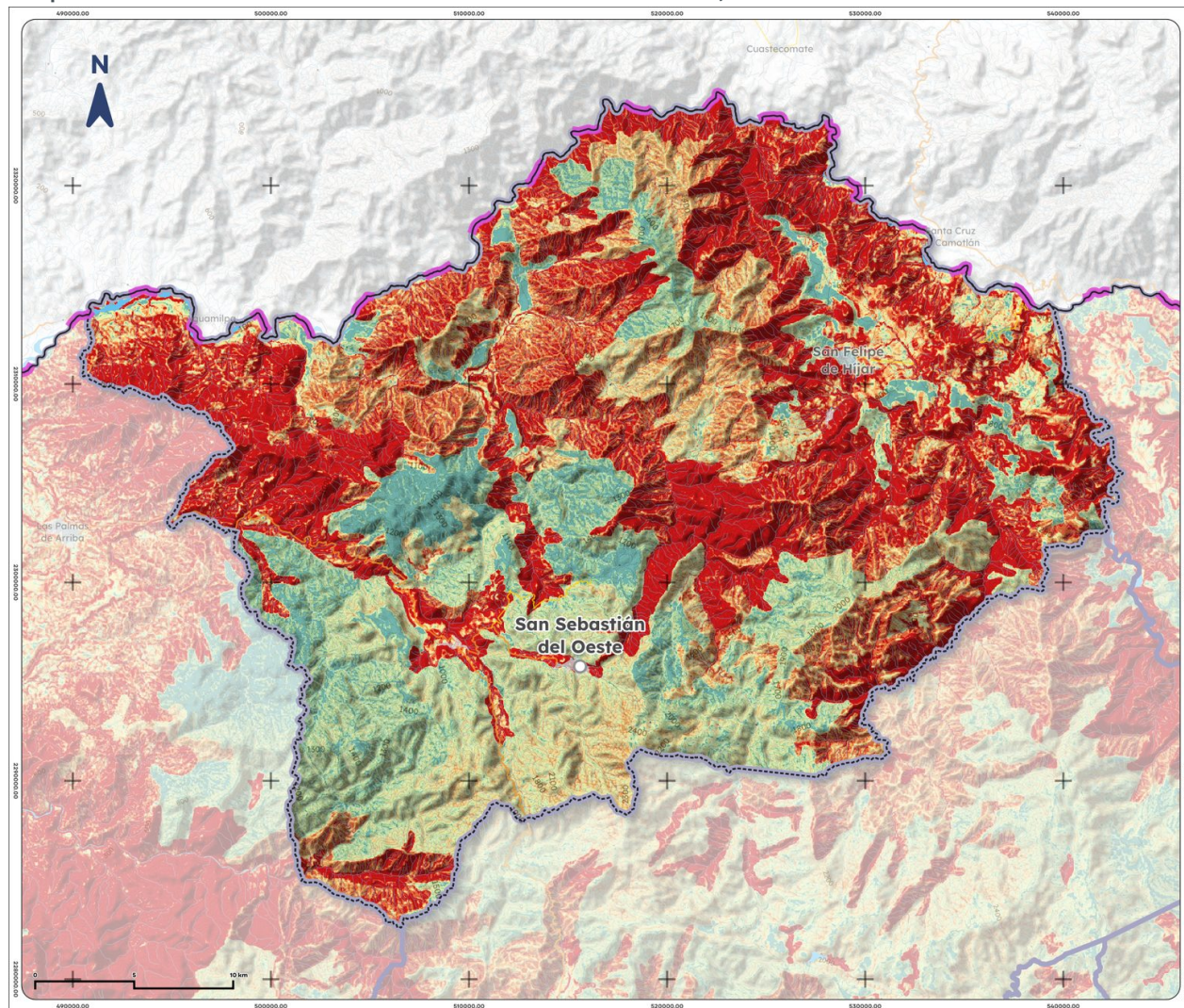
Mapa 17. Erosión efectiva de San Sebastián del Oeste, 2025
