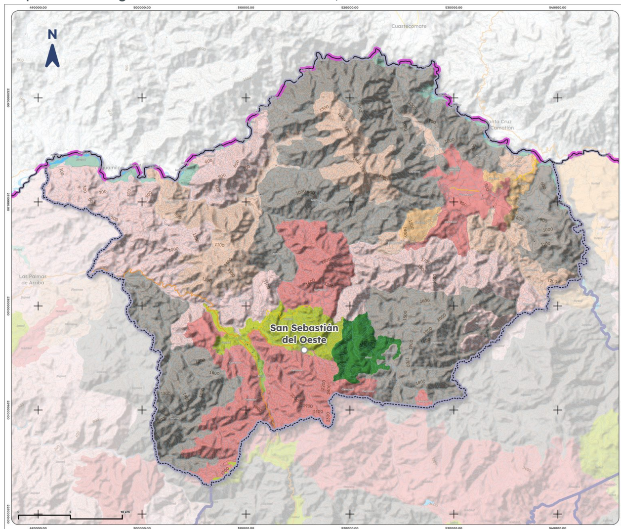
Mapa 4. Edafología de San Sebastián del Oeste, 2025
