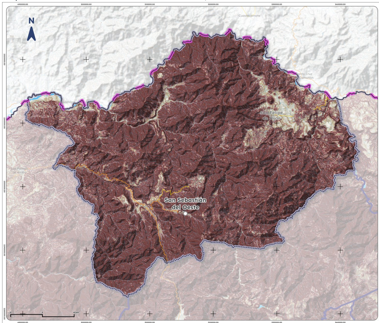
Mapa 5. Pendientes de San Sebastián del Oeste, 2025
