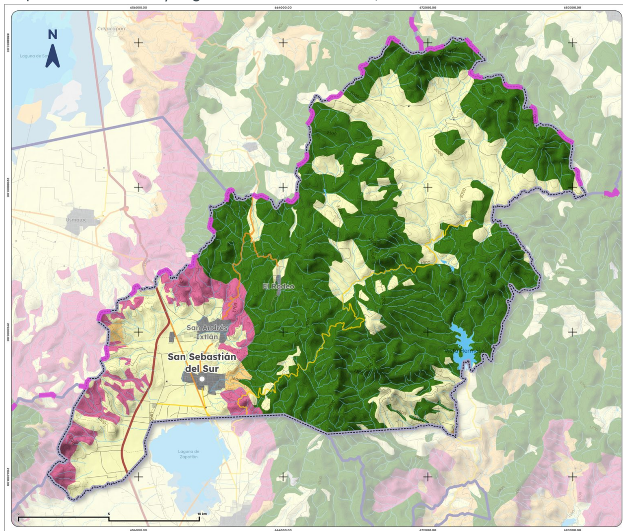
Mapa 11. Uso de suelo y vegetación de Gómez Farías, 2018
