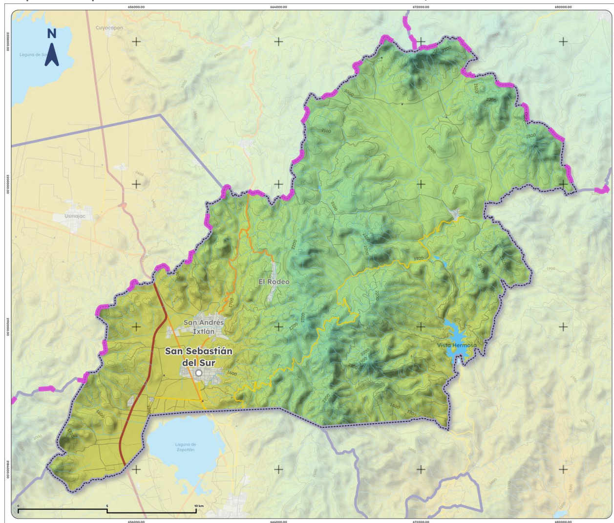
Mapa 8. Temperatura media anual histórica de Gómez Farías, 1995-2025
