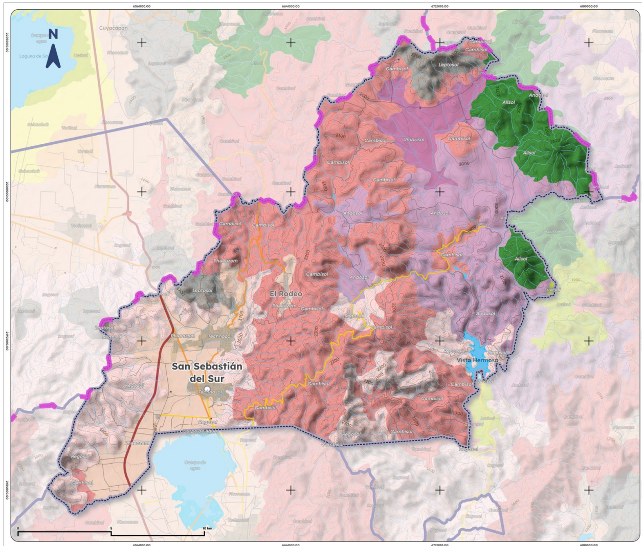
Mapa 4. Edafología de Gómez Farías, 2025
