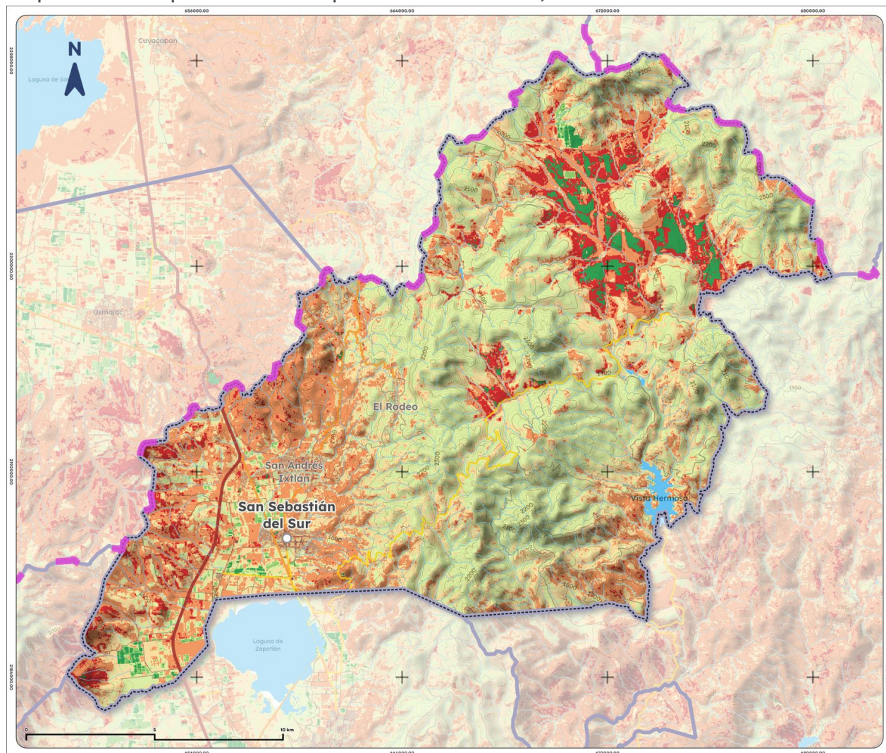
Mapa 15. Índice promedio de sequía de Gómez Farías, 2025
