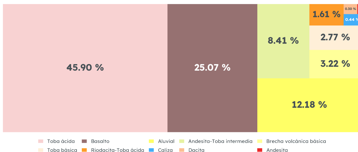
Geología de Gómez Farías, 1988
