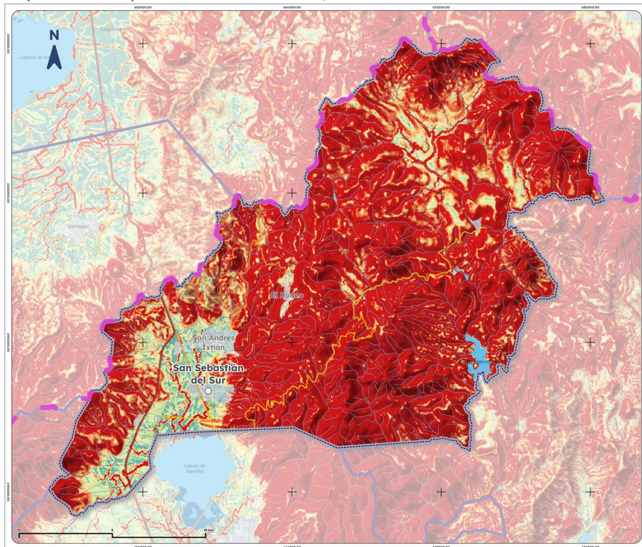
Mapa 16. Erosión potencial de Gómez Farías, 2025
