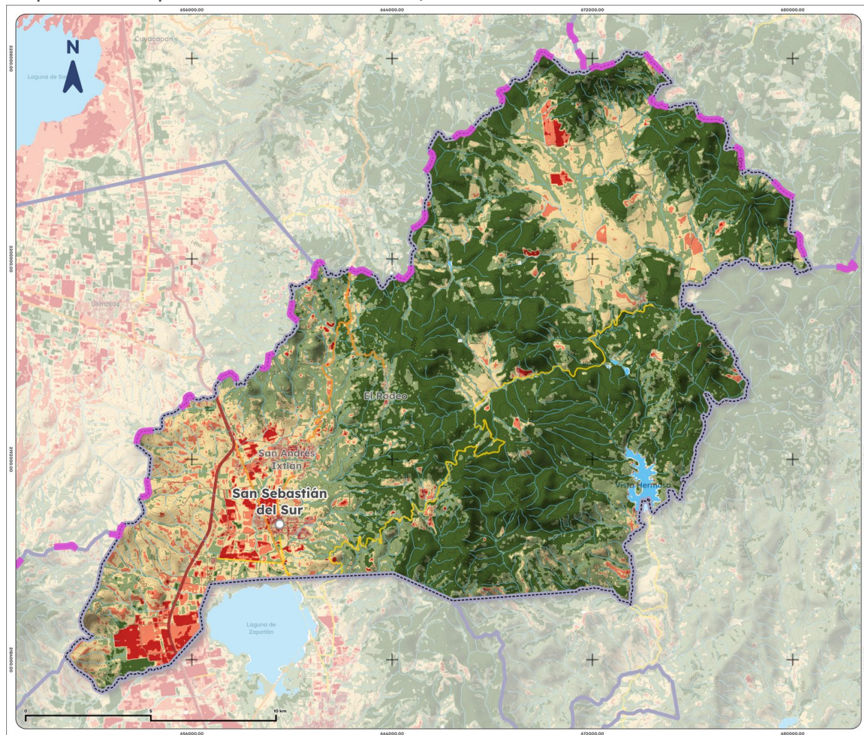
Mapa 12. NDVI promedio de Gómez Farías, 2025
