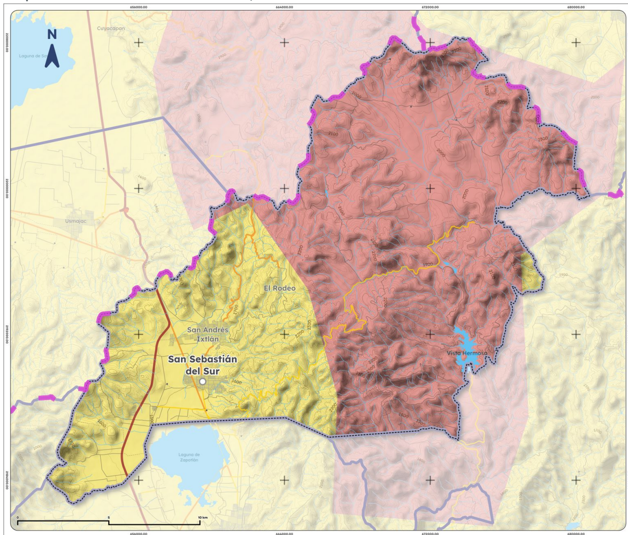
Mapa 7. Acuíferos de Gómez Farías, 2023
