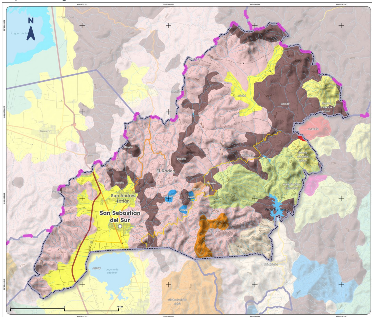
Mapa 3. Geología de Gómez Farías, 1988
