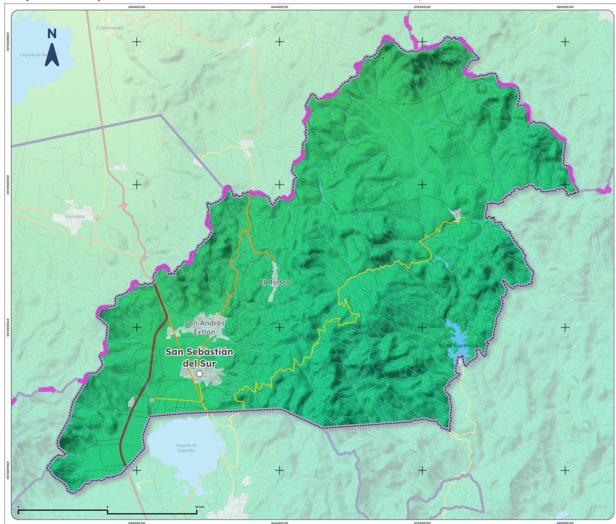
Mapa 9. Precipitación histórica acumulada de Gómez Farías, 1995-2025
