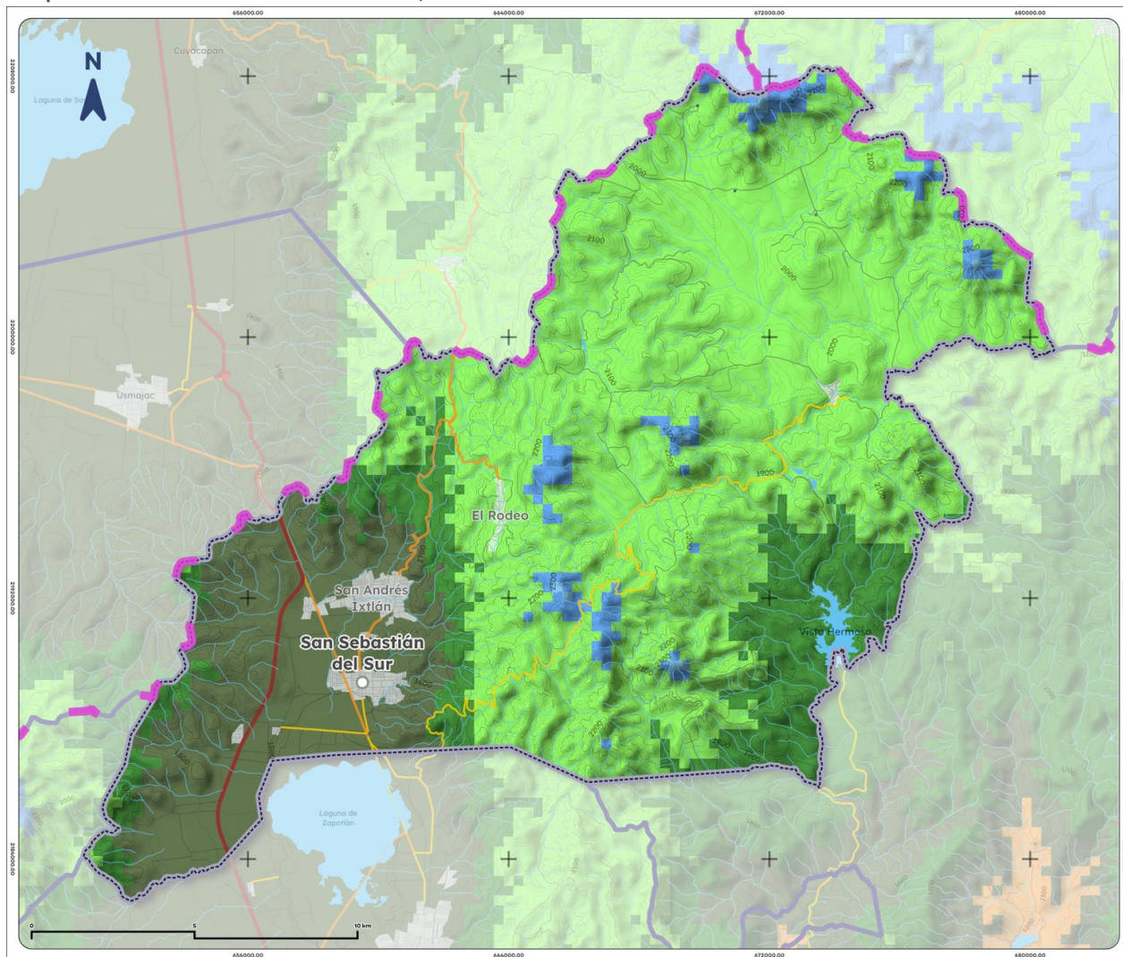
Mapa 10. Clima de Gómez Farías, 1995-2025
