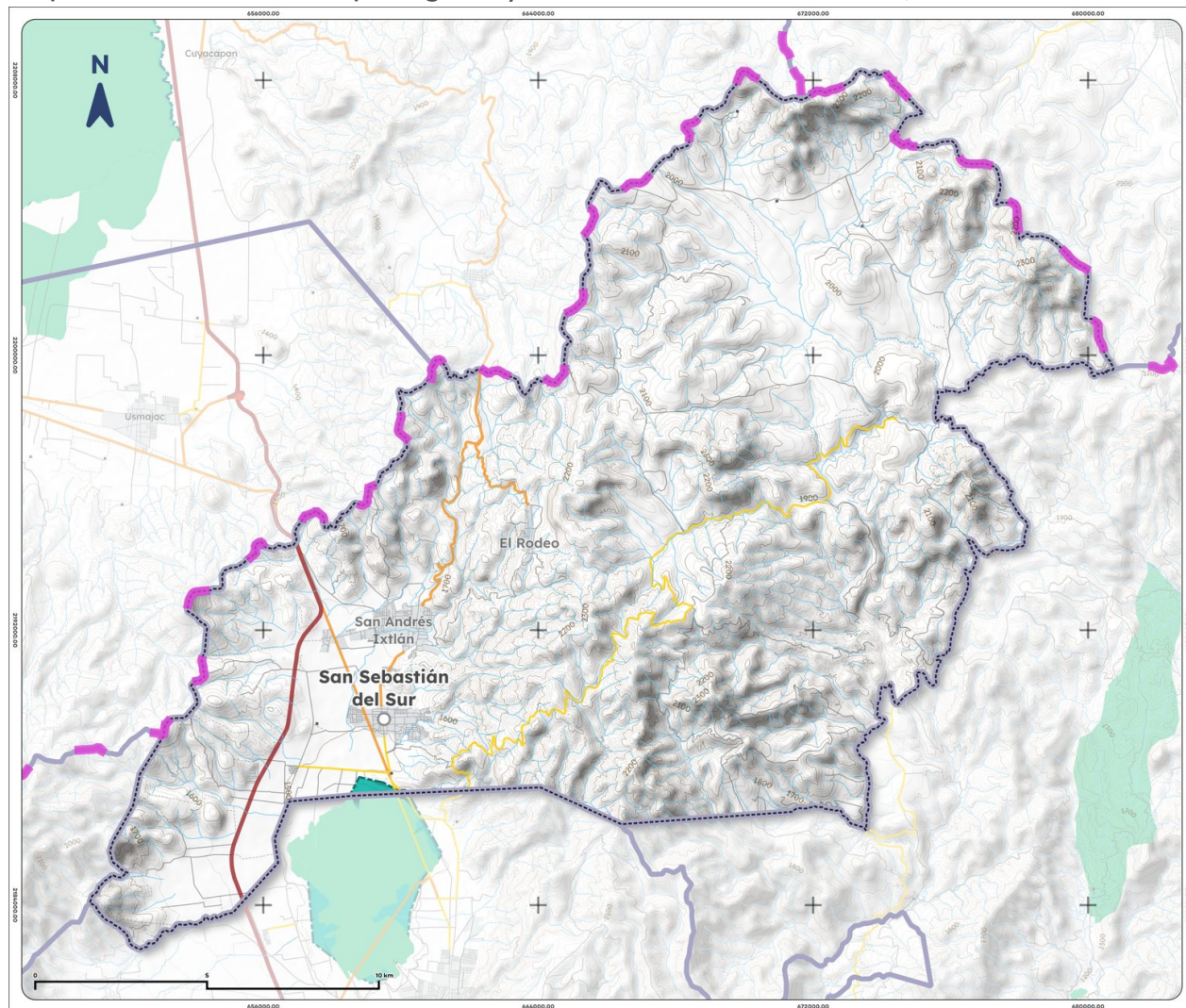
Mapa 14. Áreas naturales protegidas y humedales de Gómez Farías, 2025
