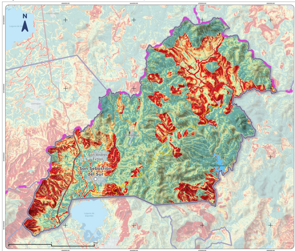
Mapa 17. Erosión efectiva de Gómez Farías, 2025
