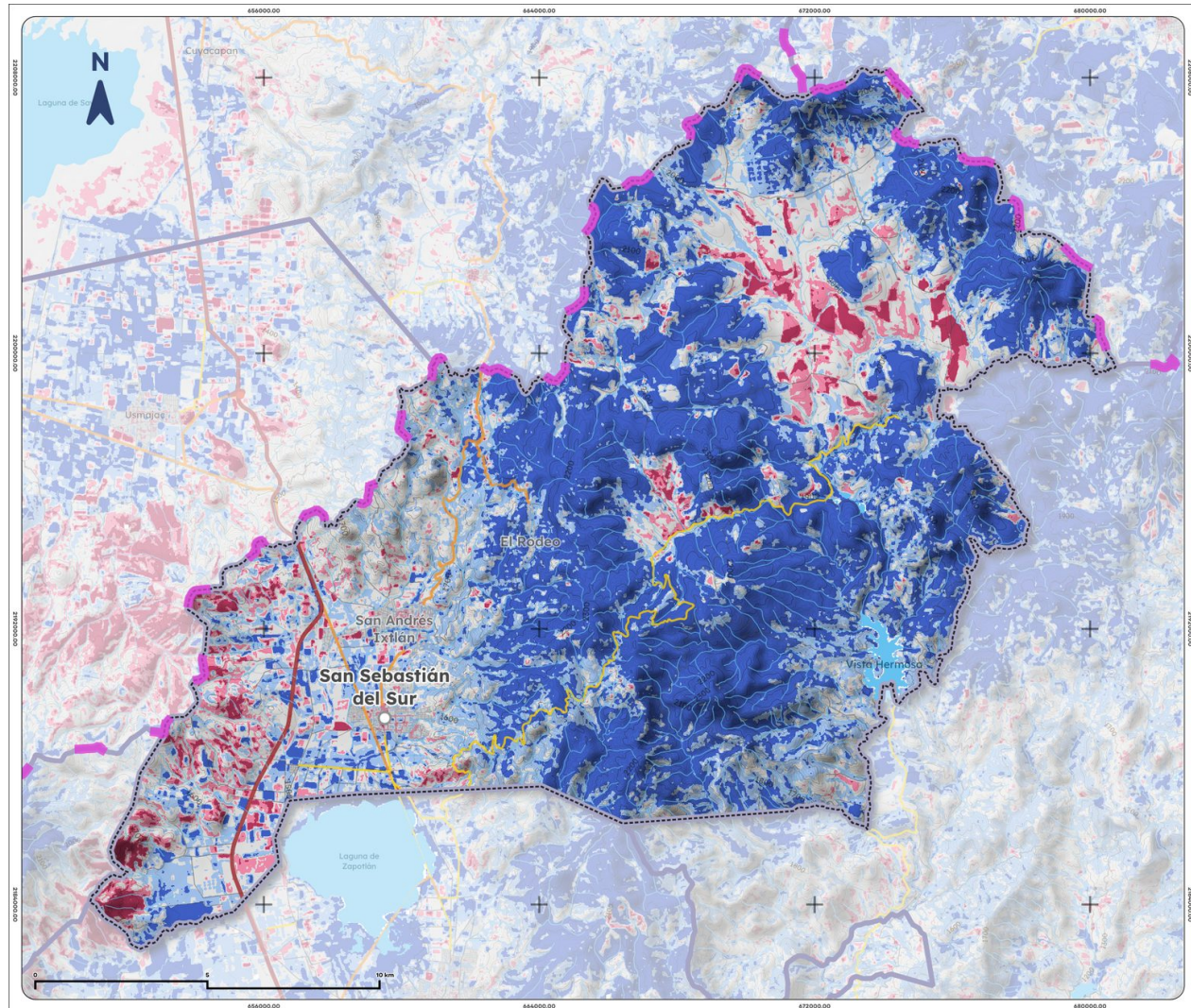
Mapa 13. NDWI promedio de Gómez Farías, 2025
