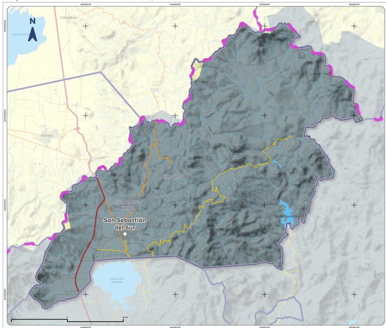
Mapa 6. Cuencas de Gómez Farías, 2023
