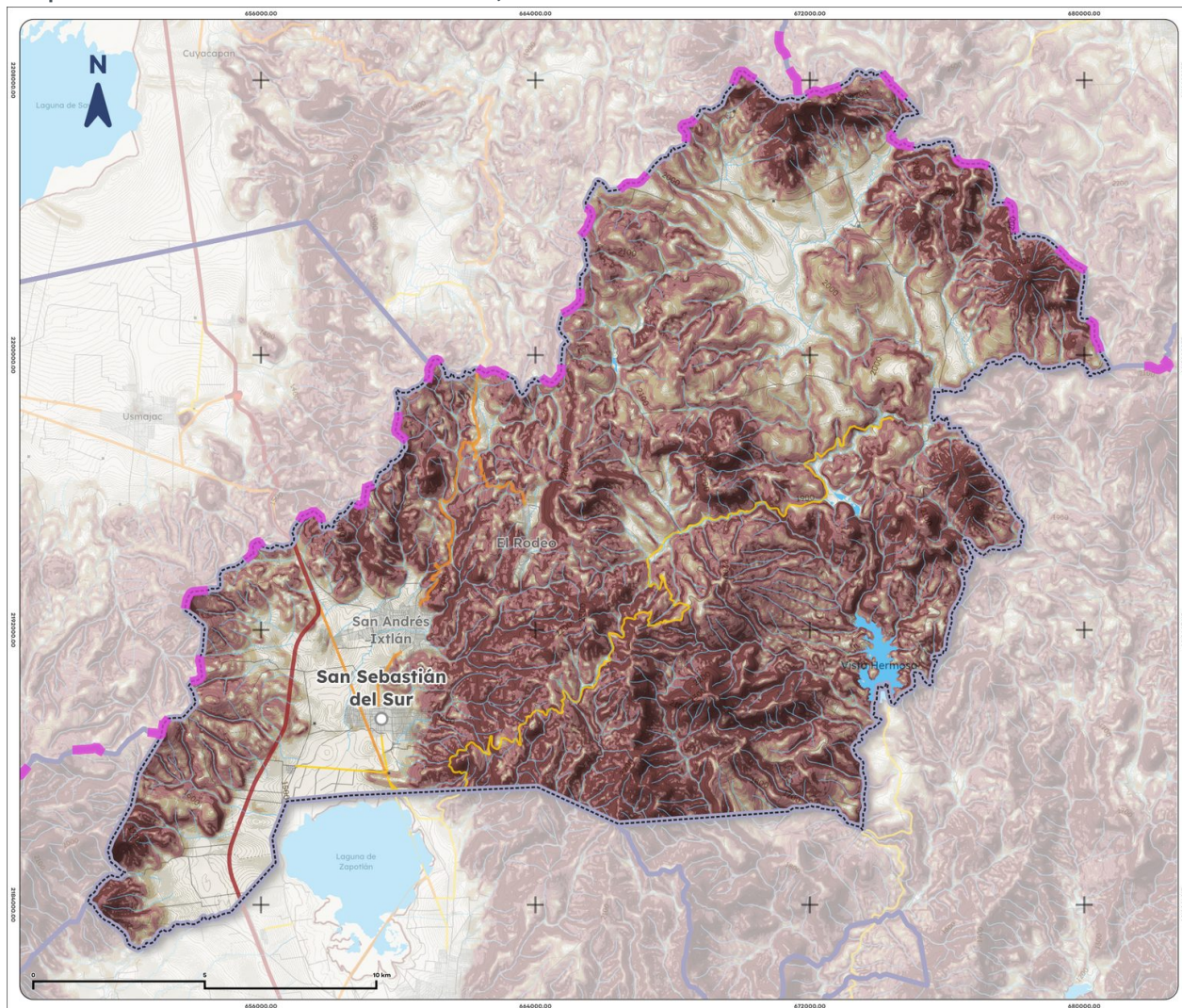
Mapa 5. Pendientes de Gómez Farías, 2025
