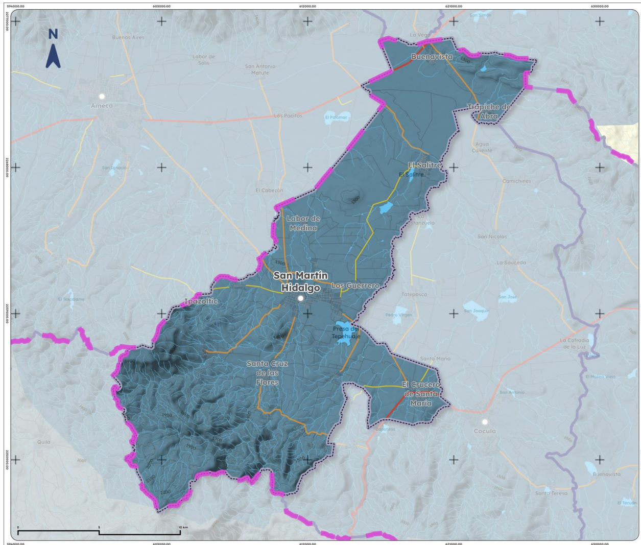
Mapa 6. Cuencas de San Martín Hidalgo, 2023
