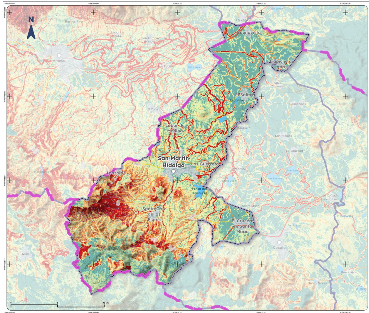
Mapa 17. Erosión efectiva de San Martín Hidalgo, 2025
