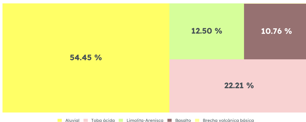
Geología de San Martín Hidalgo, 1988
