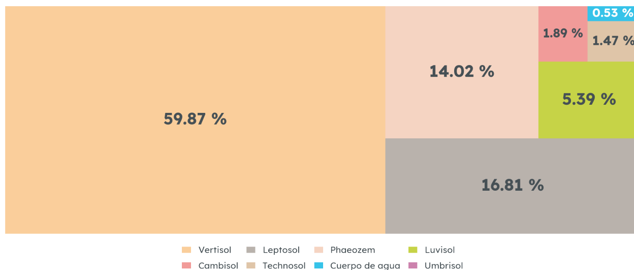
Edafología de San Martín Hidalgo, 2025
