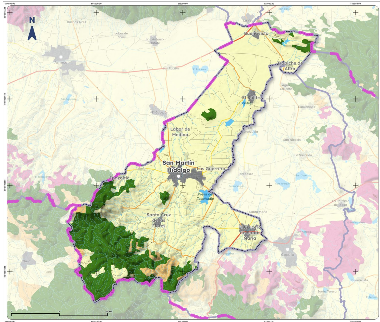
Mapa 11. Uso de suelo y vegetación de San Martín Hidalgo, 2018
