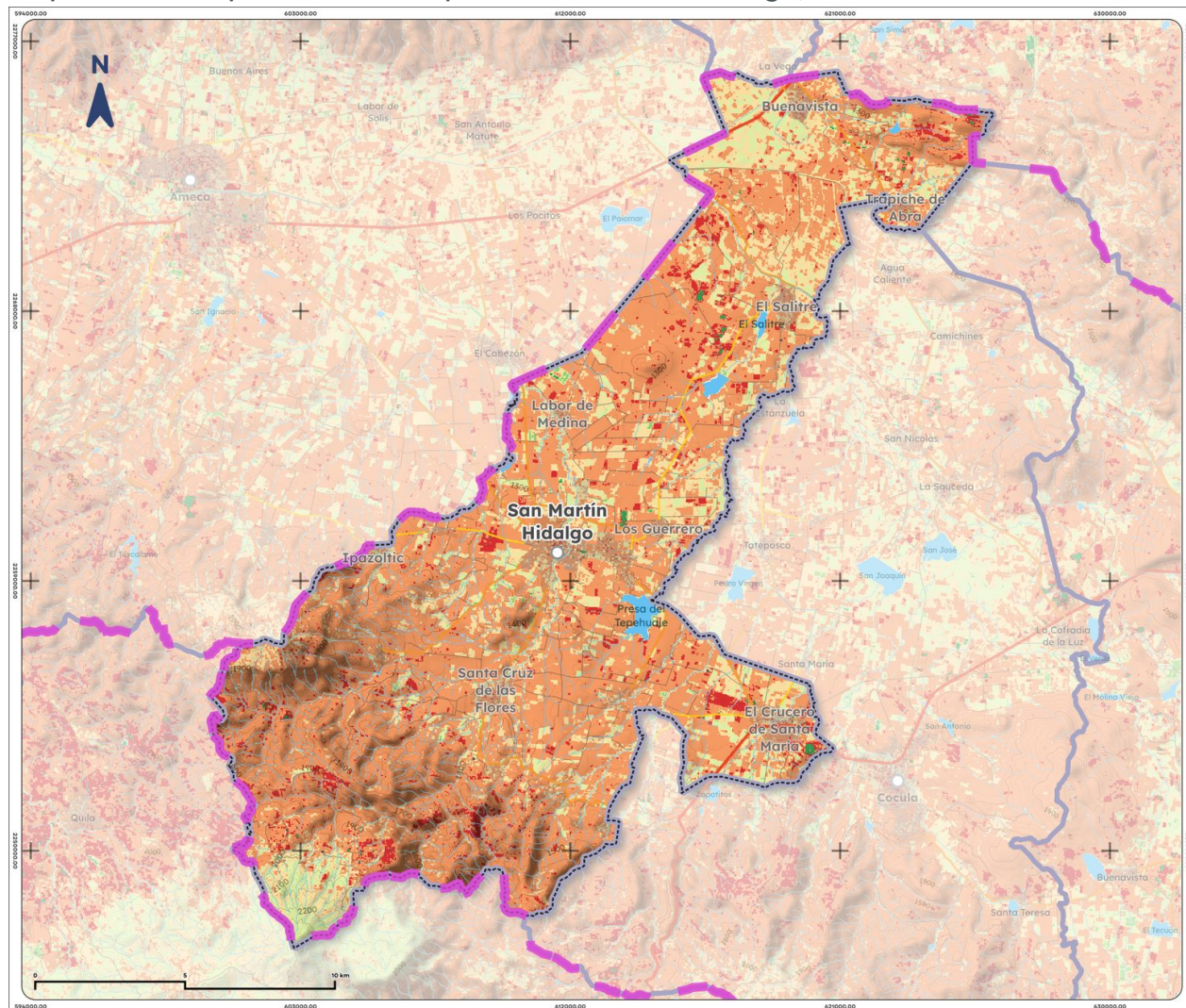
Mapa 15. Índice promedio de sequía de San Martín Hidalgo, 2025
