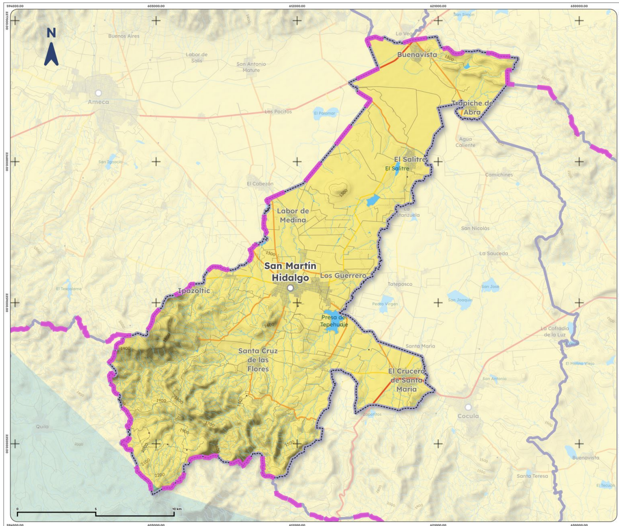
Mapa 7. Acuíferos de San Martín Hidalgo, 2023
