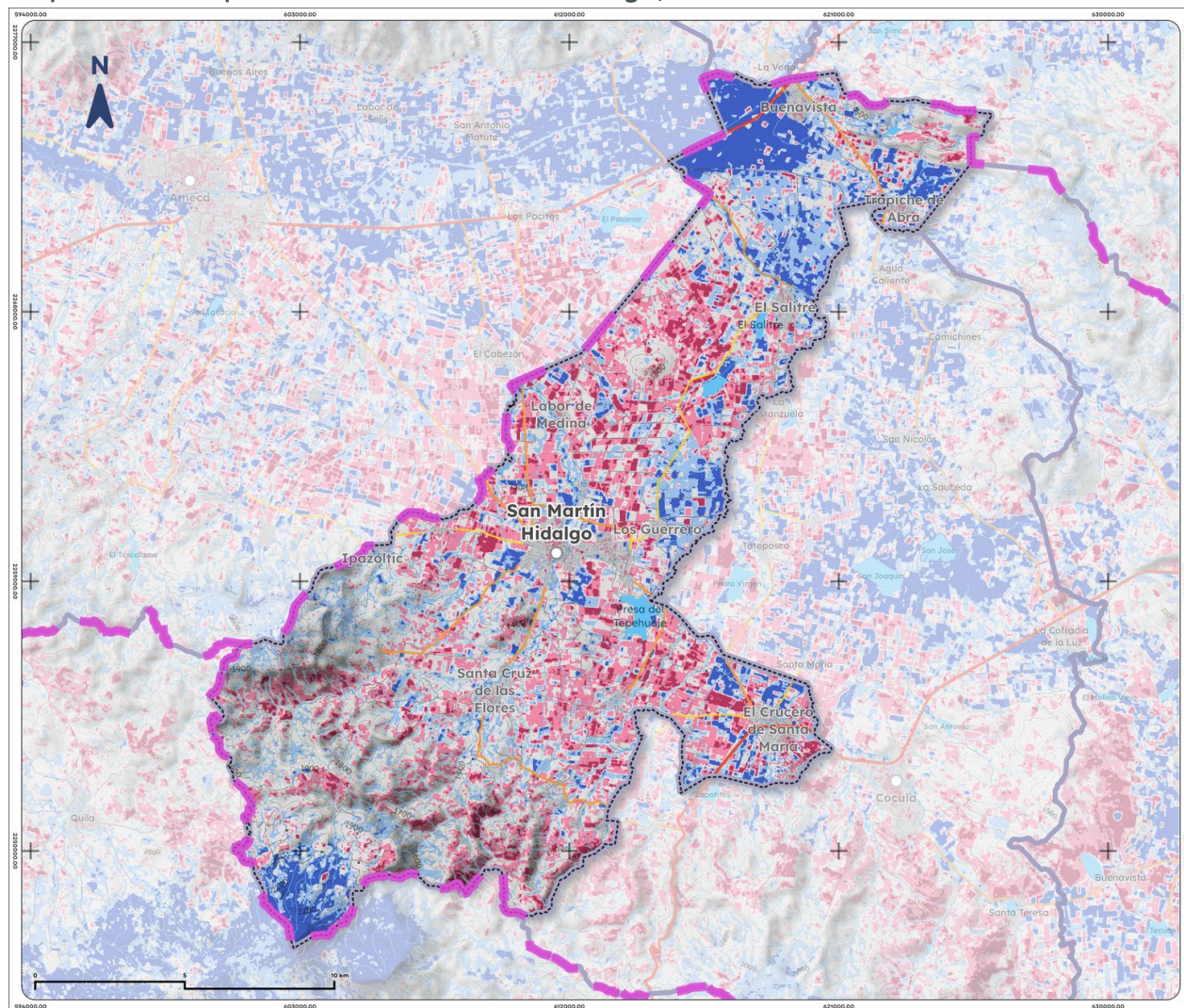
Mapa 13. NDWI promedio de San Martín Hidalgo, 2025
