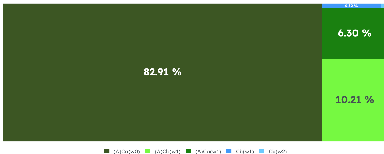
Clima de San Martín Hidalgo, 1995-2025
