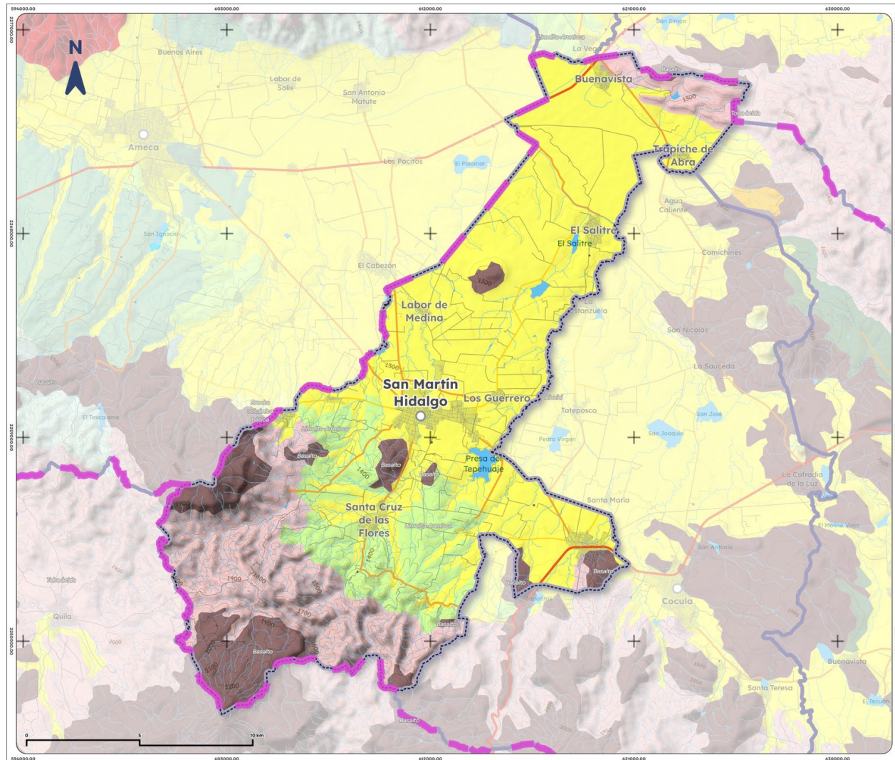
Mapa 3. Geología de San Martín Hidalgo, 1988
