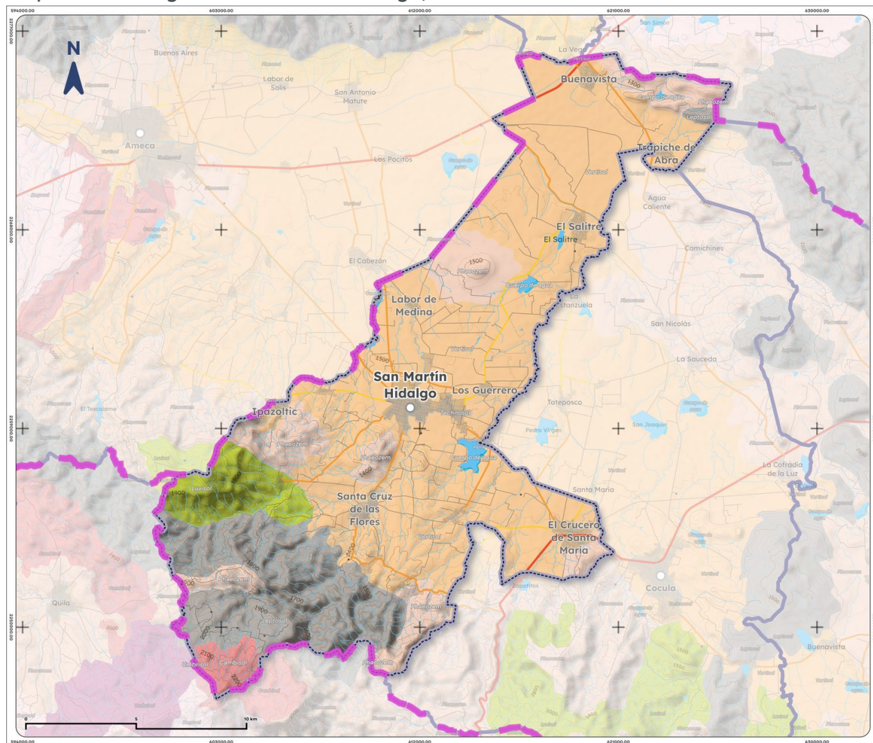
Mapa 4. Edafología de San Martín Hidalgo, 2025
