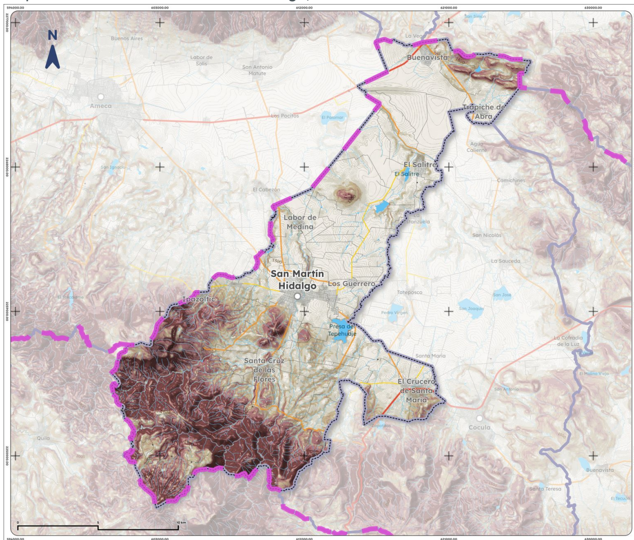
Mapa 5. Pendientes de San Martín Hidalgo, 2025
