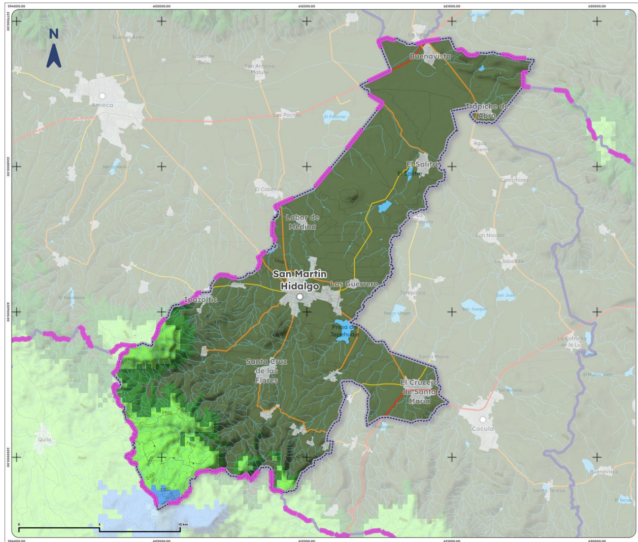
Mapa 10. Clima de San Martín Hidalgo, 1995-2025
