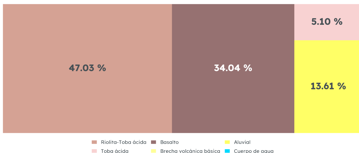
Geología de San Marcos, 1988
