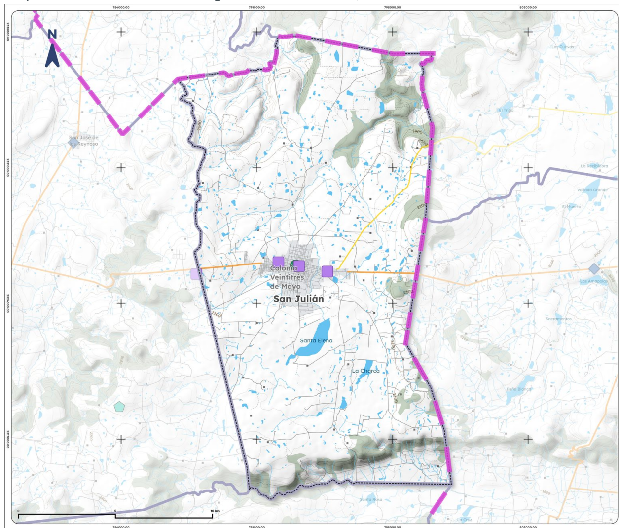
Mapa 22. Infraestructura energética de San Julián, 2025
