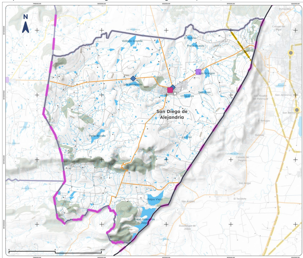
Mapa 22. Infraestructura energética de San Diego de Alejandría, 2025
