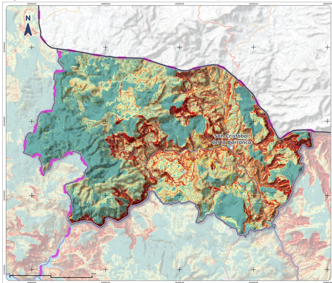
Mapa 17. Erosión efectiva de San Cristóbal de la Barranca, 2025
