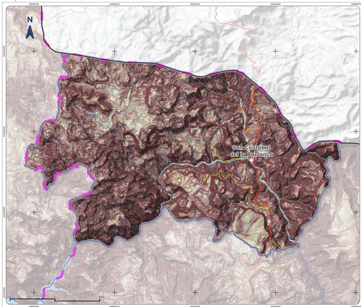
Mapa 5. Pendientes de San Cristóbal de la Barranca, 2025
