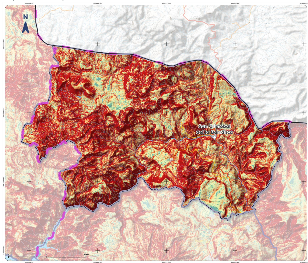
Mapa 16. Erosión potencial de San Cristóbal de la Barranca, 2025
