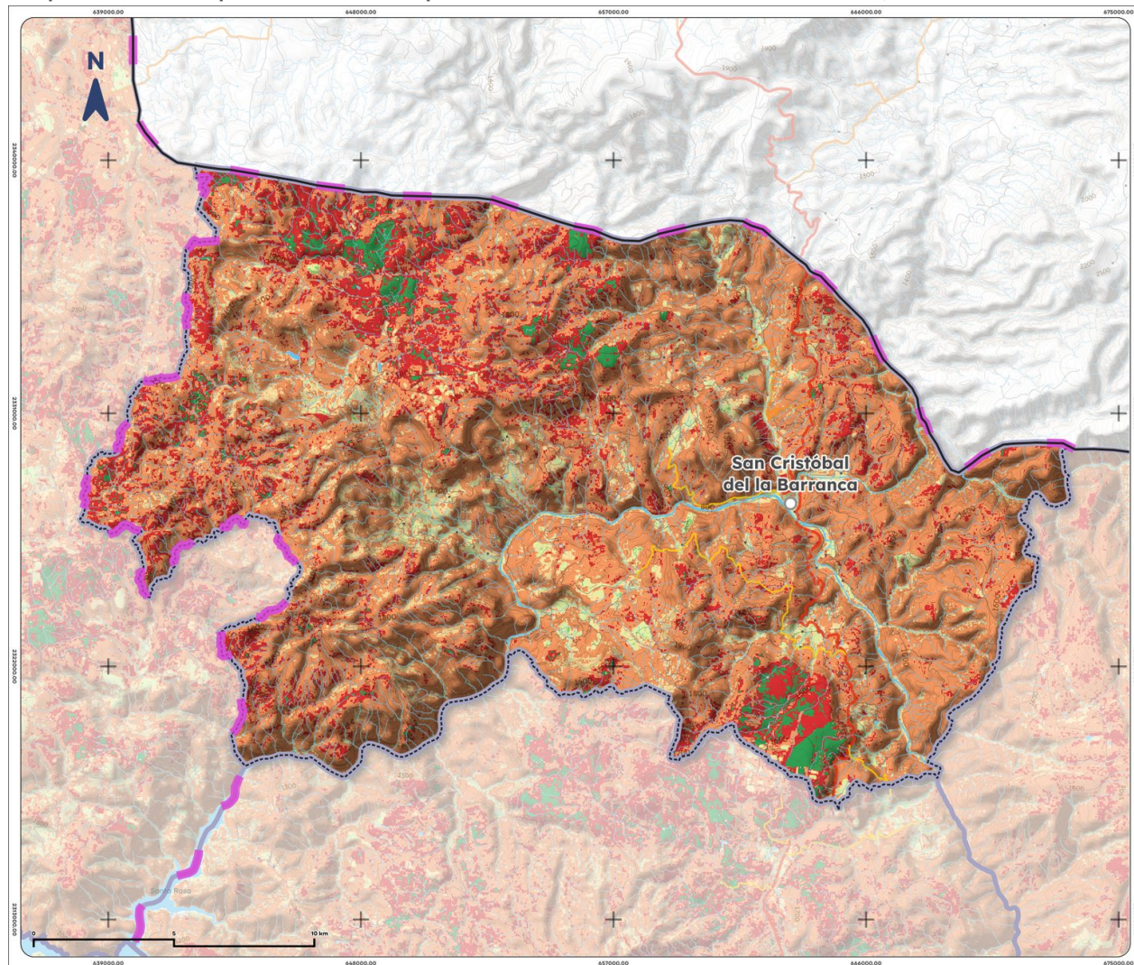
Mapa 15. Índice promedio de sequía de San Cristóbal de la Barranca, 2025
