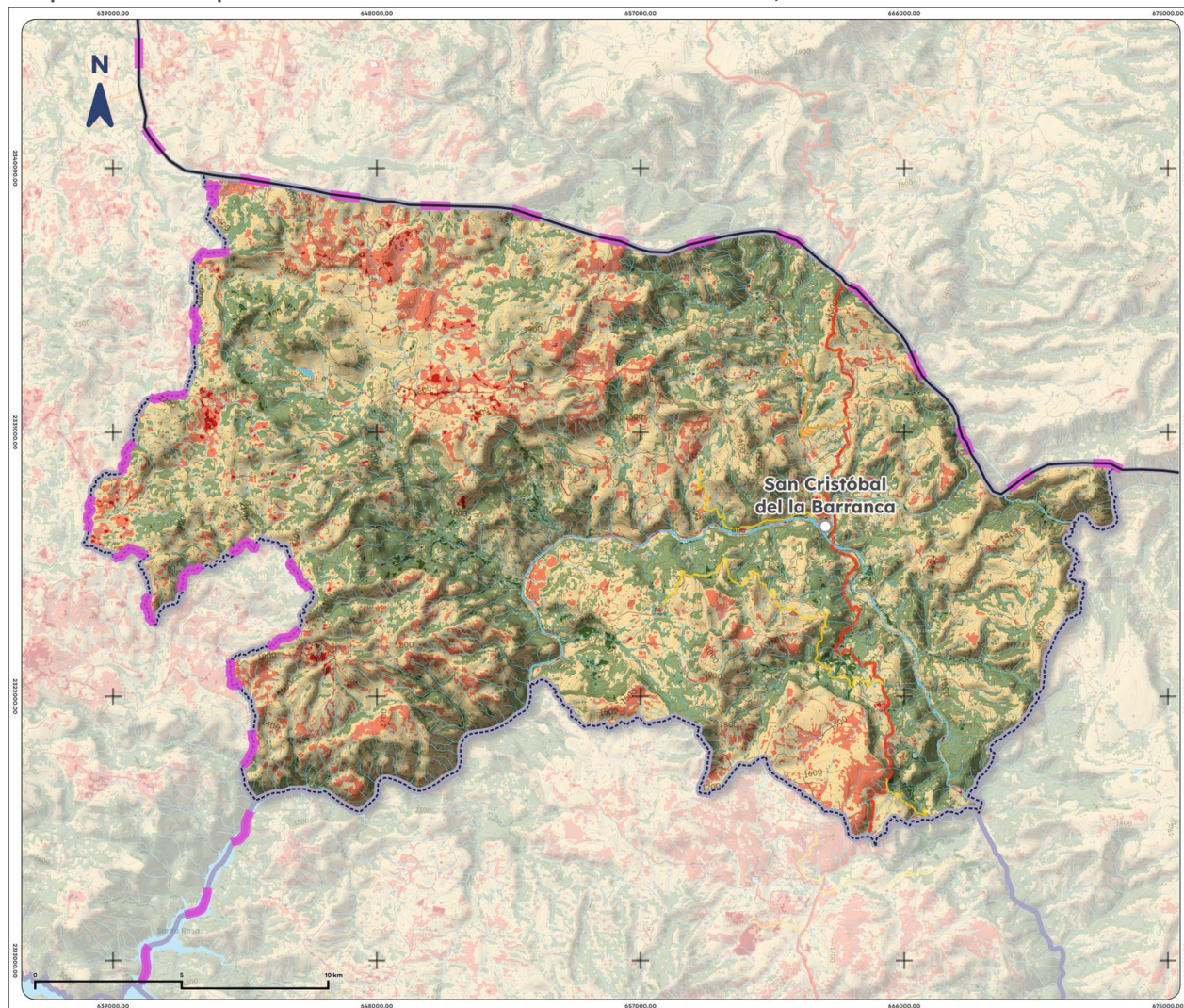
Mapa 12. NDVI promedio de San Cristóbal de la Barranca, 2025
