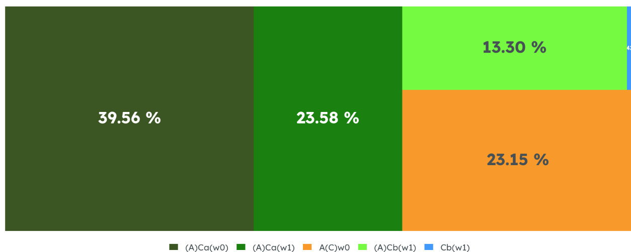
Clima de San Cristóbal de la Barranca, 1995-2025
