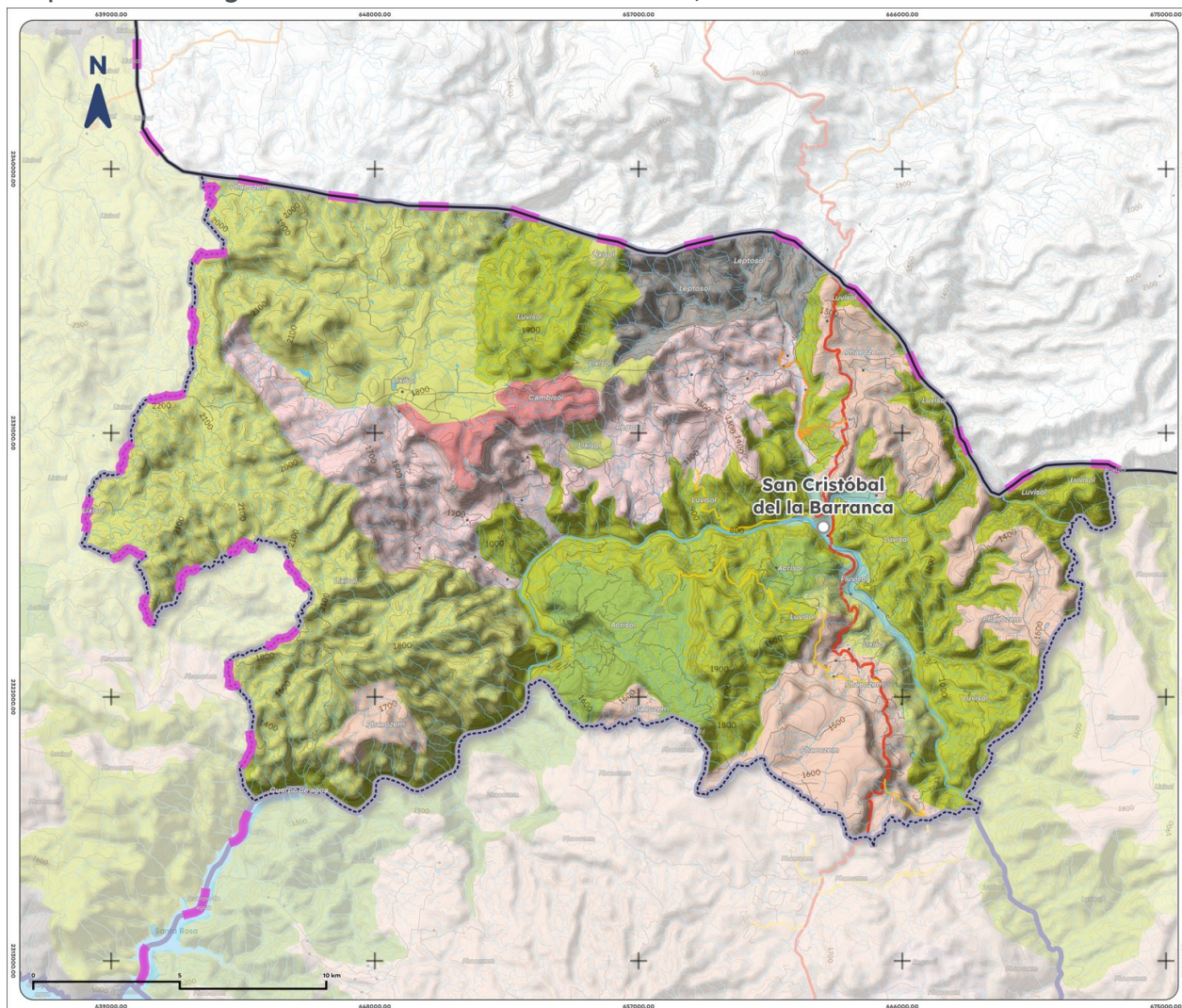
Mapa 4. Edafología de San Cristóbal de la Barranca, 2025
