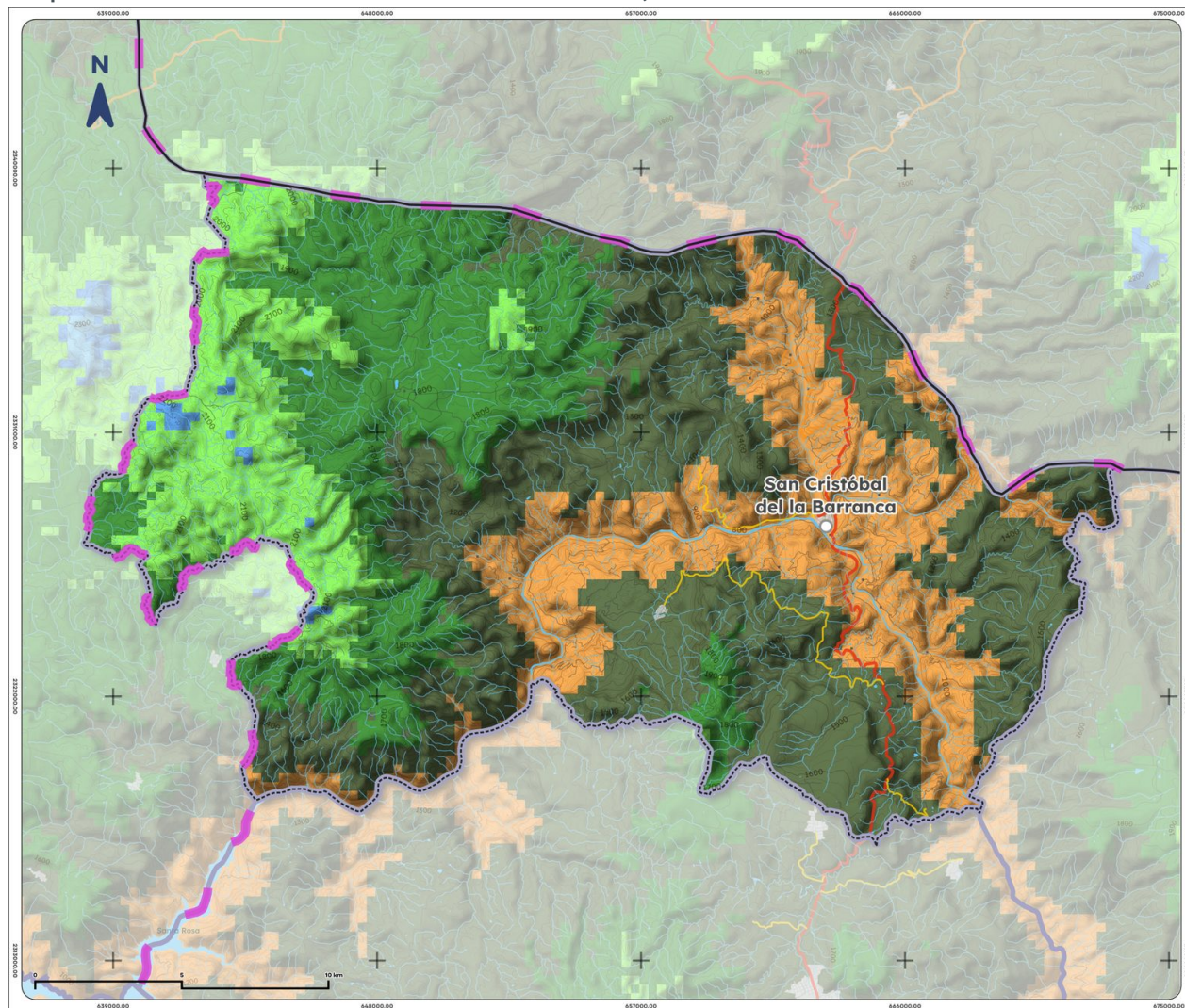
Mapa 10. Clima de San Cristóbal de la Barranca, 1995-2025
