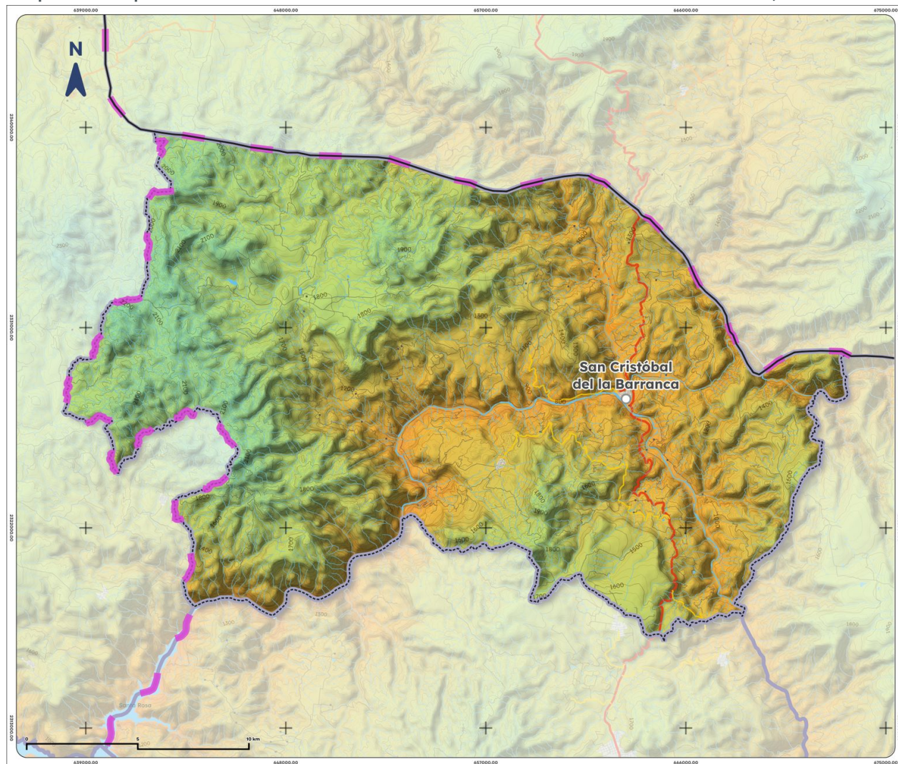
Mapa 8. Temperatura media anual histórica de San Cristóbal de la Barranca, 1995-2025
