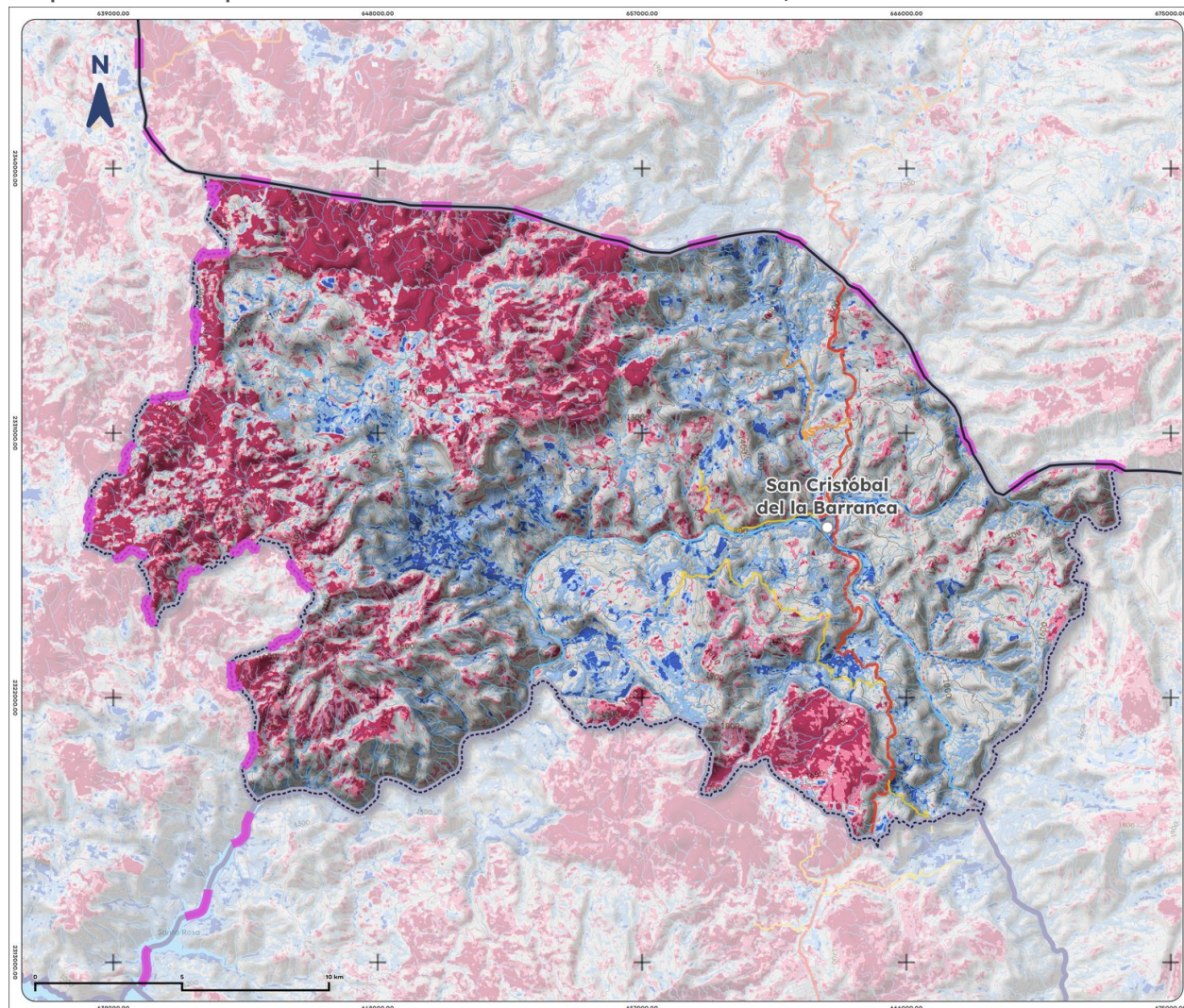
Mapa 13. NDWI promedio de San Cristóbal de la Barranca, 2025
