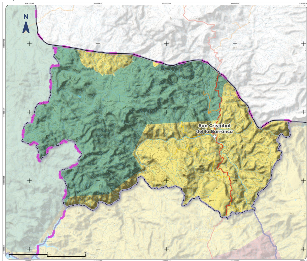
Mapa 7. Acuíferos de San Cristóbal de la Barranca, 2023
