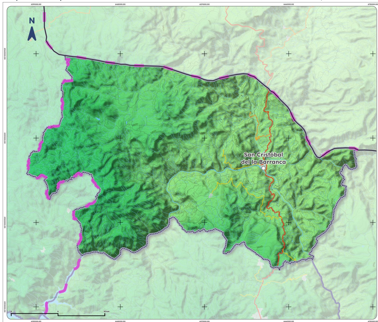
Mapa 9. Precipitación histórica acumulada de San Cristóbal de la Barranca, 1995-2025
