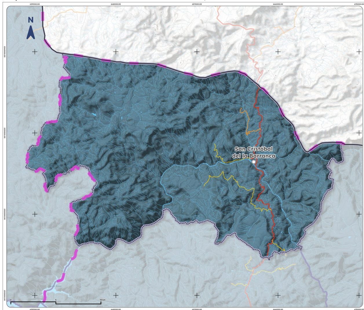
Mapa 6. Cuencas de San Cristóbal de la Barranca, 2023
