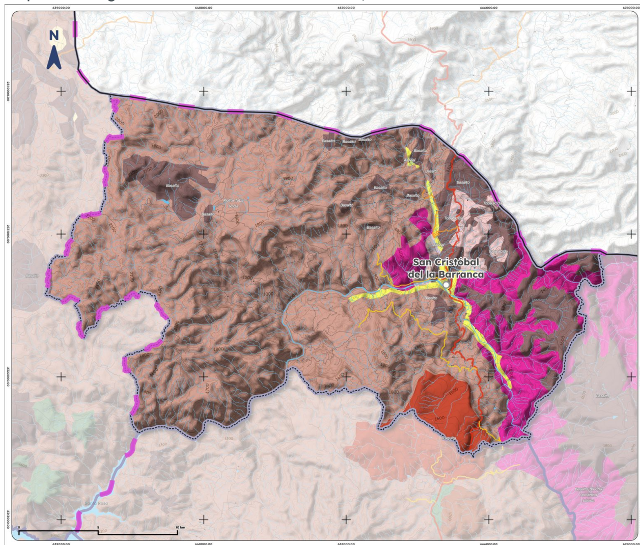
Mapa 3. Geología de San Cristóbal de la Barranca, 1988
