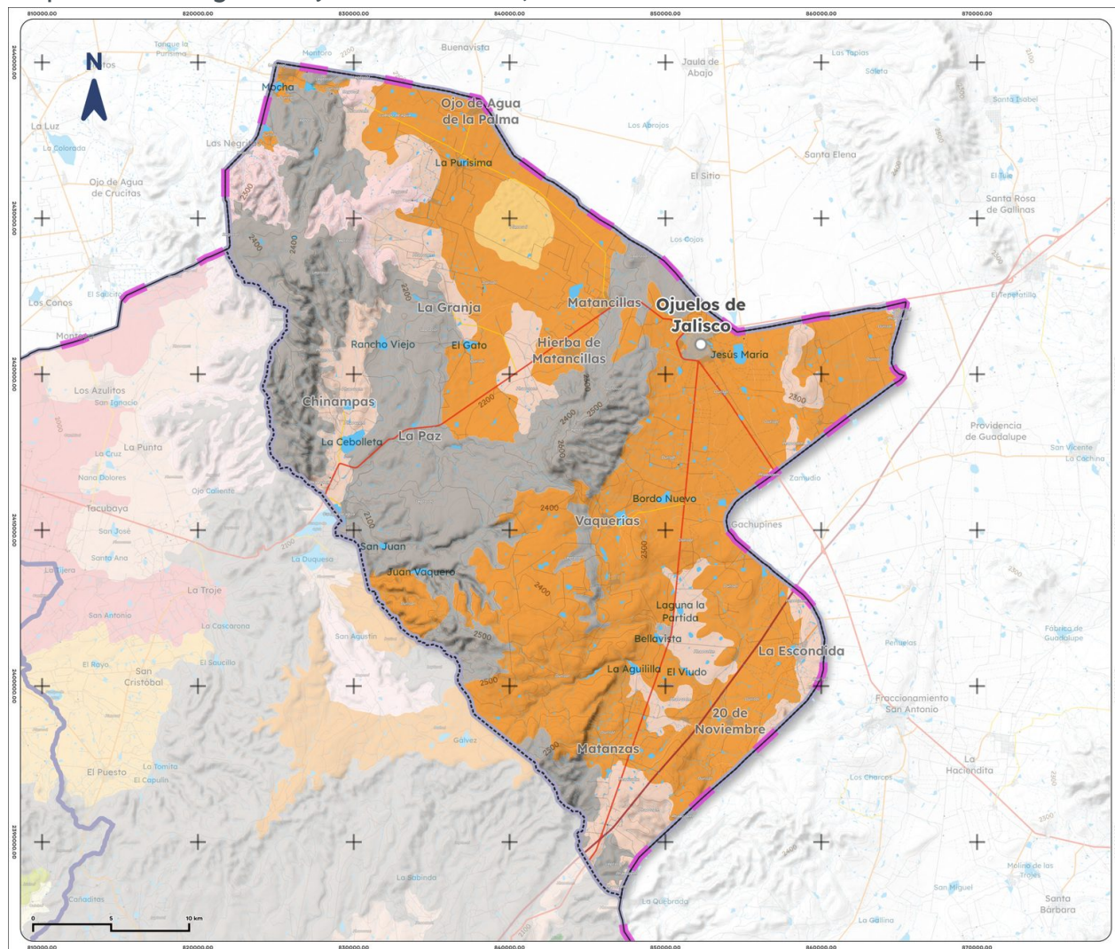
Mapa 4. Edafología de Ojuelos de Jalisco, 2025
