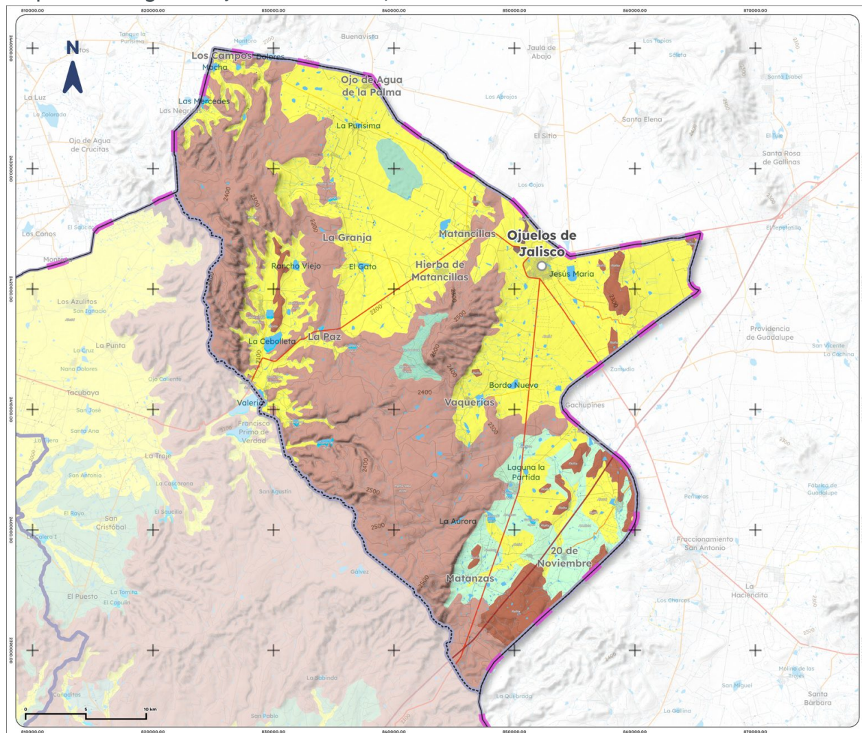
Mapa 3. Geología de Ojuelos de Jalisco, 1988
