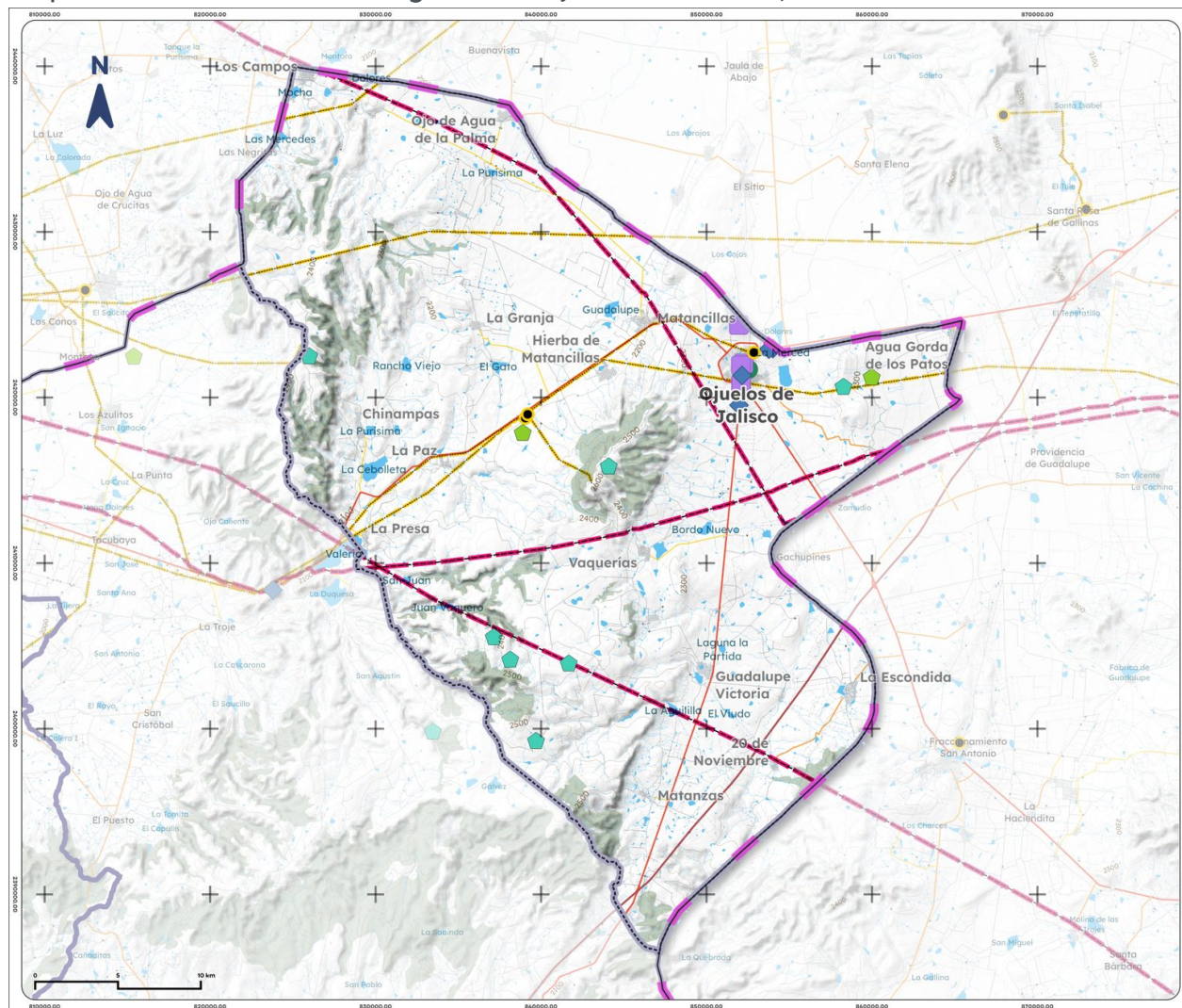
Mapa 22. Infraestructura energética de Ojuelos de Jalisco, 2025
