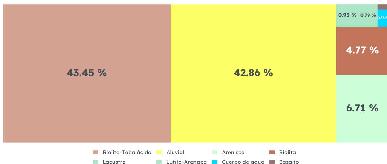
Geología de Ojuelos de Jalisco, 1988
