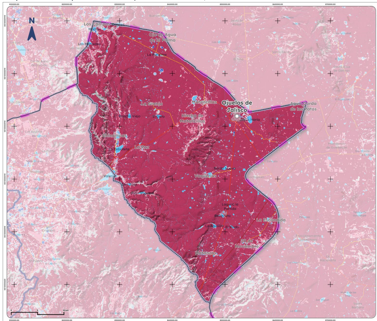
Mapa 13. NDWI promedio de Ojuelos de Jalisco, 2025
