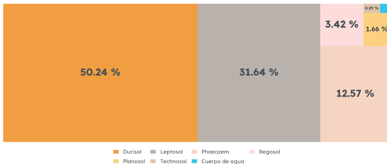
Edafología de Ojuelos de Jalisco, 2025
