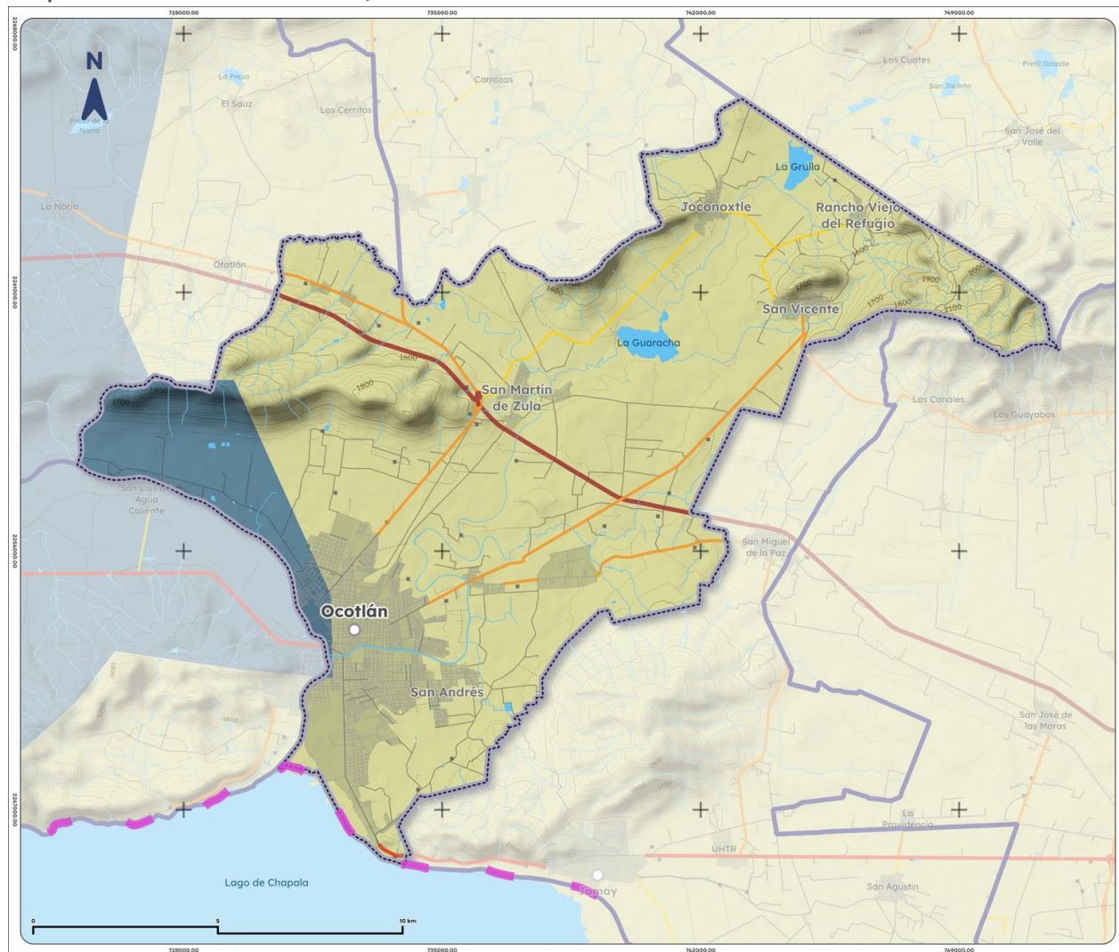
Mapa 6. Cuencas de Ocotlán, 2023
