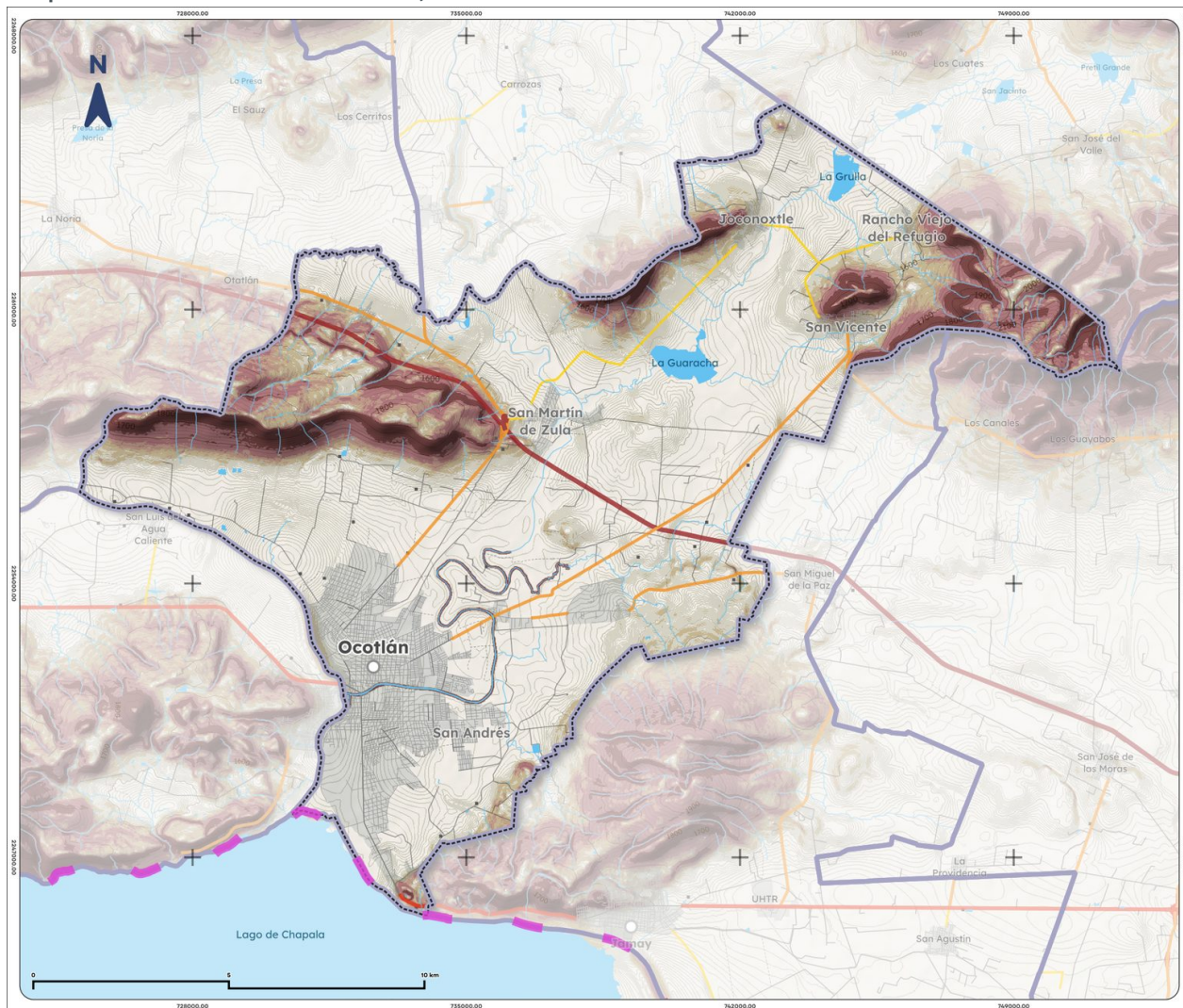
Mapa 5. Pendientes de Ocotlán, 2025
