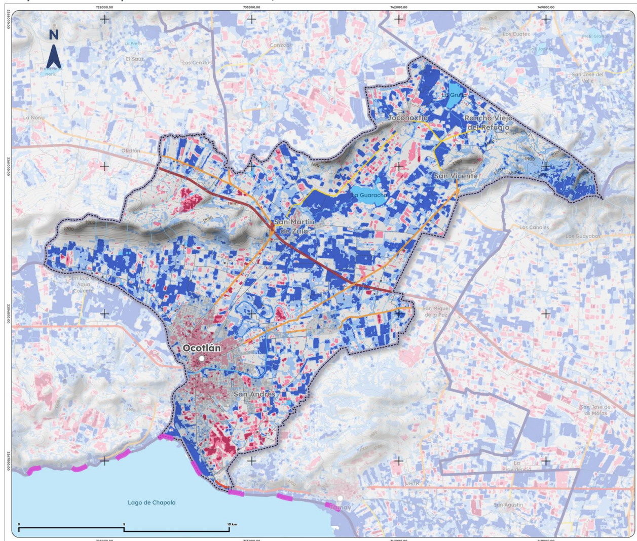
Mapa 13. NDWI promedio de Ocotlán, 2025
