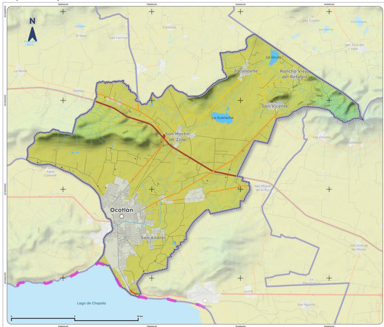
Mapa 8. Temperatura media anual histórica de Ocotlán, 1995-2025
