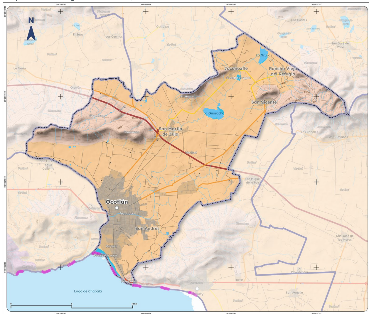
Mapa 4. Edafología de Ocotlán, 2025
