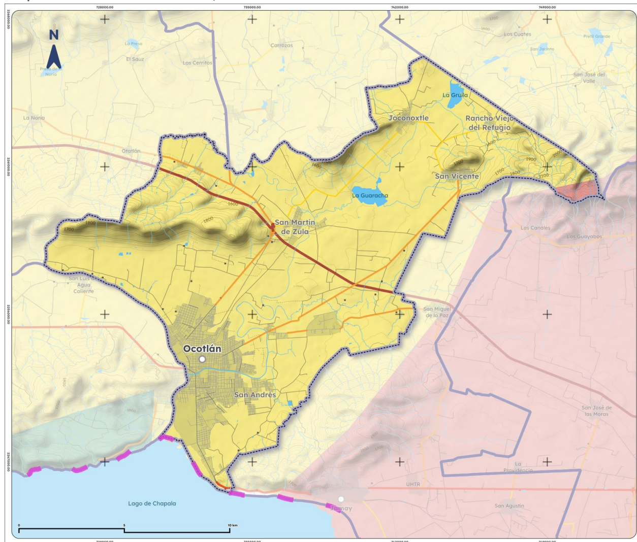
Mapa 7. Acuíferos de Ocotlán, 2023
