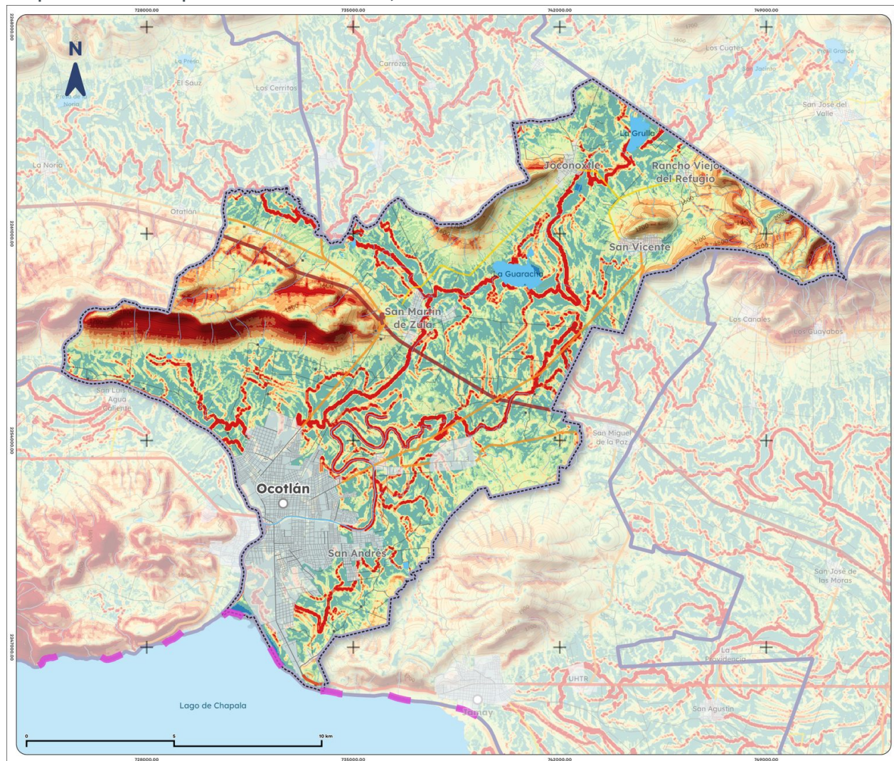
Mapa 16. Erosión potencial de Ocotlán, 2025
