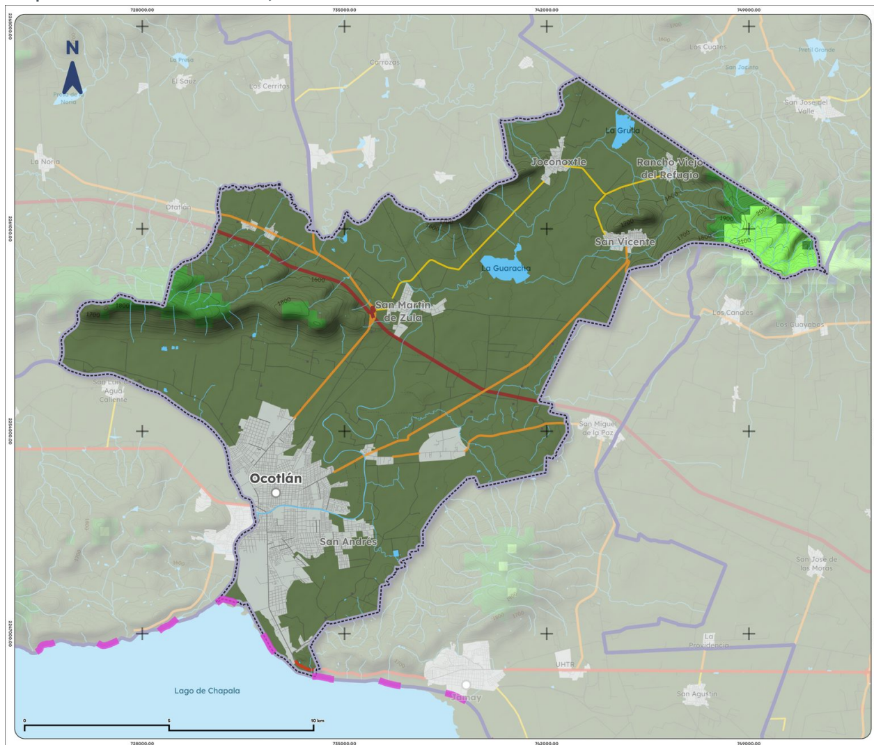
Mapa 10. Clima de Ocotlán, 1995-2025
