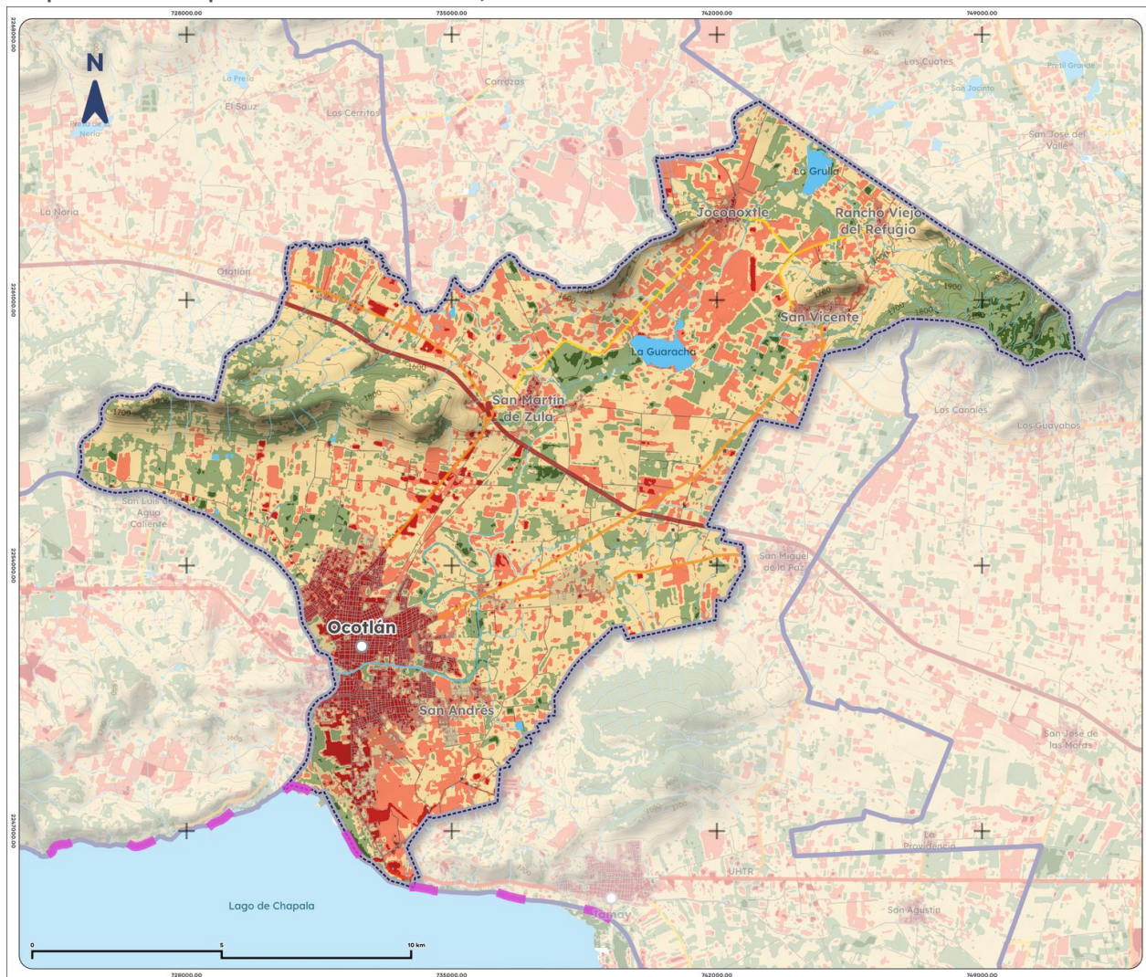
Mapa 12. NDVI promedio de Ocotlán, 2025
