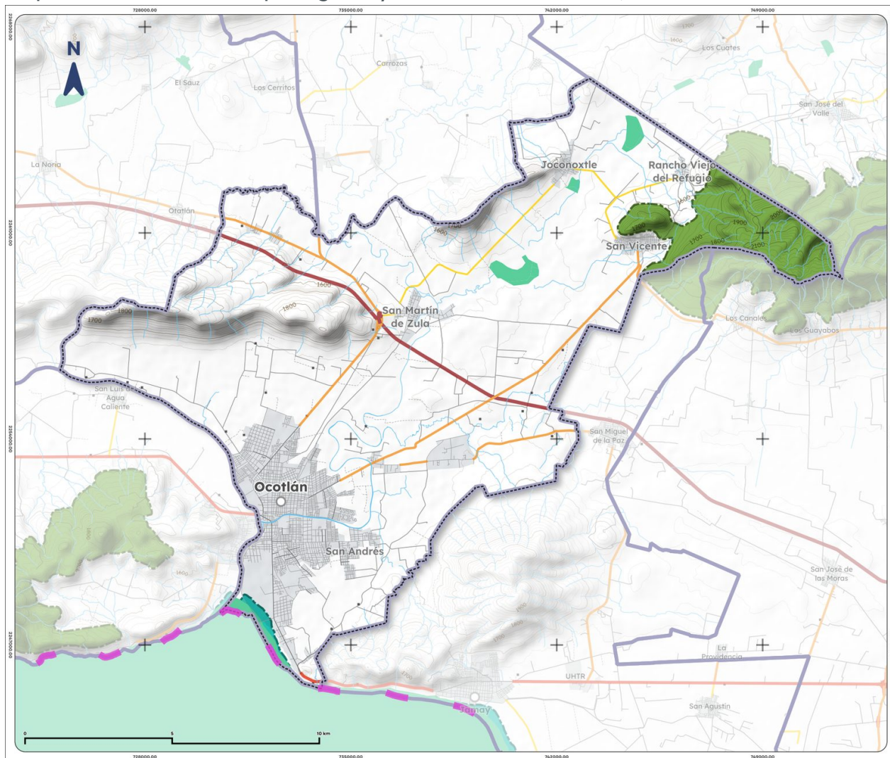
Mapa 14. Áreas naturales protegidas y humedales de Ocotlán, 2025
