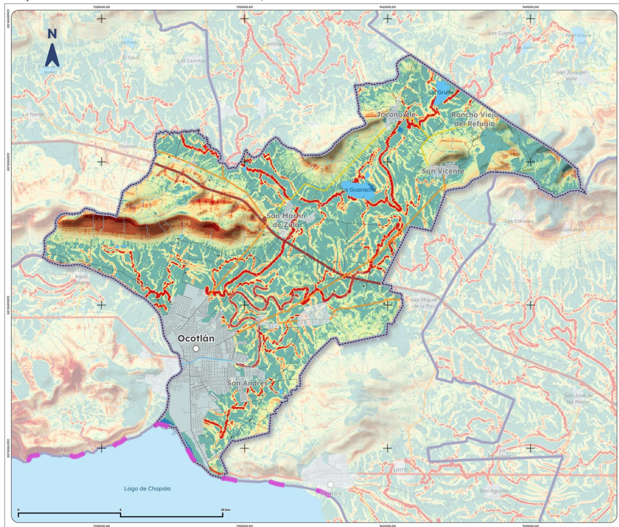
Mapa 17. Erosión efectiva de Ocotlán, 2025
