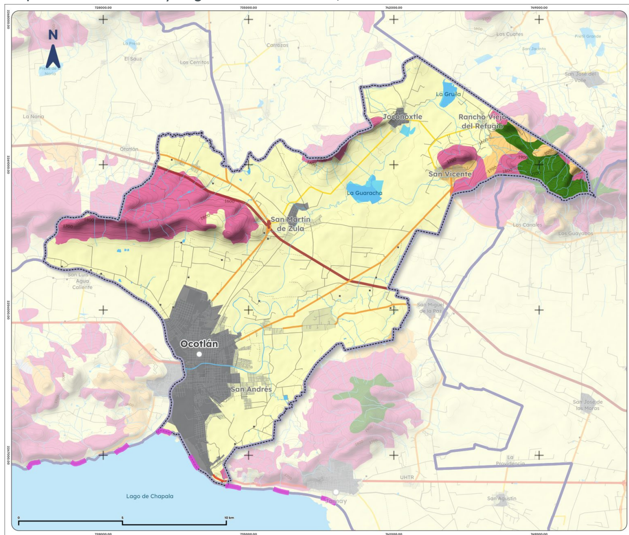
Mapa 11. Uso de suelo y vegetación de Ocotlán, 2018
