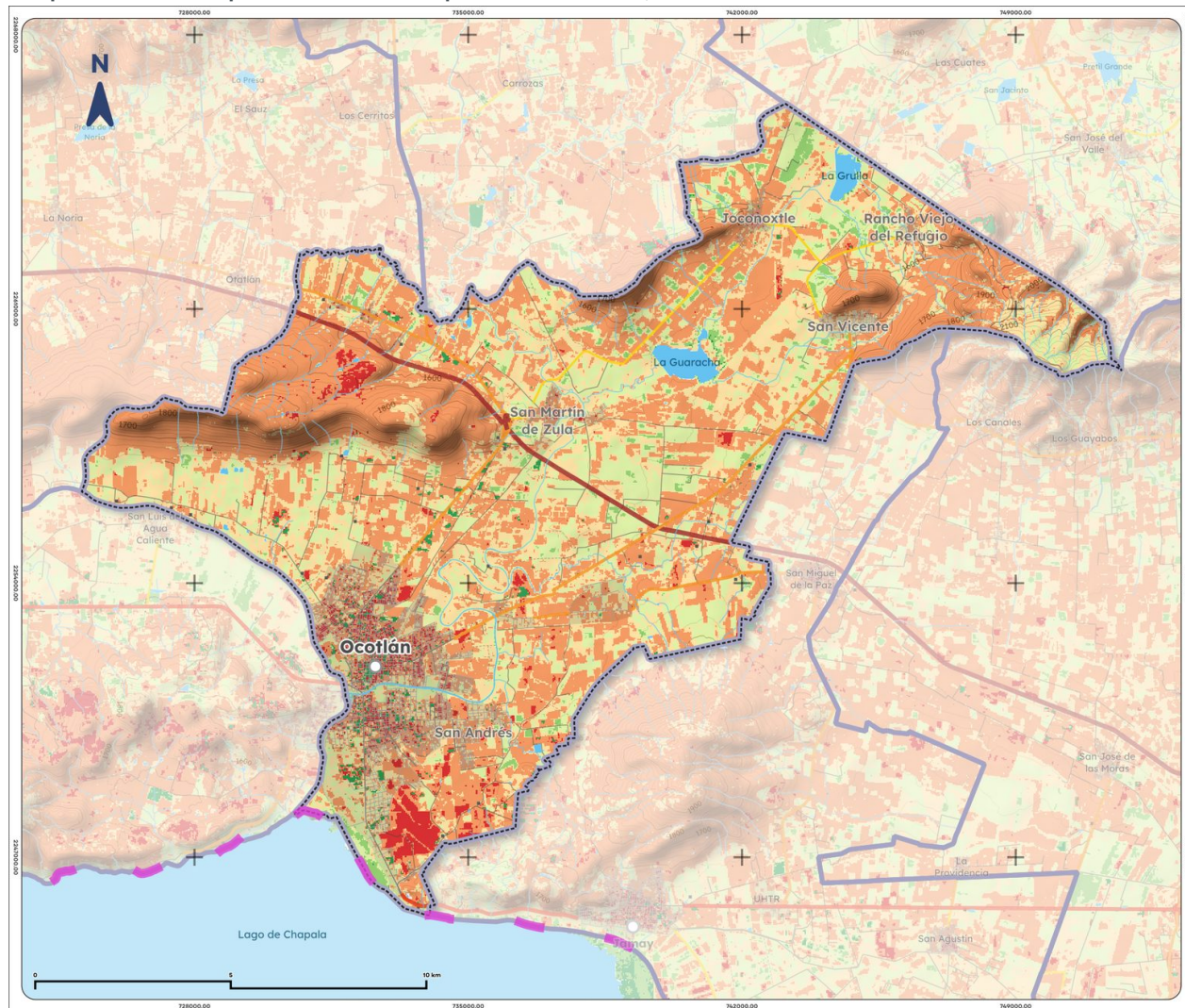
Mapa 15. Índice promedio de sequía de Ocotlán, 2025
