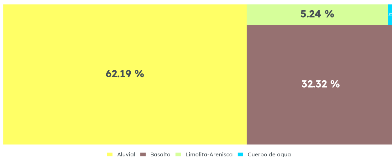
Geología de Ocotlán, 1988
