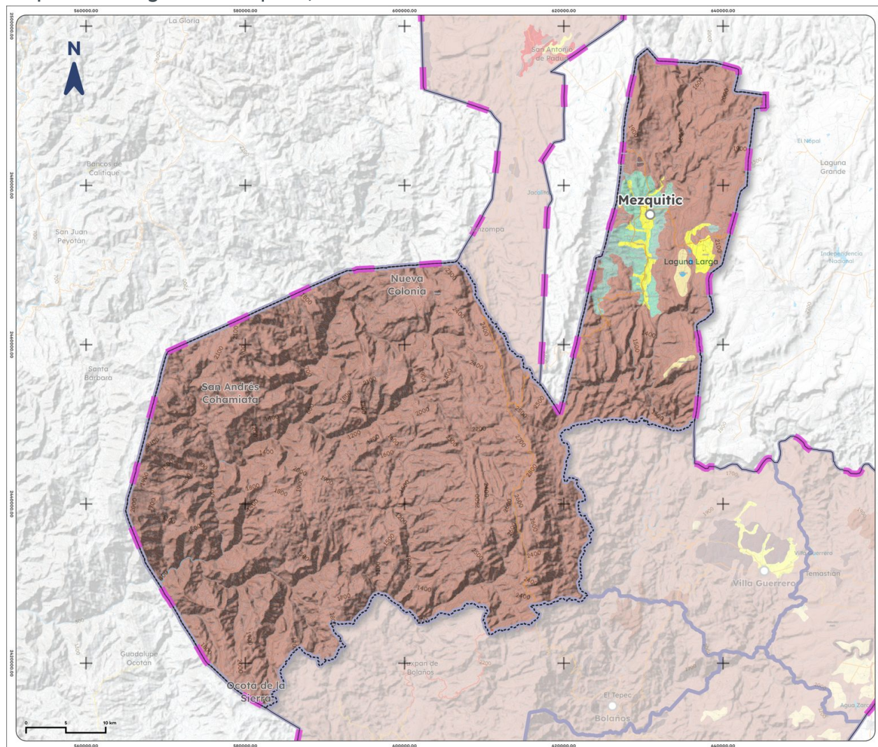
Mapa 3. Geología de Mezquitic, 1988
