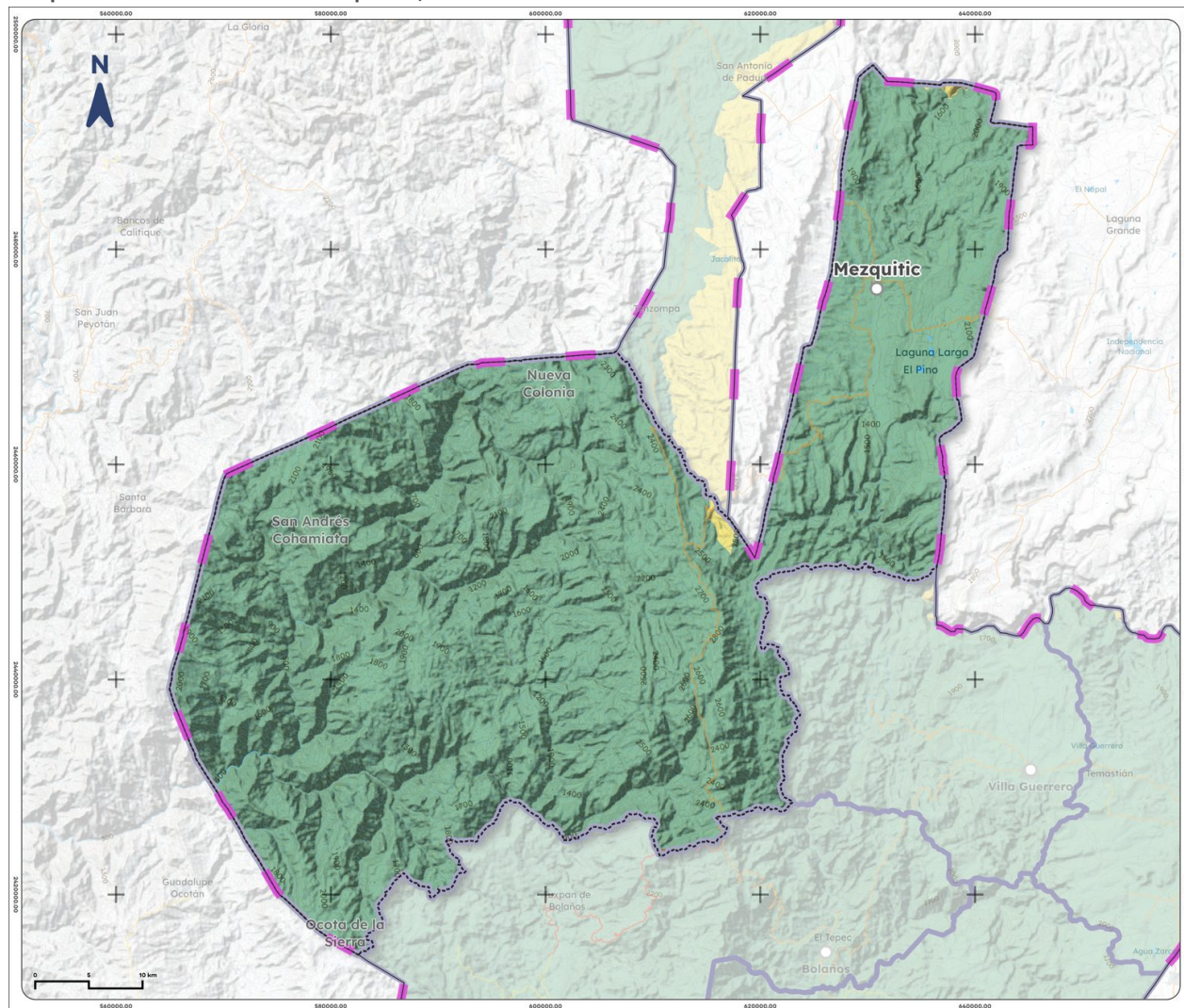
Mapa 7. Acuíferos de Mezquitic, 2023
