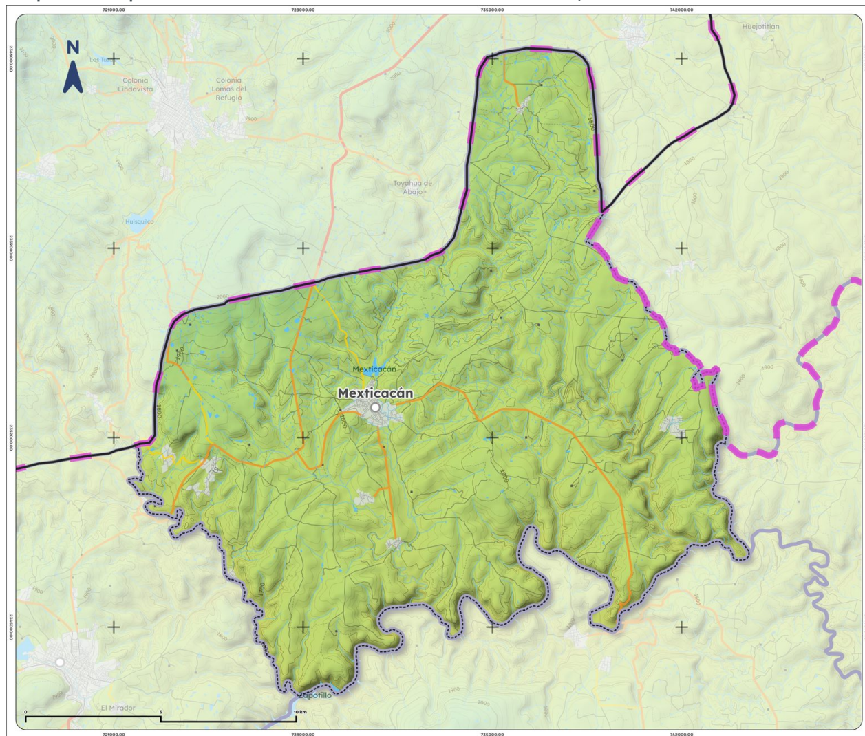
Mapa 8. Temperatura media anual histórica de Mexitacacán, 1995-2025
