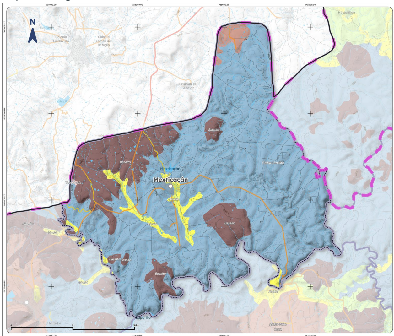
Mapa 3. Geología de Mexitcacán, 1988
