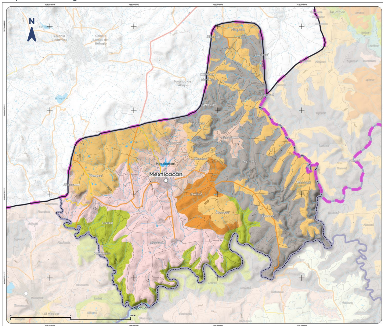
Mapa 4. Edafología de Mexxicacán, 2025
