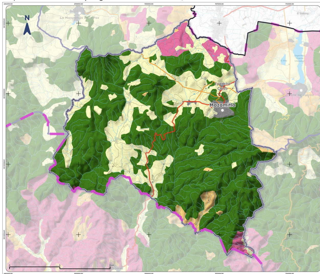
Mapa 11. Uso de suelo y vegetación de Mazamitla, 2018
