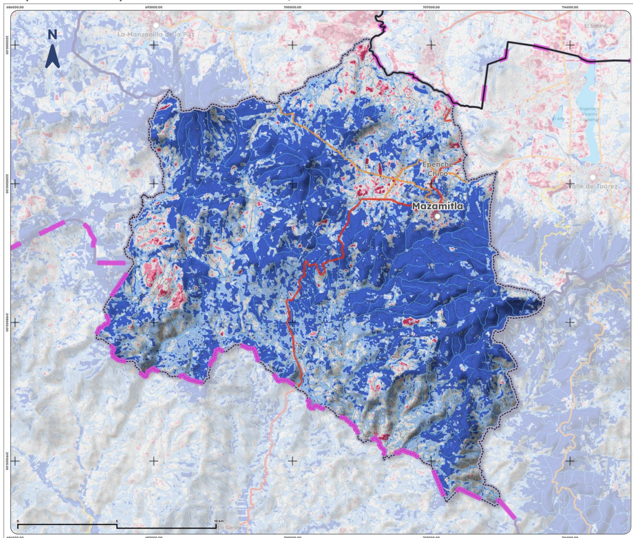
Mapa 13. NDWI promedio de Mazamitla, 2025
