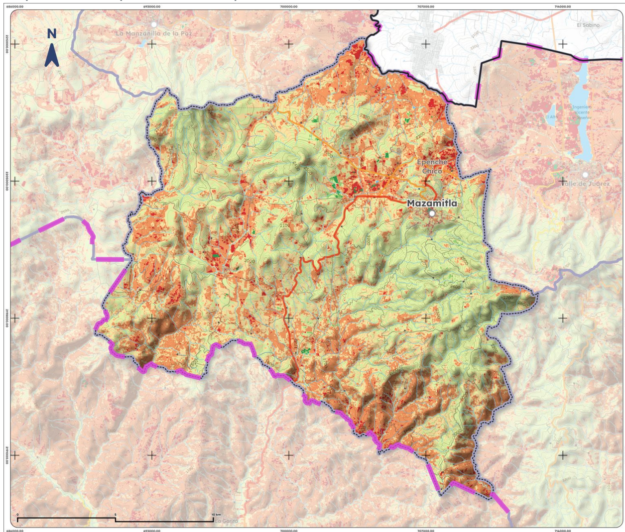
Mapa 15. Índice promedio de sequía de Mazamitla, 2025
