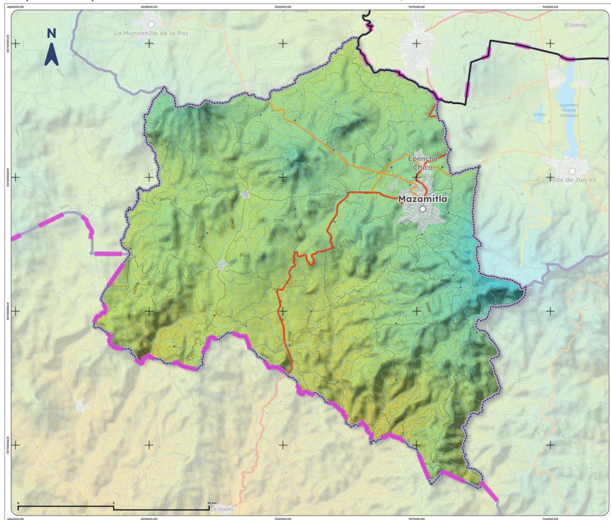
Mapa 8. Temperatura media anual histórica de Mazamitla, 1995-2025
