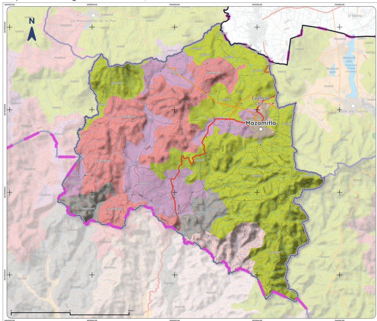
Mapa 4. Edafología de Mazamitla, 2025
