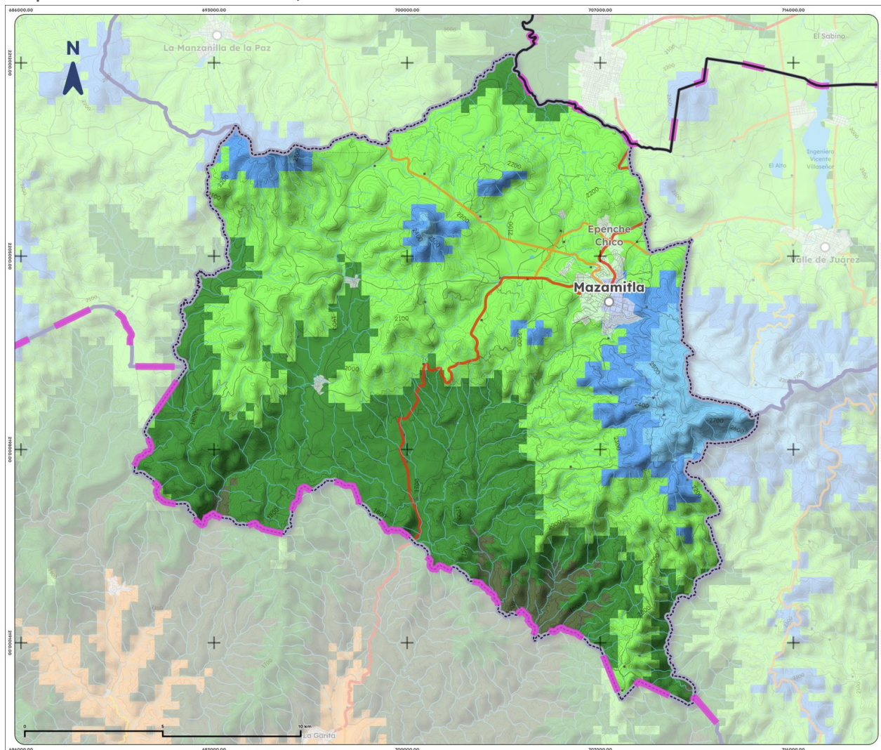
Mapa 10. Clima de Mazamitla, 1995-2025
