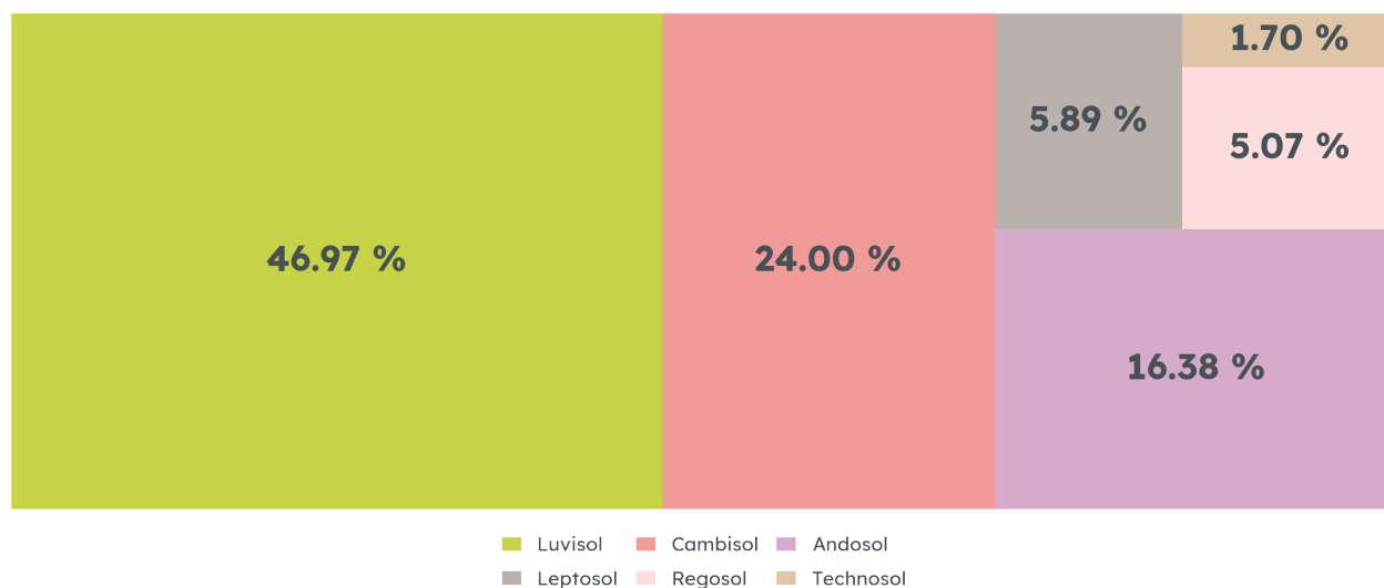
Edafología de Mazamitla, 2025
