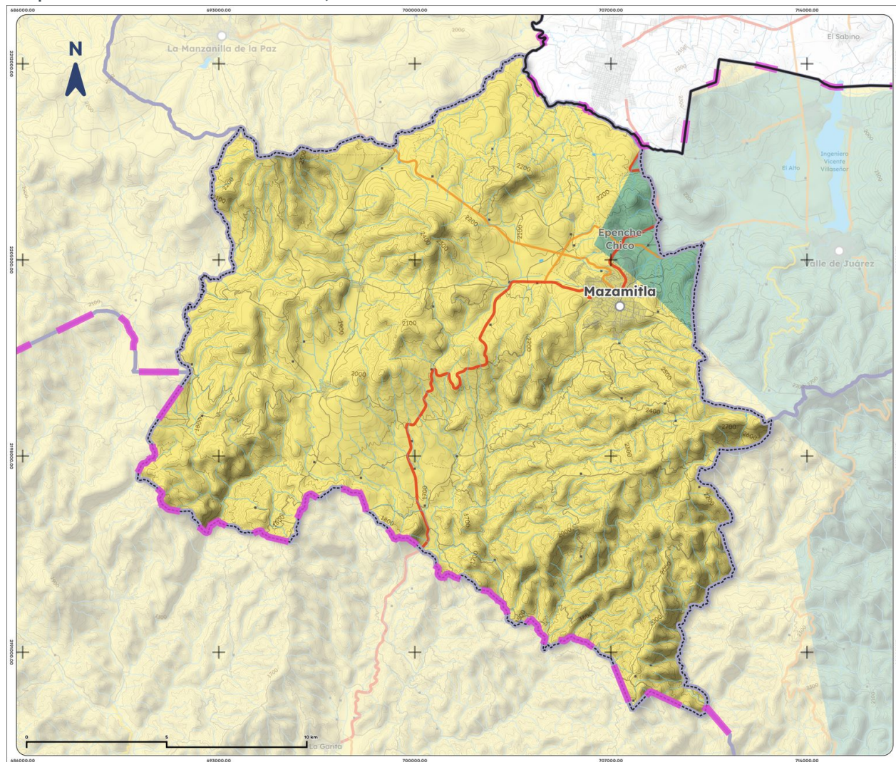
Mapa 7. Acuíferos de Mazamitla, 2023
