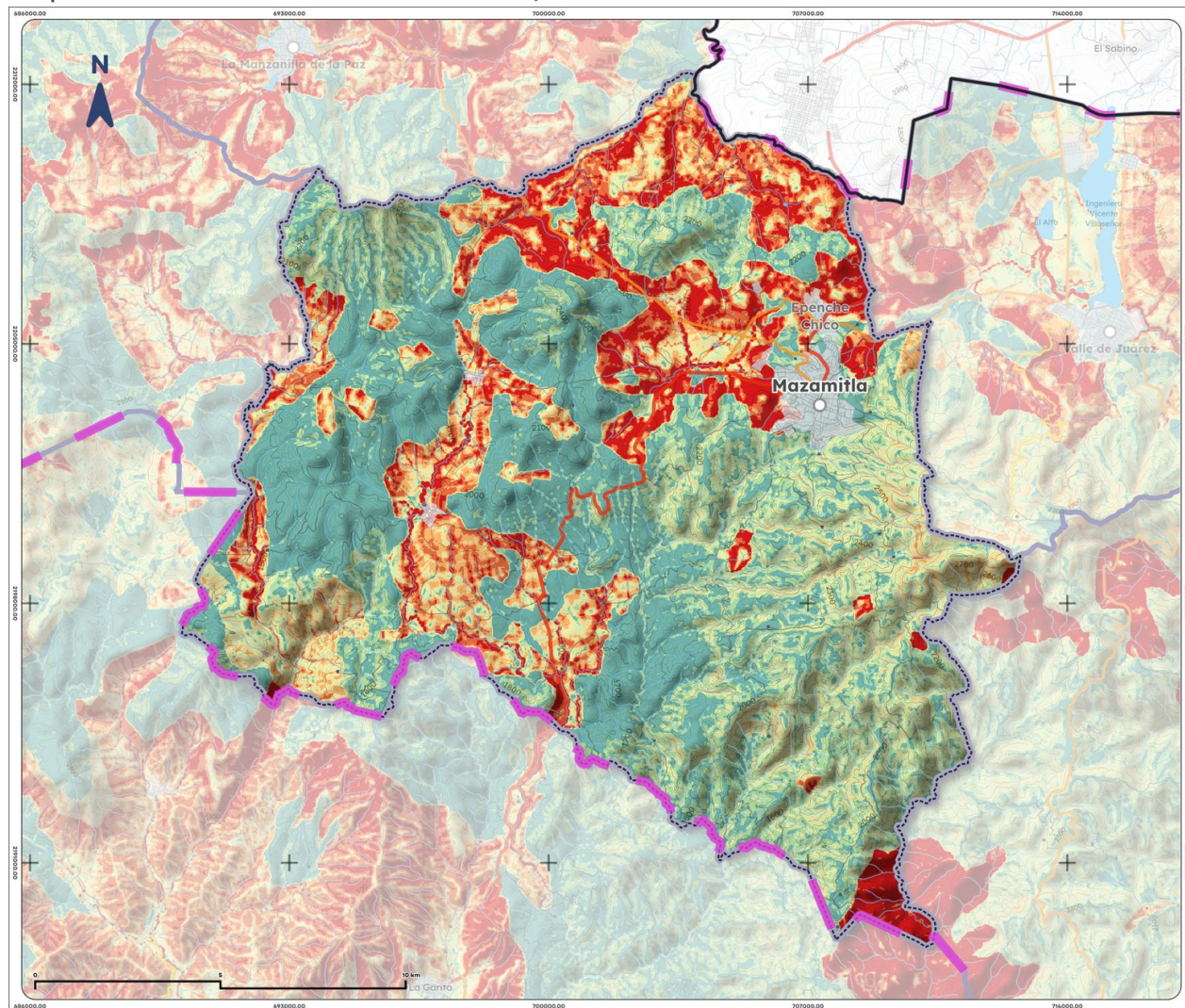
Mapa 17. Erosión efectiva de Mazamitla, 2025
