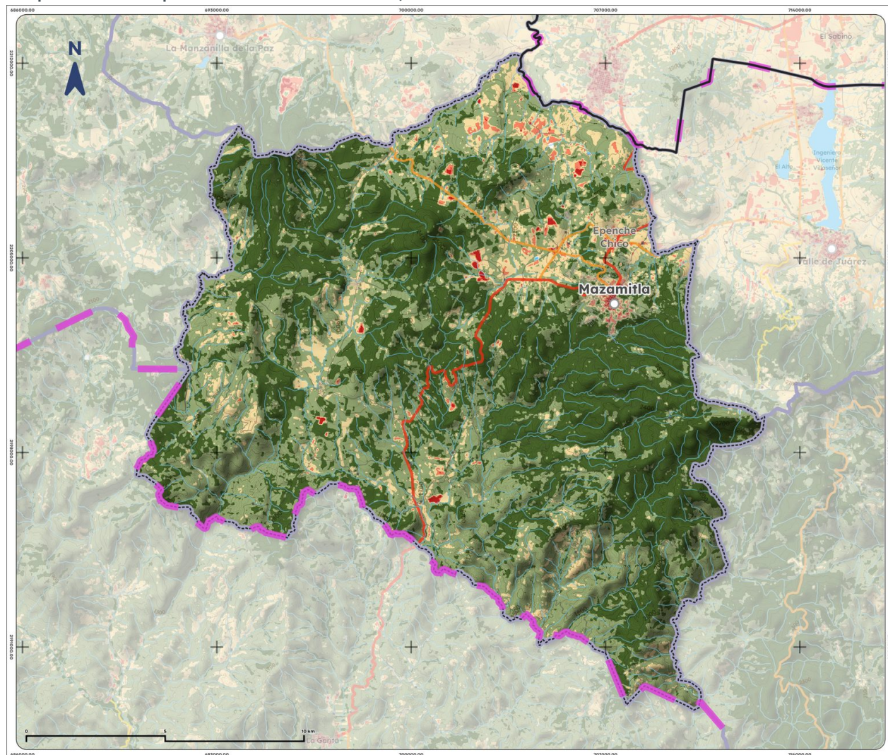
Mapa 12. NDVI promedio de Mazamitla, 2025
