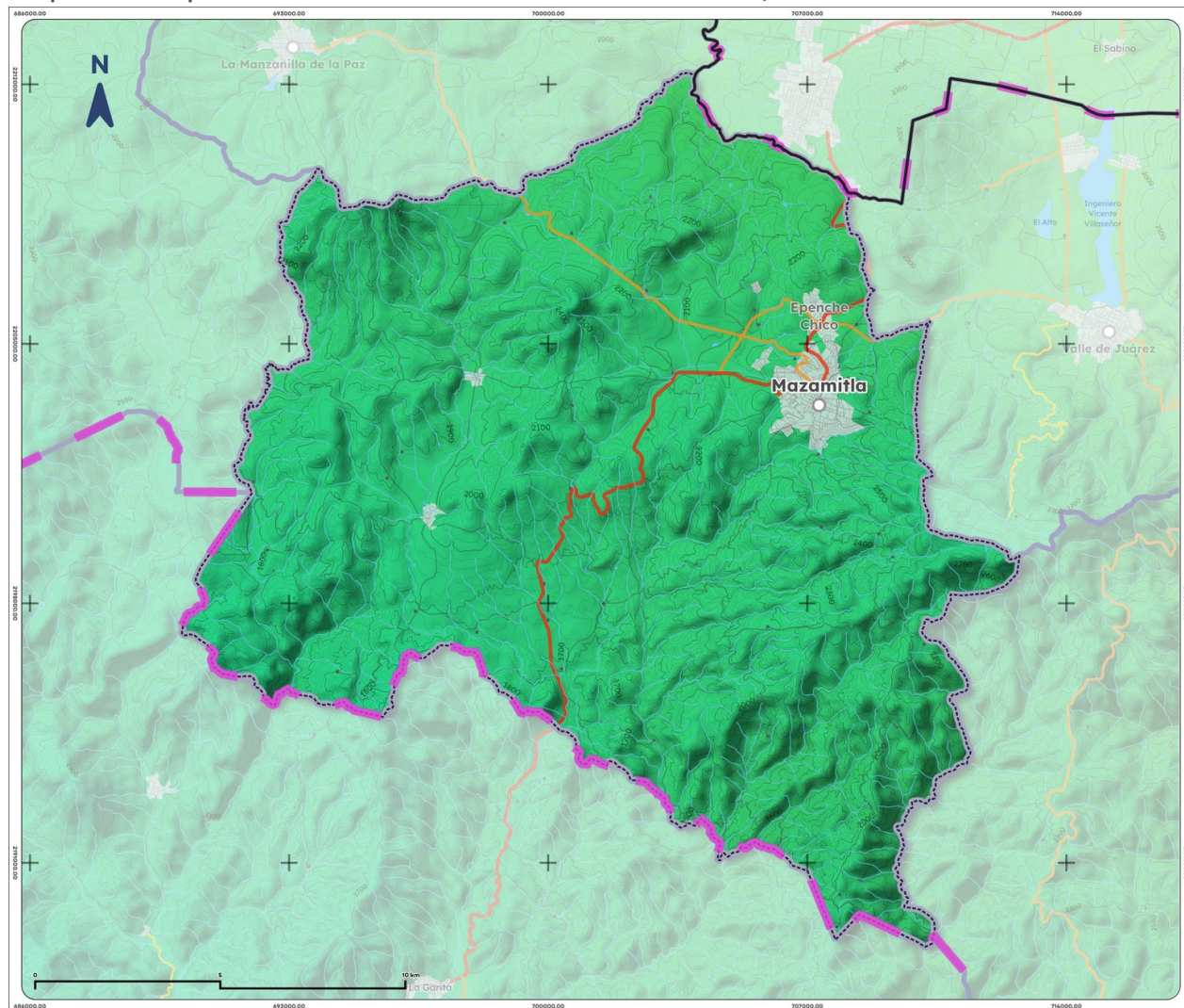
Mapa 9. Precipitación histórica acumulada de Mazamitla, 1995-2025
