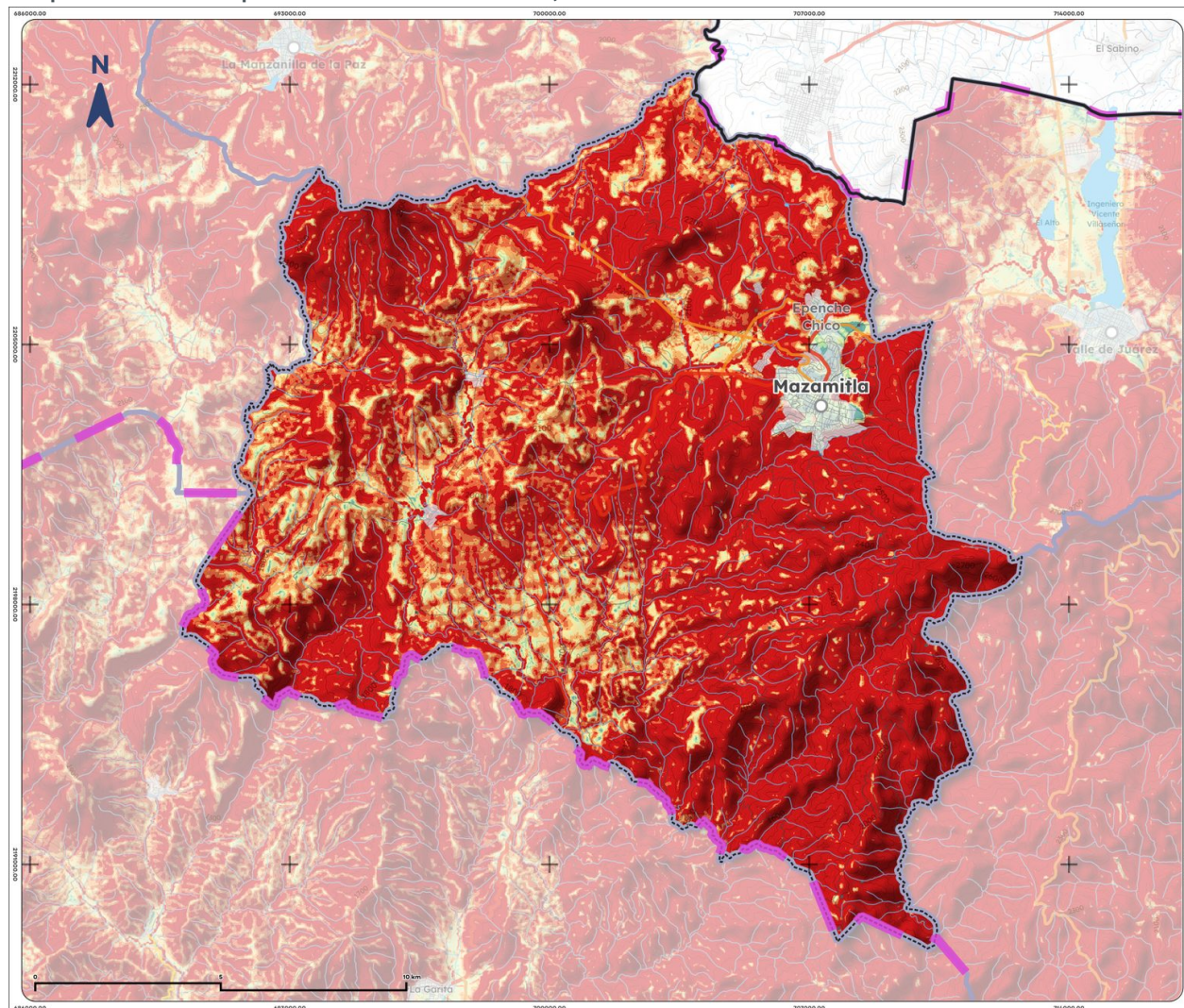
Mapa 16. Erosión potencial de Mazamitla, 2025
