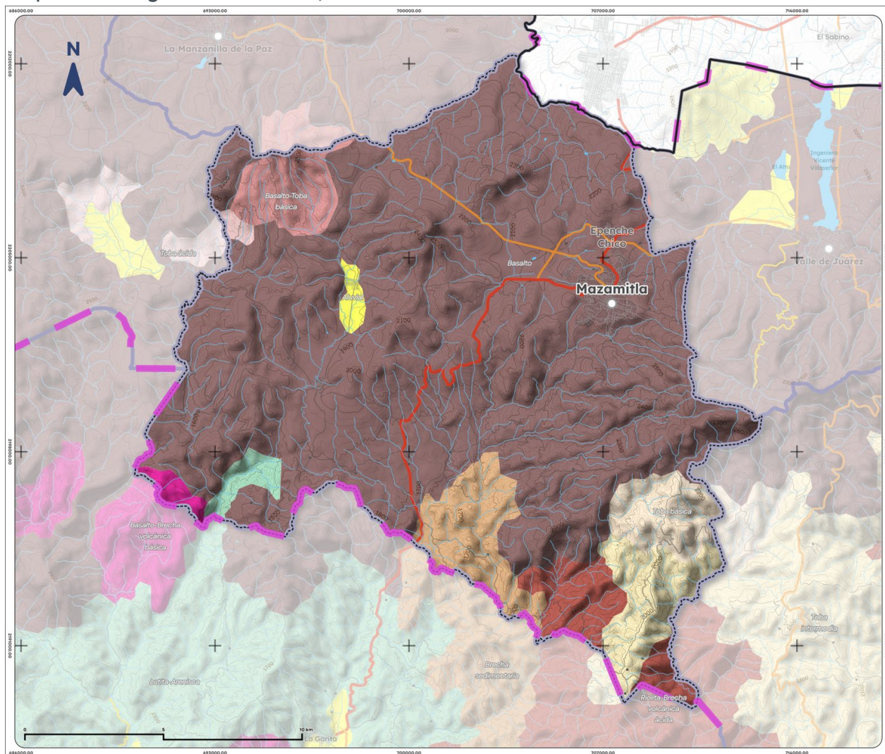
Mapa 3. Geología de Mazamitla, 1988
