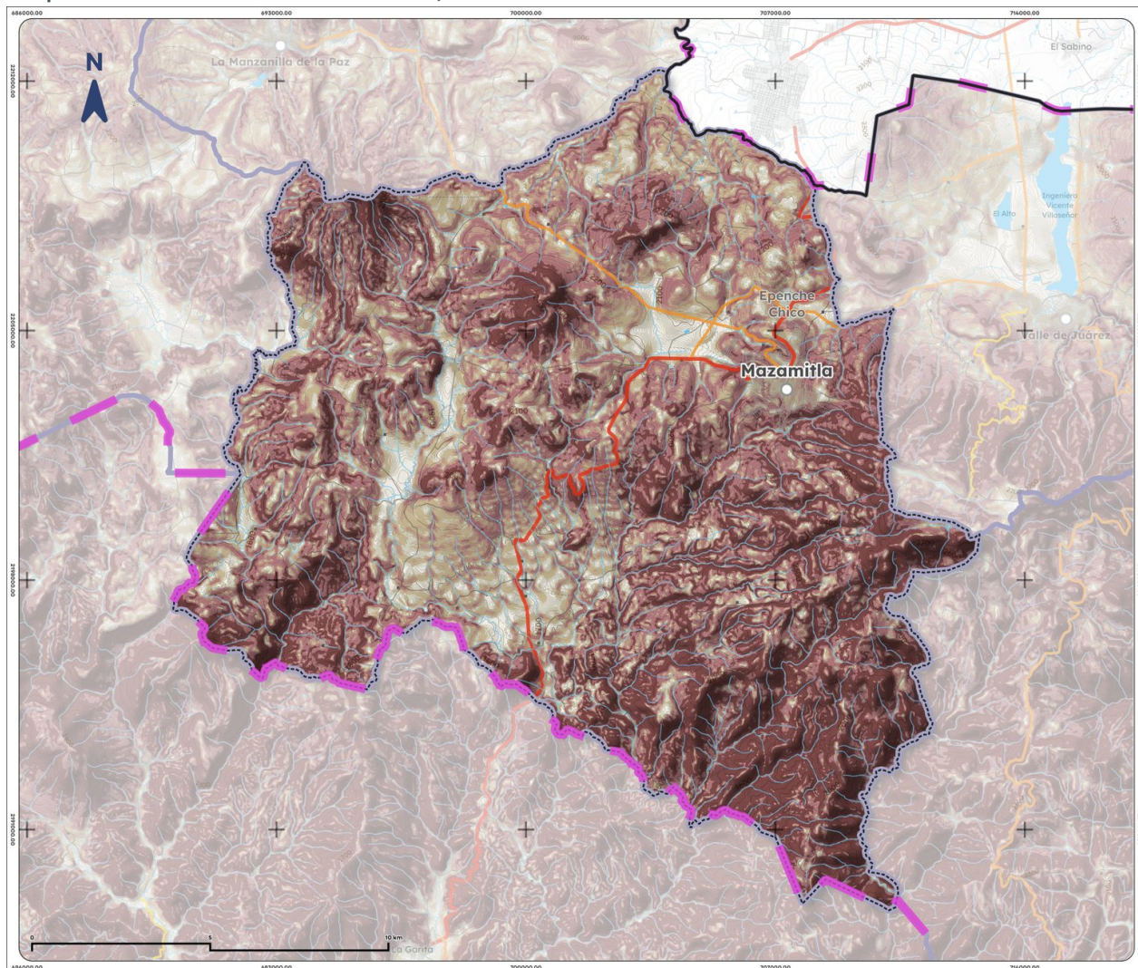
Mapa 5. Pendientes de Mazamitla, 2025
