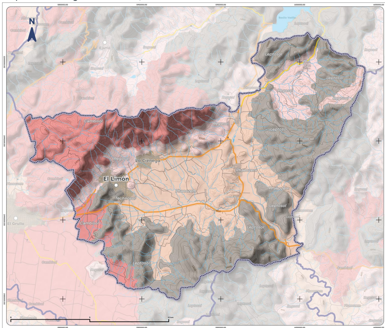
Mapa 4. Edafología de El Limón, 2025
