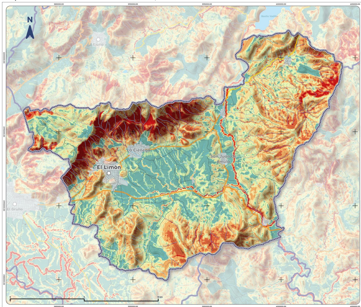
Mapa 17. Erosión efectiva de El Limón, 2025
