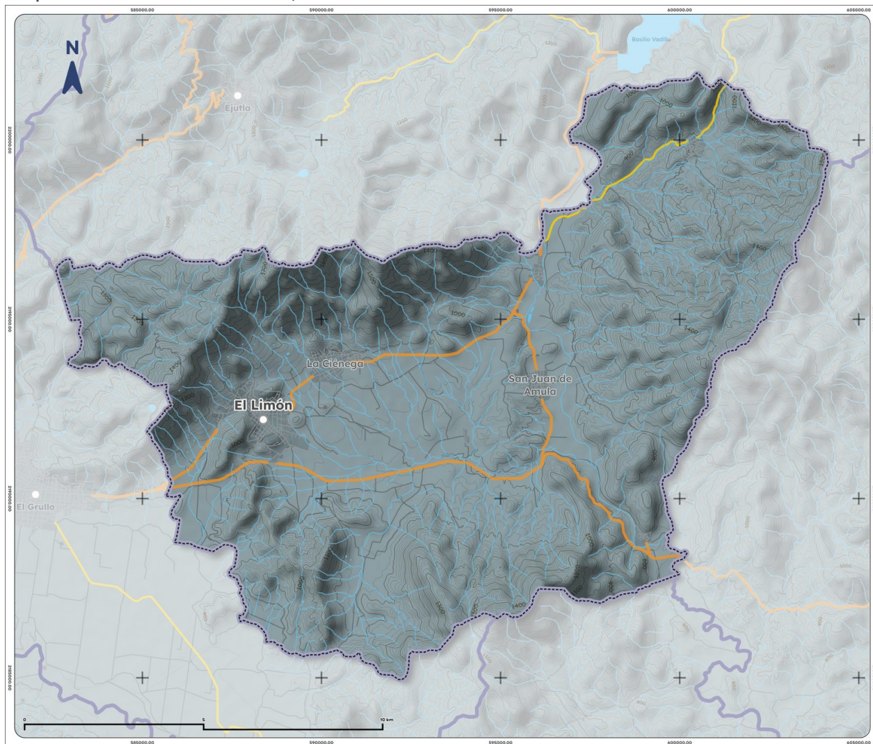
Mapa 6. Cuencas de El Limón, 2023
