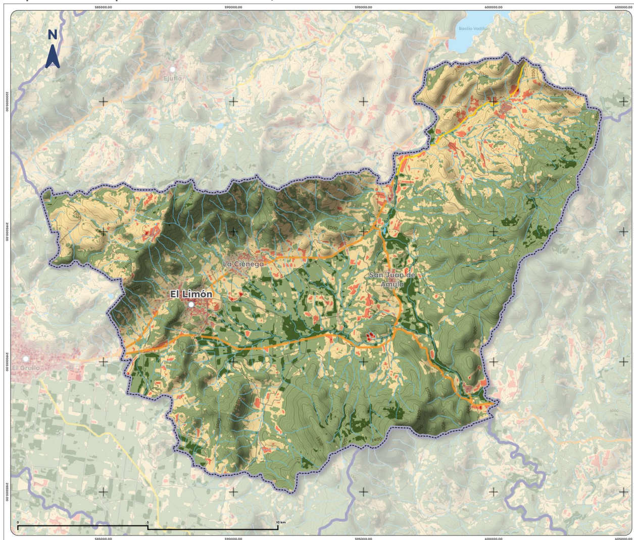
Mapa 12. NDVI promedio de El Limón, 2025
