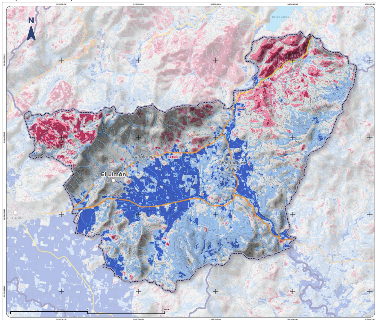
Mapa 13. NDWI promedio de El Limón, 2025
