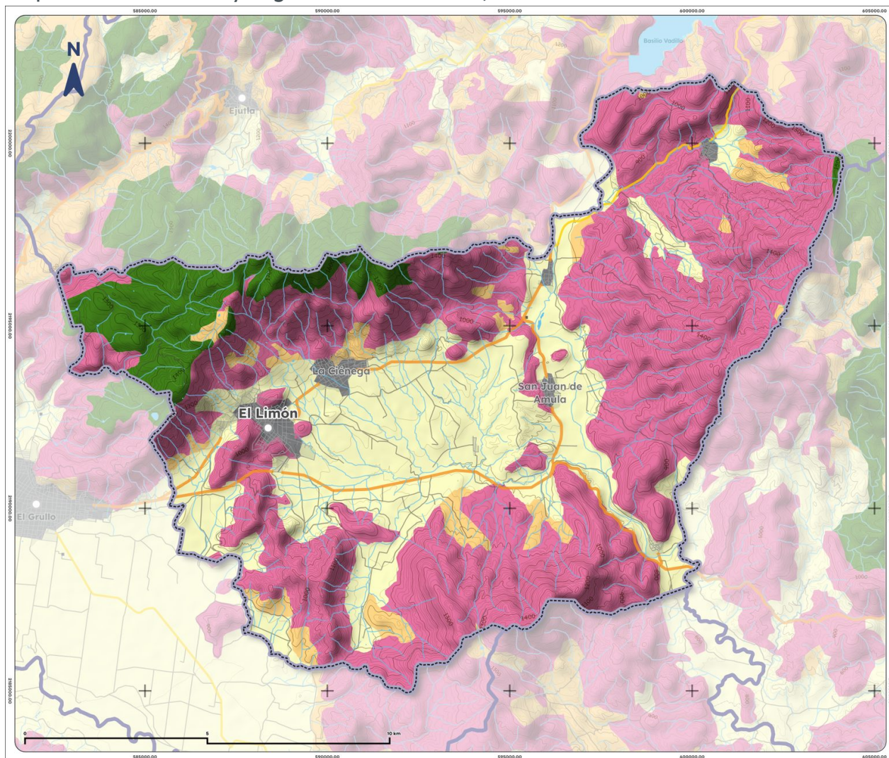
Mapa 11. Uso de suelo y vegetación de El Limón, 2018
