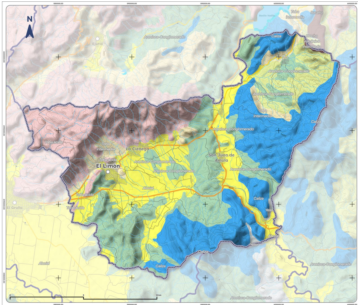
Mapa 3. Geología de El Limón, 1988
