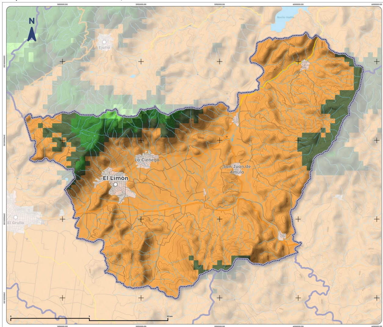
Mapa 10. Clima de El Limón, 1995-2025
