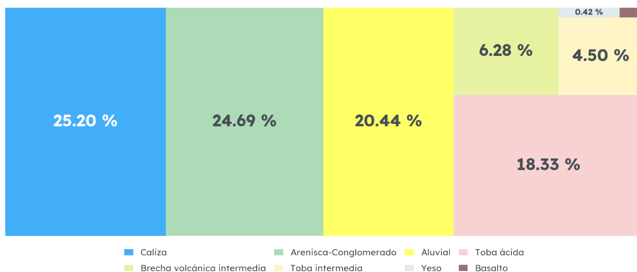
Geología de El Limón, 1988
