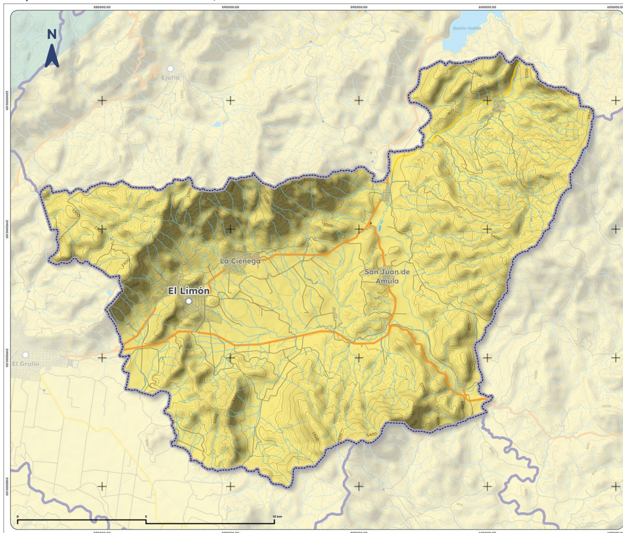
Mapa 7. Acuíferos de El Limón, 2023
