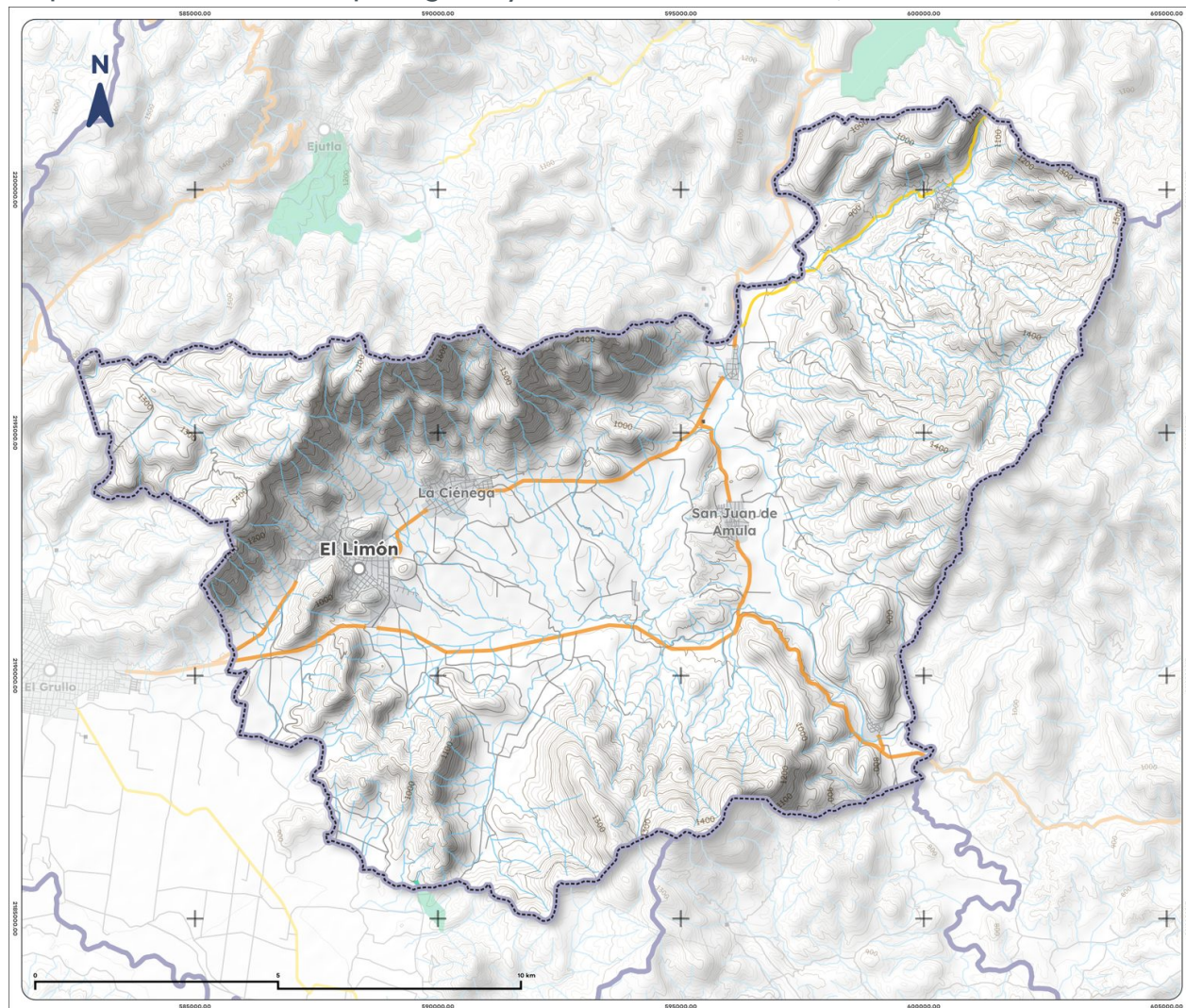
Mapa 14. Áreas naturales protegidas y humedales de El Limón, 2025
