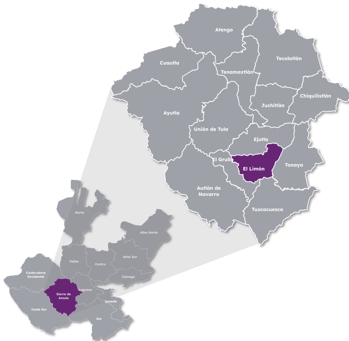
Mapa 1. Localización geográfica de El Limón, Jalisco
