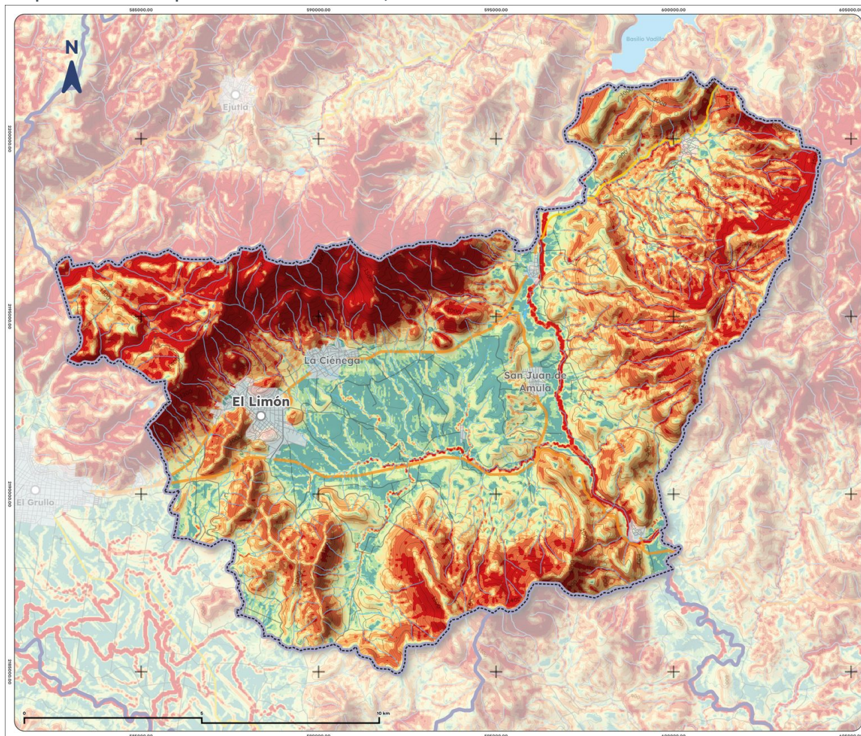
Mapa 16. Erosión potencial de El Limón, 2025
