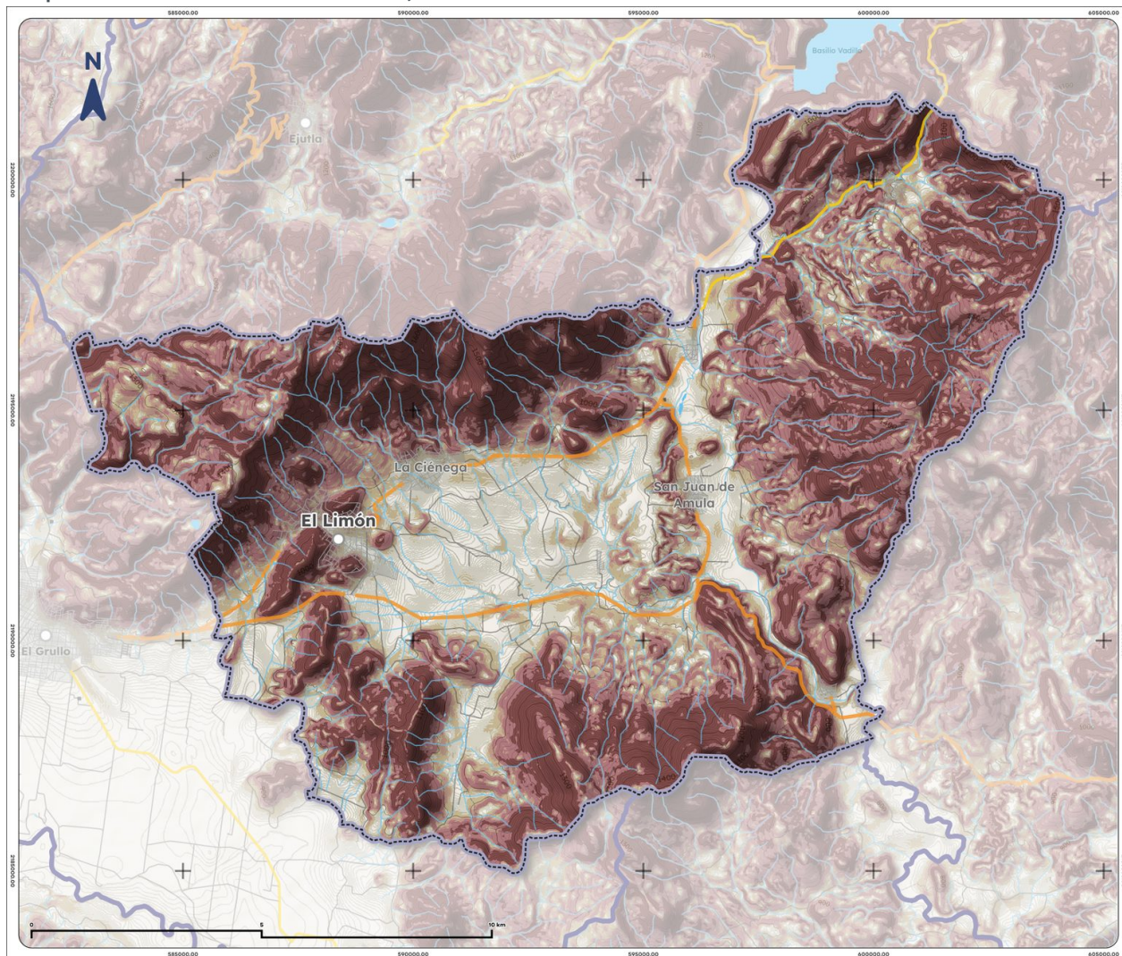
Mapa 5. Pendientes de El Limón, 2025
