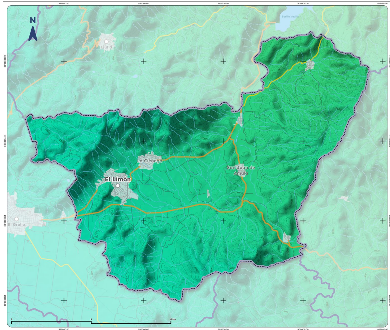
Mapa 9. Precipitación histórica acumulada de El Limón, 1995-2025
