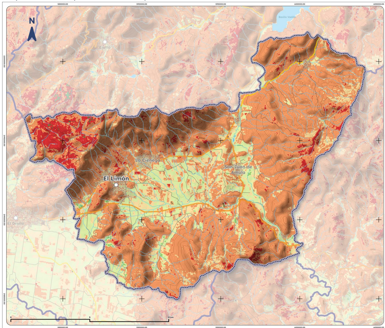
Mapa 15. Índice promedio de sequía de El Limón, 2025
