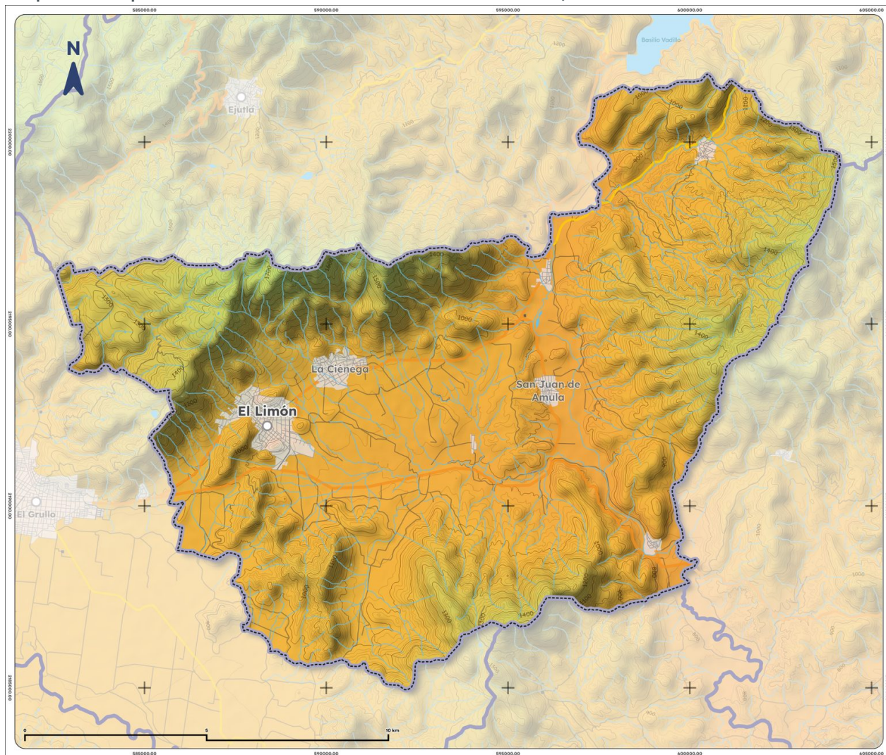
Mapa 8. Temperatura media anual histórica de El Limón, 1995-2025
