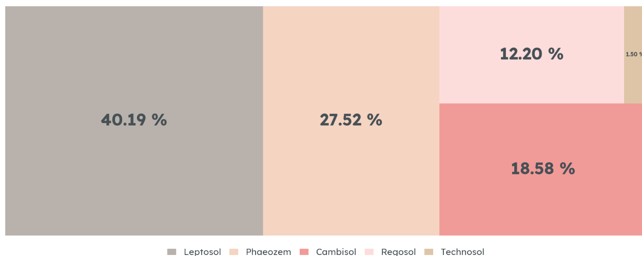
Edafología de El Limón, 2025
