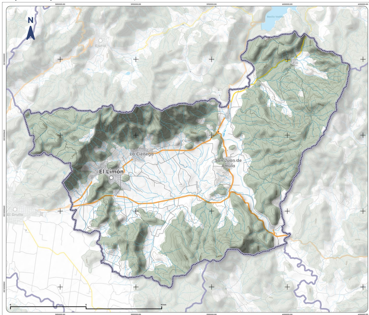
Mapa 2. Mapa base de El Limón, 2025
