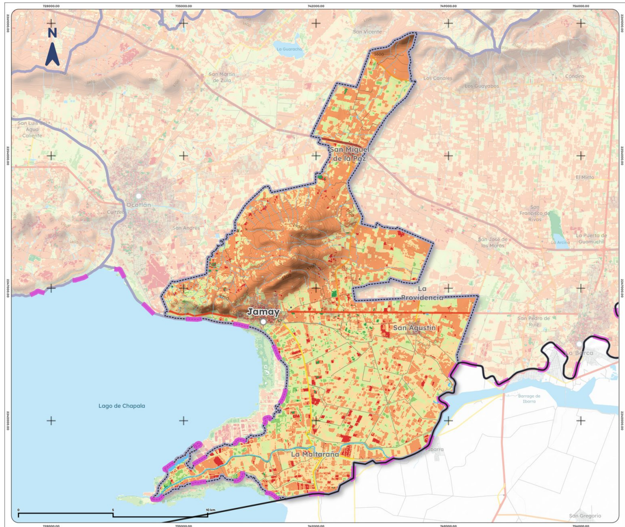
Mapa 15. Índice promedio de sequía de Jamay, 2025
