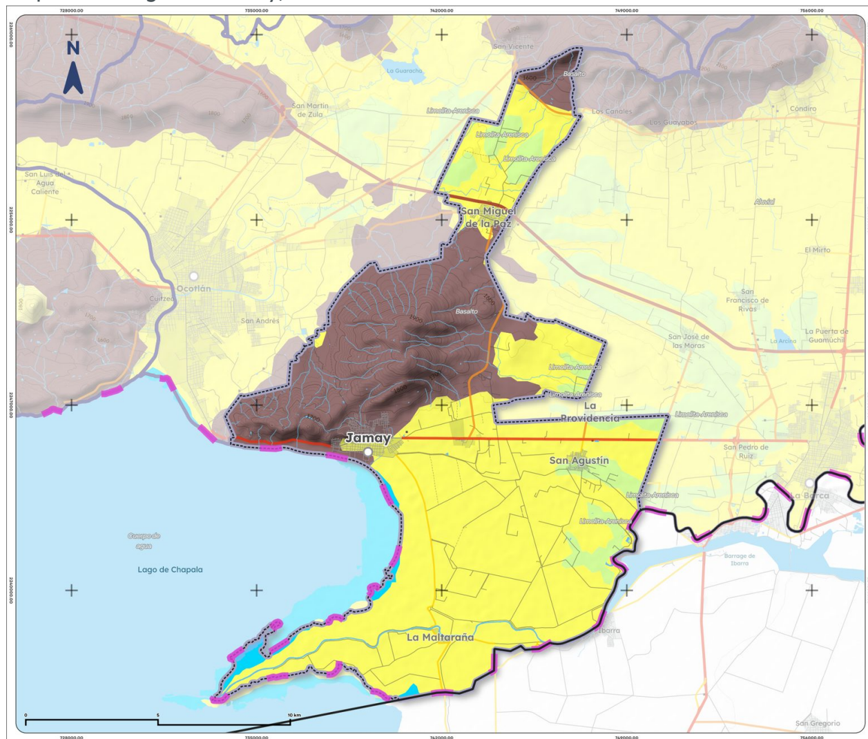
Mapa 3. Geología de Jamay, 1988
