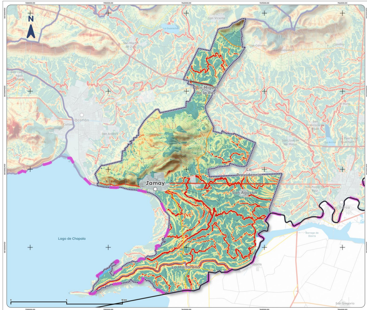
Mapa 17. Erosión efectiva de Jamay, 2025
