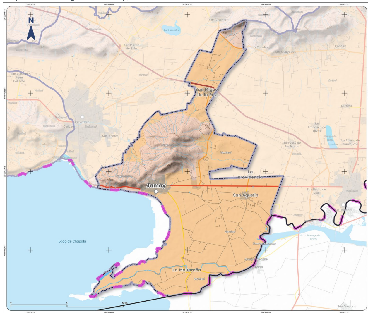
Mapa 4. Edafología de Jamay, 2025
