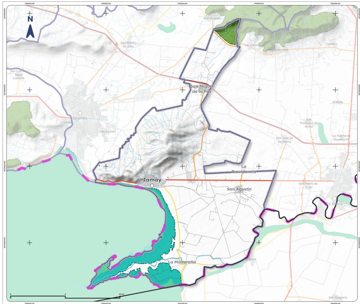
Mapa 14. Áreas naturales protegidas y humedales de Jamay, 2025
