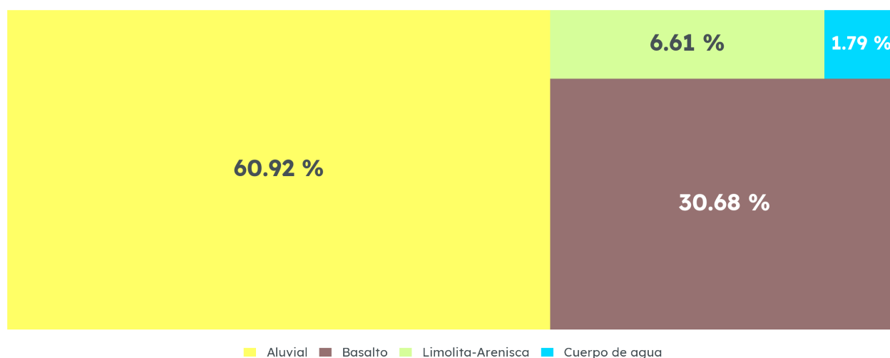
Geología de Jamay, 1988
