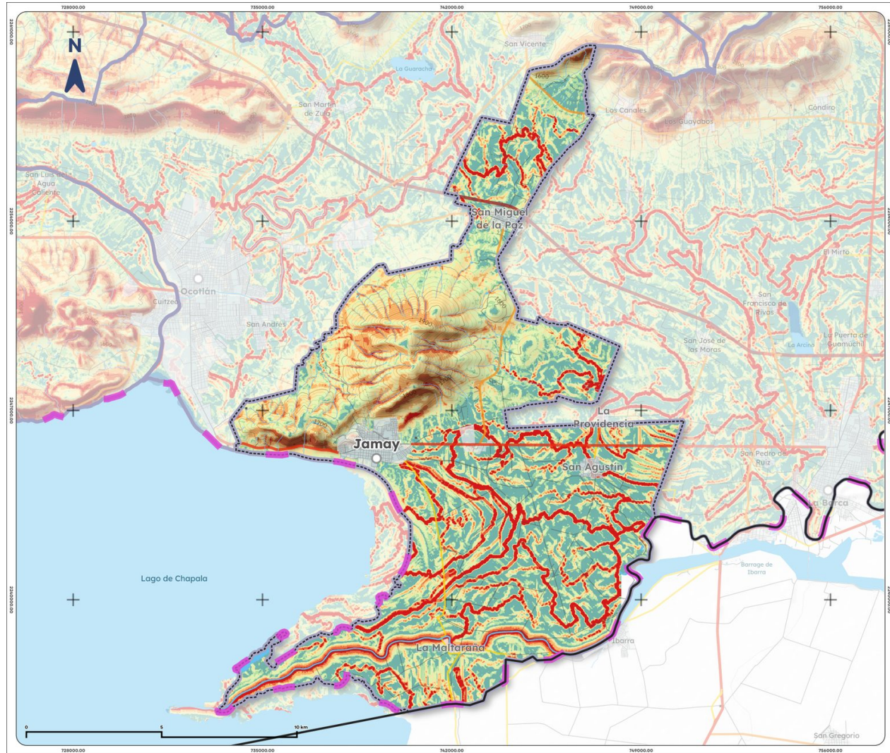
Mapa 16. Erosión potencial de Jamay, 2025
