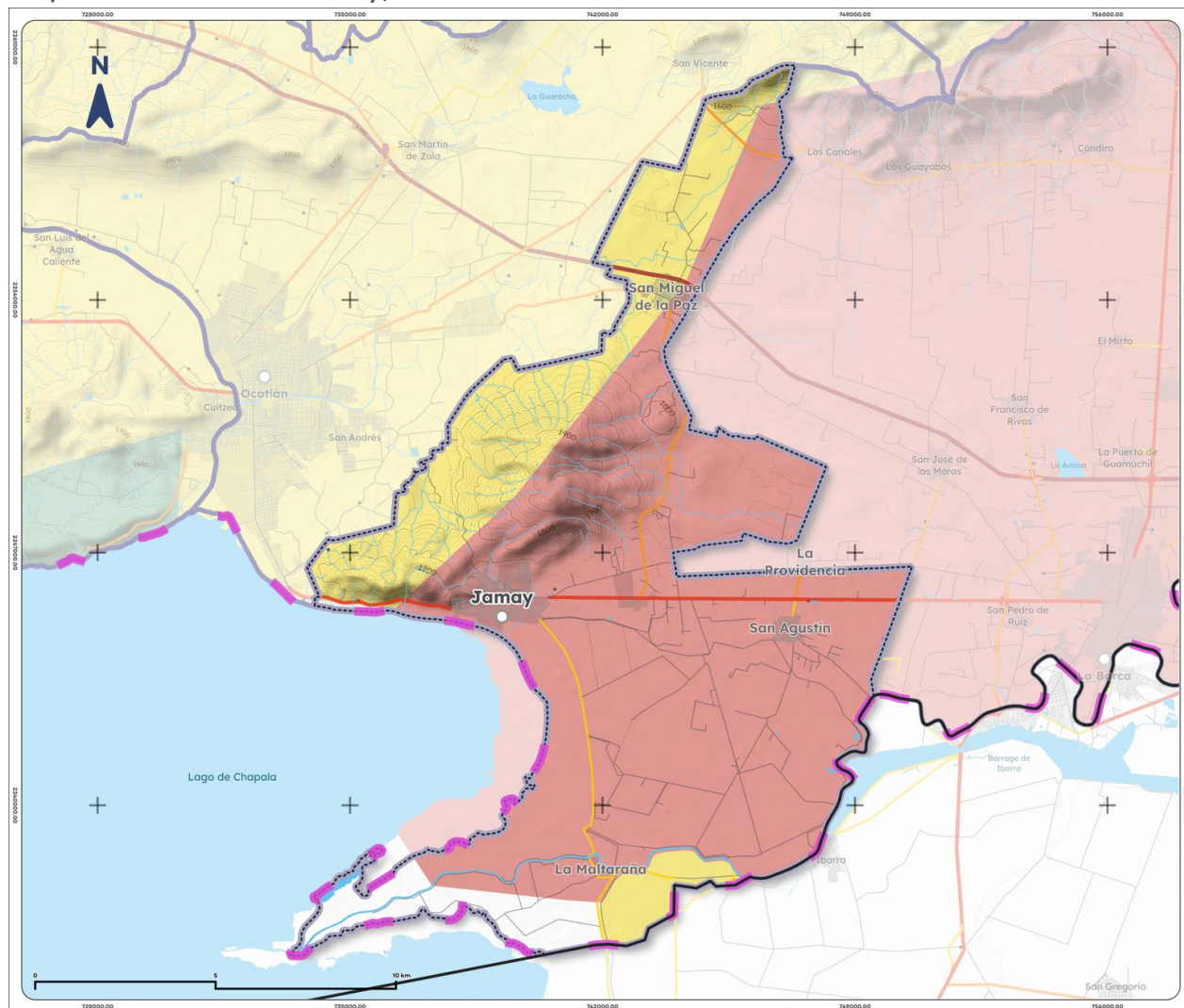
Mapa 7. Acuíferos de Jamay, 2023
