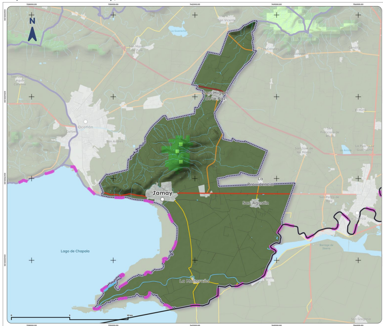
Mapa 10. Clima de Jamay, 1995-2025
