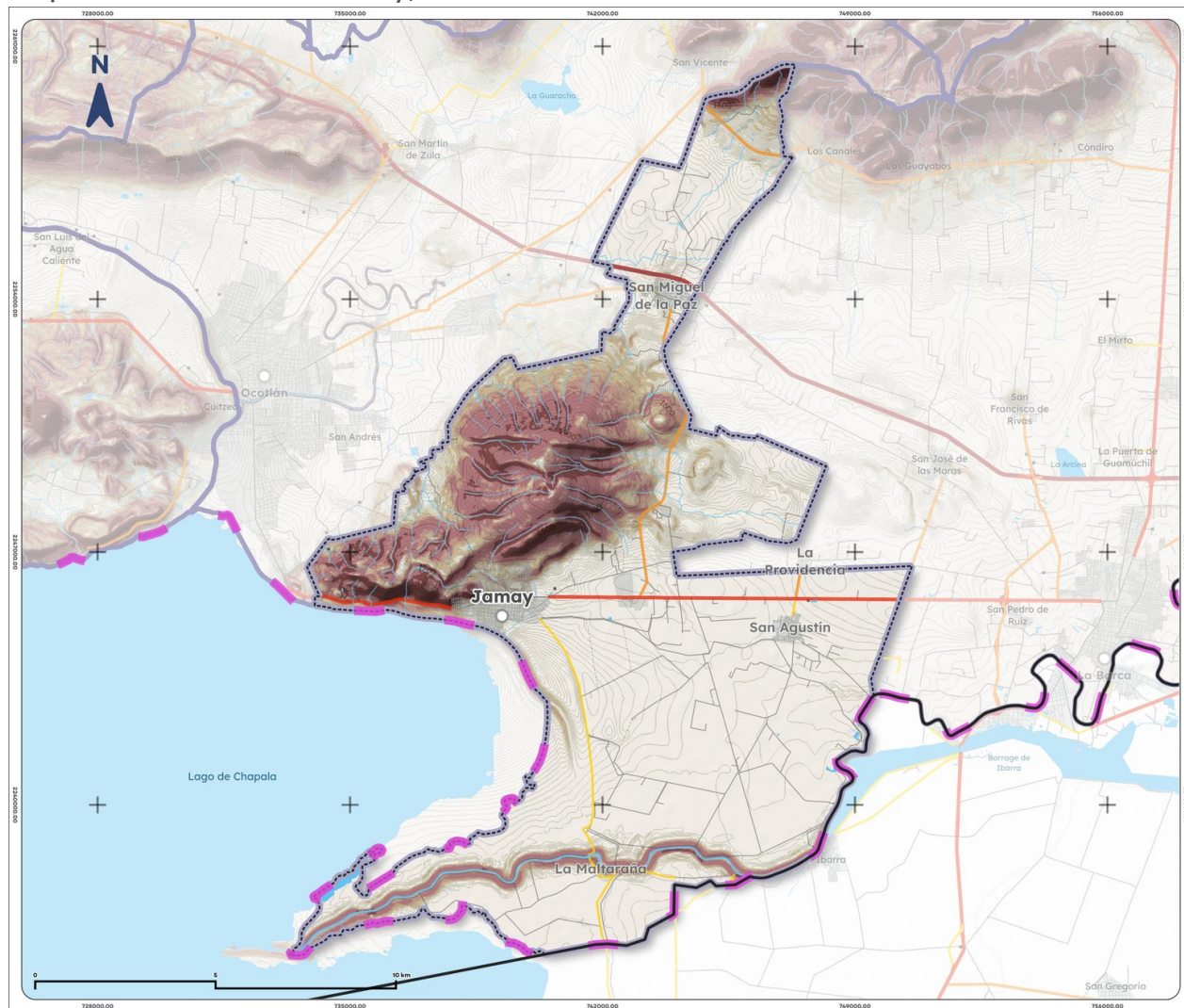
Mapa 5. Pendientes de Jamay, 2025
