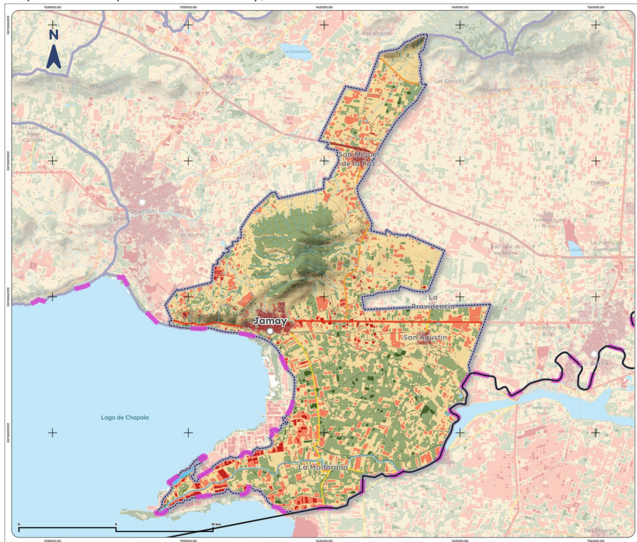
Mapa 12. NDVI promedio de Jamay, 2025
