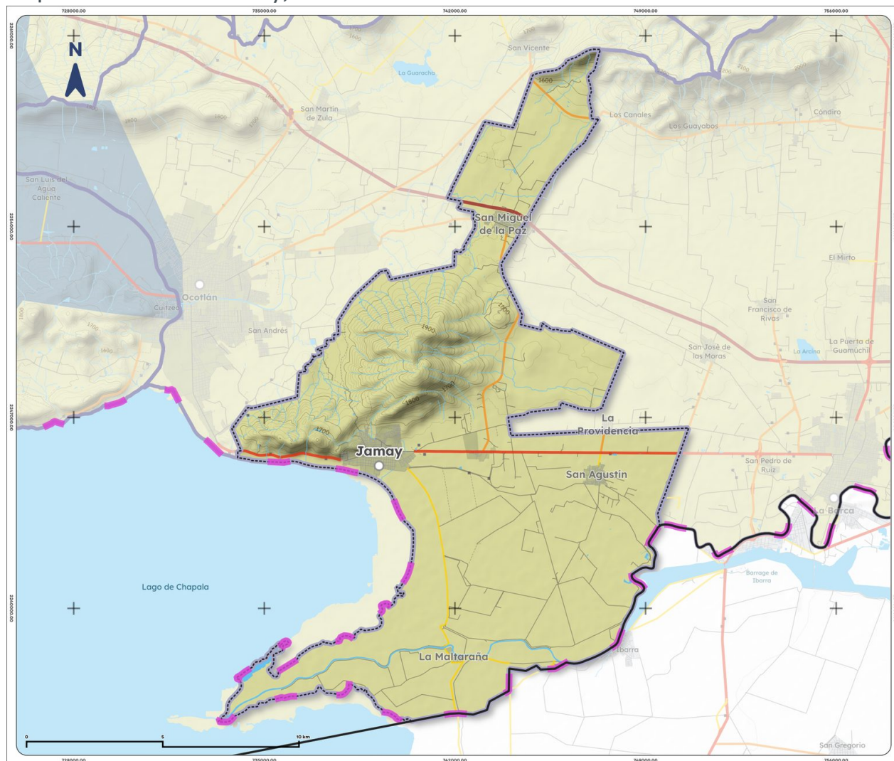
Mapa 6. Cuencas de Jamay, 2023
