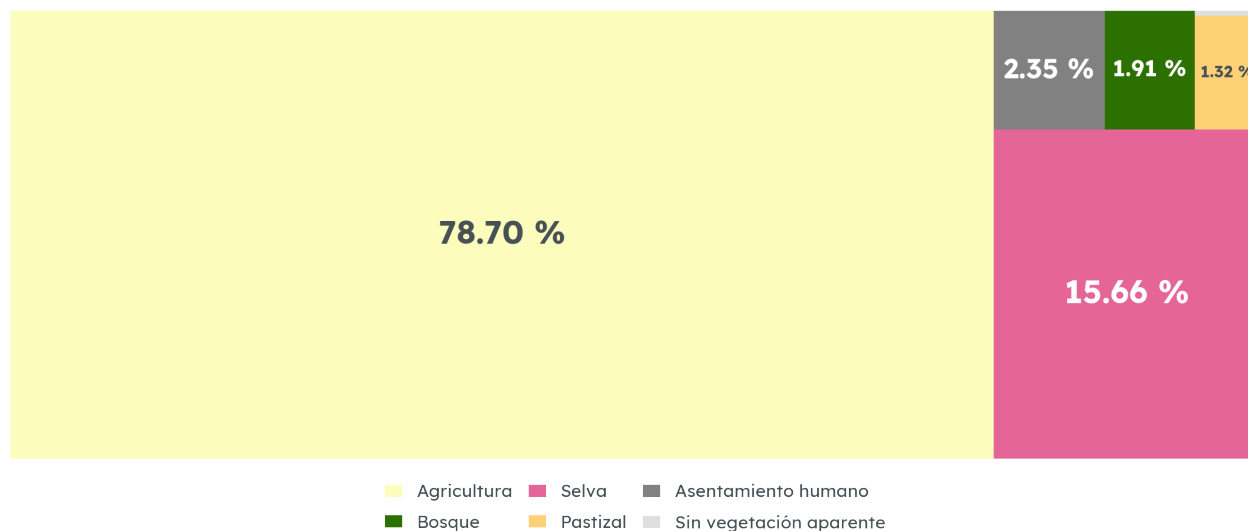
Uso de suelo y vegetación de Jamay, 2018
