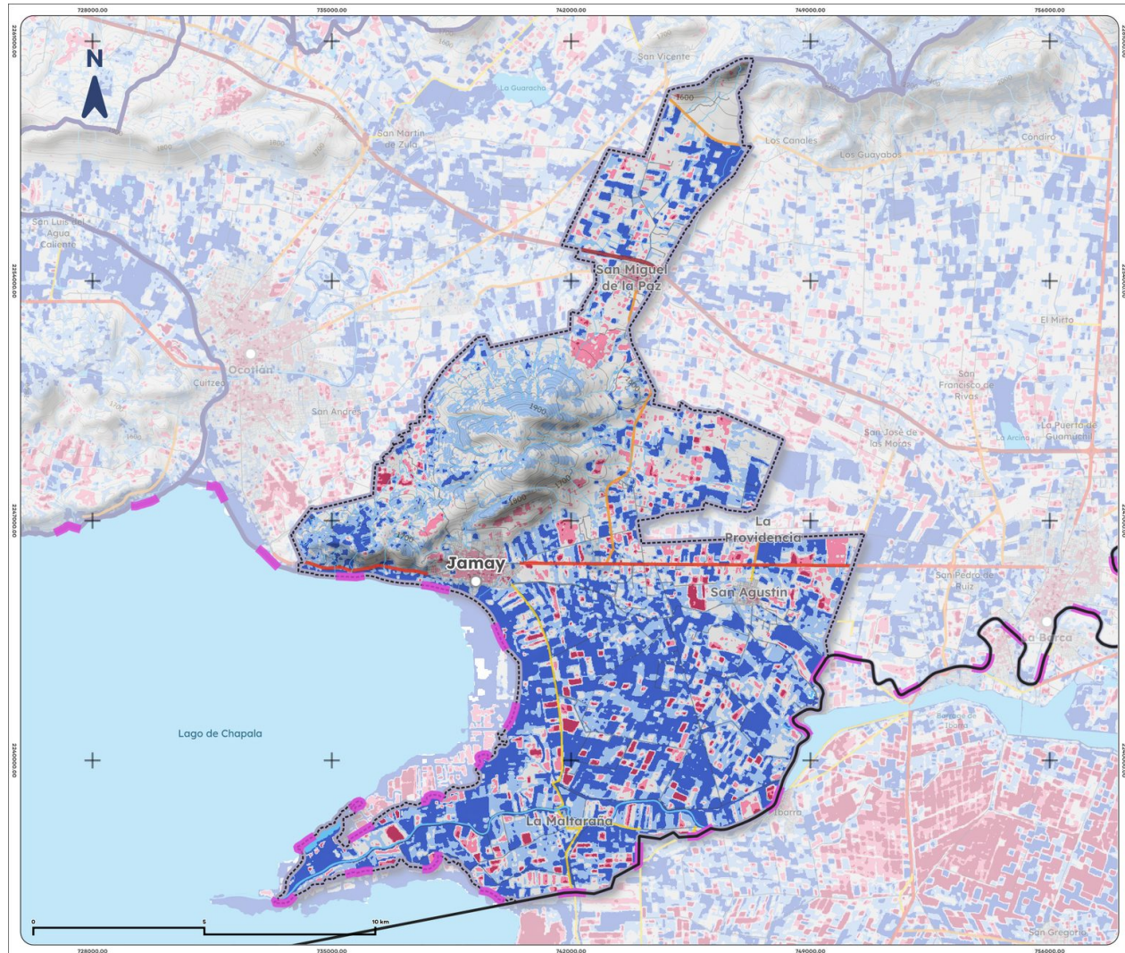
Mapa 13. NDWI promedio de Jamay, 2025
