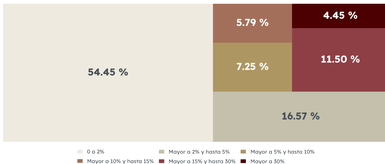
Topografía y pendientes de Jamay, 2025
