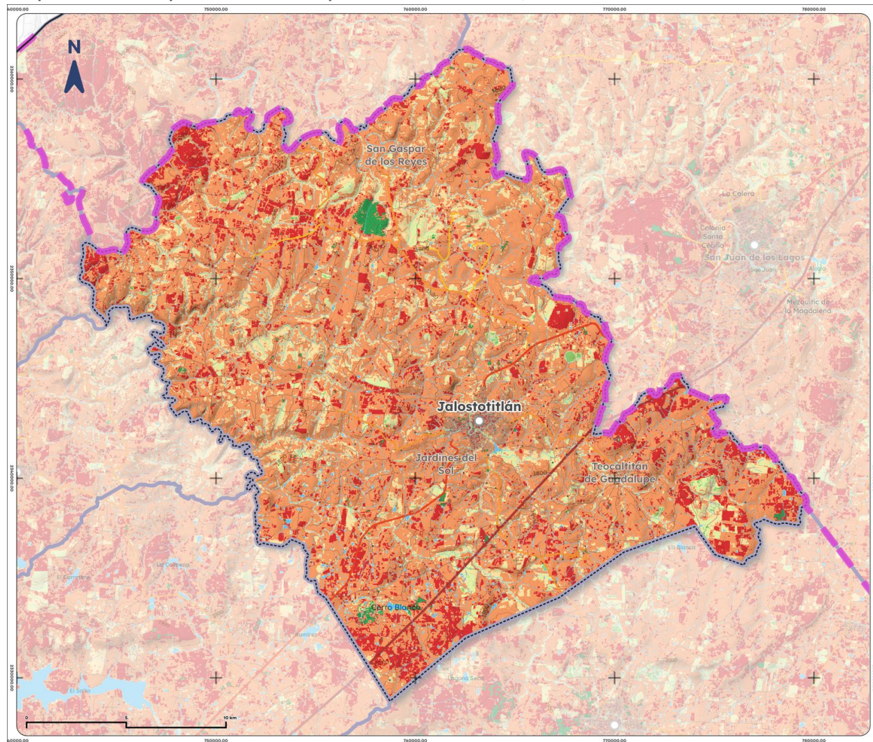
Mapa 15. Índice promedio de sequía de Jalostotitlán, 2025
