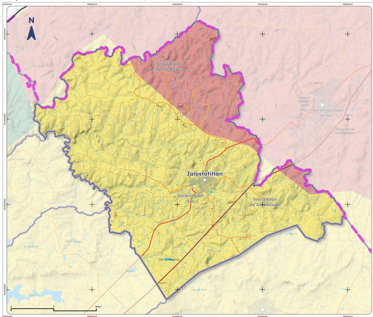
Mapa 7. Acuíferos de Jalostotitlán, 2023
