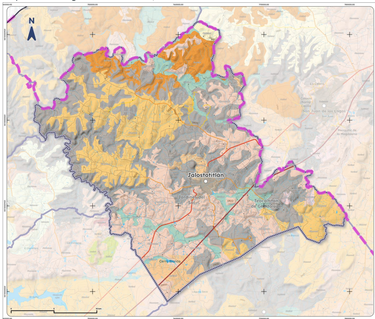
Mapa 4. Edafología de Jalostotitlán, 2025
