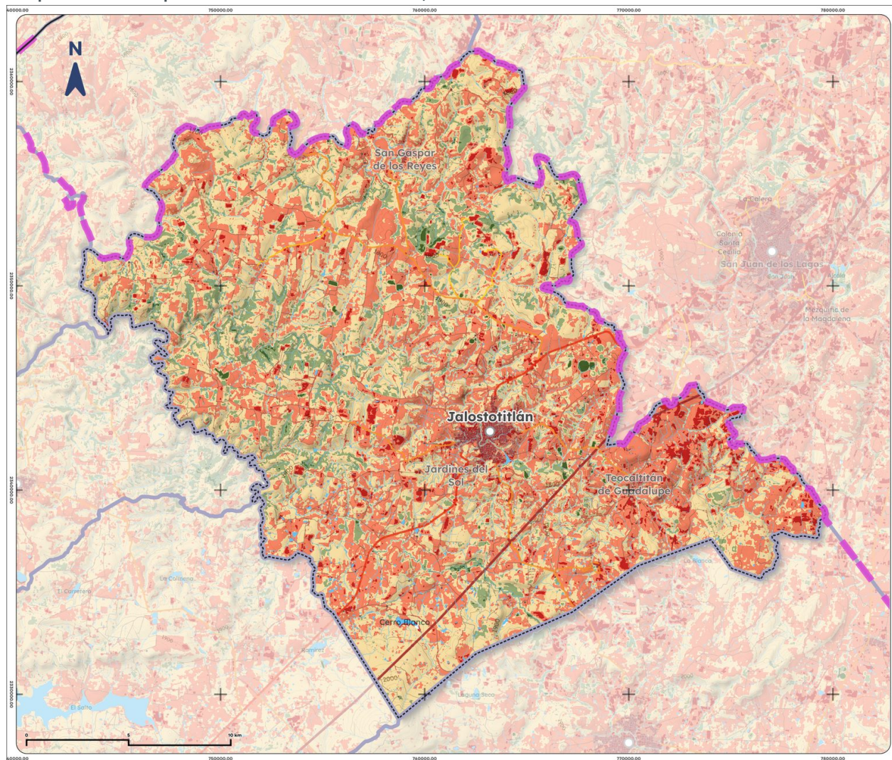
Mapa 12. NDVI promedio de Jalostotitlán, 2025
