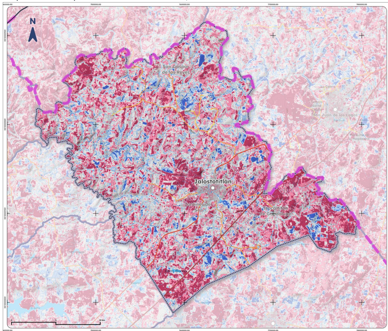
Mapa 13. NDWI promedio de Jalostotitlán, 2025
