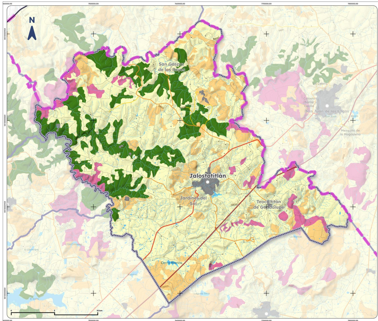
Mapa 11. Uso de suelo y vegetación de Jalostotitlán, 2018
