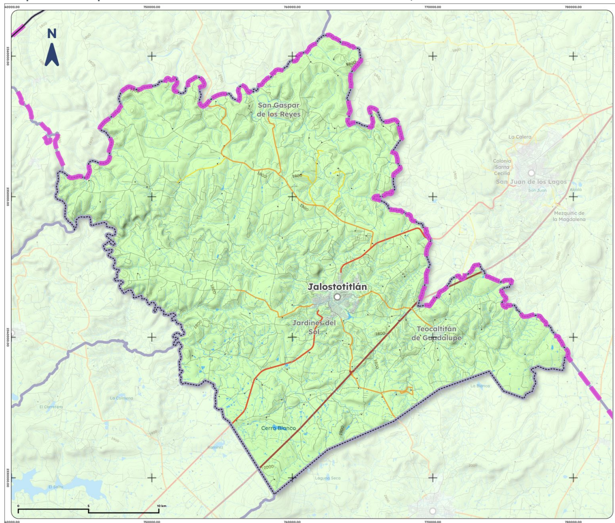
Mapa 9. Precipitación histórica acumulada de Jalostotitlán, 1995-2025
