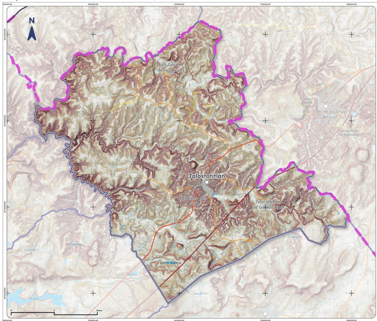
Mapa 5. Pendientes de Jalostotitlán, 2025
