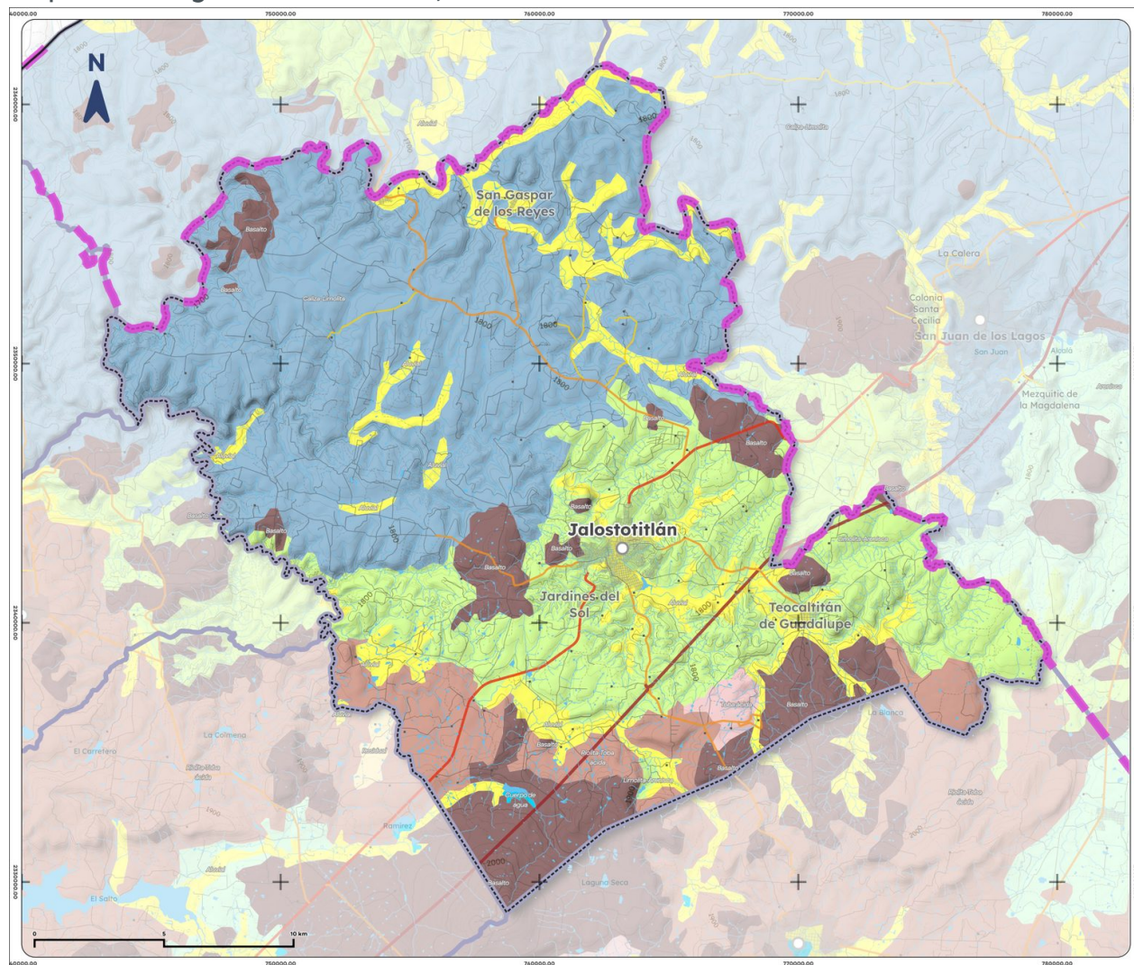
Mapa 3. Geología de Jalostotitlán, 1988
