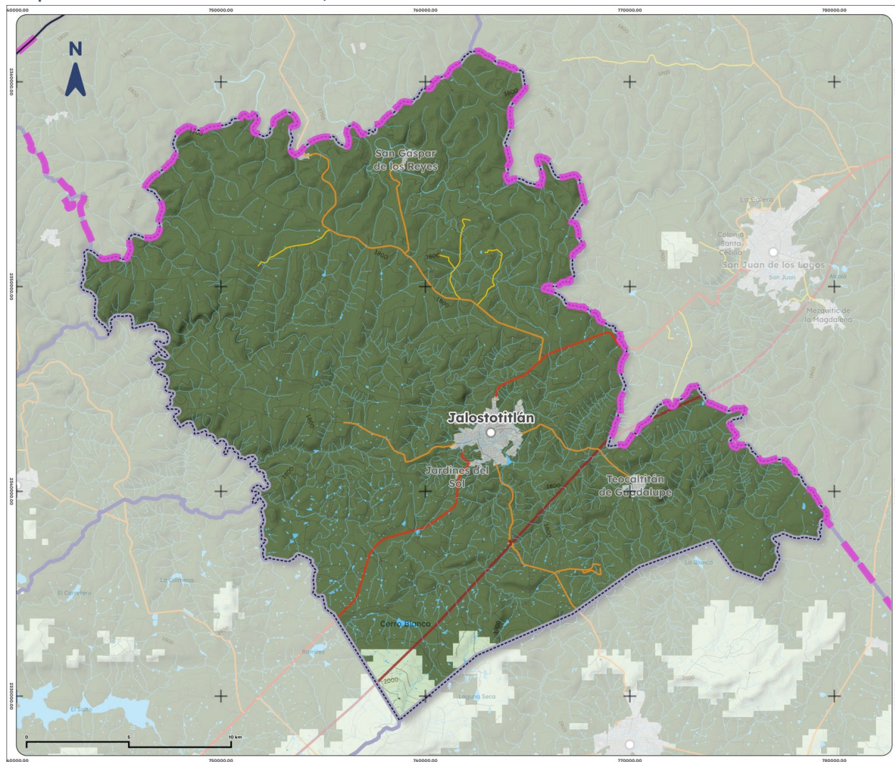
Mapa 10. Clima de Jalostotitlán, 1995-2025
