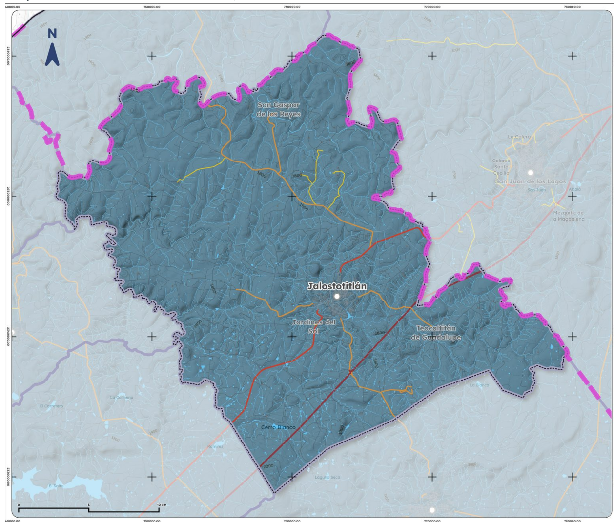
Mapa 6. Cuencas de Jalostotitlán, 2023
