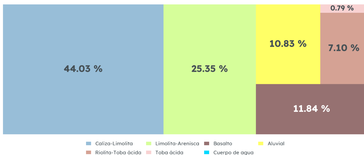
Geología de Jalostotitlán, 1988
