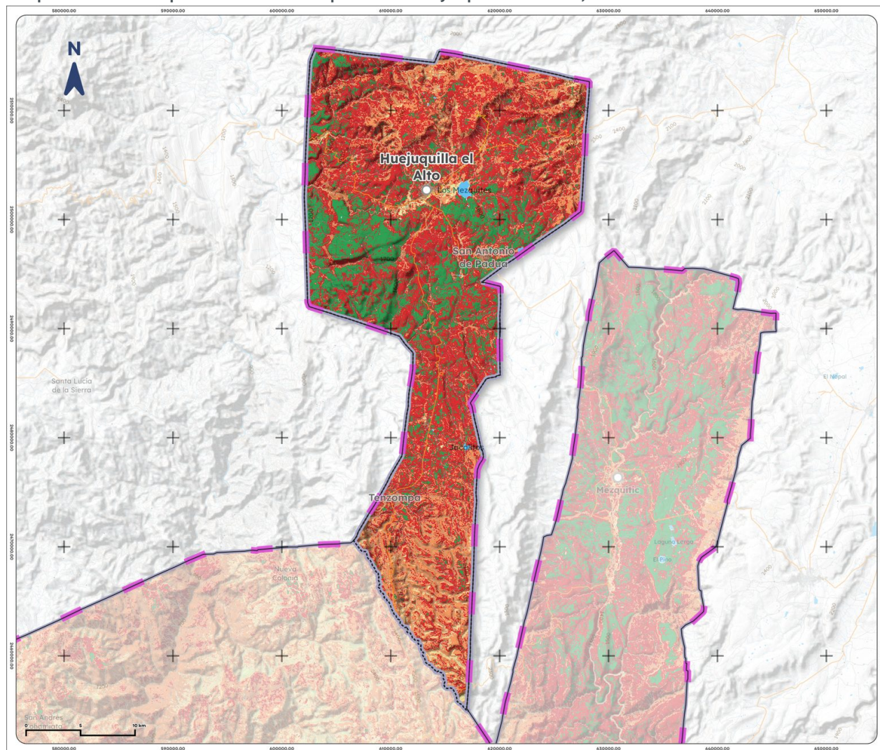
Mapa 15. Índice promedio de sequía de Huejuquilla el Alto, 2025
