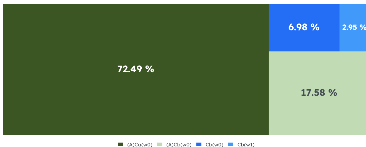
Clima de Huejuquilla el Alto, 1995-2025
