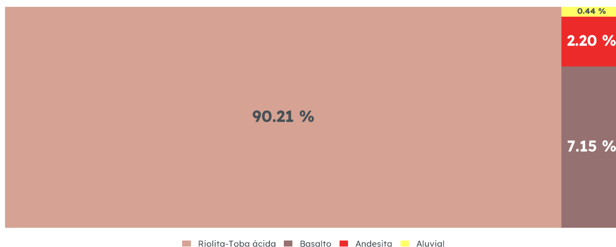
Geología de Huejuquilla el Alto, 1988
