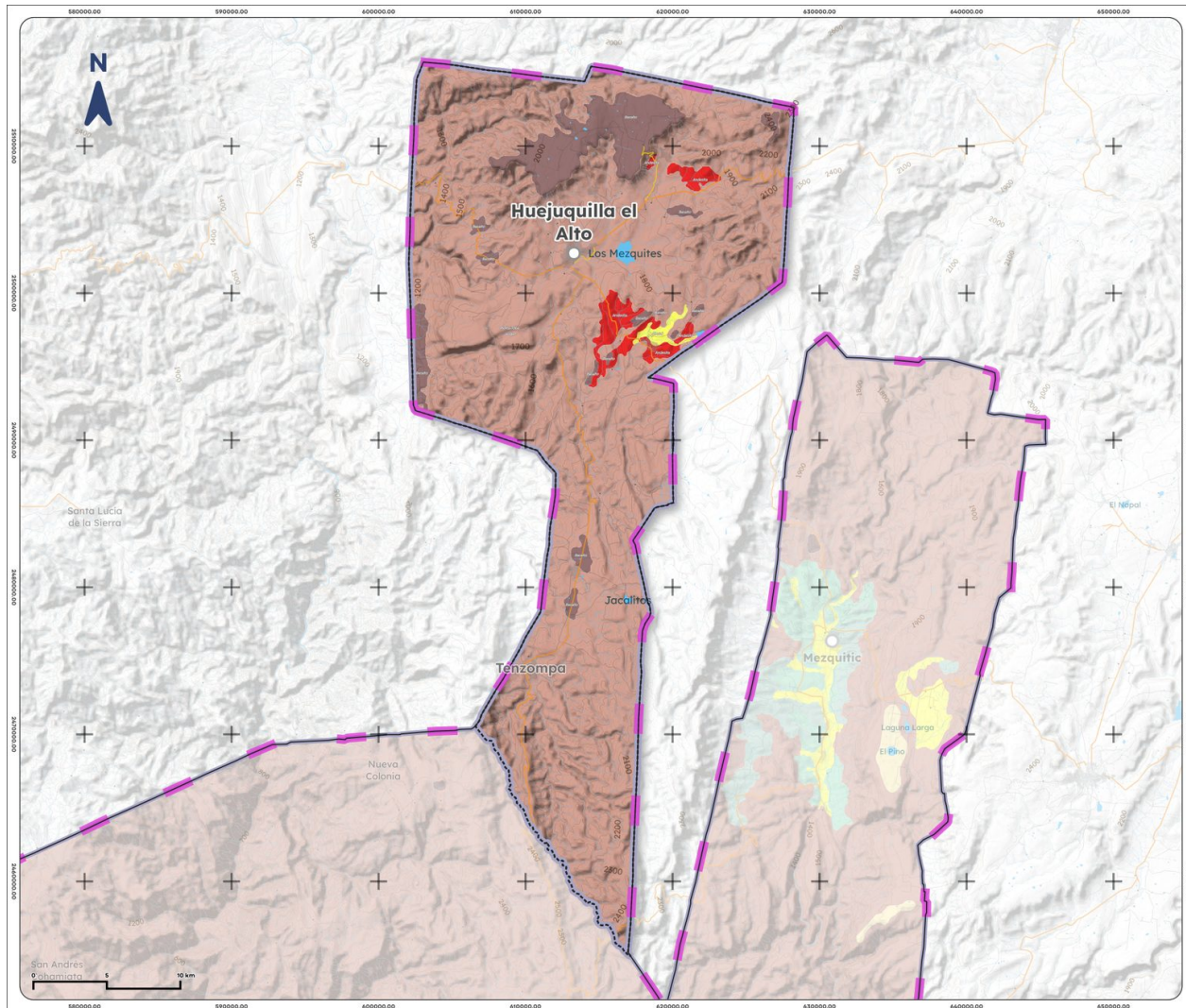
Mapa 3. Geología de Huejuquilla el Alto, 1988
