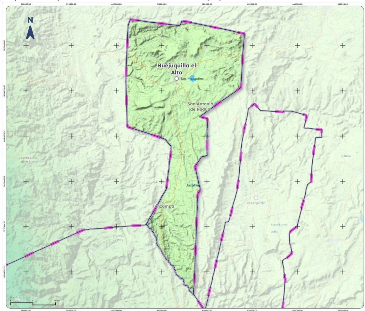
Mapa 9. Precipitación histórica acumulada de Huejuquilla el Alto, 1995-2025
