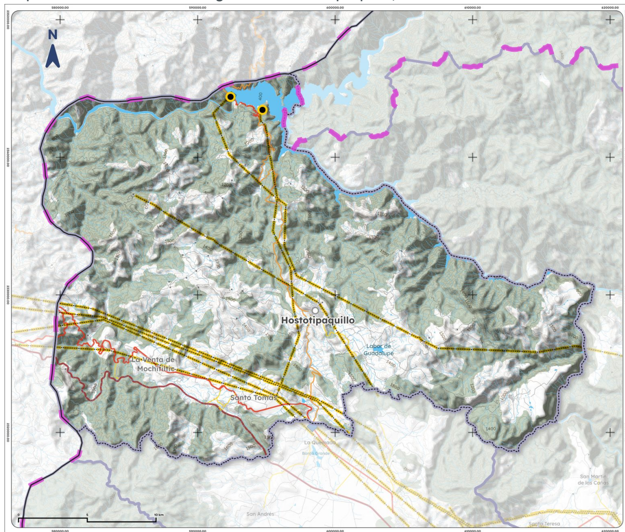
Mapa 22. Infraestructura energética de Hostotipaquillo, 2025
