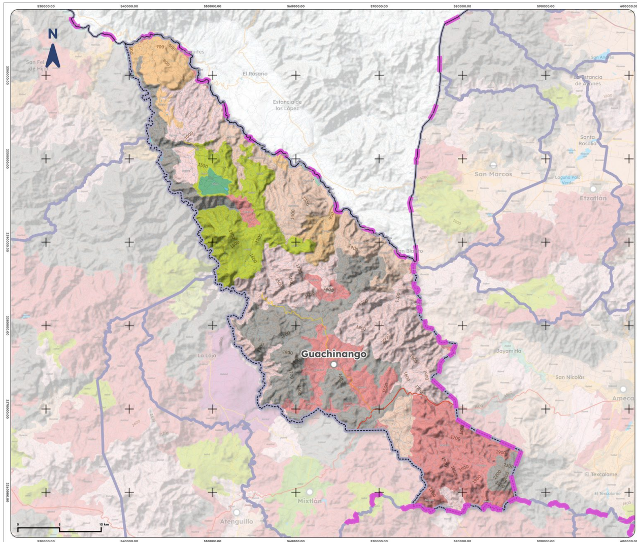
Mapa 4. Edafología de Guachinango, 2025
