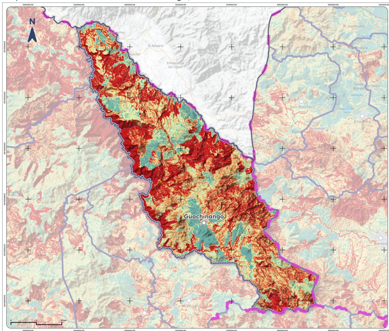
Mapa 17. Erosión efectiva de Guachinango, 2025
