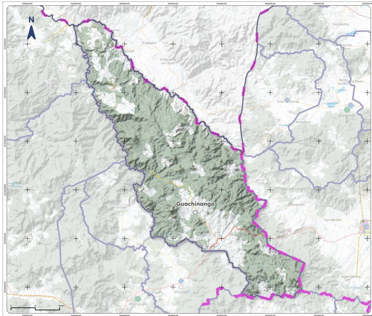
Mapa 22. Infraestructura energética de Guachinango, 2025
