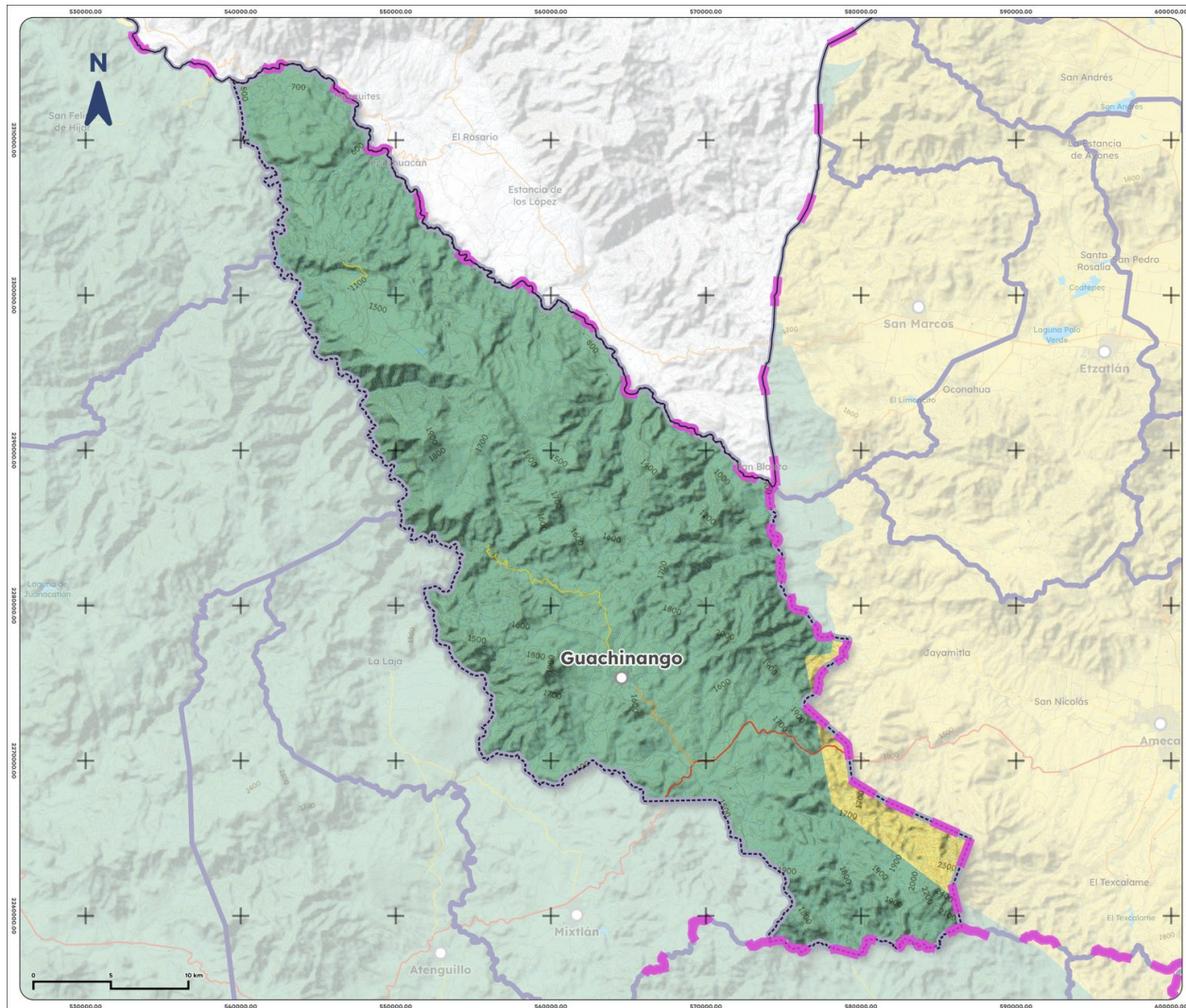
Mapa 7. Acuíferos de Guachinango, 2023
