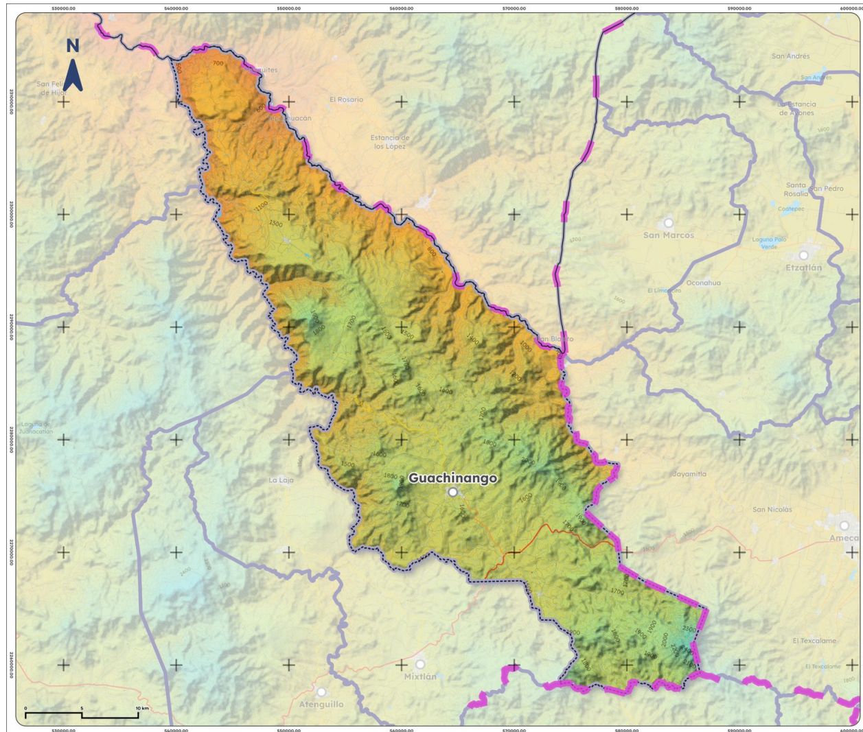
Mapa 8. Temperatura media anual histórica de Guachinango, 1995-2025
