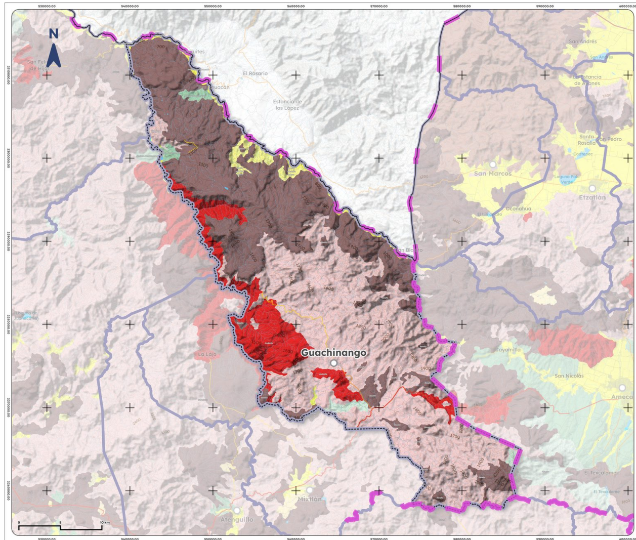
Mapa 3. Geología de Guachinango, 1988
