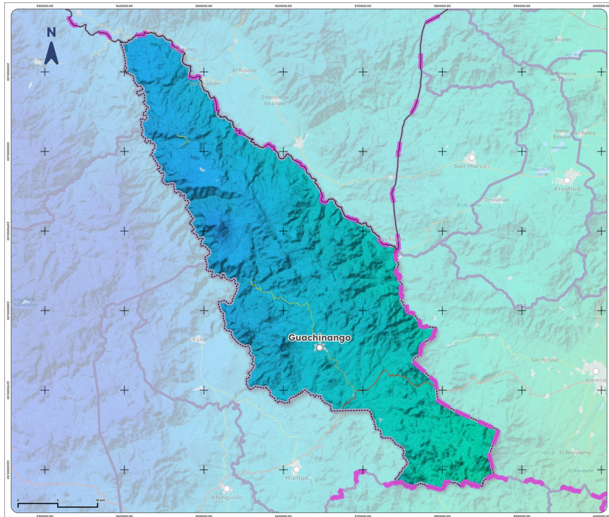
Mapa 9. Precipitación histórica acumulada de Guachinango, 1995-2025
