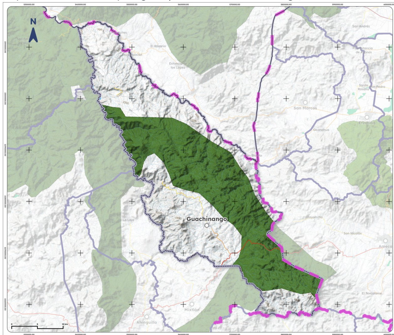
Mapa 14. Áreas naturales protegidas y humedales de Guachinango, 2025
