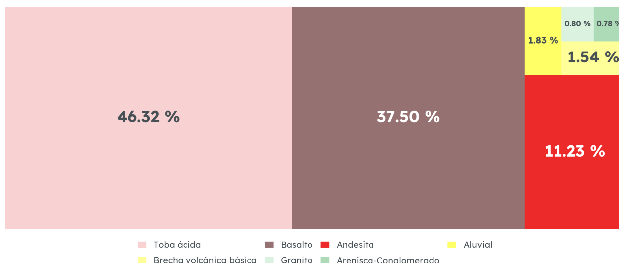
Geología de Guachinango, 1988
