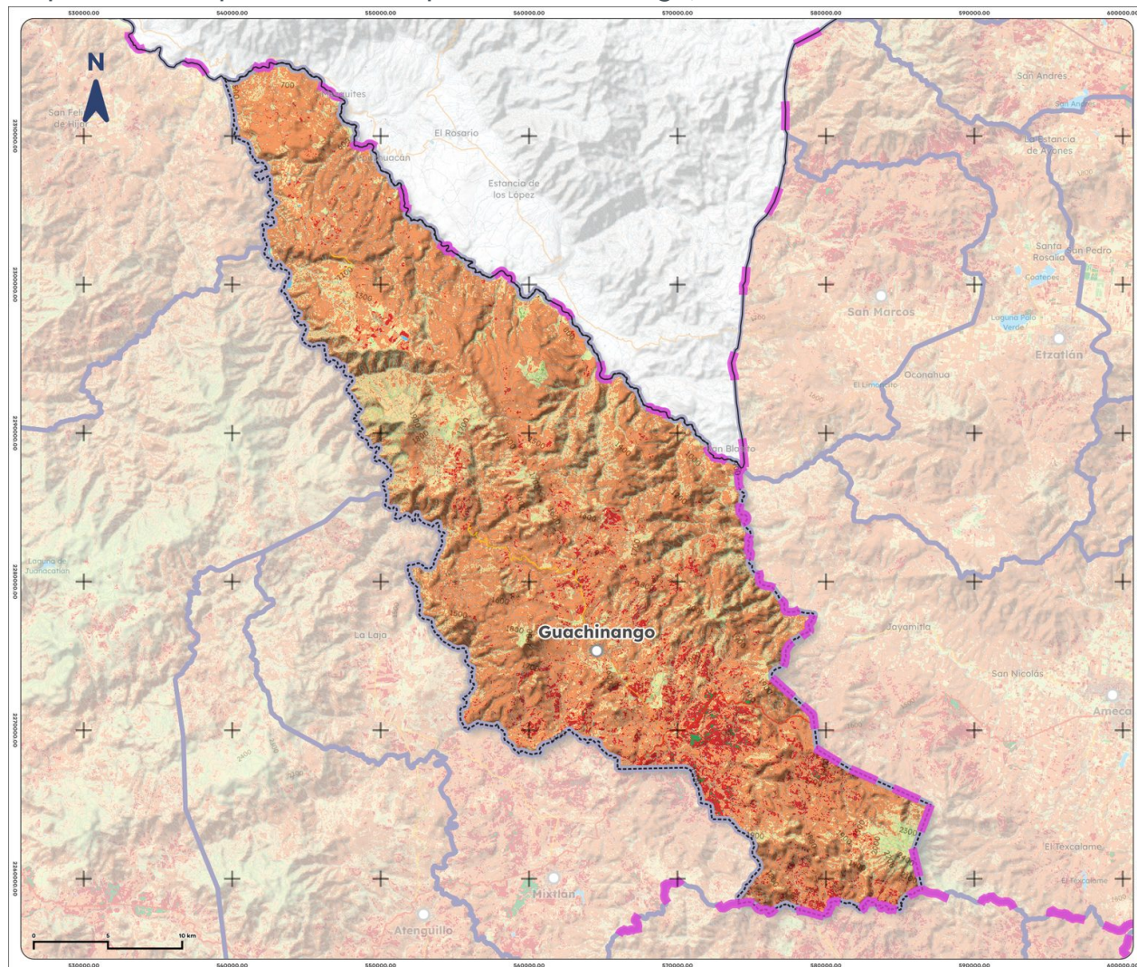
Mapa 15. Índice promedio de sequía de Guachinango, 2025
