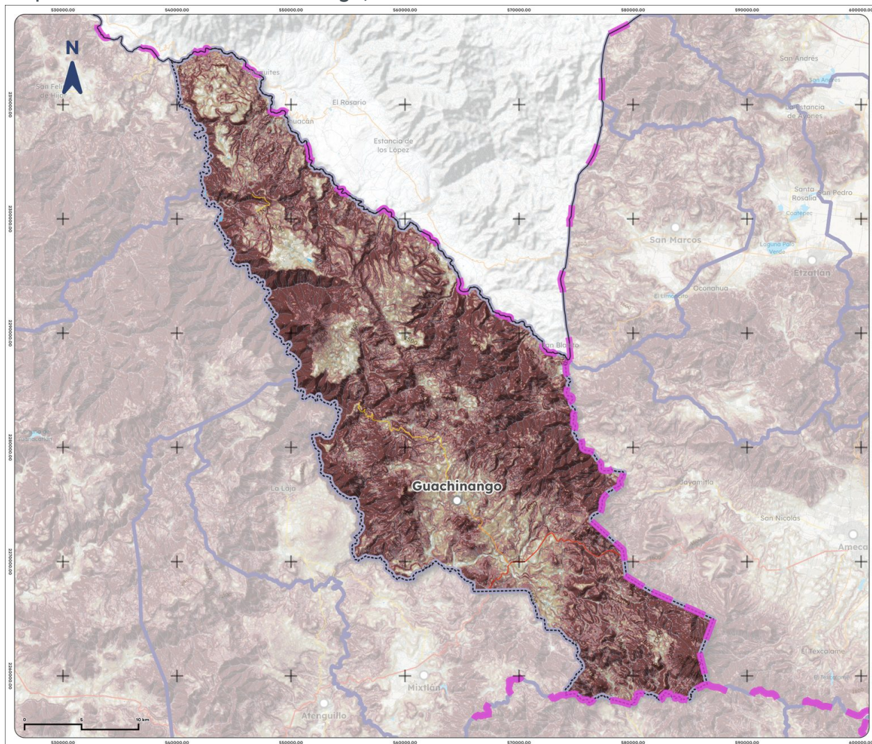
Mapa 5. Pendientes de Guachinango, 2025
