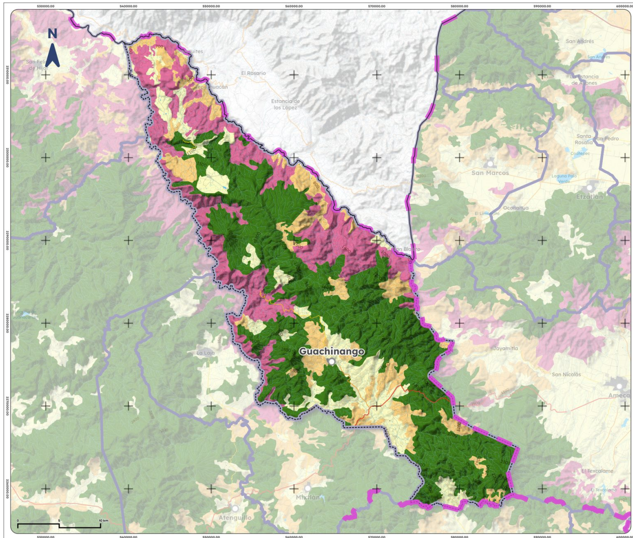
Mapa 11. Uso de suelo y vegetación de Guachinango, 2018
