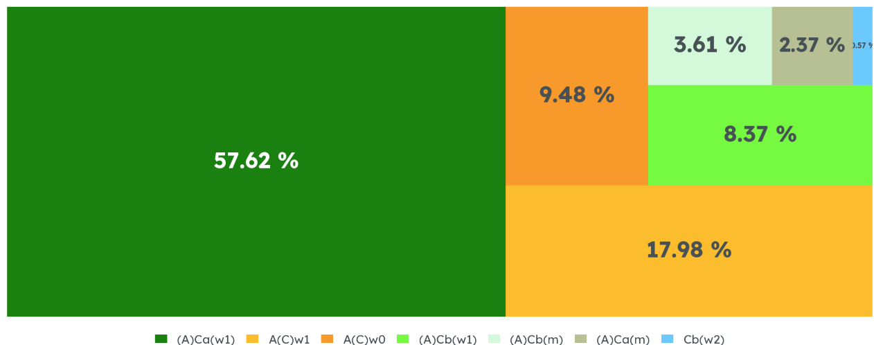
Clima de Guachinango, 1995-2025
