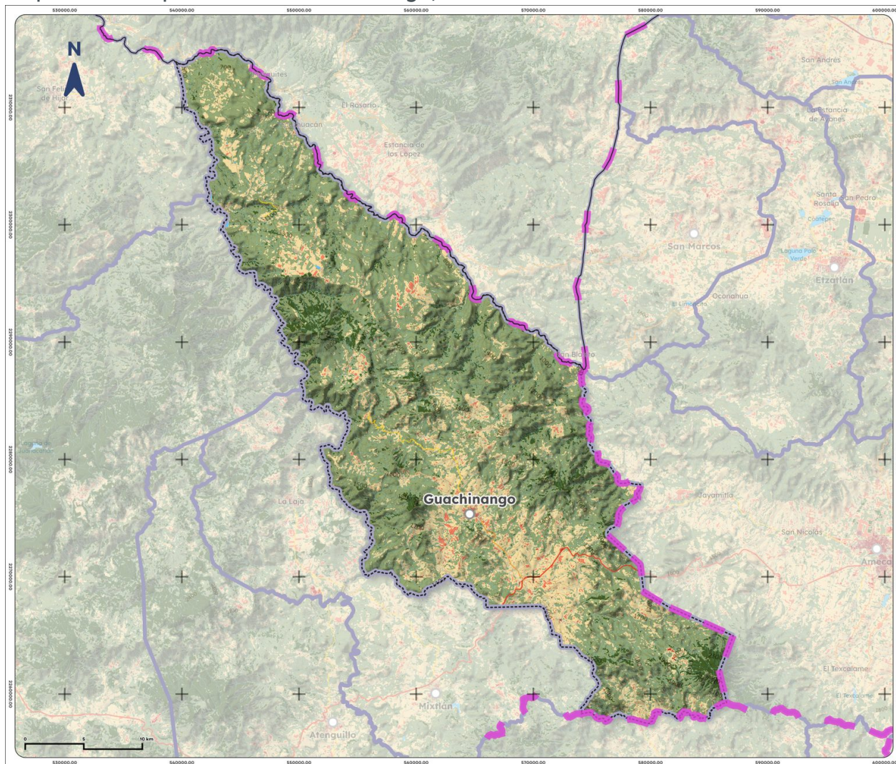
Mapa 12. NDVI promedio de Guachinango, 2025
