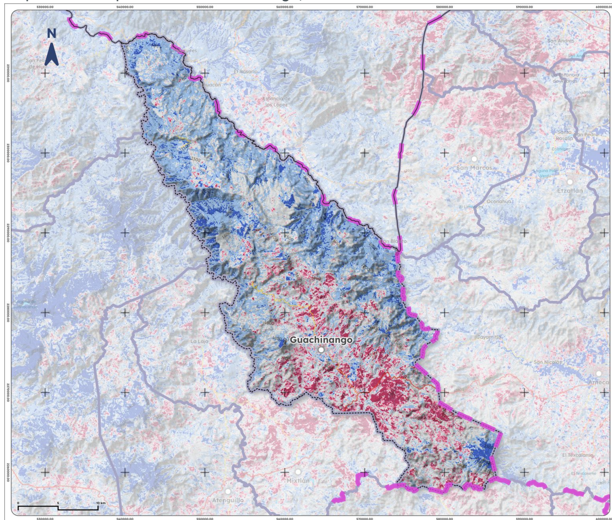
Mapa 13. NDWI promedio de Guachinango, 2025
