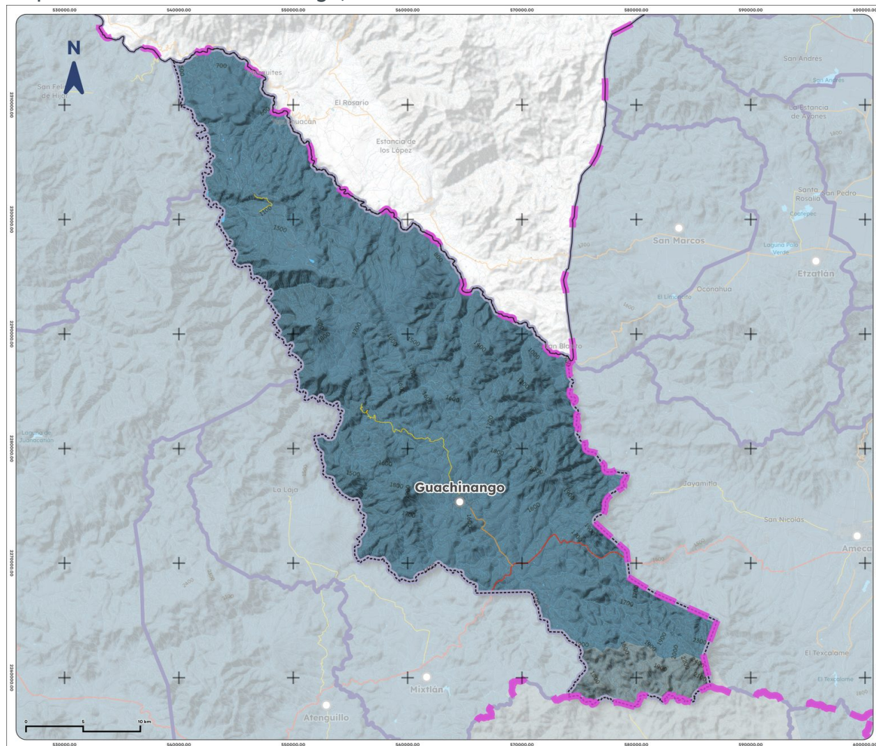
Mapa 6. Cuencas de Guachinango, 2023
