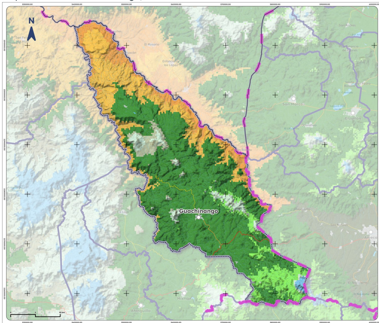
Mapa 10. Clima de Guachinango, 1995-2025
