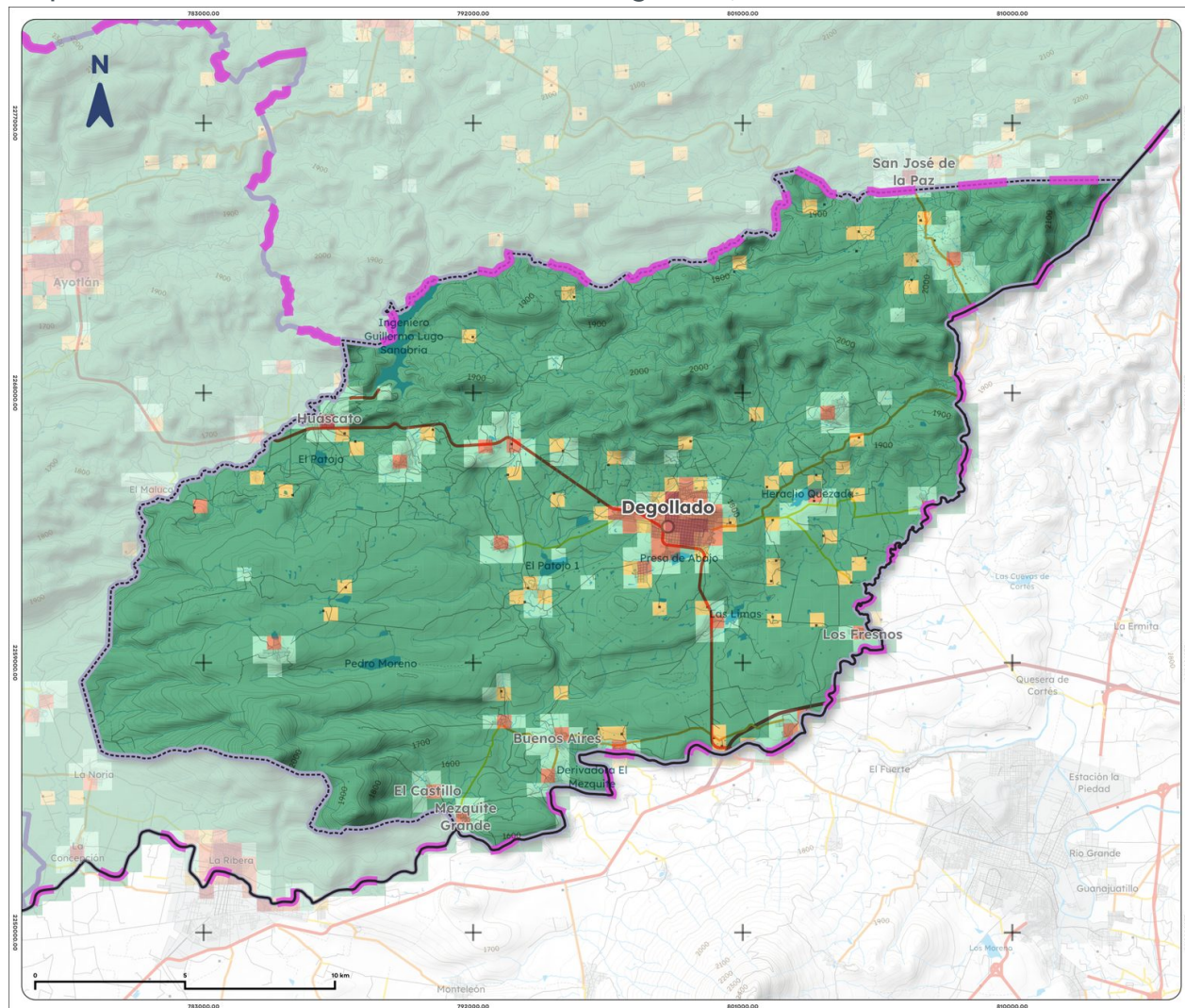
Mapa 18. Índice Territorial Urbano-Rural de Degollado, 2025
