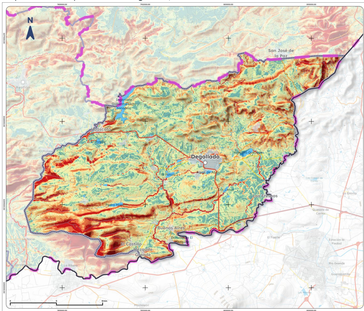
Mapa 16. Erosión potencial de Degollado, 2025
