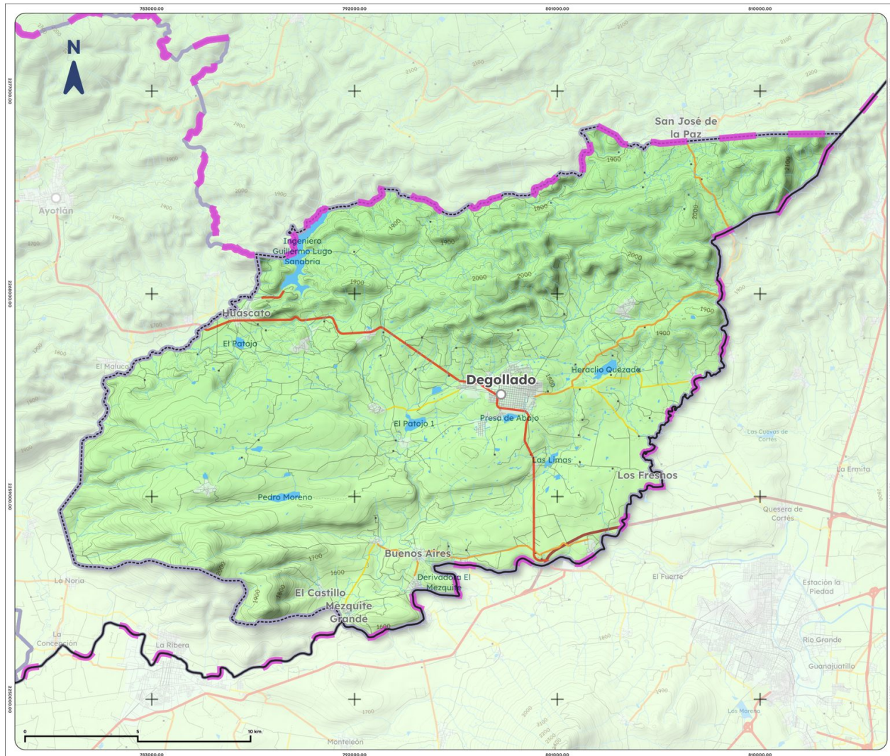
Mapa 9. Precipitación histórica acumulada de Degollado, 1995-2025
