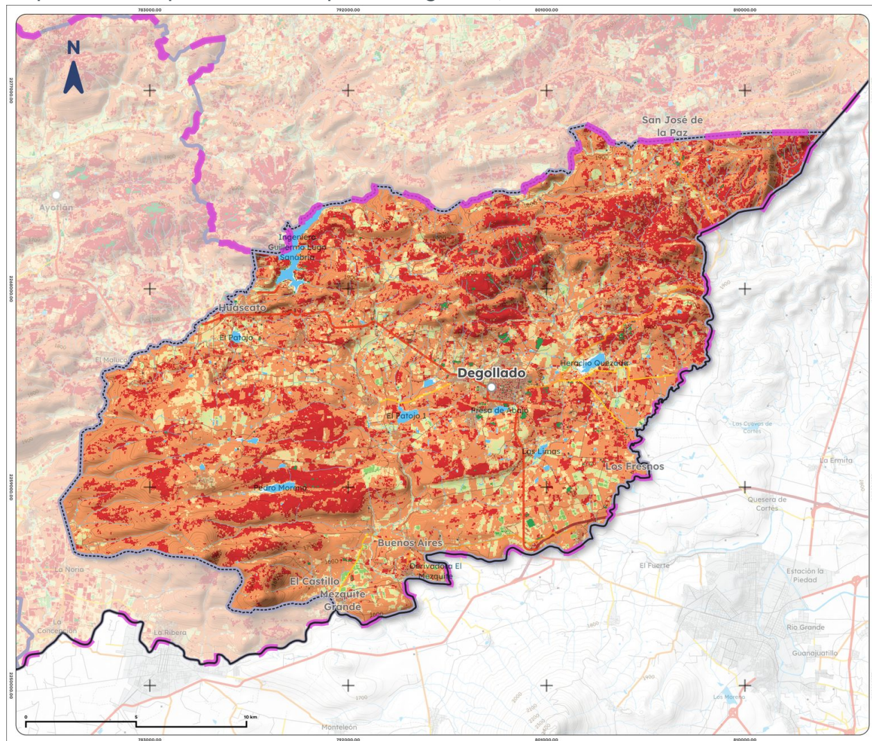
Mapa 15. Índice promedio de sequía de Degollado, 2025
