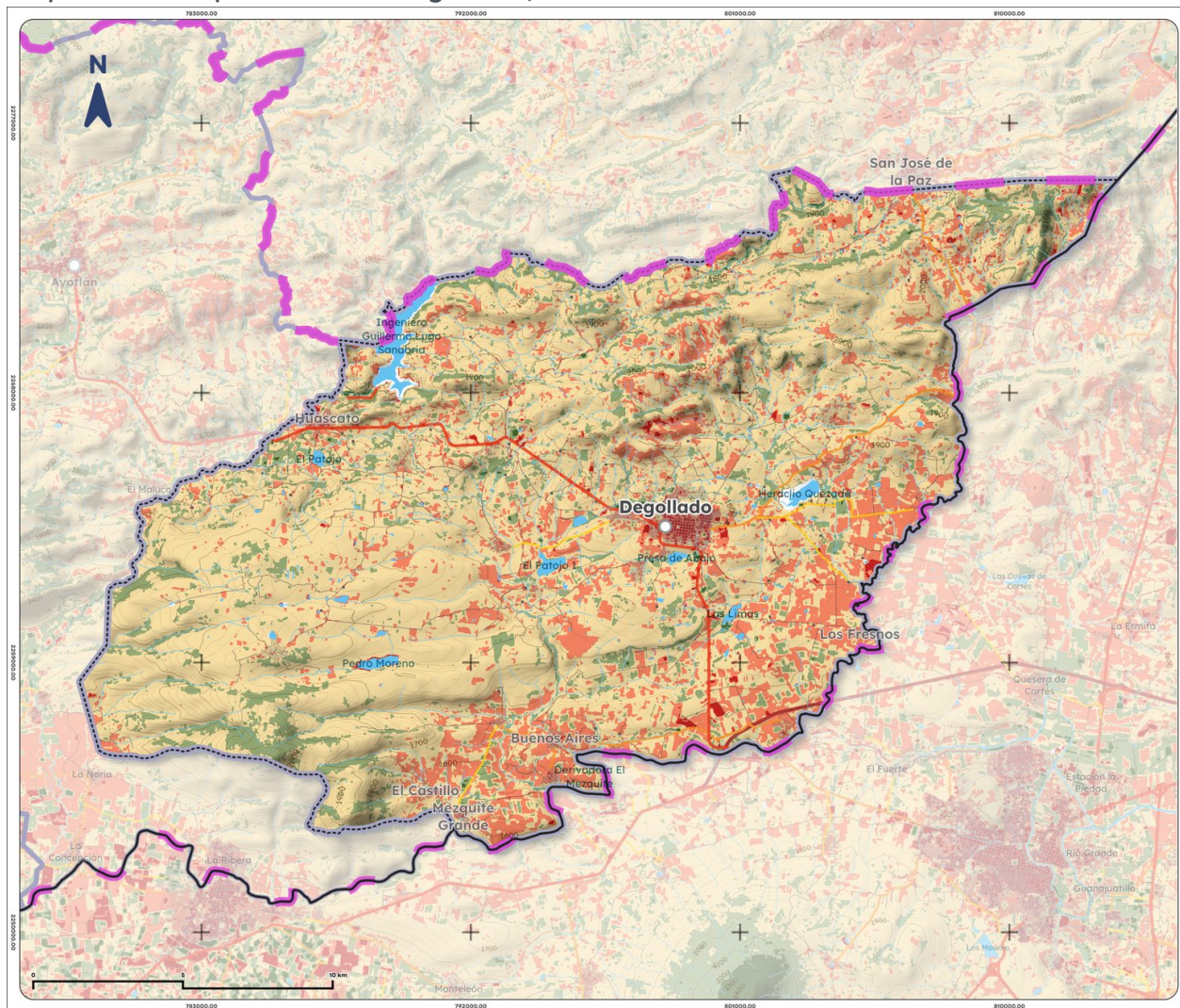
Mapa 12. NDVI promedio de Degollado, 2025
