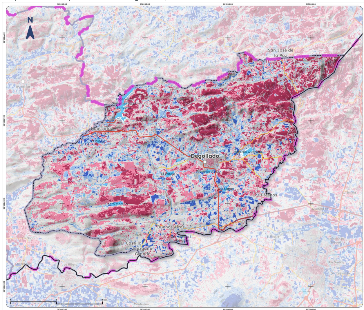
Mapa 13. NDWI promedio de Degollado, 2025
