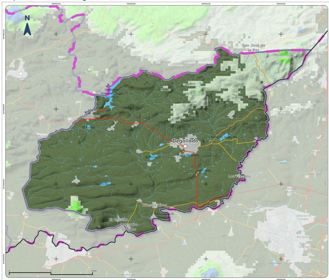
Mapa 10. Clima de Degollado, 1995-2025
