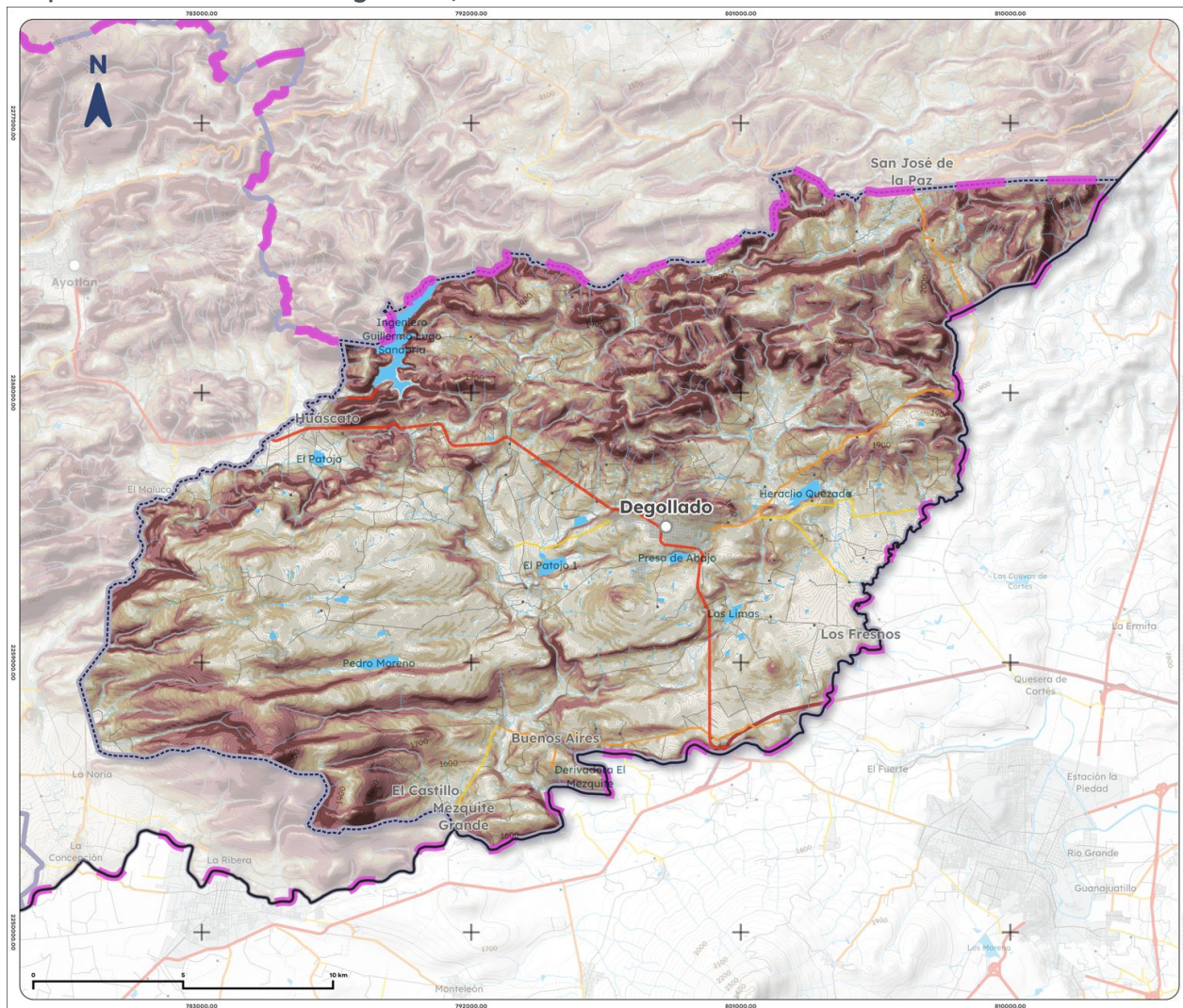
Mapa 5. Pendientes de Degollado, 2025
