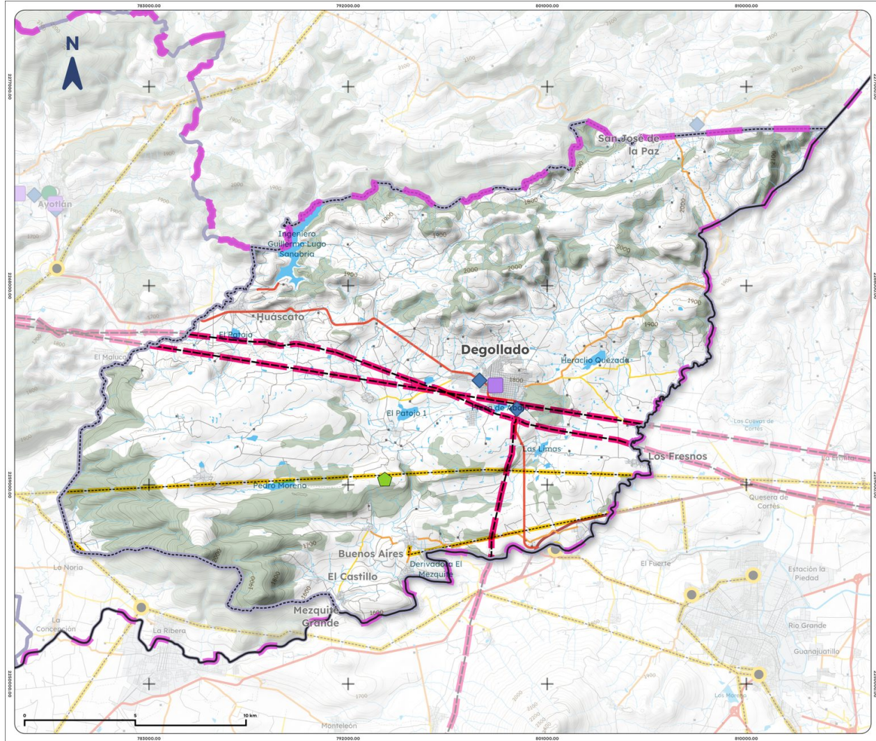
Mapa 22. Infraestructura energética de Degollado, 2025
