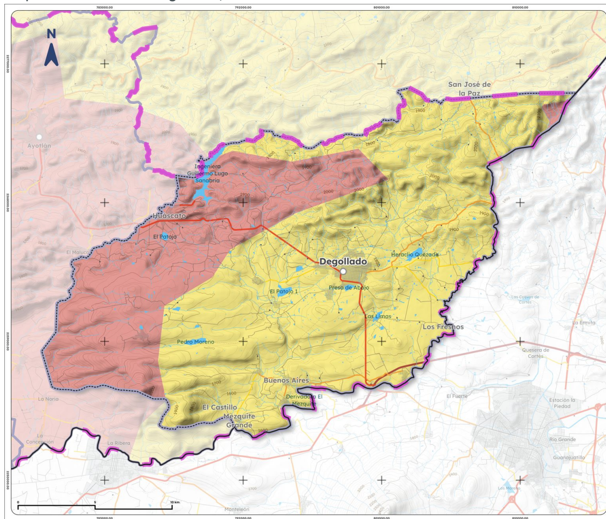
Mapa 7. Acuíferos de Degollado, 2023
