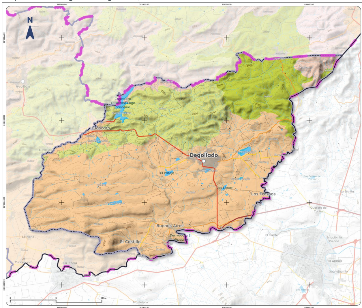
Mapa 4. Edafología de Degollado, 2025
