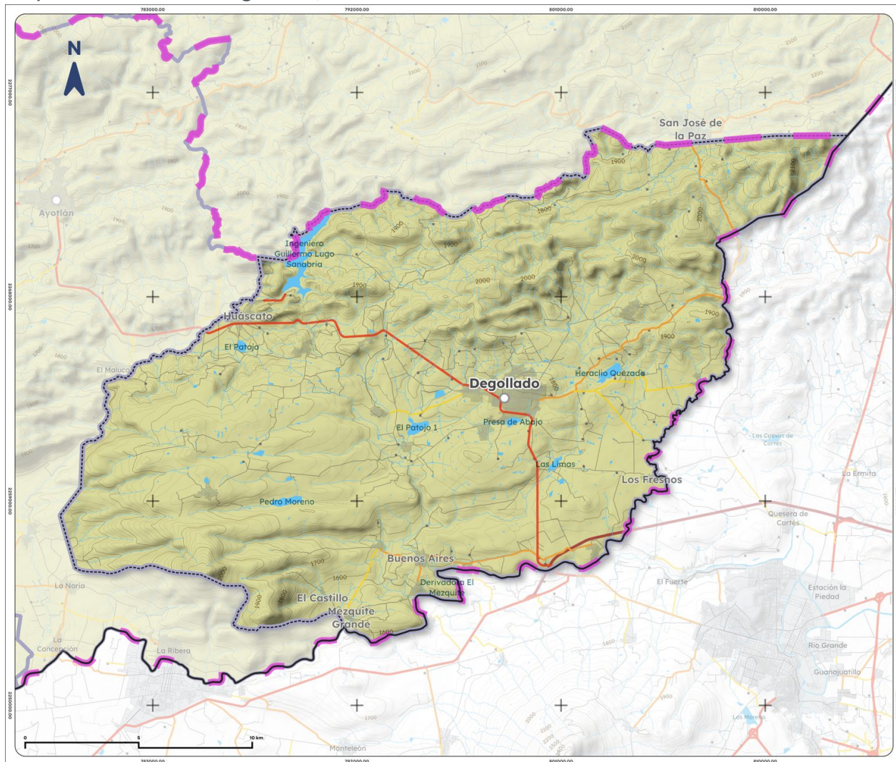
Mapa 6. Cuencas de Degollado, 2023
