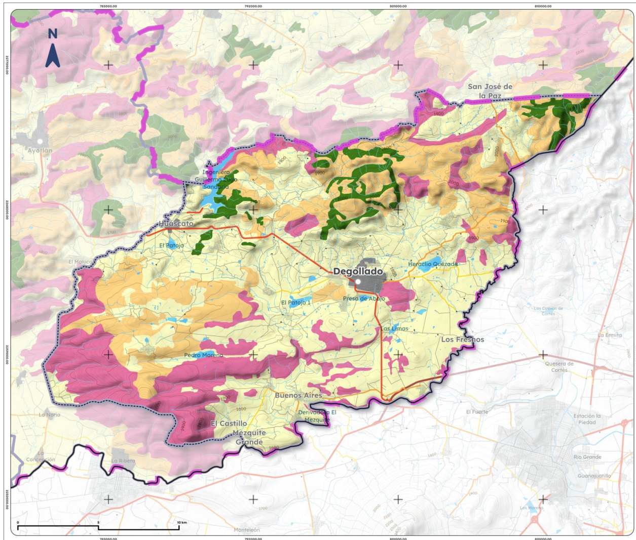
Mapa 11. Uso de suelo y vegetación de Degollado, 2018
