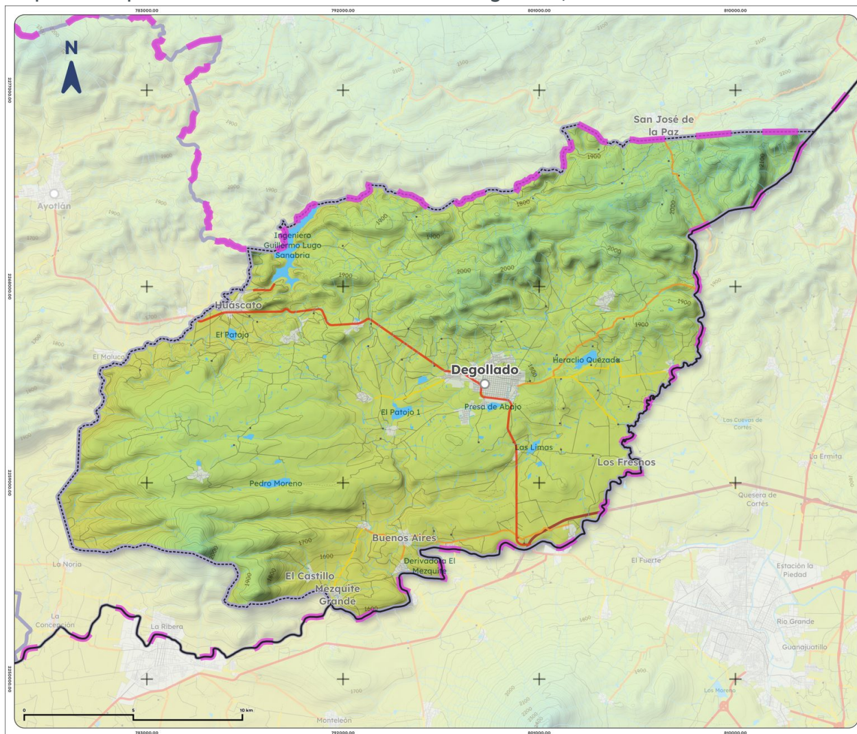
Mapa 8. Temperatura media anual histórica de Degollado, 1995-2025
