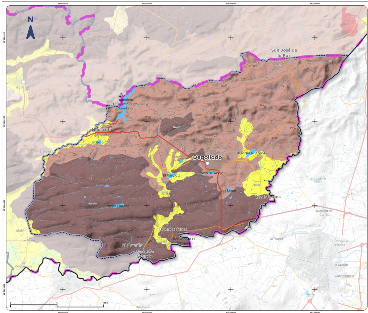
Mapa 3. Geología de Degollado, 1988
