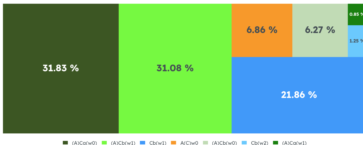
Clima de Chimaltitán, 1995-2025
