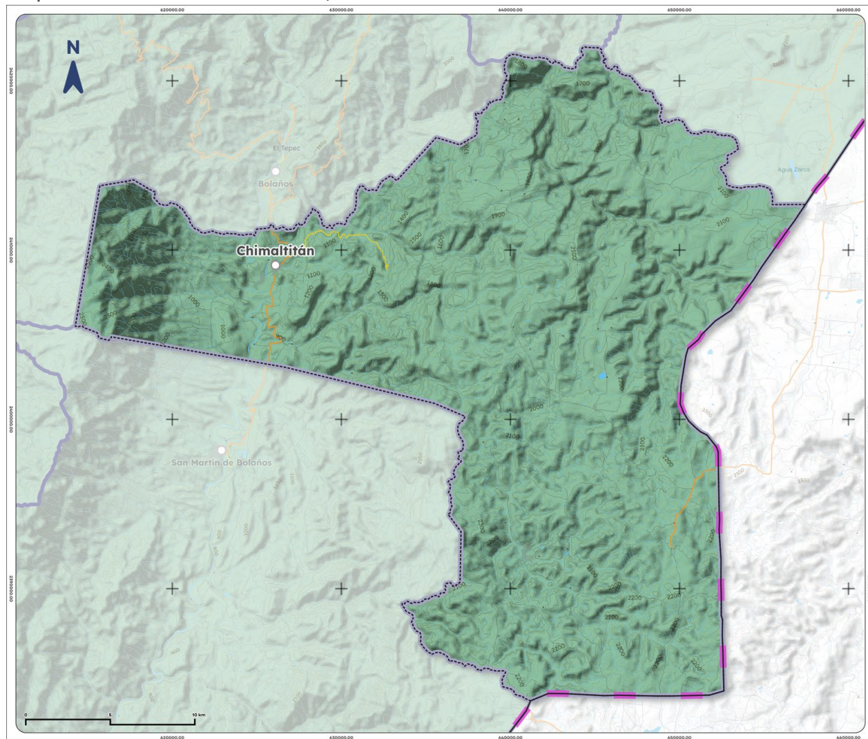
Mapa 7. Acuíferos de Chimaltitán, 2023
