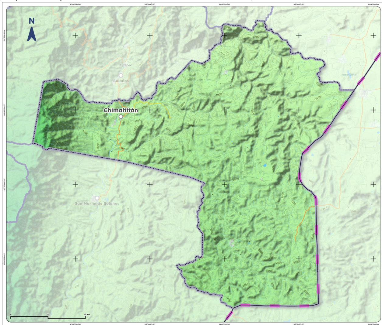
Mapa 9. Precipitación histórica acumulada de Chimaltitán, 1995-2025
