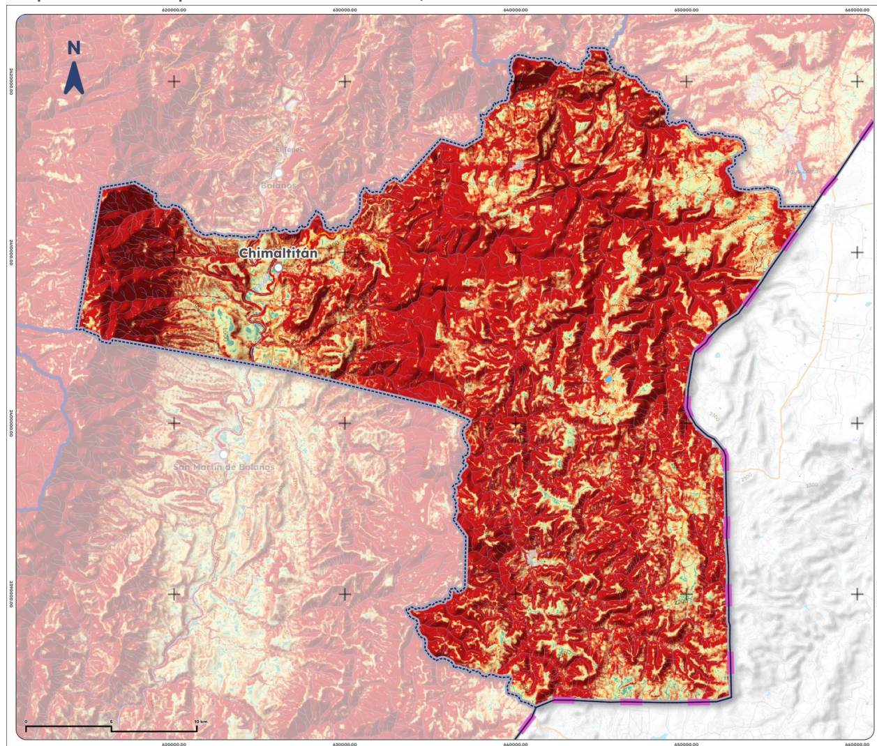
Mapa 16. Erosión potencial de Chimaltitán, 2025
