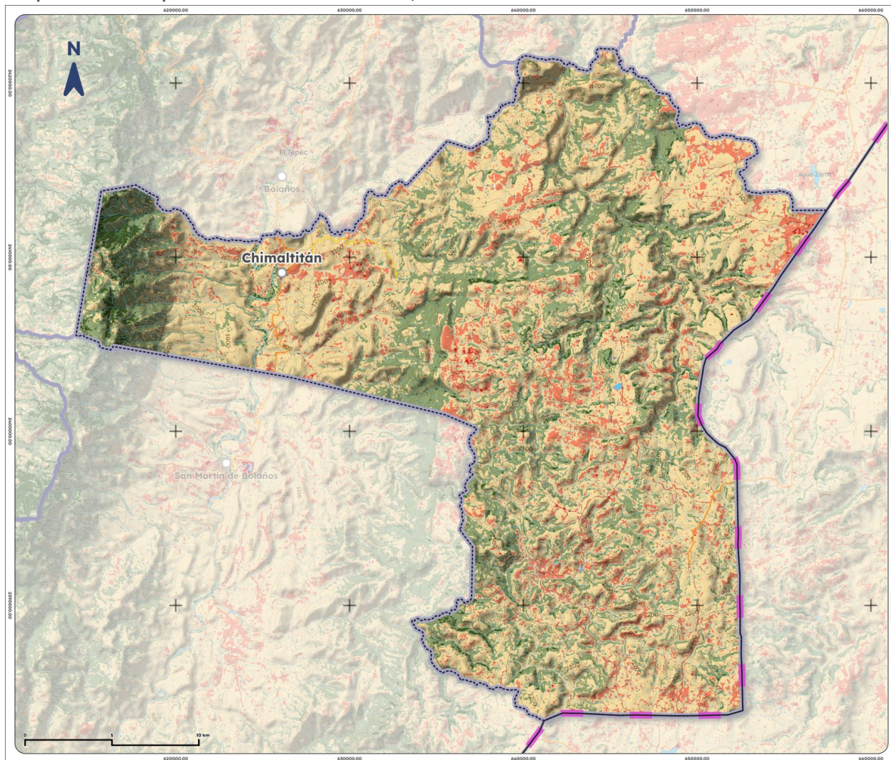
Mapa 12. NDVI promedio de Chimaltitán, 2025
