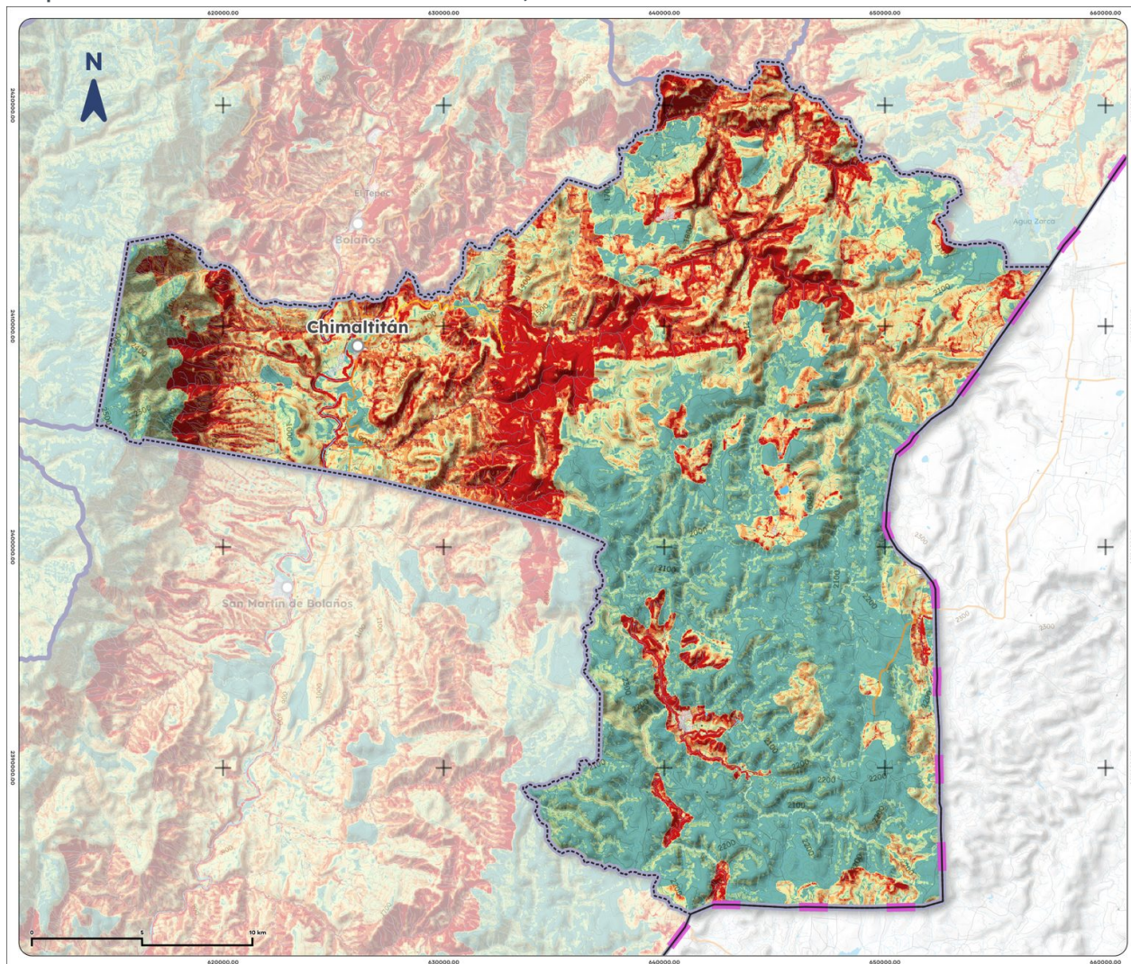
Mapa 17. Erosión efectiva de Chimaltitán, 2025
