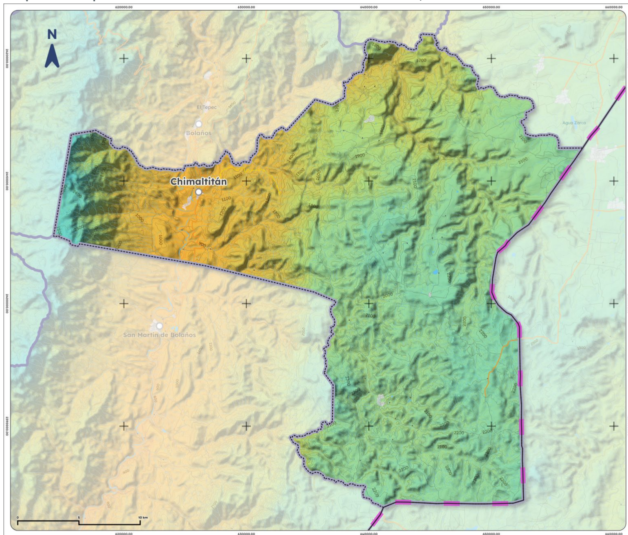
Mapa 8. Temperatura media anual histórica de Chimaltitán, 1995-2025
