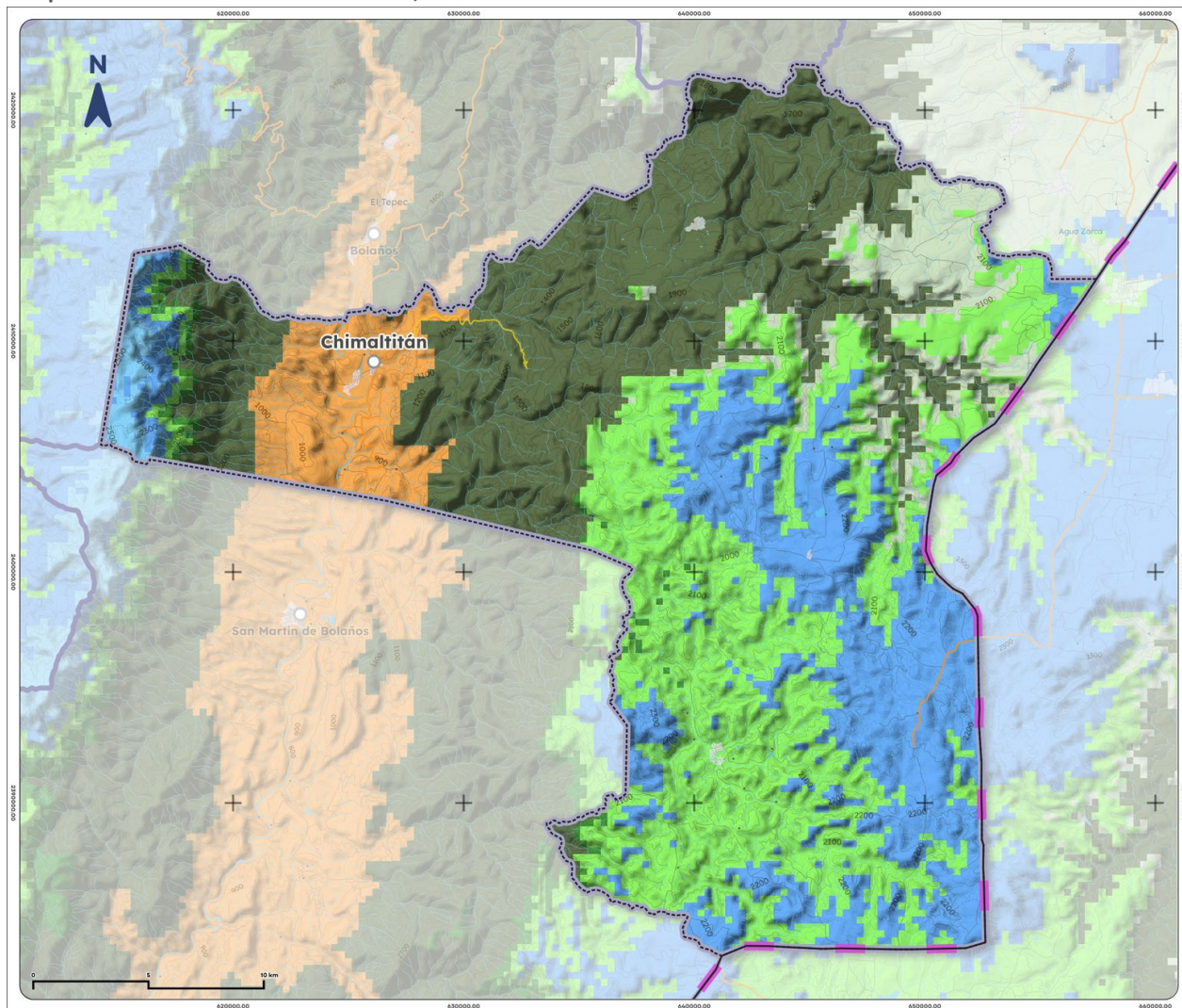
Mapa 10. Clima de Chimaltitán, 1995-2025
