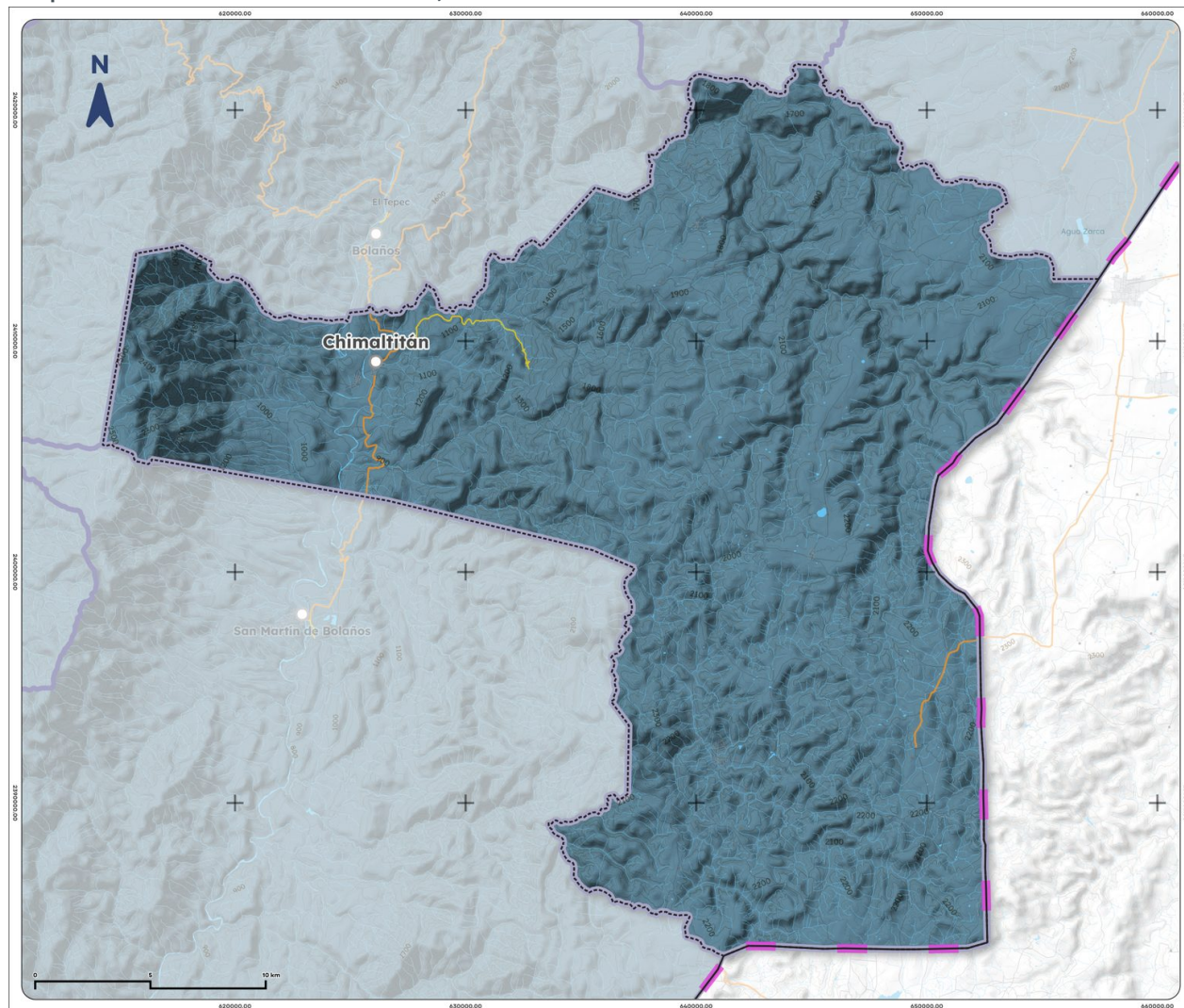
Mapa 6. Cuencas de Chimaltitán, 2023
