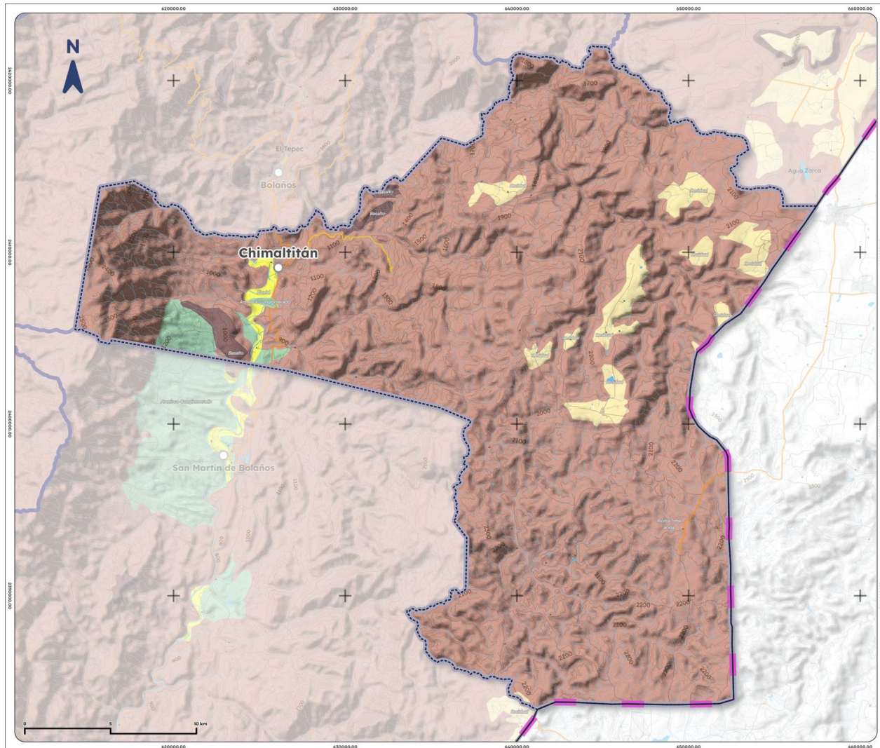
Mapa 3. Geología de Chimaltitán, 1988
