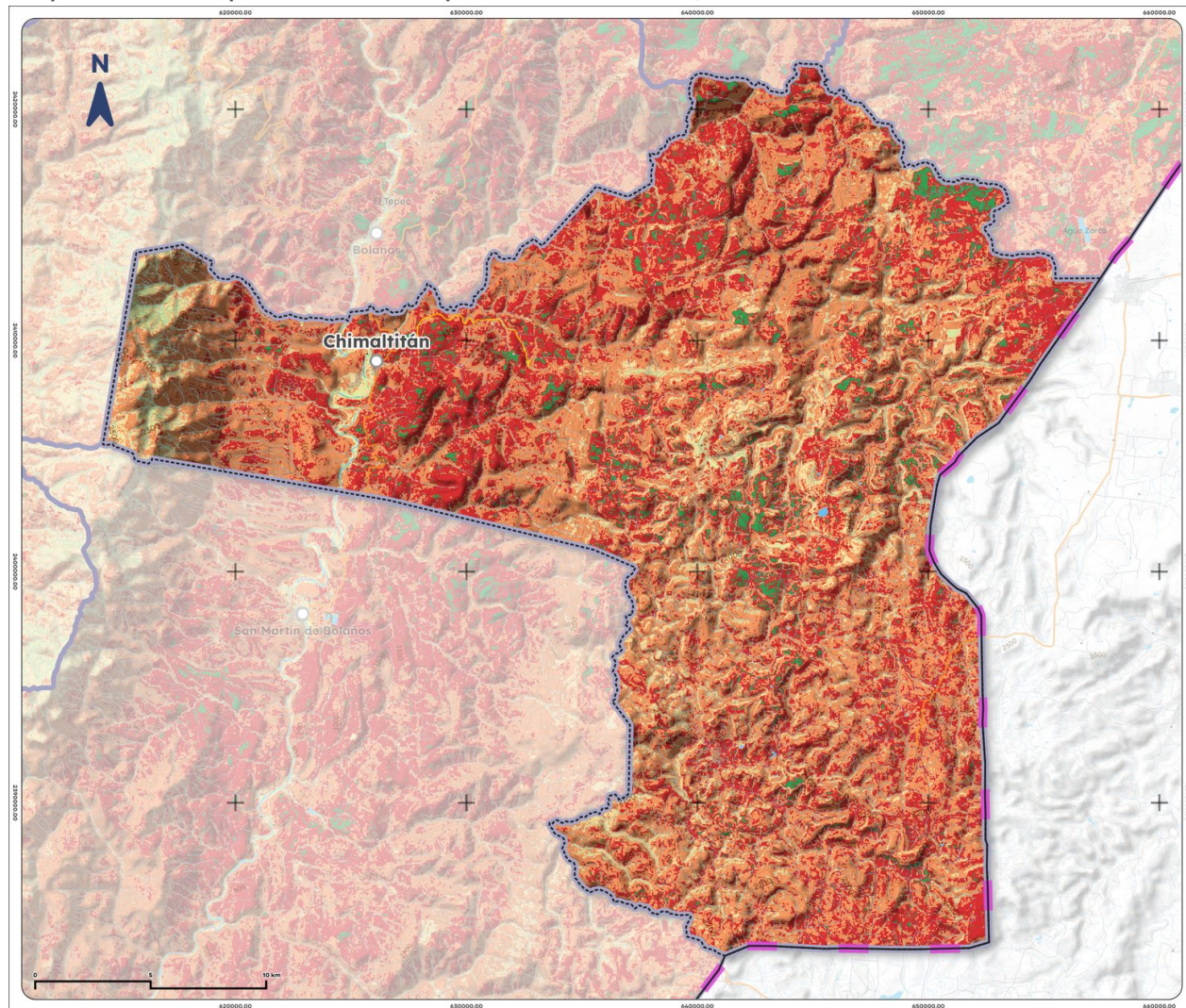
Mapa 15. Índice promedio de sequía de Chimaltitán, 2025
