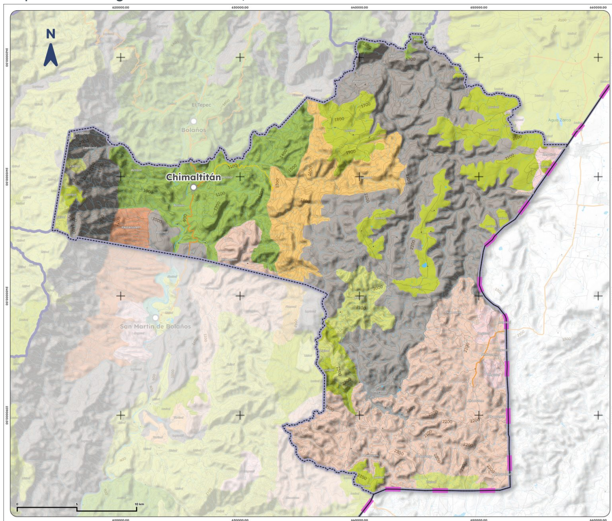
Mapa 4. Edafología de Chimaltitán, 2025
