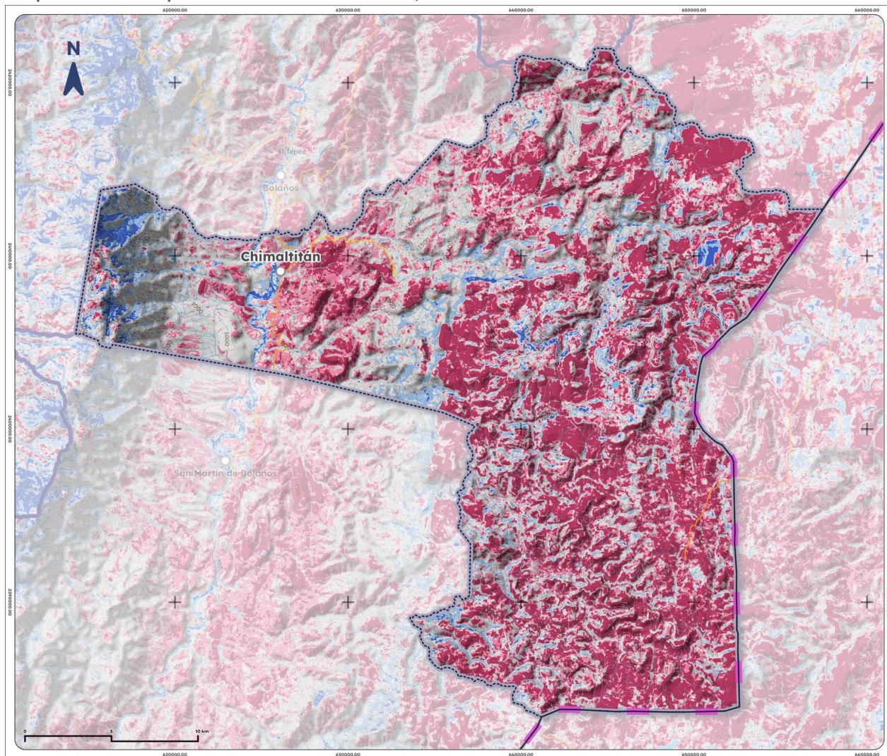
Mapa 13. NDWI promedio de Chimaltitán, 2025
