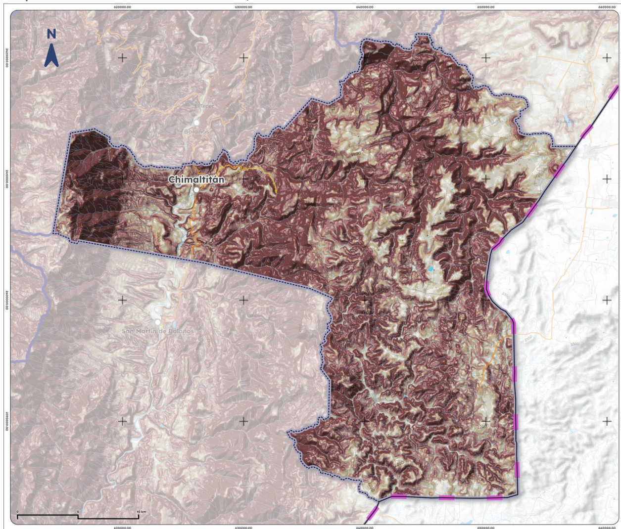
Mapa 5. Pendientes de Chimaltitán, 2025
