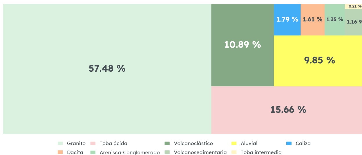
Geología de Cuautitlán de García Barragán, 1988
