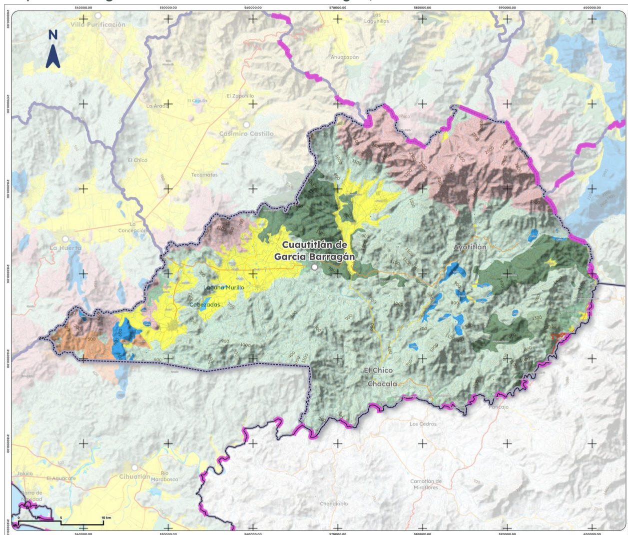
Mapa 3. Geología de Cuautitlán de García Barragán, 1988
