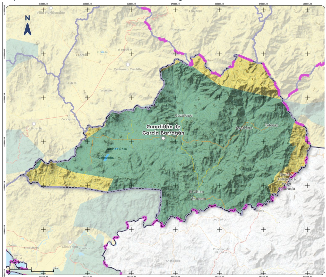
Mapa 7. Acuíferos de Cuautitlán de García Barragán, 2023
