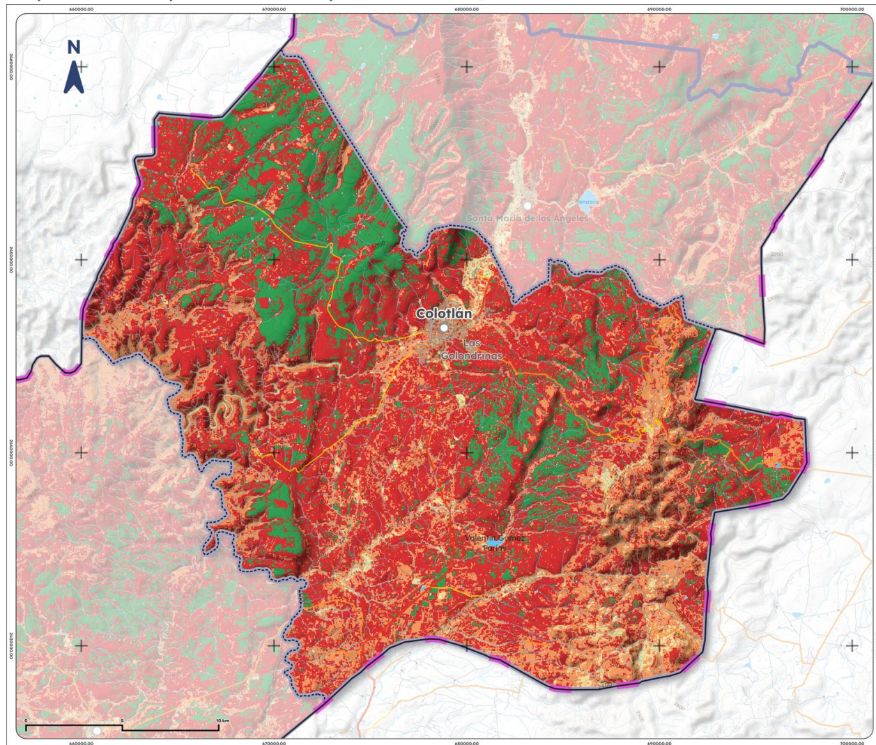
Mapa 15. Índice promedio de sequía de Colotlán, 2025
