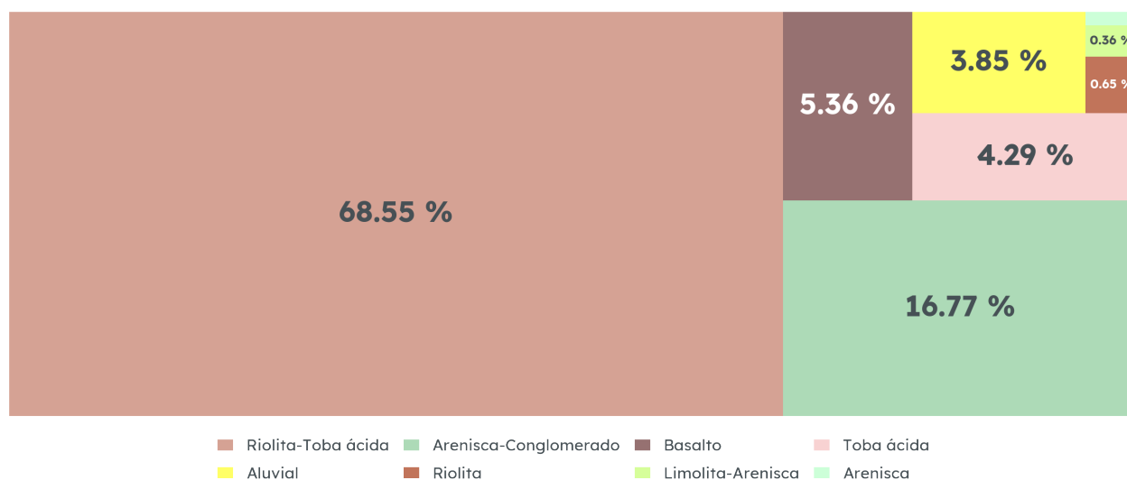
Geología de Colotlán, 1988
