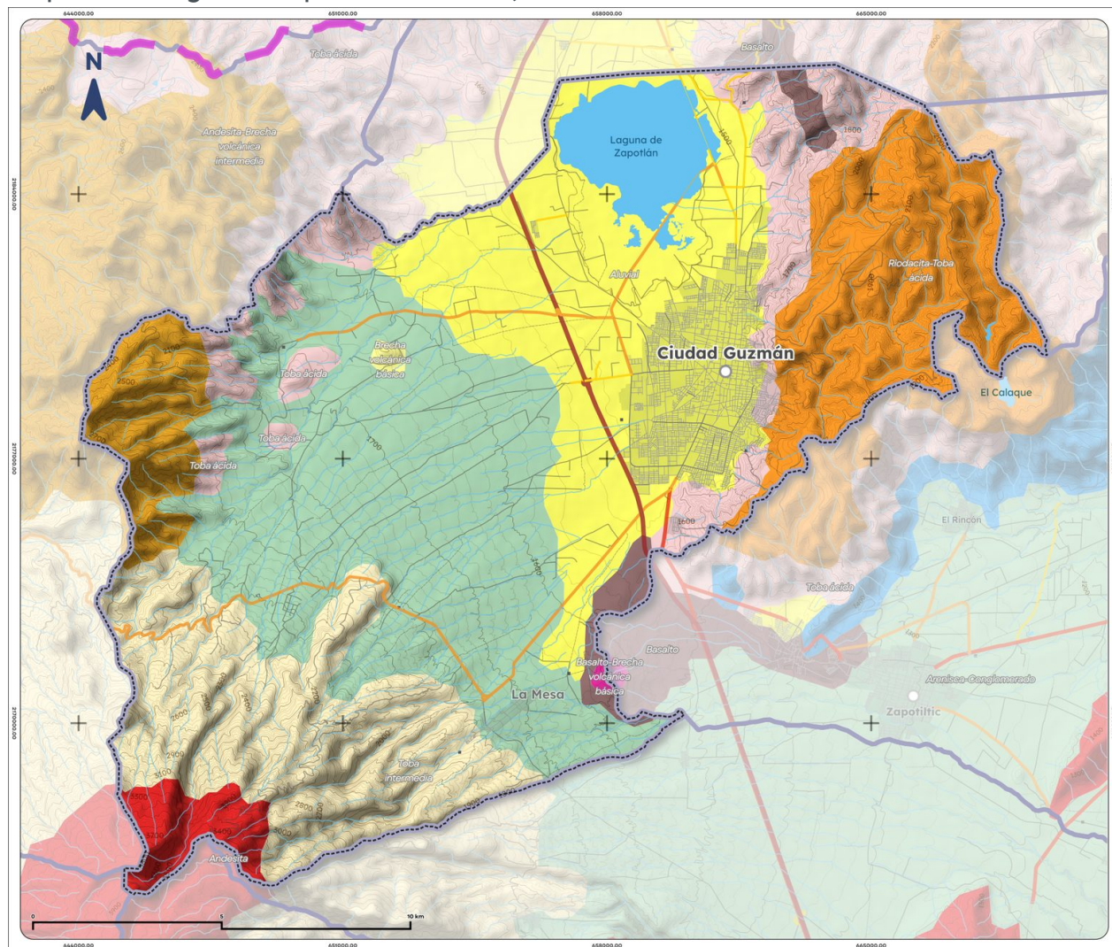
Mapa 3. Geología de Zapotlán el Grande, 1988
