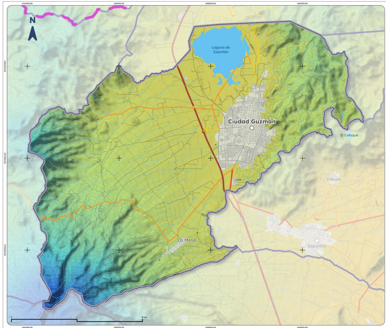
Mapa 8. Temperatura media anual histórica de Zapotlán el Grande, 1995-2025
