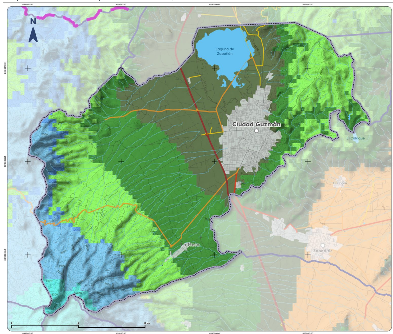
Mapa 10. Clima de Zapotlán el Grande, 1995-2025
