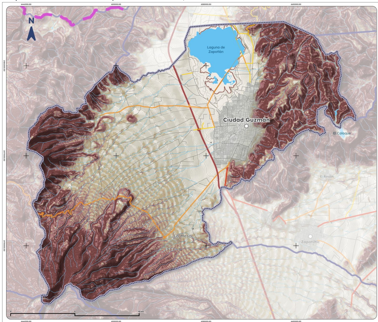
Mapa 5. Pendientes de Zapotlán el Grande, 2025
