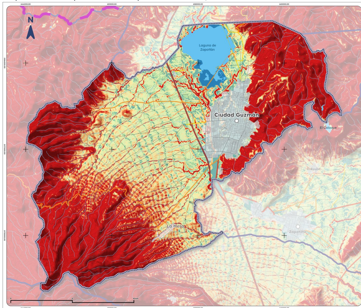
Mapa 16. Erosión potencial de Zapotlán el Grande, 2025
