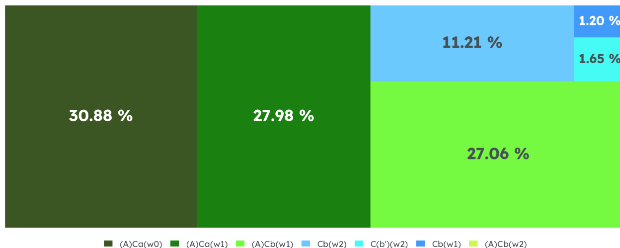
Clima de Zapotlán el Grande, 1995-2025
