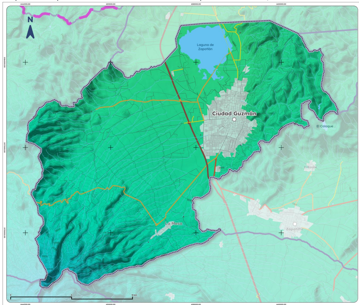
Mapa 9. Precipitación histórica acumulada de Zapotlán el Grande, 1995-2025
