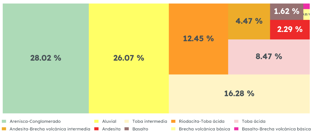
Geología de Zapotlán el Grande, 1988
