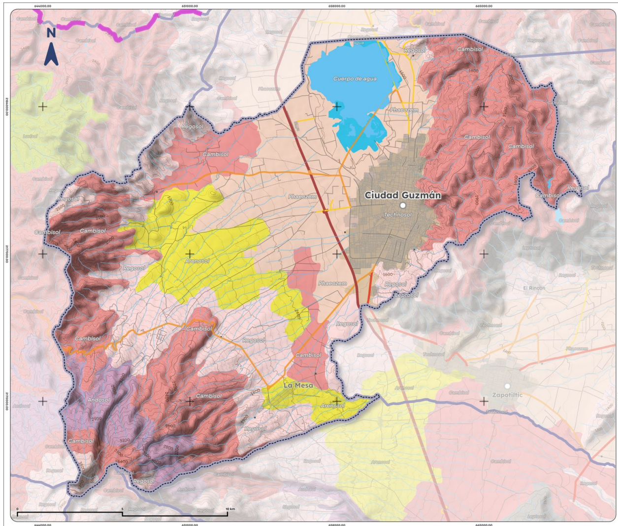
Mapa 4. Edafología de Zapotlán el Grande, 2025
