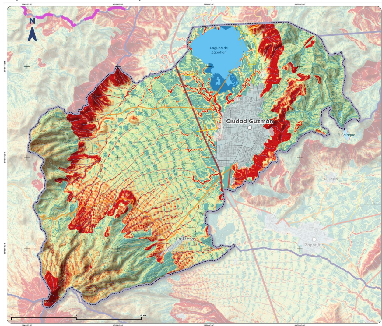
Mapa 17. Erosión efectiva de Zapotlán el Grande, 2025
