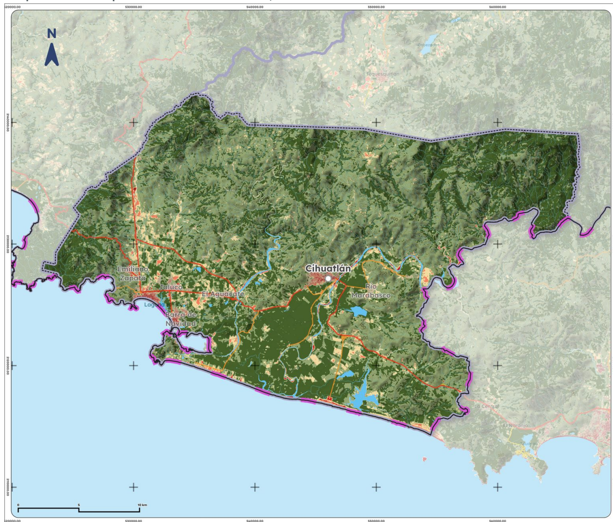
Mapa 12. NDVI promedio de Cihuatlán, 2025
