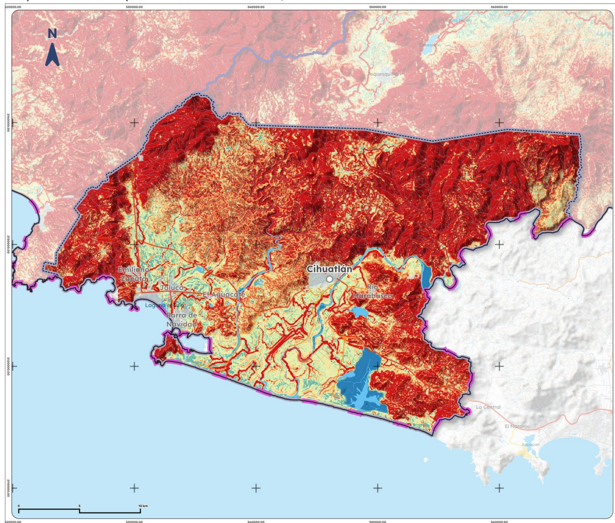
Mapa 16. Erosión potencial de Cihuatlán, 2025
