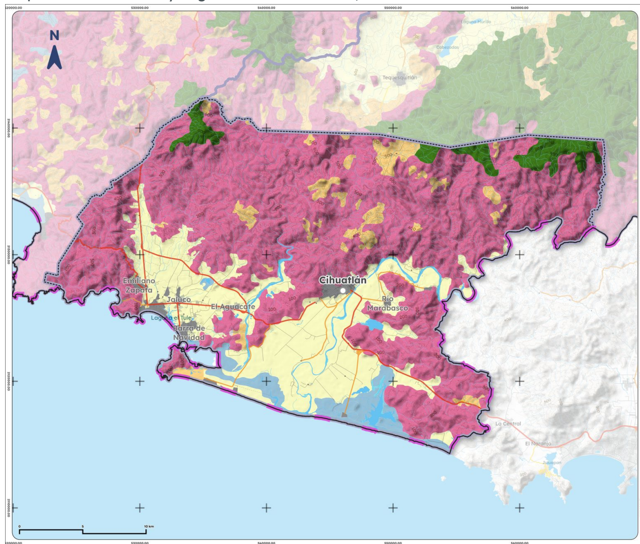
Mapa 11. Uso de suelo y vegetación de Cihuatlán, 2018
