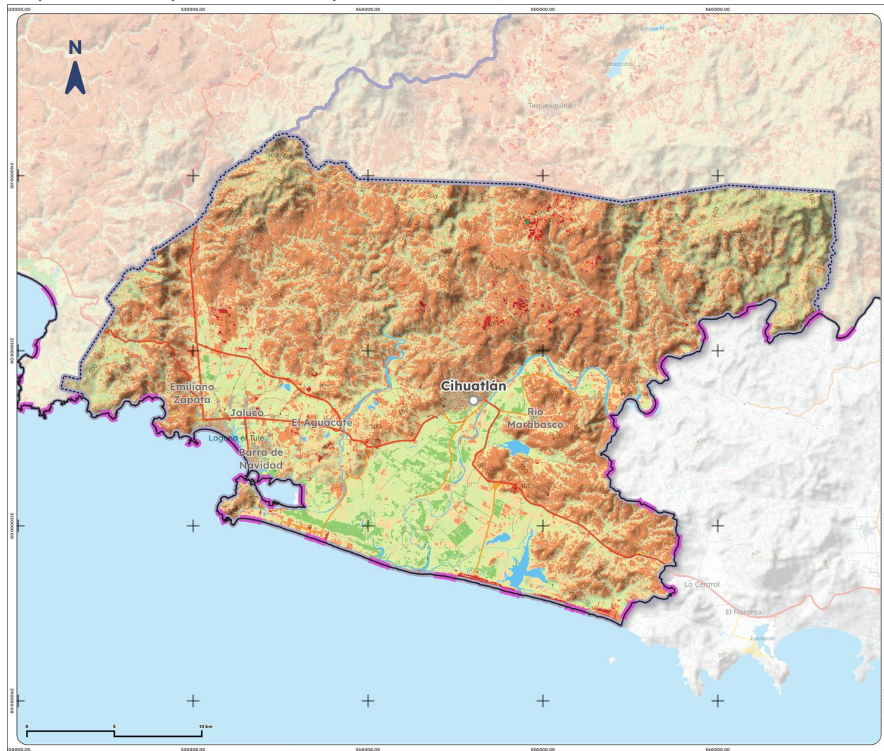
Mapa 15. Índice promedio de sequía de Cihuatlán, 2025
