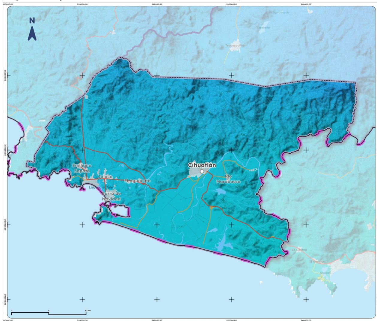
Mapa 9. Precipitación histórica acumulada de Cihuatlán, 1995-2025
