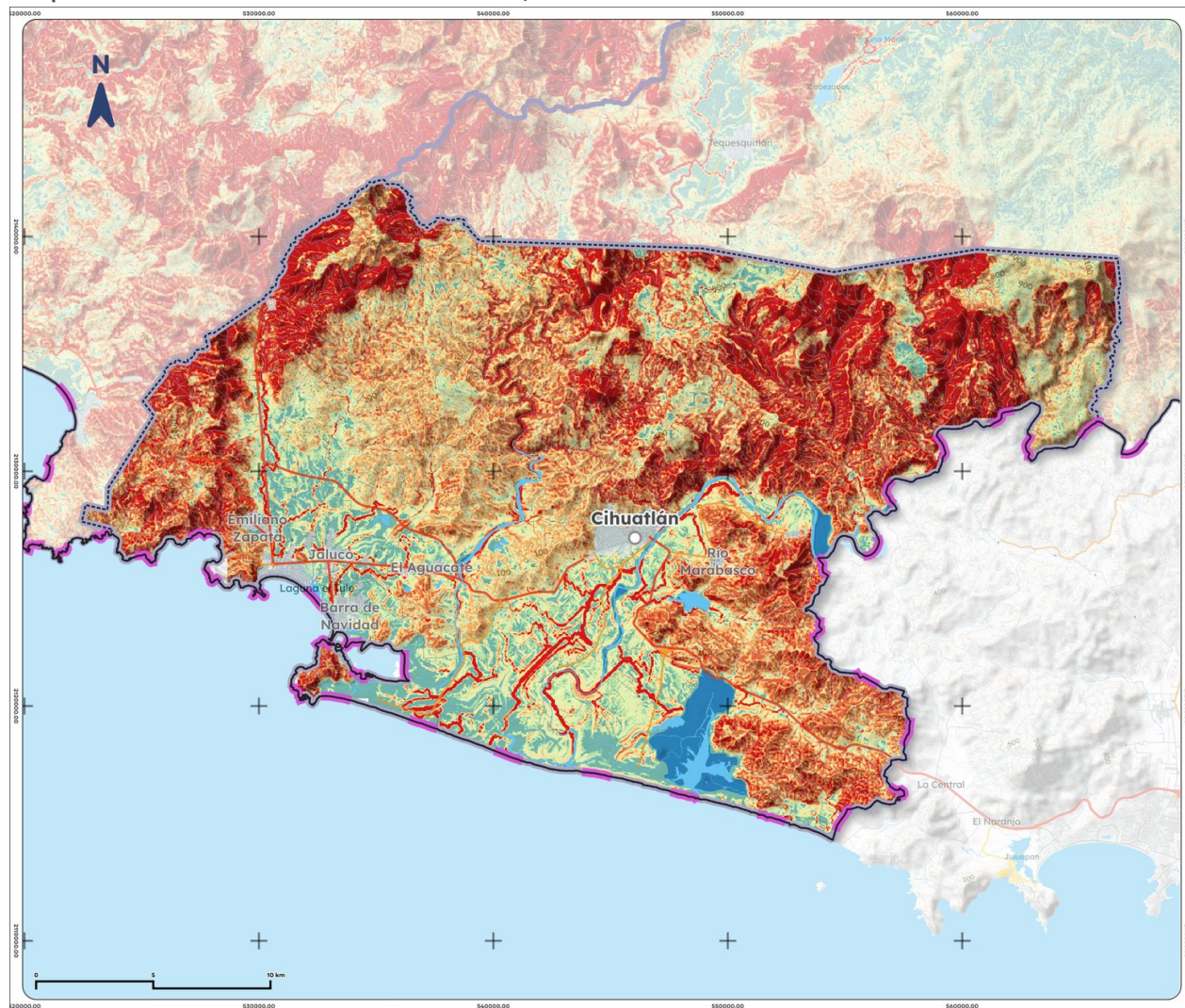
Mapa 17. Erosión efectiva de Cihuatlán, 2025
