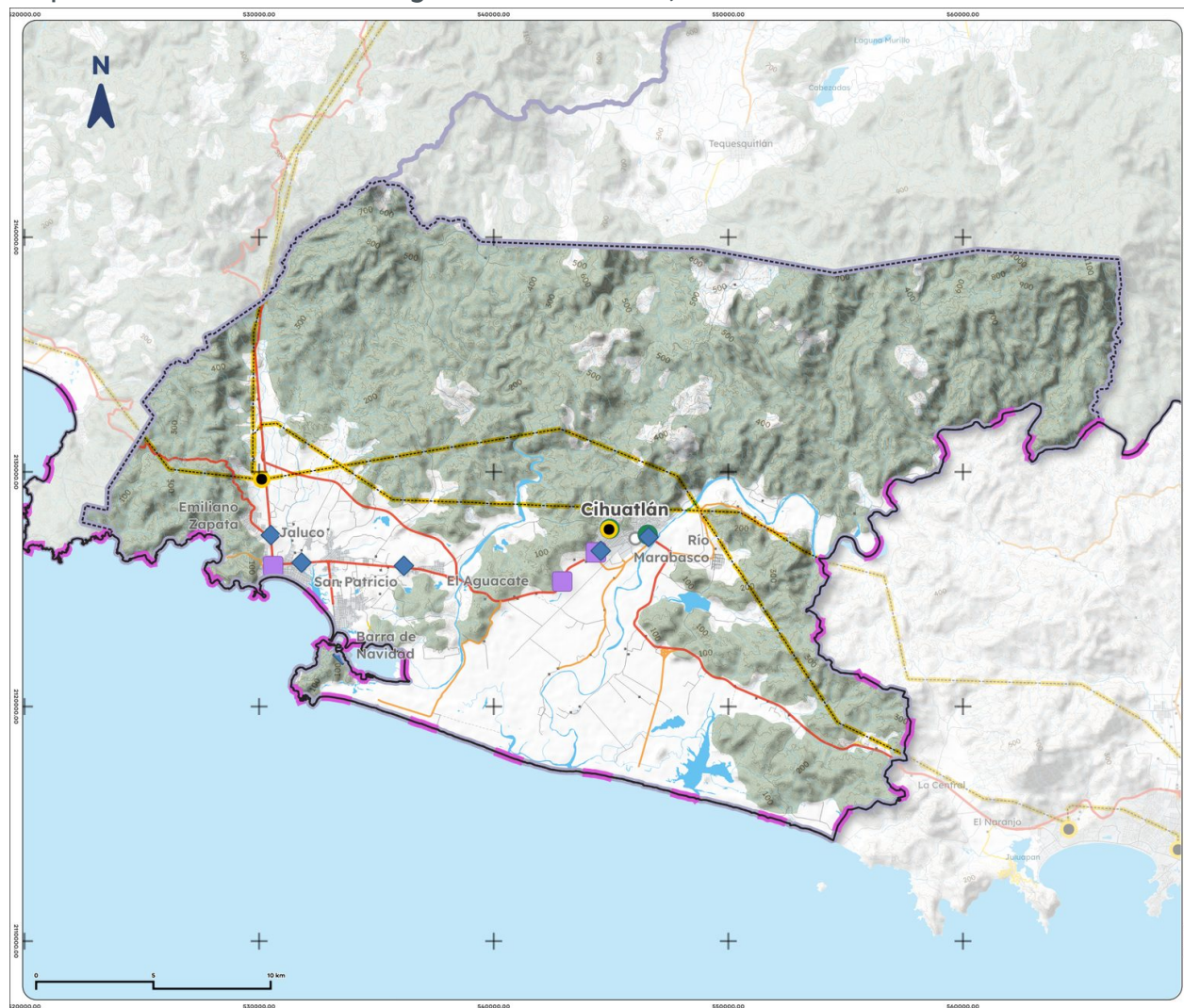
Mapa 22. Infraestructura energética de Cihuatlán, 2025
