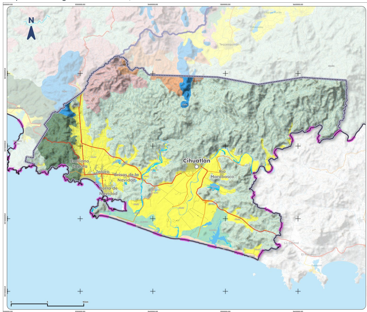
Mapa 3. Geología de Cihuatlán, 1988
