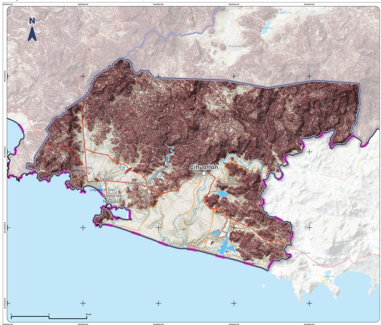
Mapa 5. Pendientes de Cihuatlán, 2025
