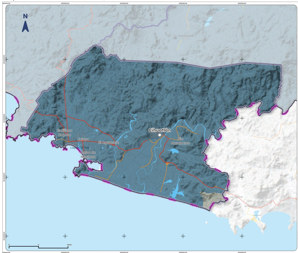
Mapa 6. Cuencas de Cihuatlán, 2023
