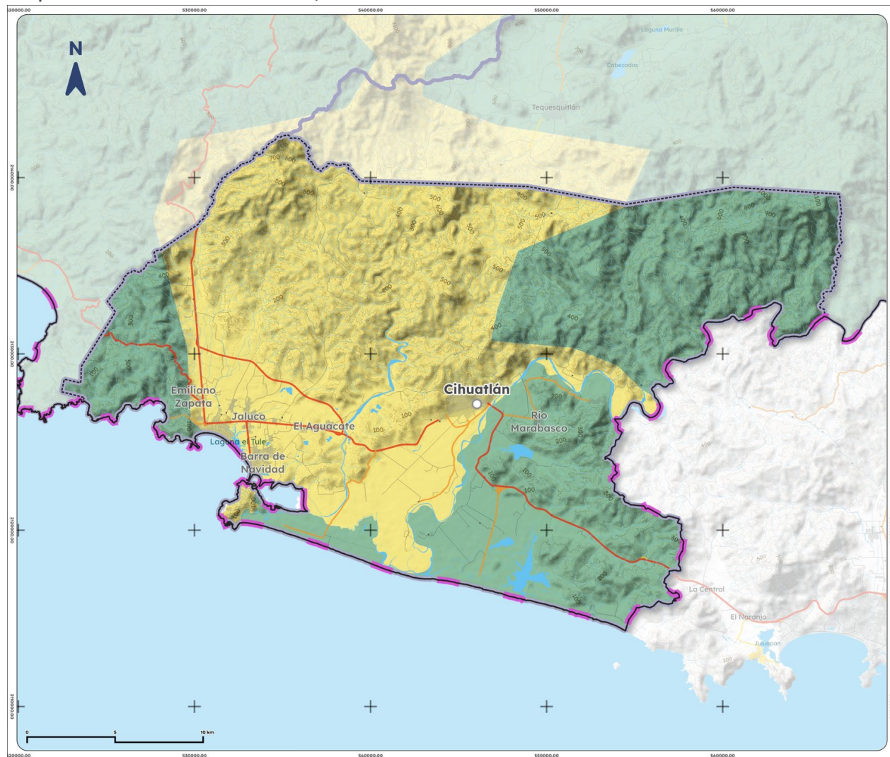
Mapa 7. Acuíferos de Cihuatlán, 2023
