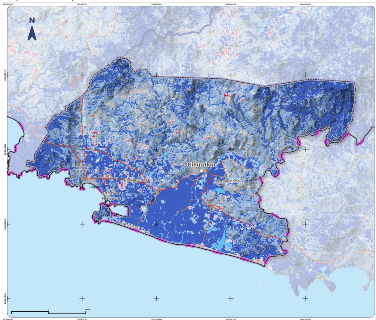
Mapa 13. NDWI promedio de Cihuatlán, 2025
