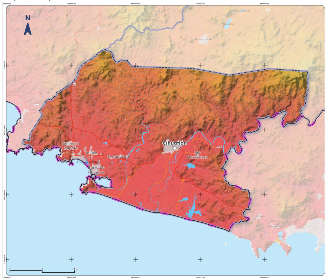
Mapa 8. Temperatura media anual histórica de Cihuatlán, 1995-2025
