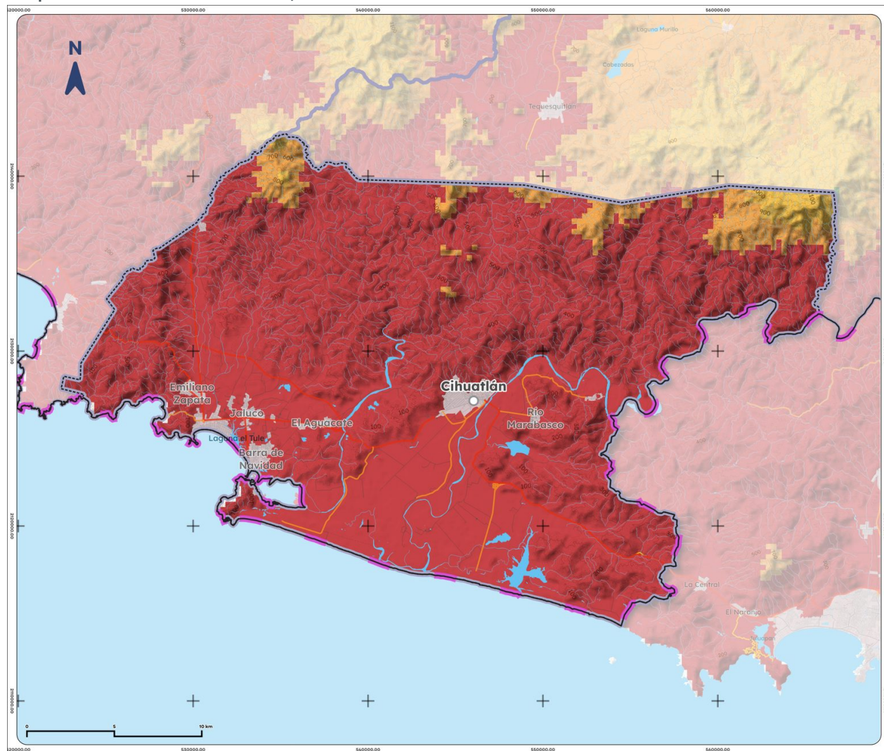
Mapa 10. Clima de Cihuatlán, 1995-2025
