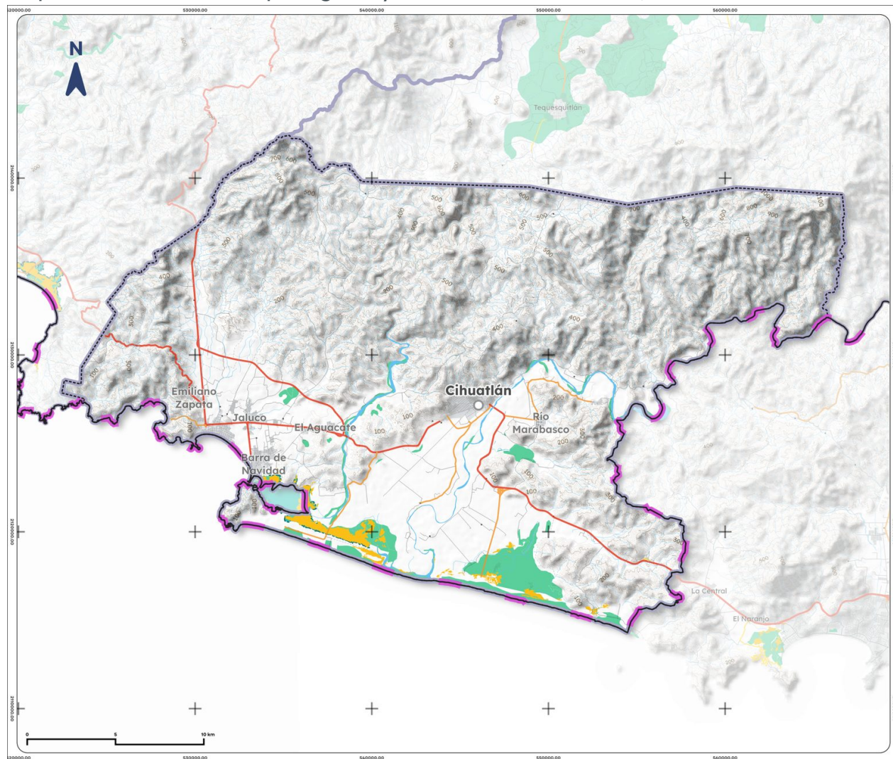
Mapa 14. Áreas naturales protegidas y humedales de Cihuatlán, 2025
