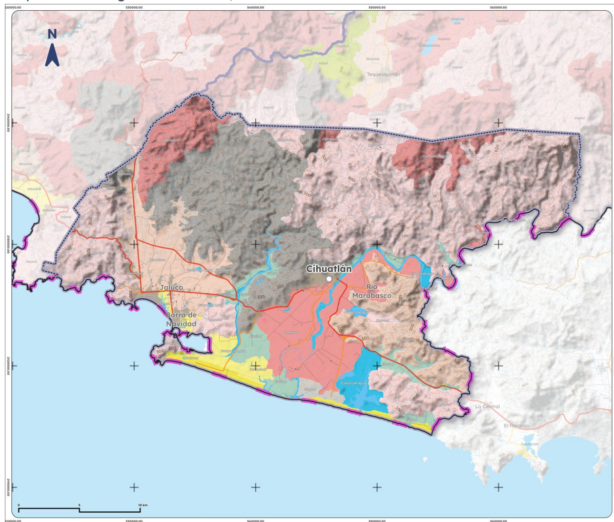
Mapa 4. Edafología de Cihuatlán, 2025
