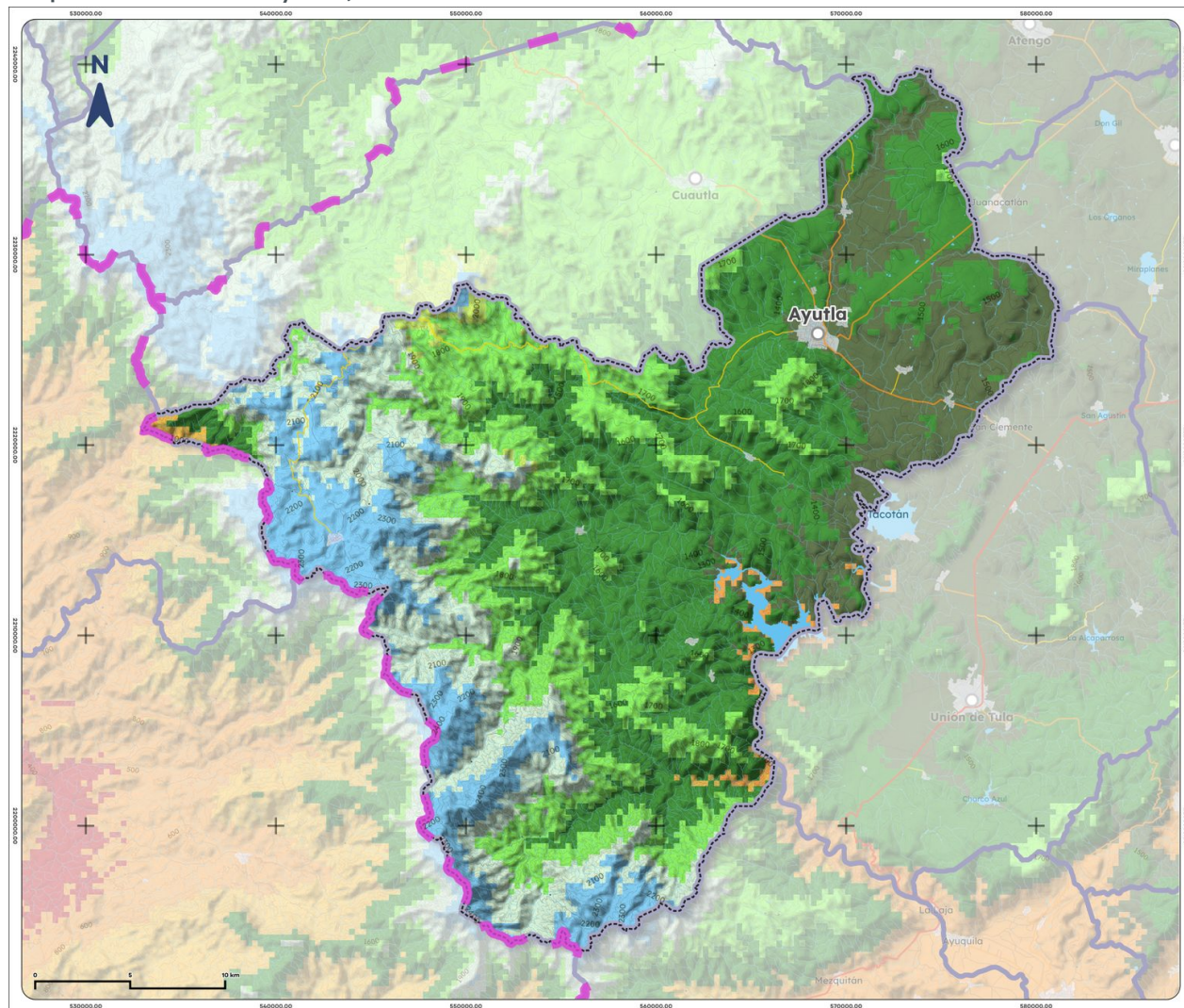
Mapa 10. Clima de Ayutla, 1995-2025
