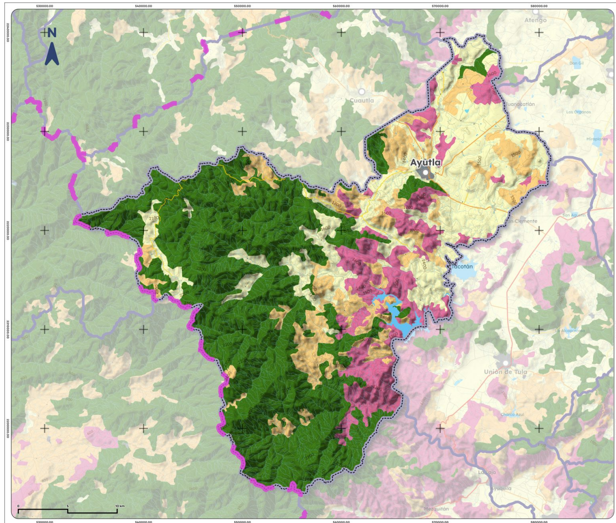
Mapa 11. Uso de suelo y vegetación de Ayutla, 2018
