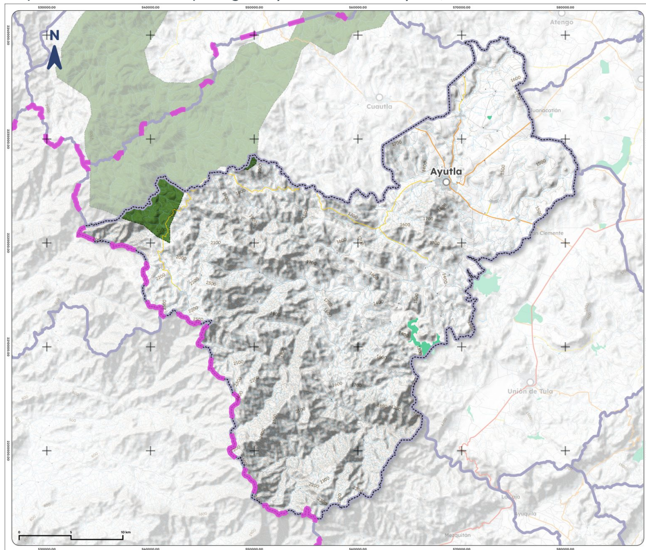
Mapa 14. Áreas naturales protegidas y humedales de Ayutla, 2025
