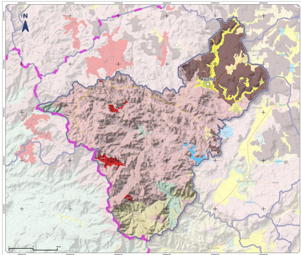
Mapa 3. Geología de Ayutla, 1988
