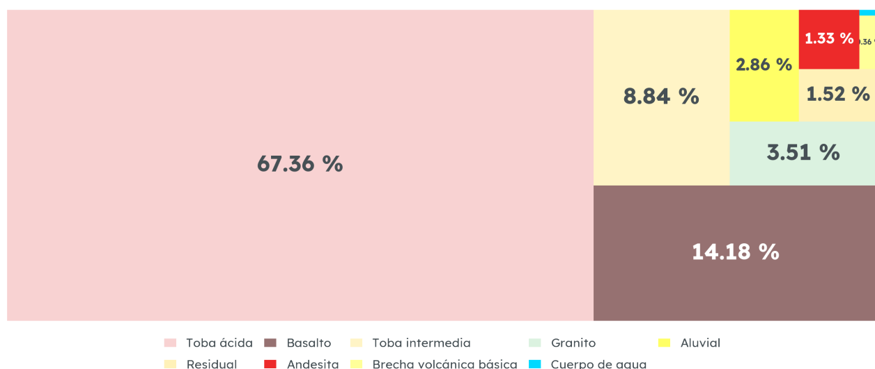
Geología de Ayutla, 1988
