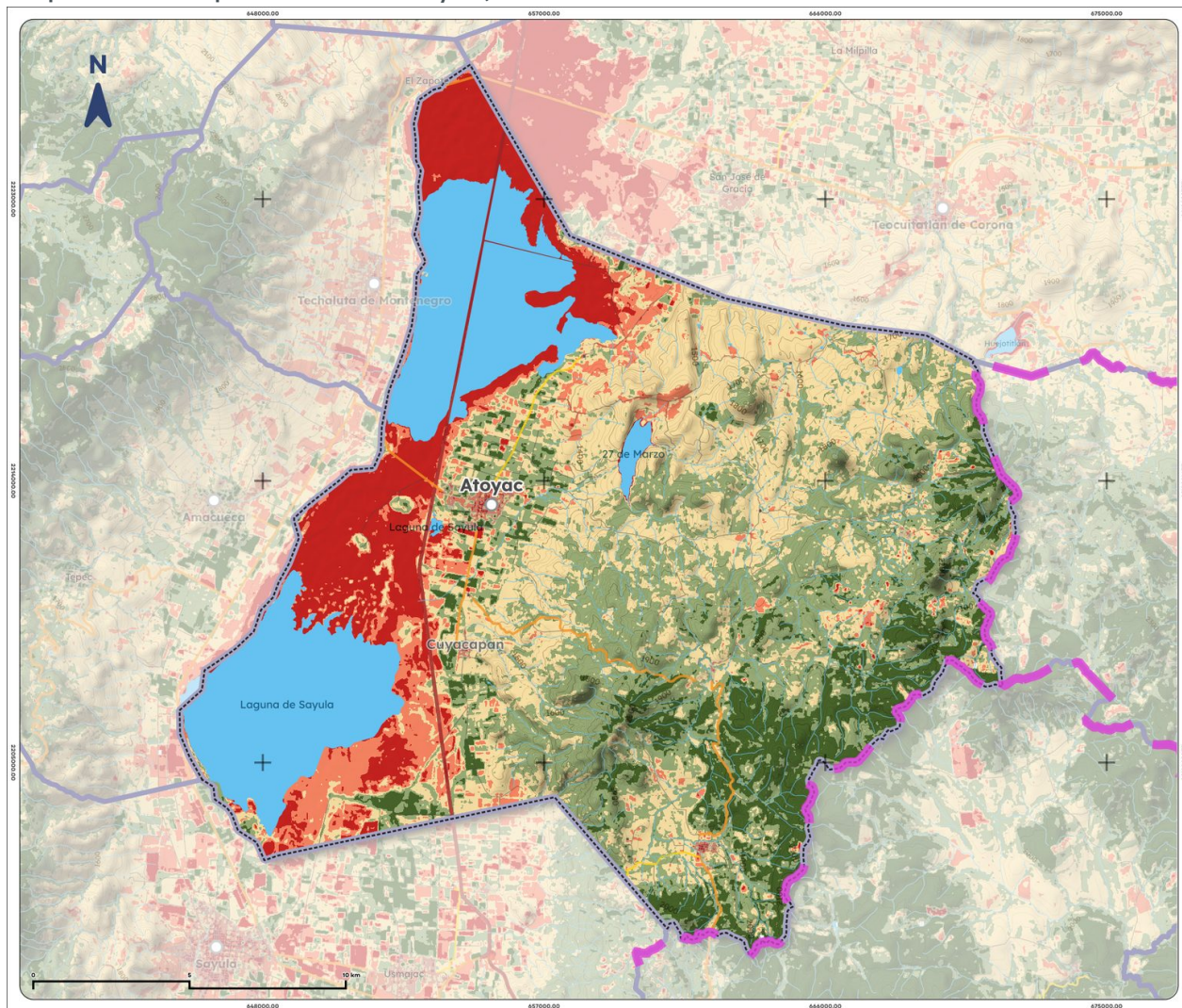
Mapa 12. NDVI promedio de Atoyac, 2025
