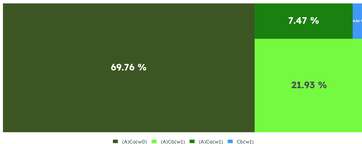
Clima de Atoyac, 1995-2025
