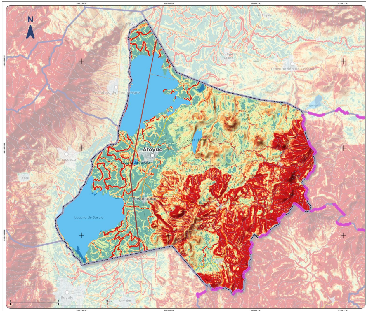
Mapa 16. Erosión potencial de Atoyac, 2025
