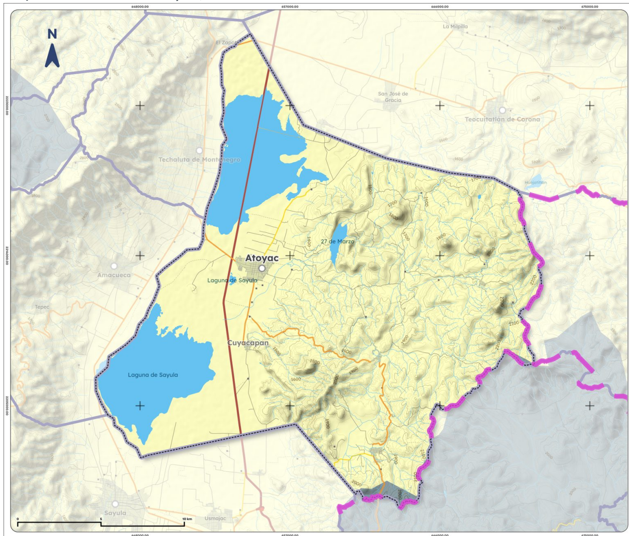
Mapa 6. Cuencas de Atoyac, 2023
