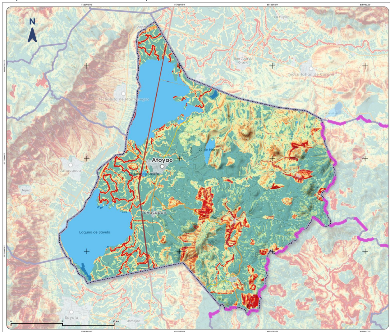
Mapa 17. Erosión efectiva de Atoyac, 2025
