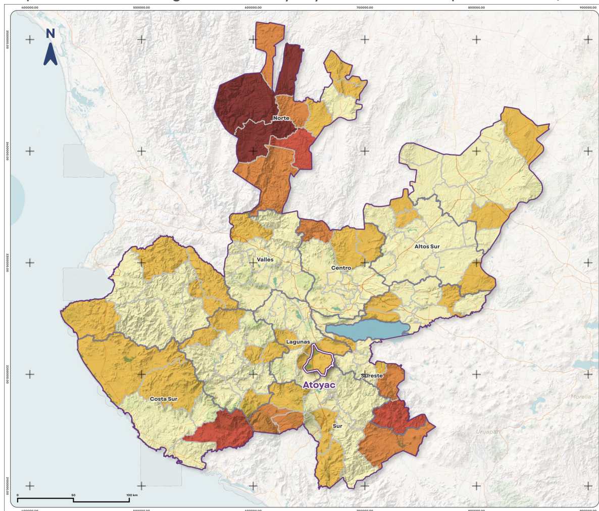
Mapa 25. Grado de marginación en Atoyac y el resto de municipios de Jalisco, 2020
