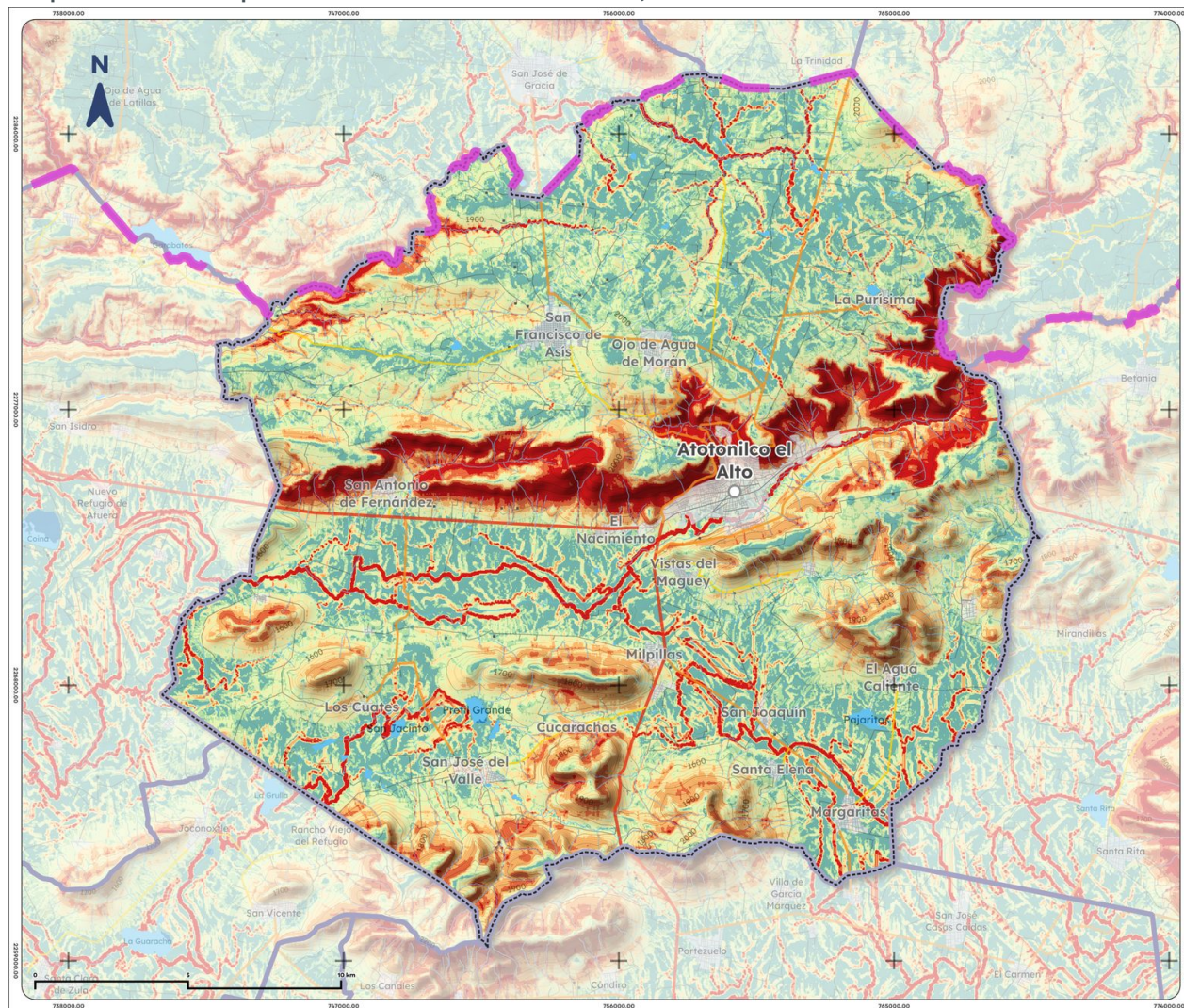
Mapa 16. Erosión potencial de Atotonilco el Alto, 2025
