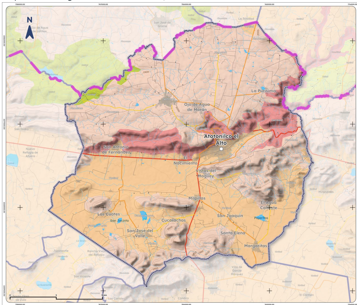
Mapa 4. Edafología de Atotonilco el Alto, 2025
