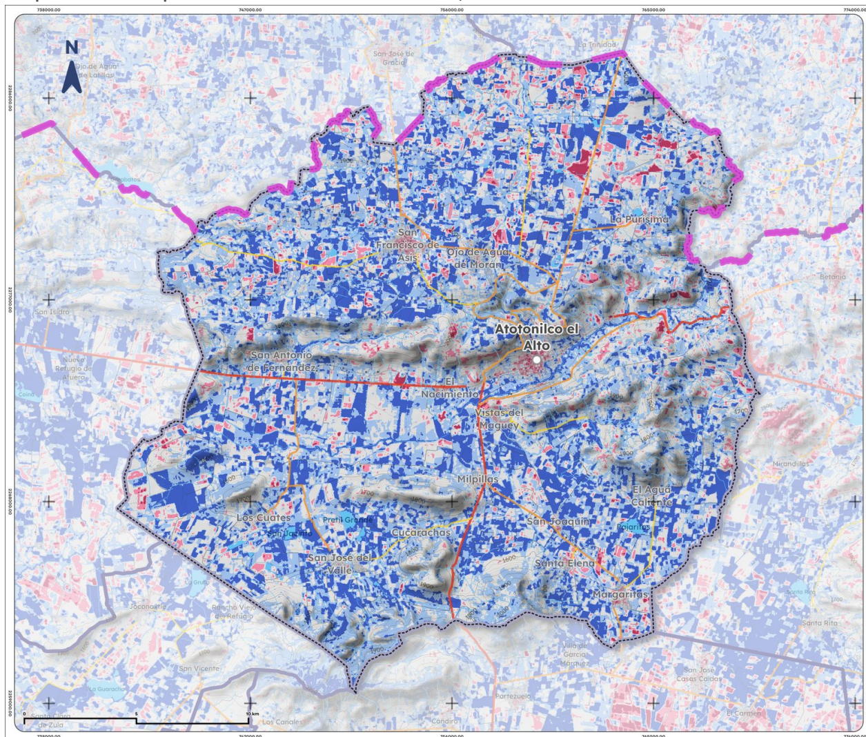
Mapa 13. NDWI promedio de Atotonilco el Alto, 2025
