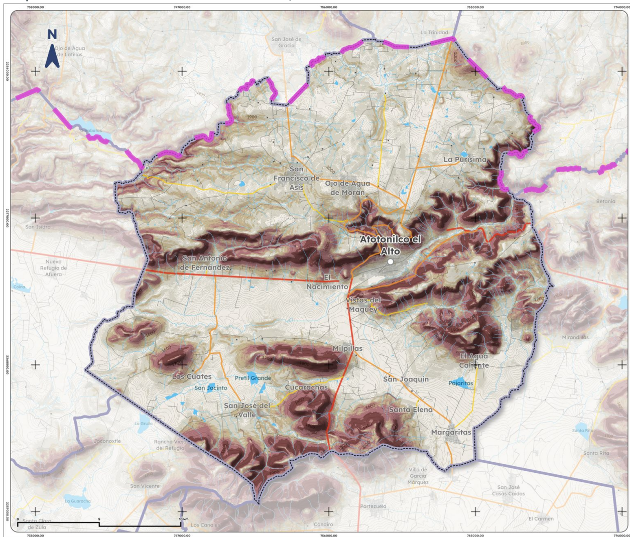
Mapa 5. Pendientes de Atotonilco el Alto, 2025
