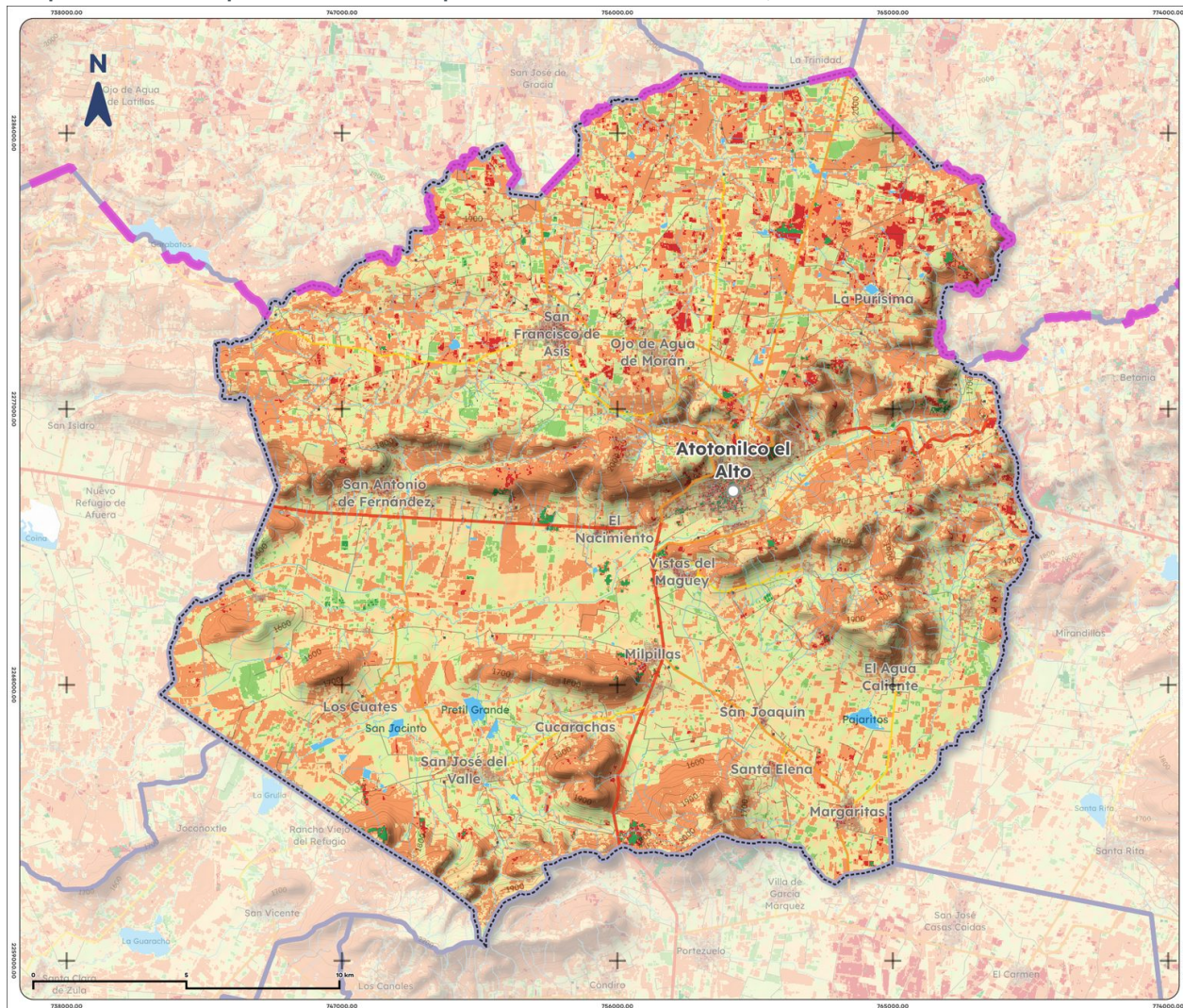
Mapa 15. Índice promedio de sequía de Atotonilco el Alto, 2025
