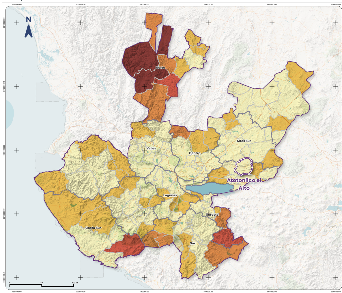
Mapa 25. Grado de marginación en Atotonilco el Alto y el resto de municipios de Jalisco, 2020
