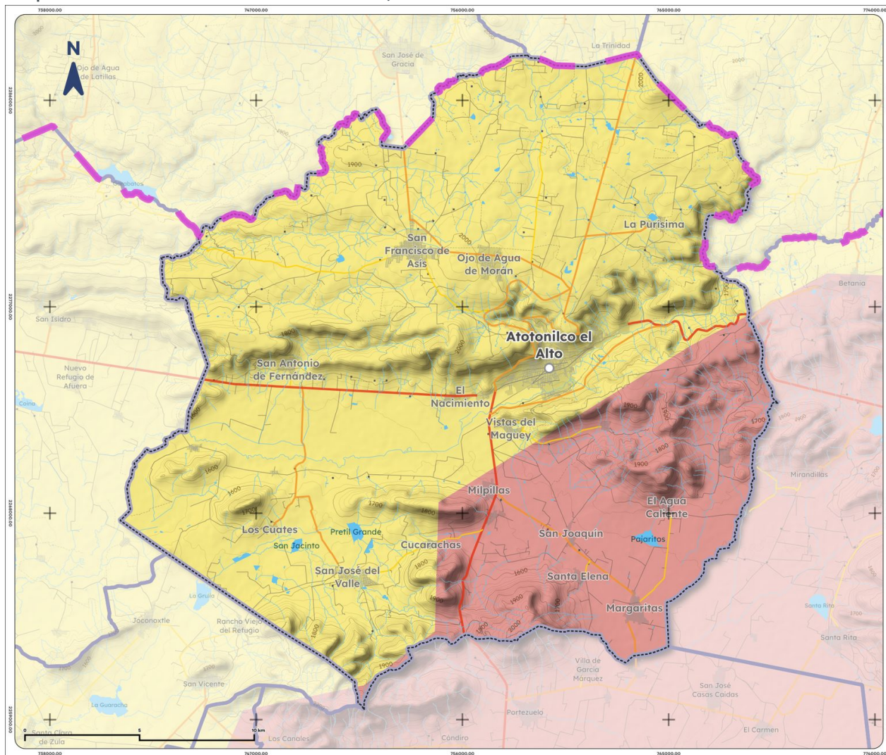
Mapa 7. Acuíferos de Atotonilco el Alto, 2023
