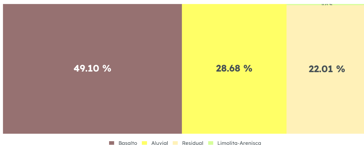
Geología de Atotonilco el Alto, 1988
