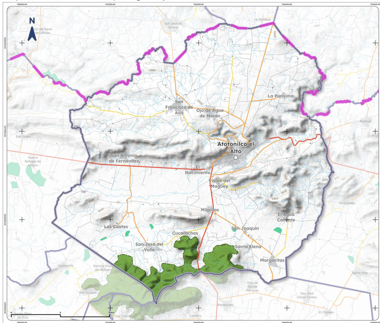
Mapa 14. Áreas naturales protegidas y humedales de Atotonilco el Alto, 2025
