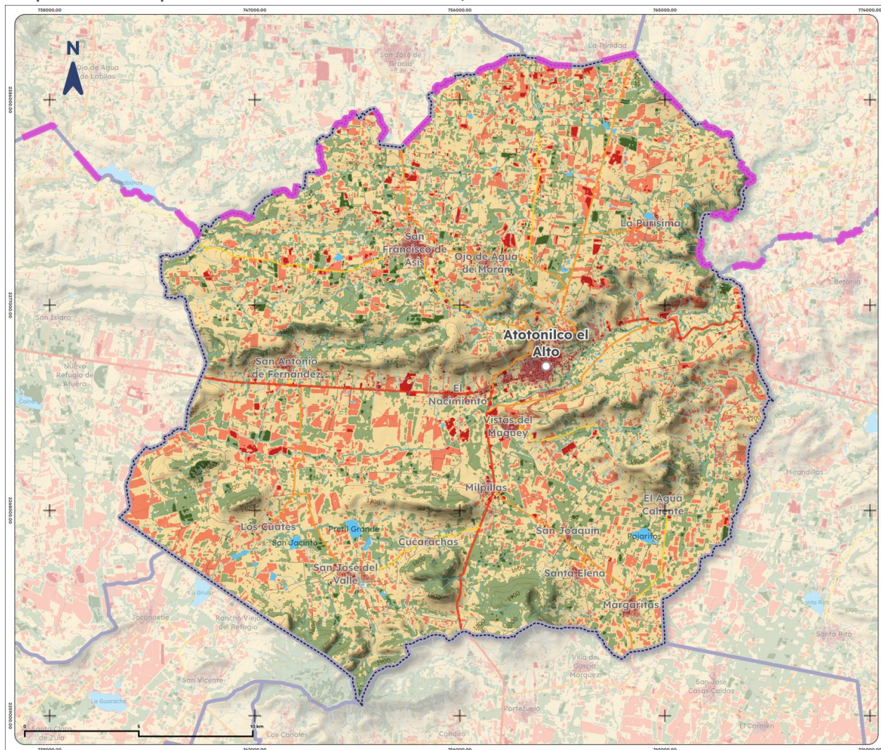
Mapa 12. NDVI promedio de Atotonilco el Alto, 2025
