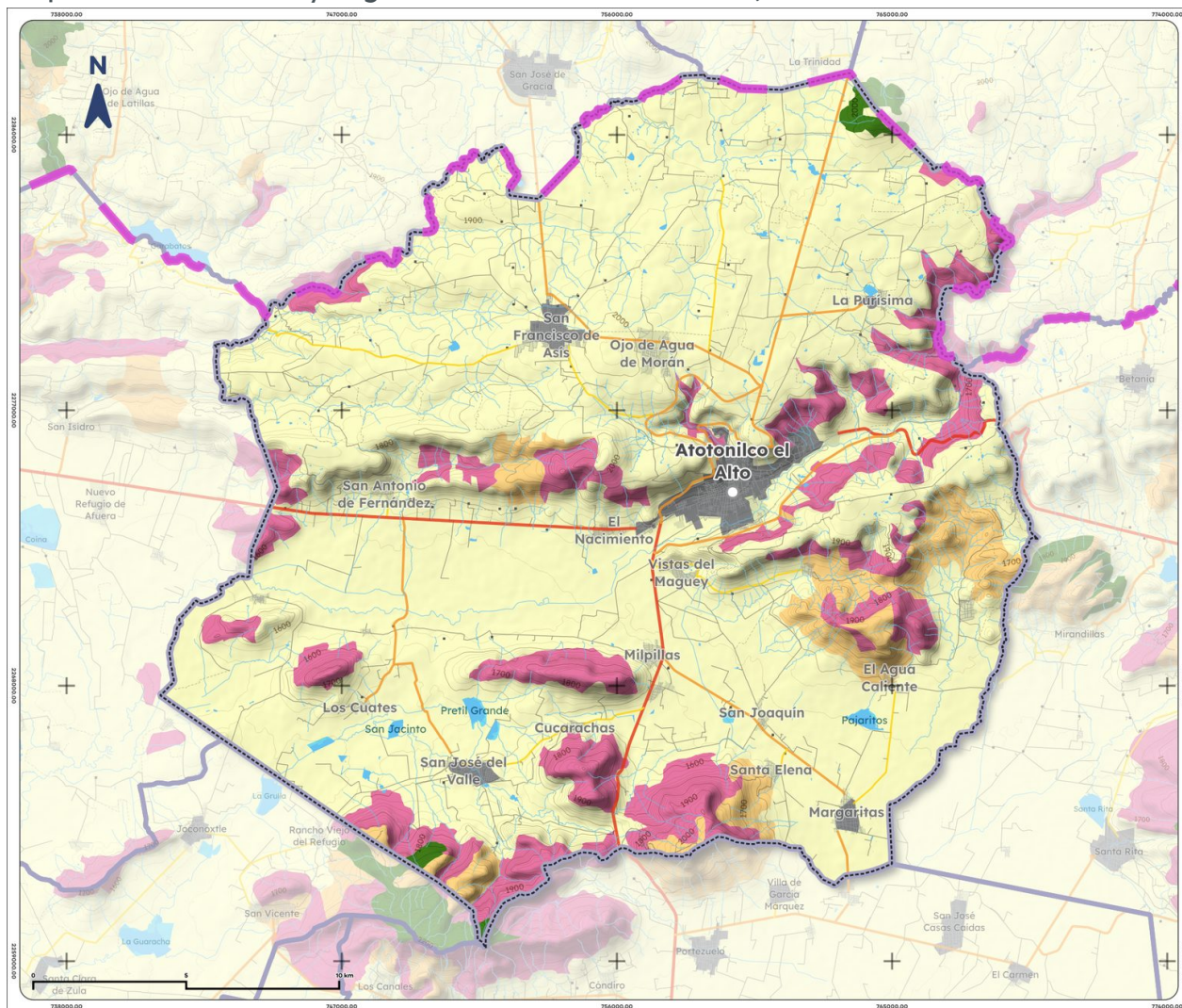
Mapa 11. Uso de suelo y vegetación de Atotonilco el Alto, 2018
