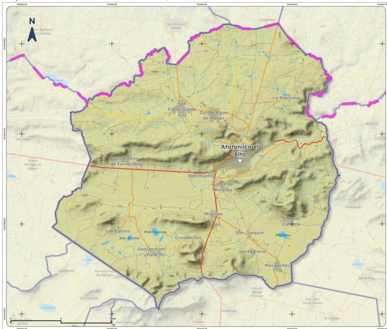
Mapa 6. Cuencas de Atotonilco el Alto, 2023
