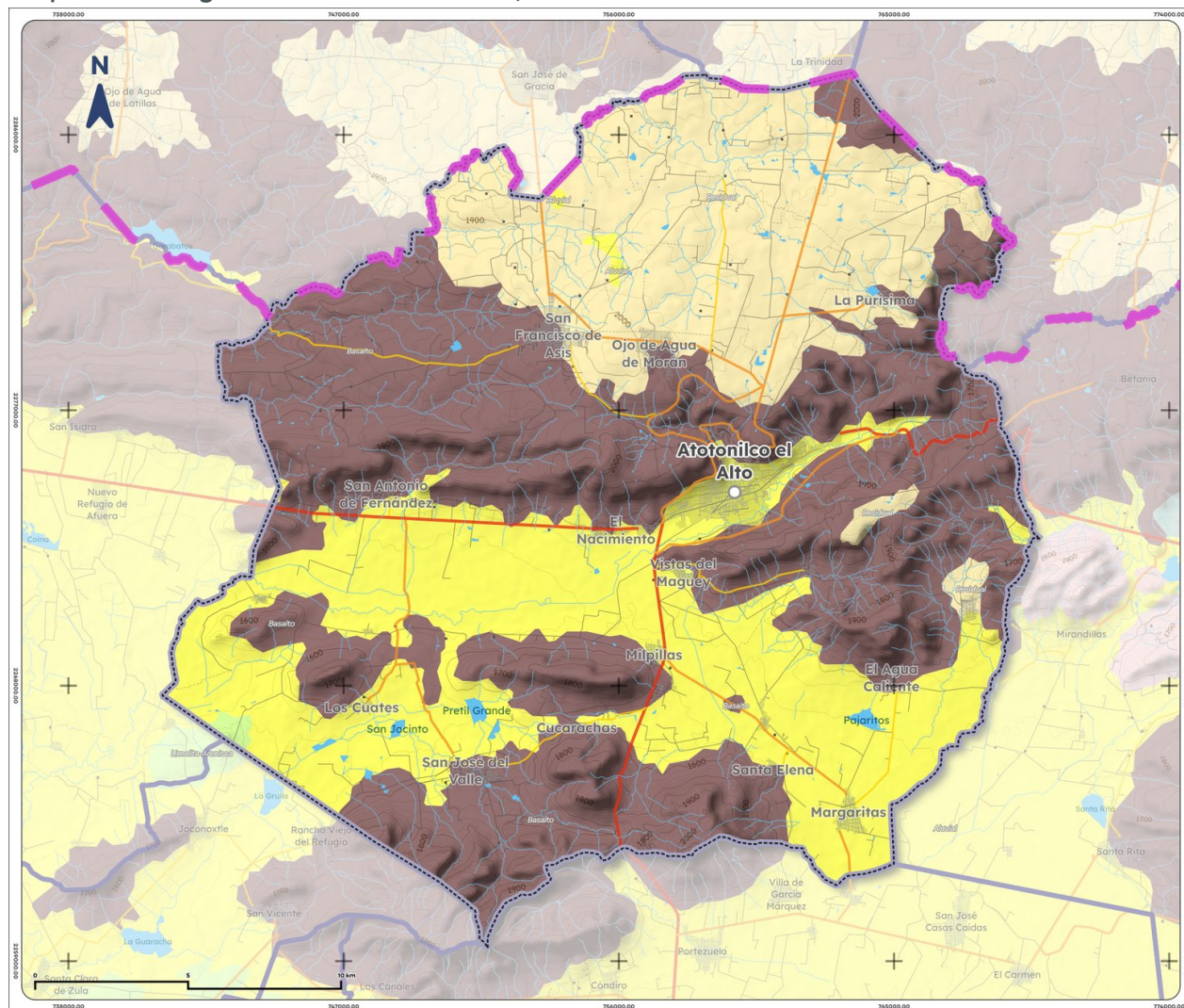
Mapa 3. Geología de Atotonilco el Alto, 1988
