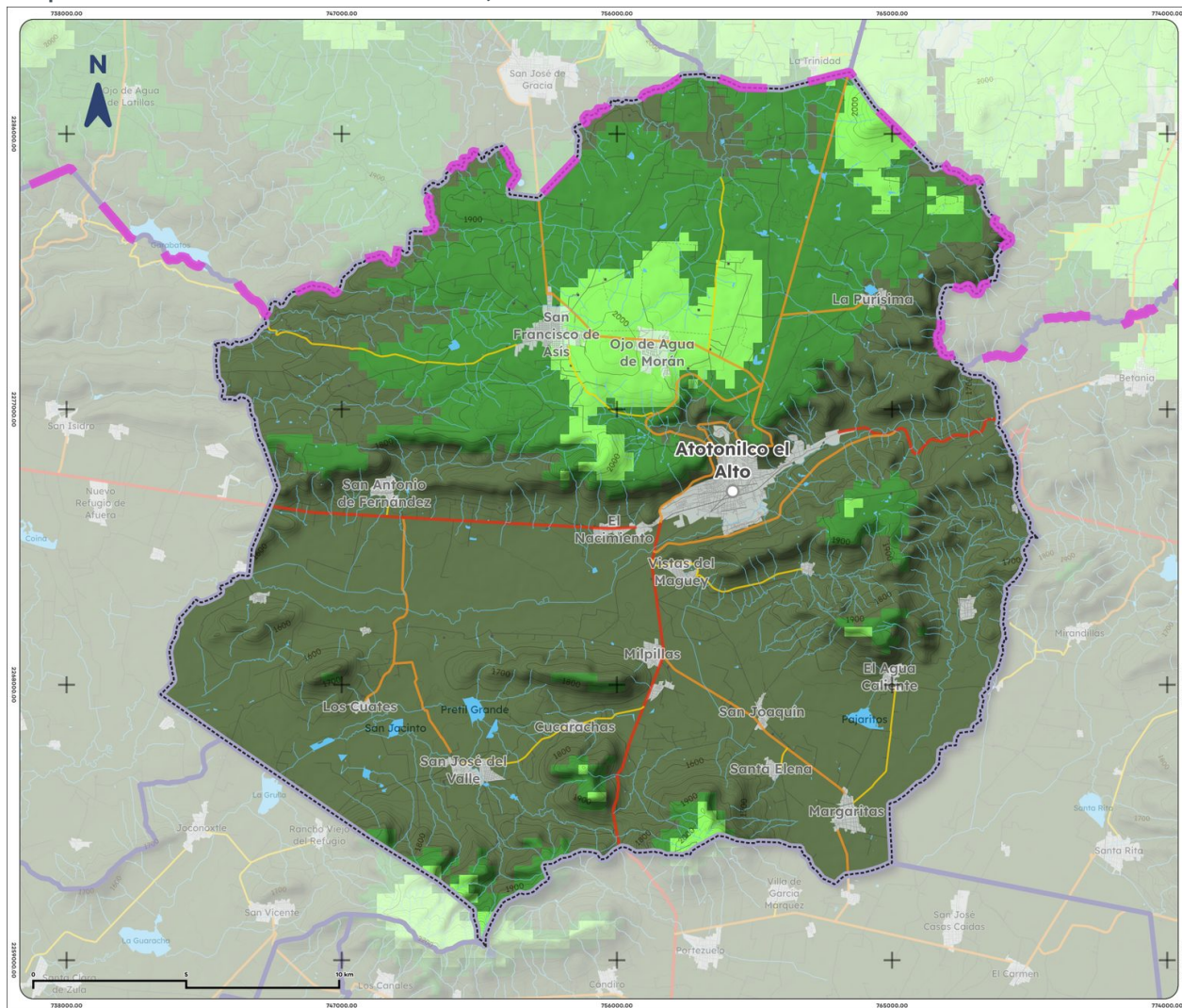
Mapa 10. Clima de Atotonilco el Alto, 1995-2025
