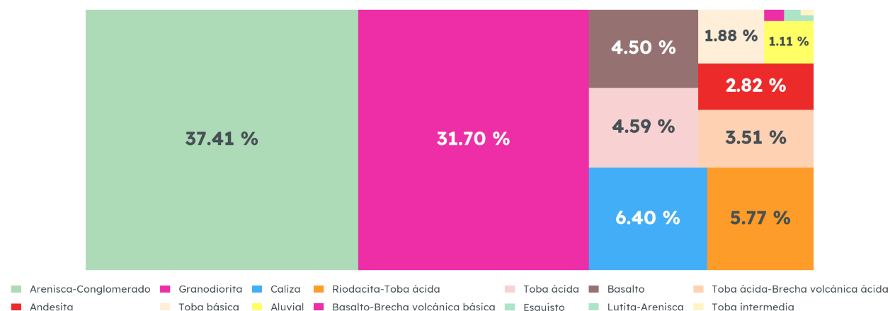
Geología de Zapotiltic, 1988
