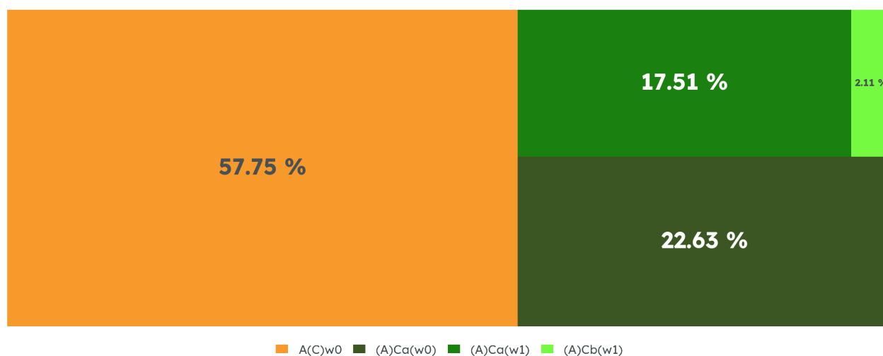
Clima de Zapotiltic, 1995-2025
