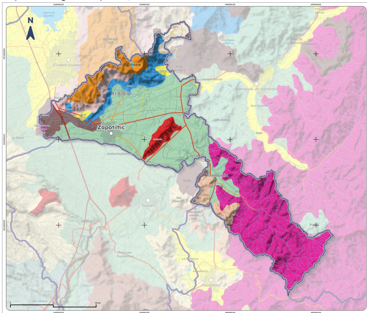
Mapa 3. Geología de Zapotiltic, 1988
