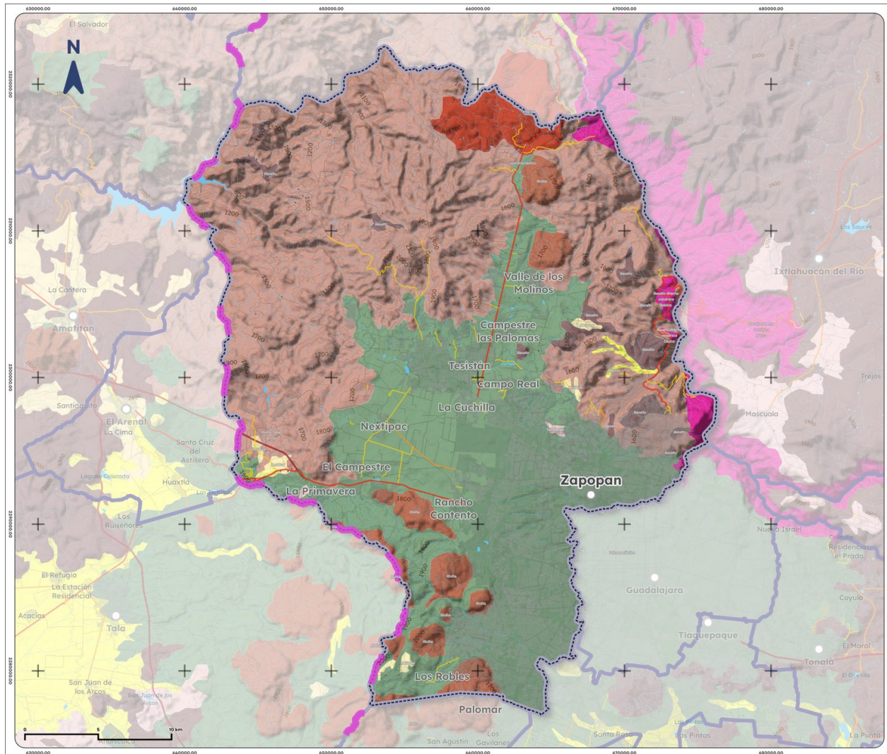
Mapa 3. Geología de Zapopan, 1988
