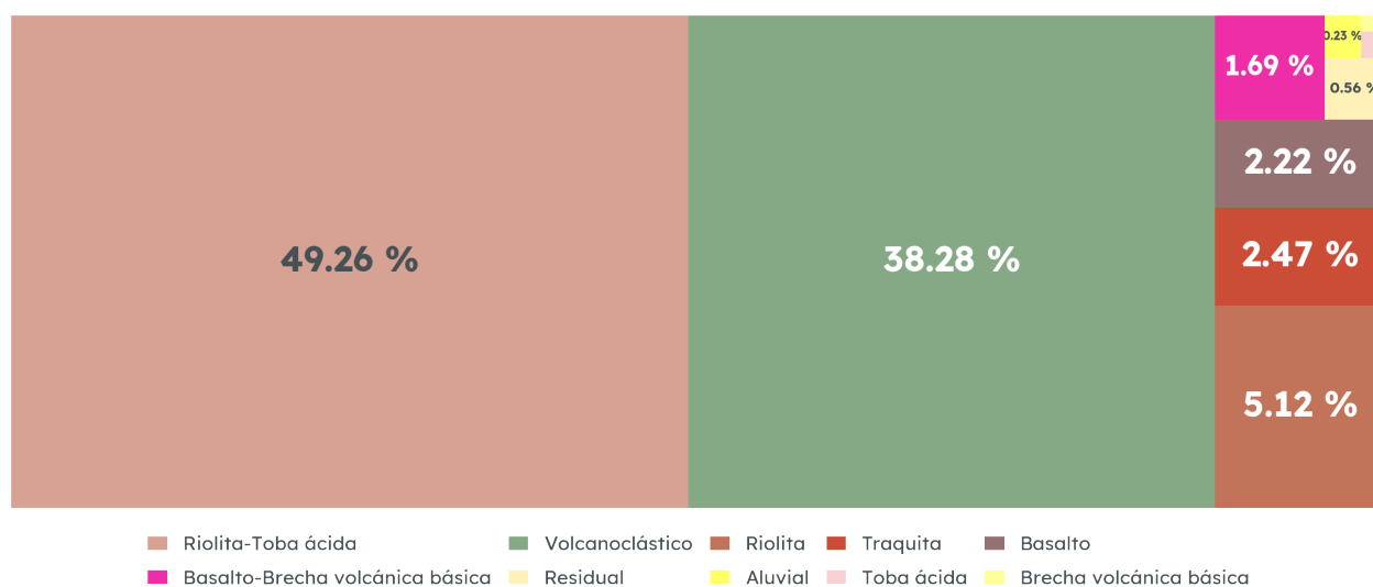
Geología de Zapopan, 1988
