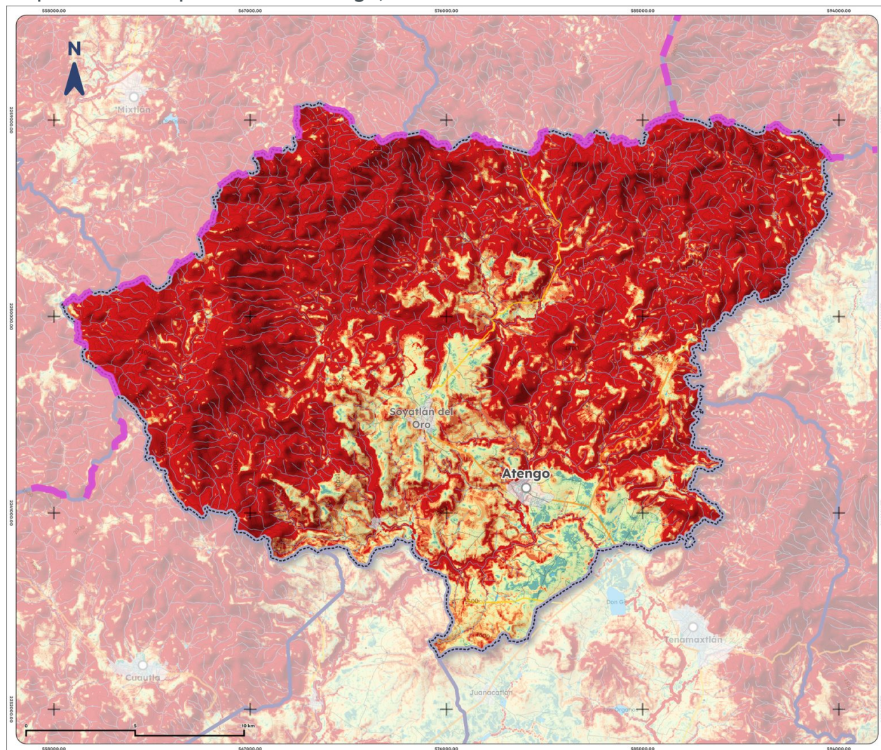
Mapa 16. Erosión potencial de Atengo, 2025
