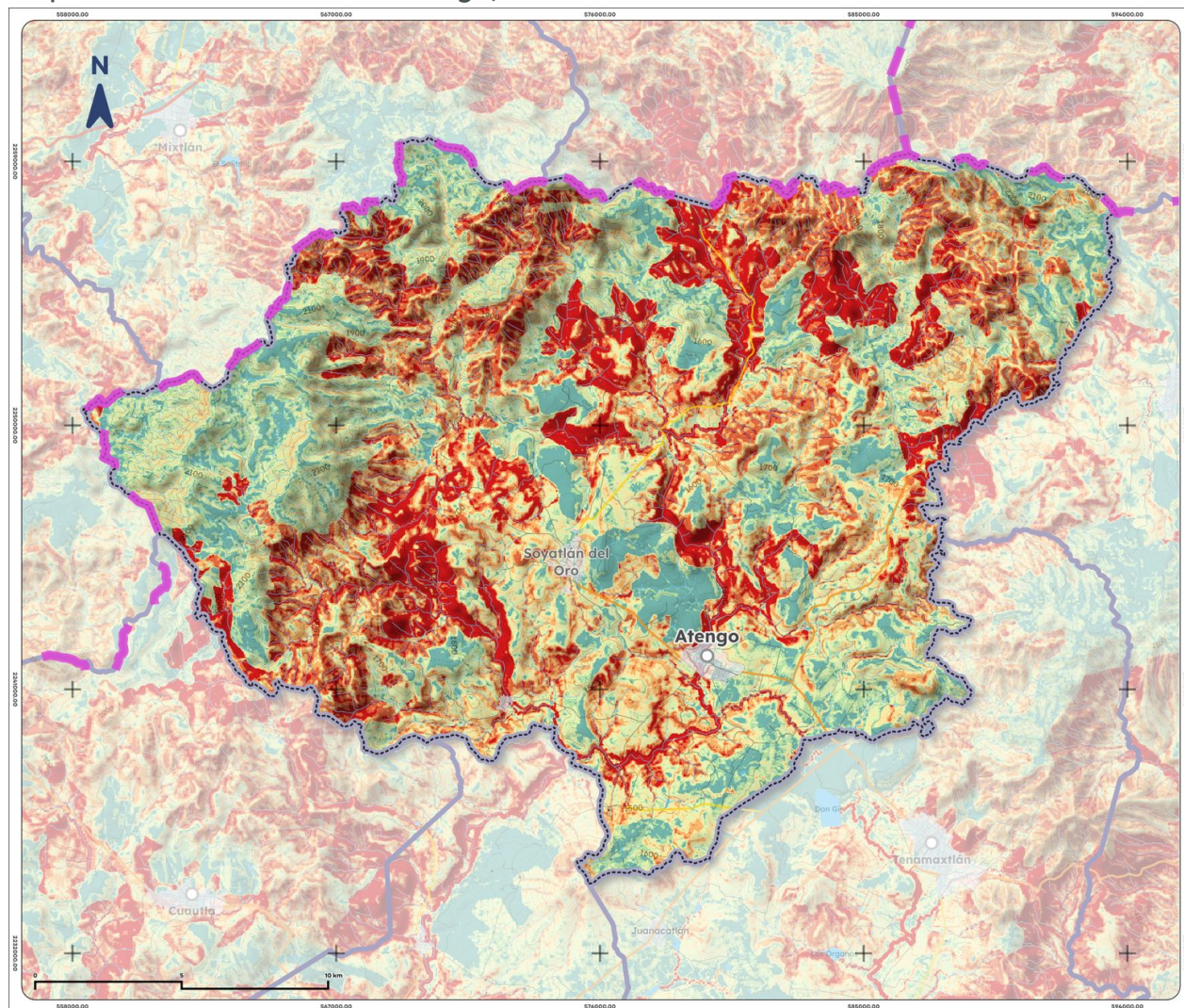
Mapa 17. Erosión efectiva de Atengo, 2025
