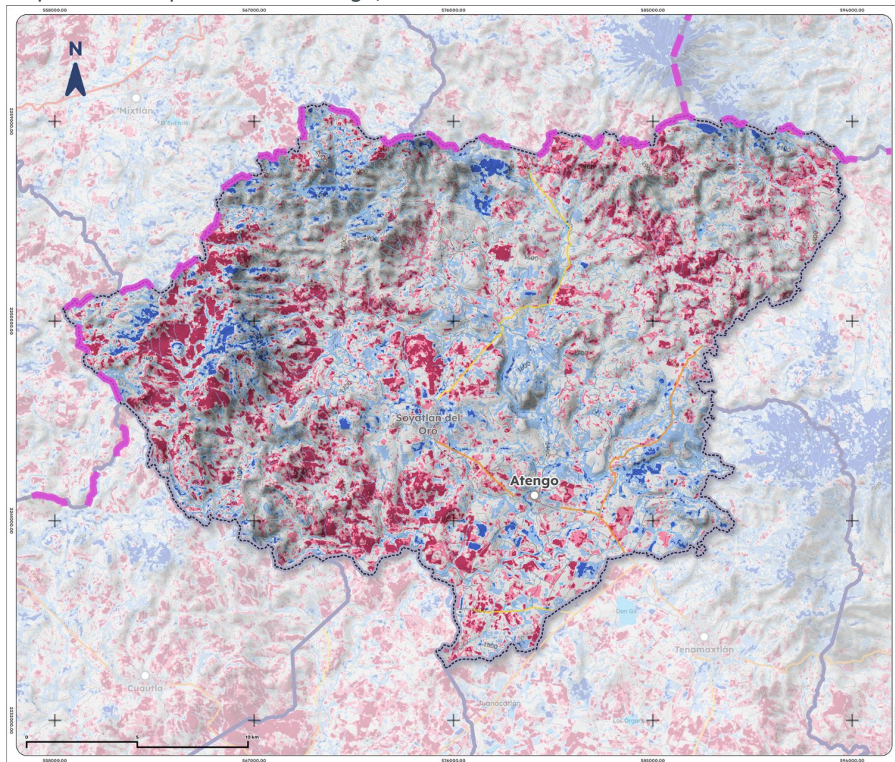
Mapa 13. NDWI promedio de Atengo, 2025
