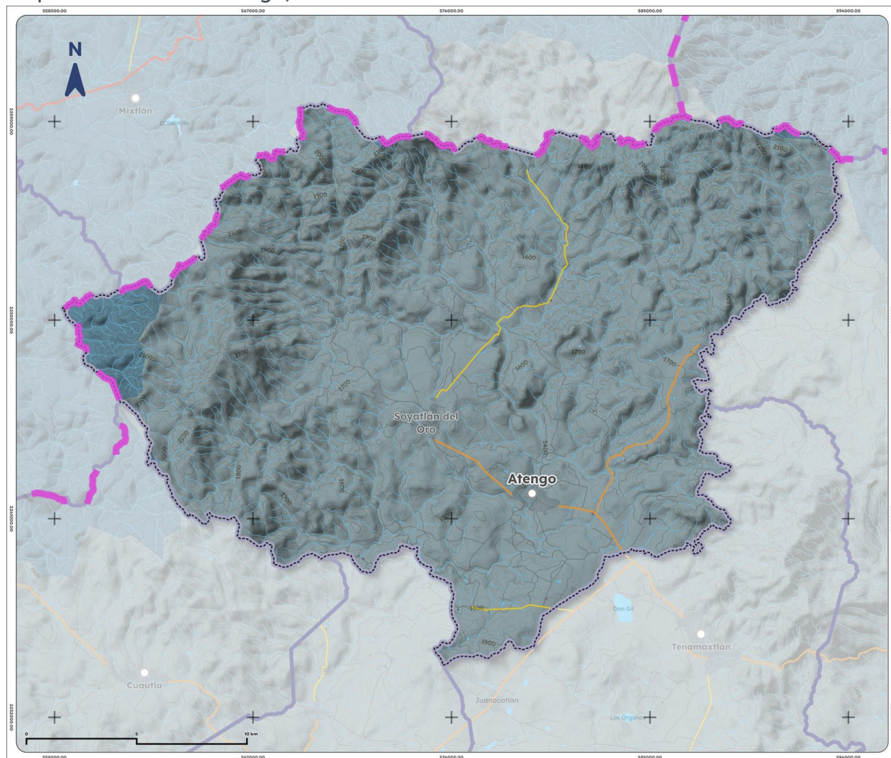
Mapa 6. Cuencas de Atengo, 2023
