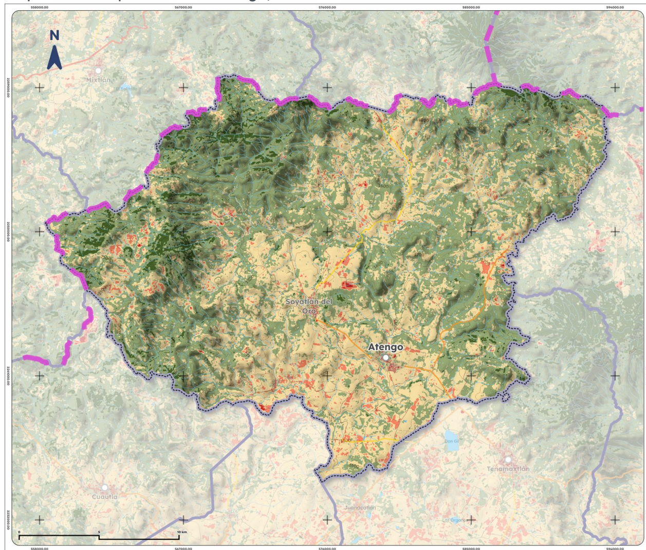
Mapa 12. NDVI promedio de Atengo, 2025
