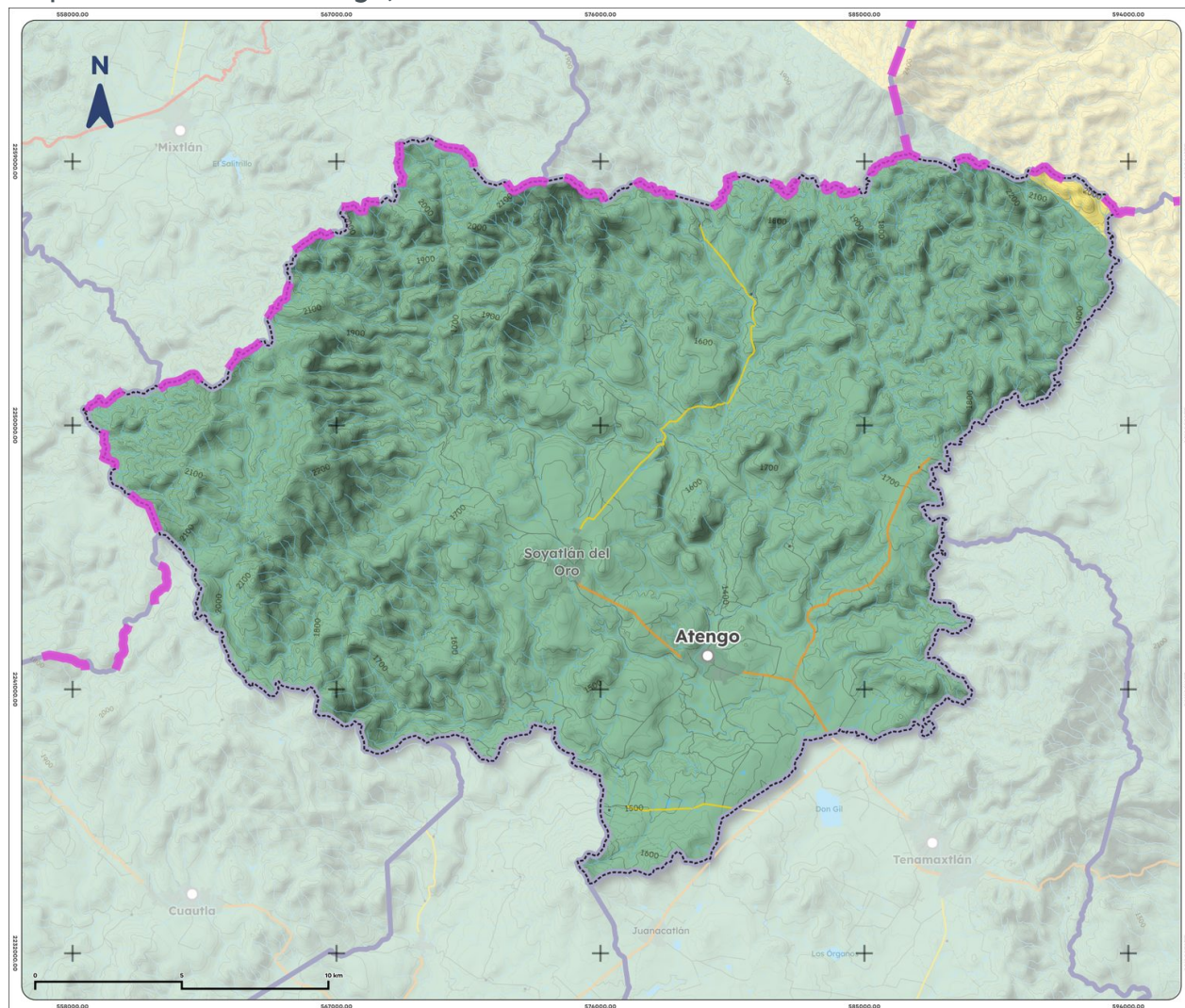
Mapa 7. Acuíferos de Atengo, 2023
