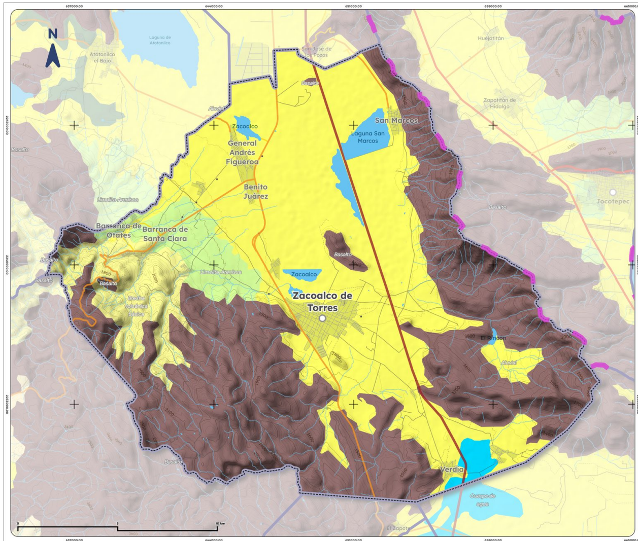
Mapa 3. Geología de Zacoalco de Torres, 1988
