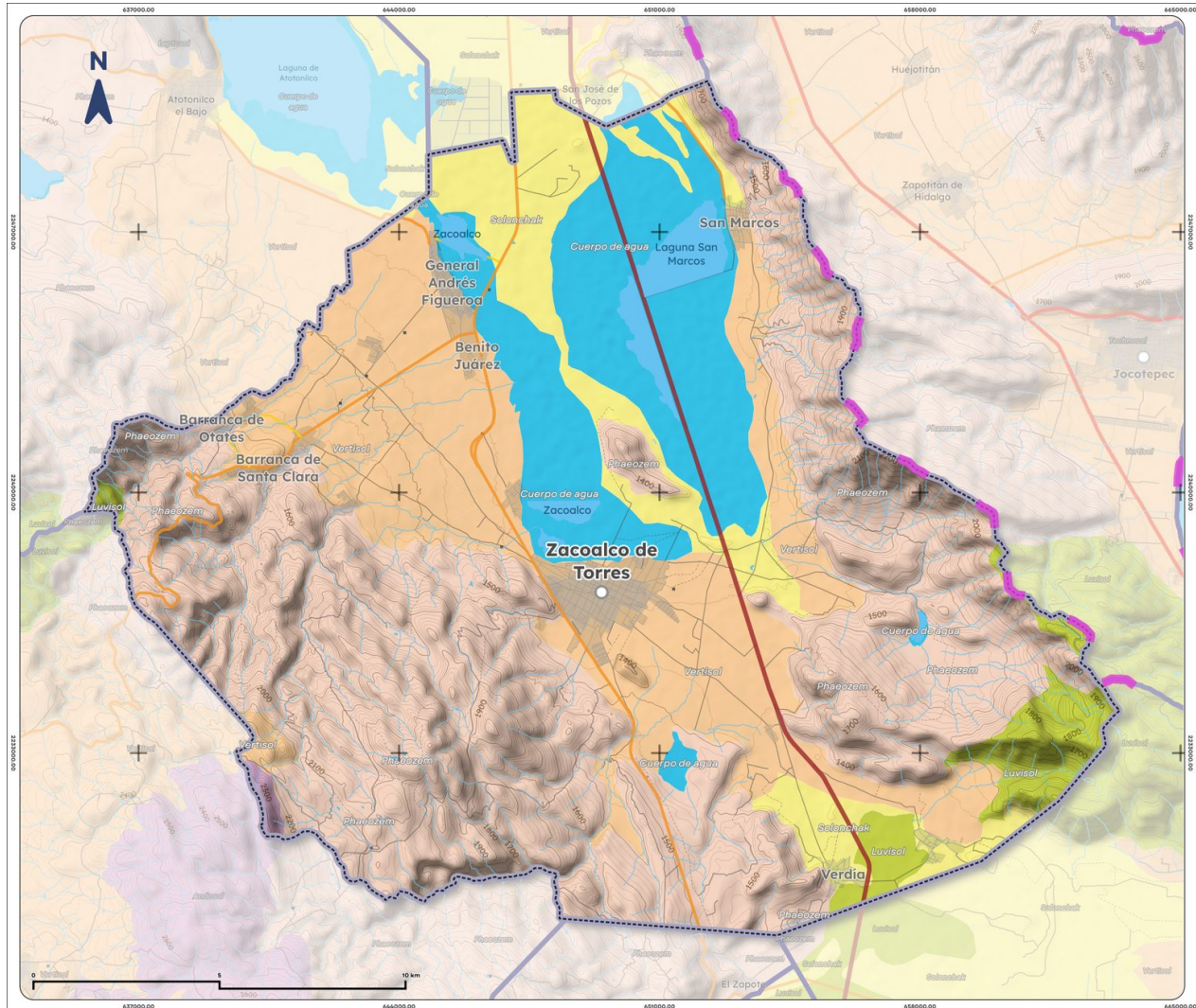
Mapa 4. Edafología de Zacoalco de Torres, 2025
