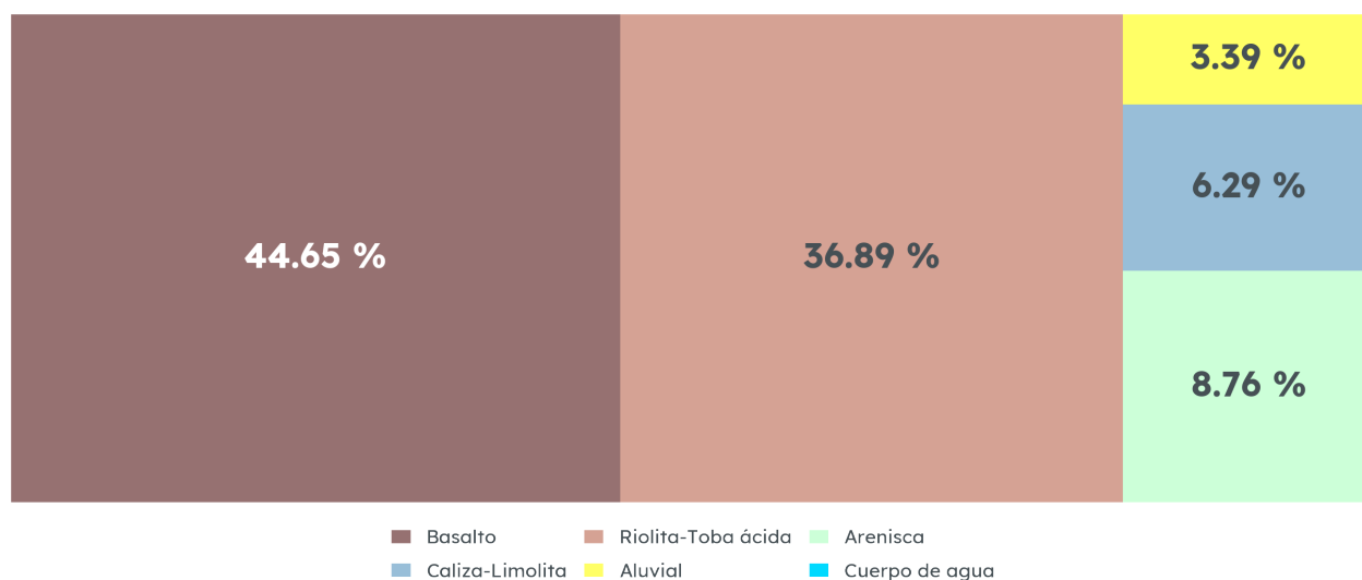
Geología de Yahualica de González Gallo, 1988
