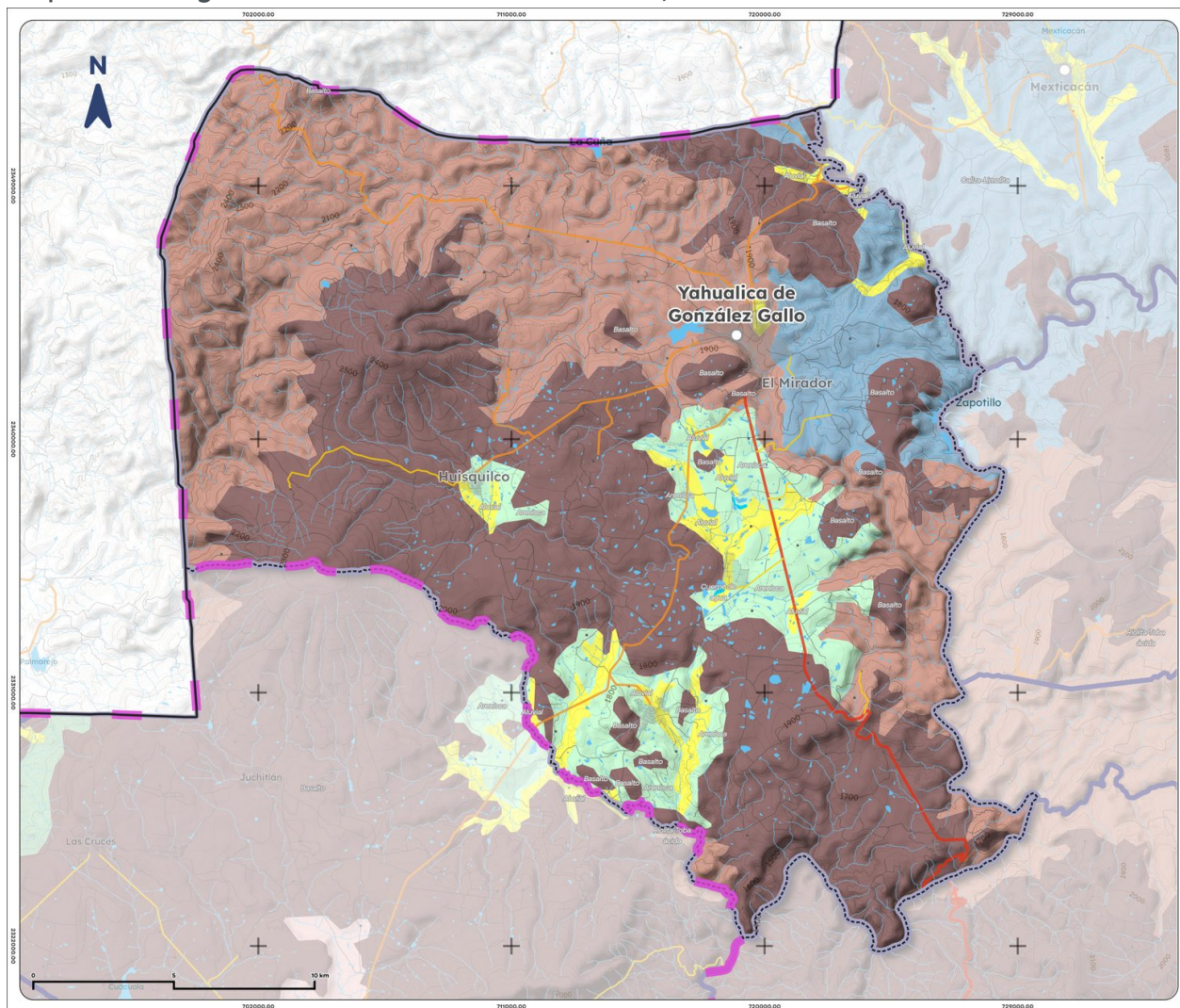
Mapa 3. Geología de Yahualica de González Gallo, 1988
