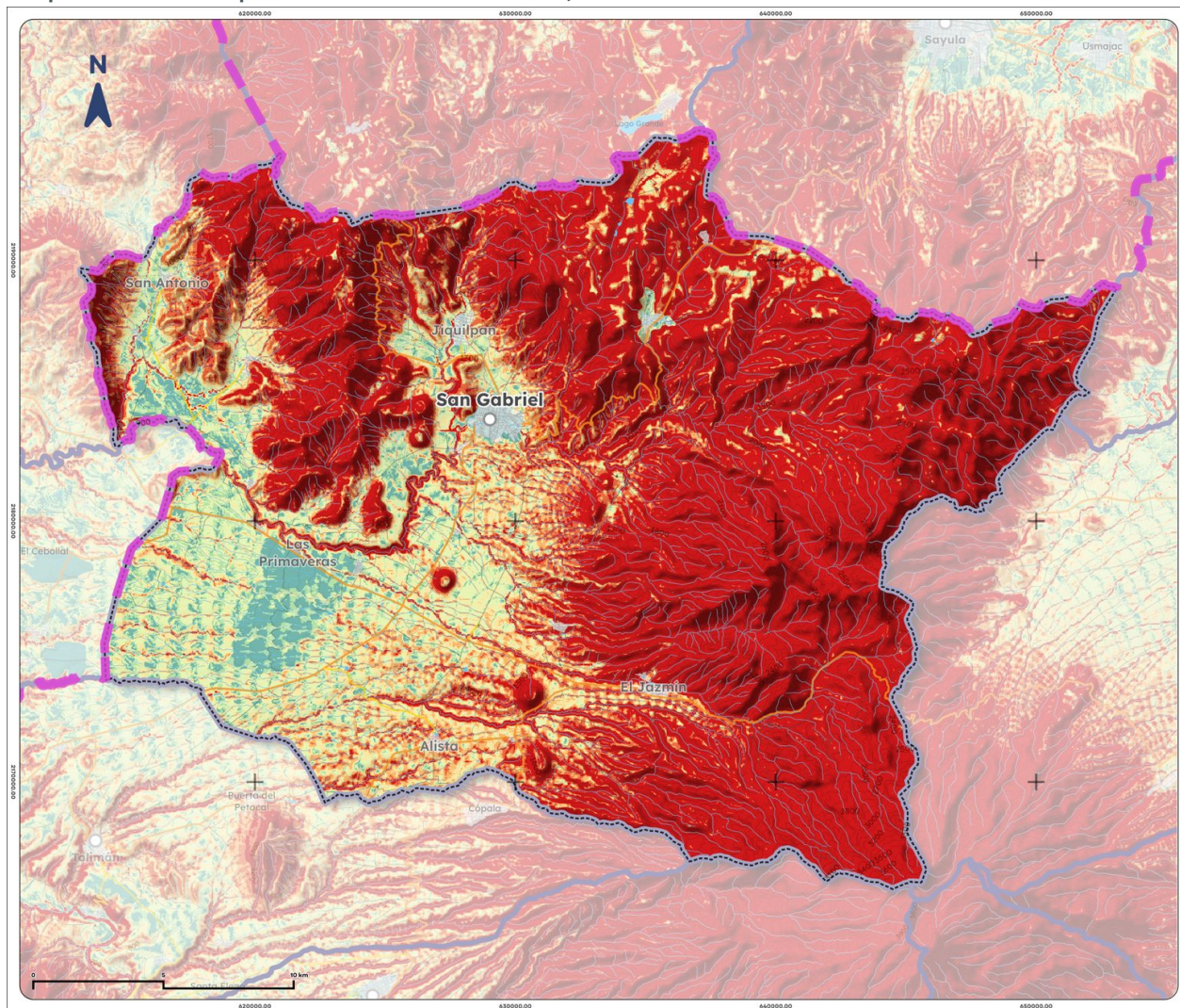
Mapa 16. Erosión potencial de San Gabriel, 2025
