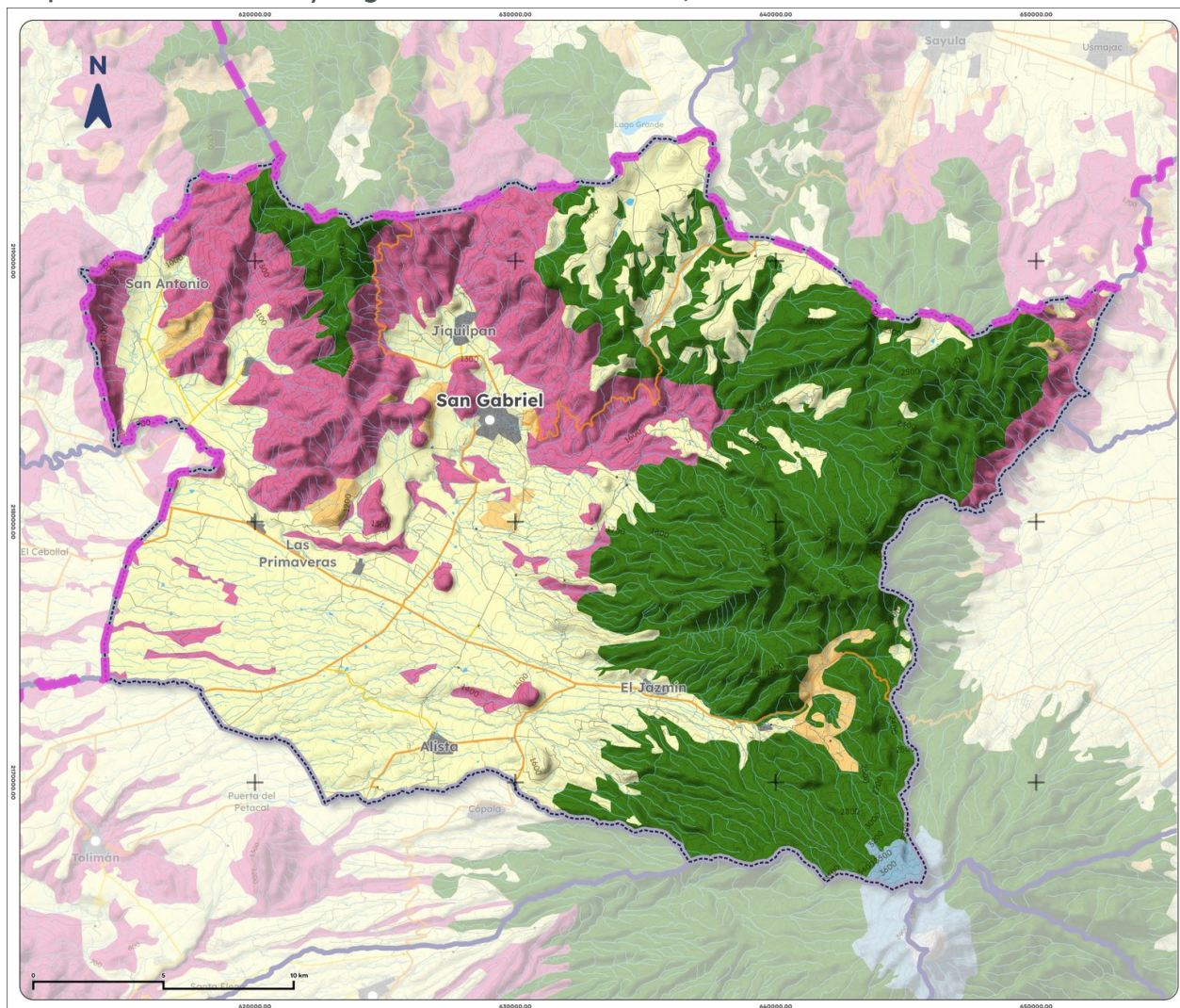
Mapa 11. Uso de suelo y vegetación de San Gabriel, 2018
