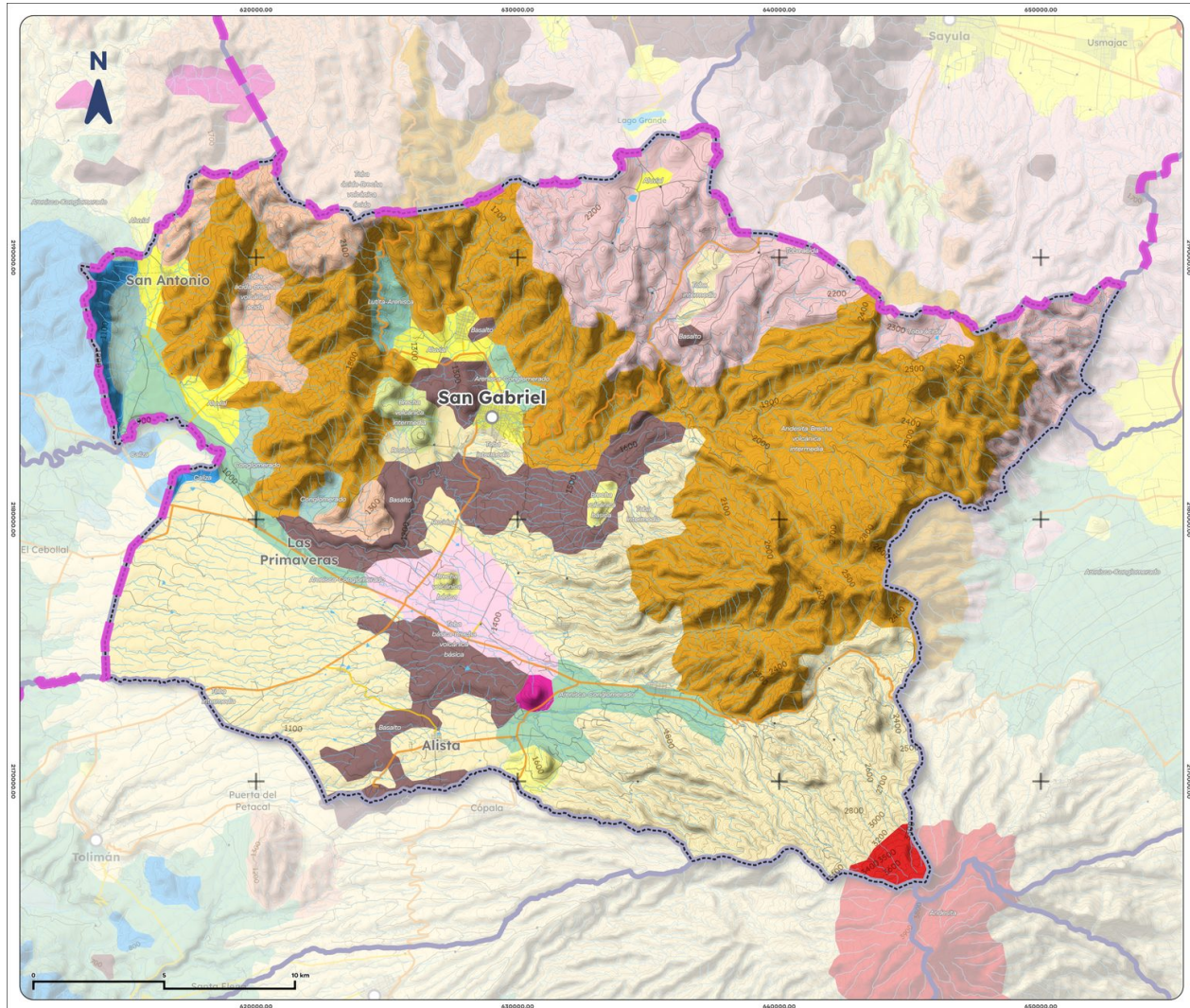
Mapa 3. Geología de San Gabriel, 1988
