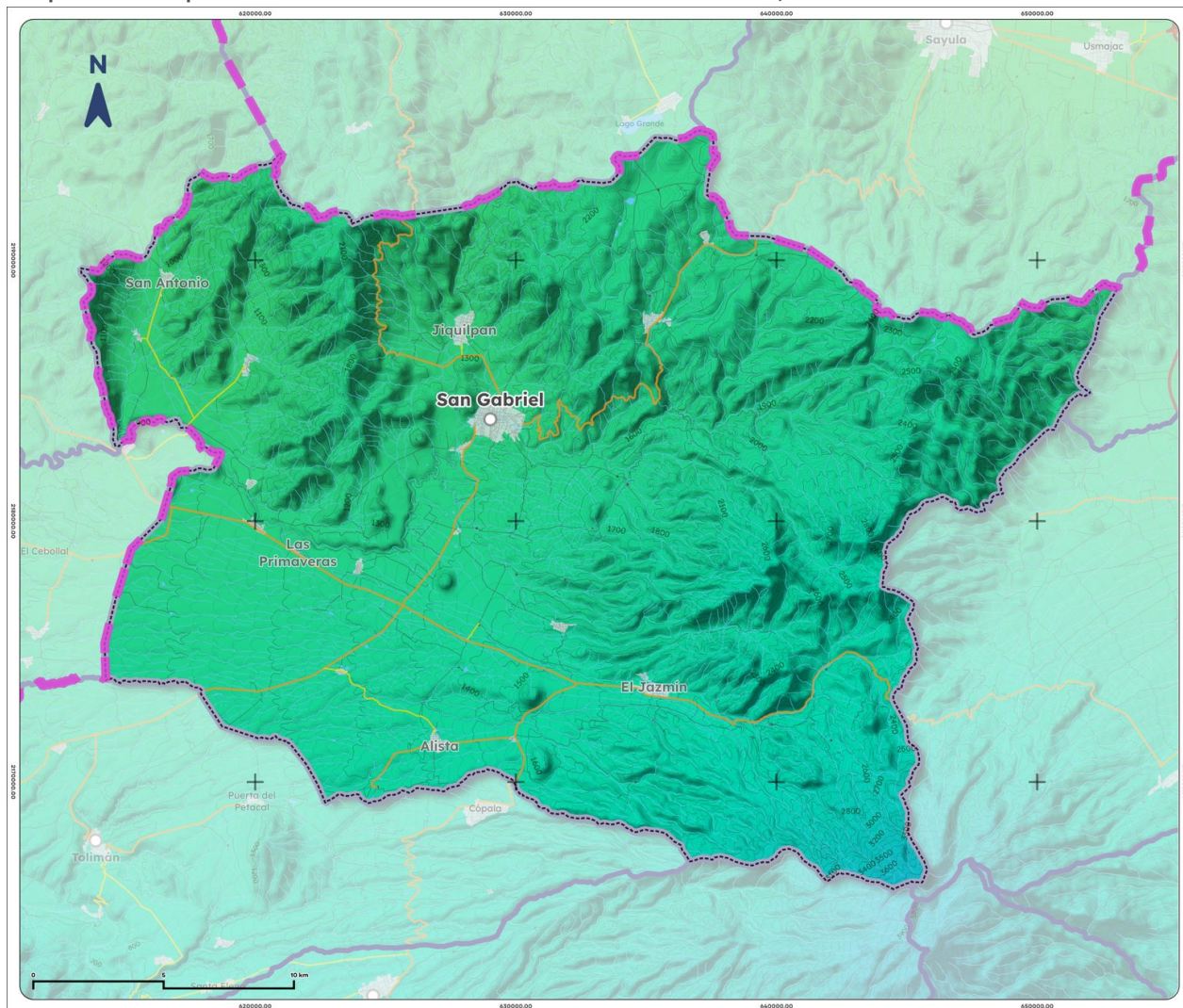
Mapa 9. Precipitación histórica acumulada de San Gabriel, 1995-2025
