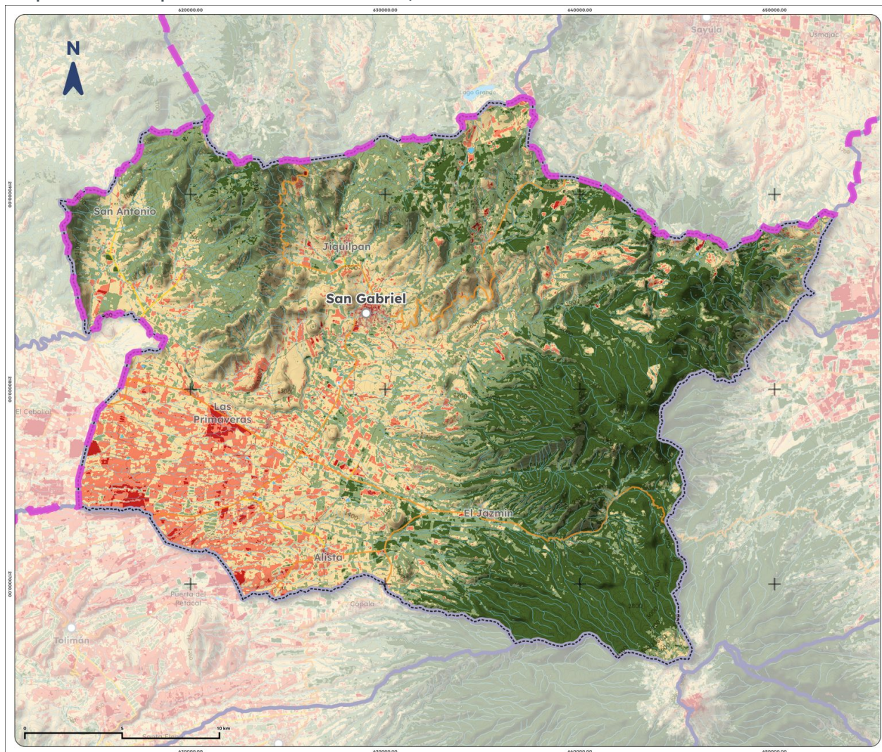
Mapa 12. NDVI promedio de San Gabriel, 2025
