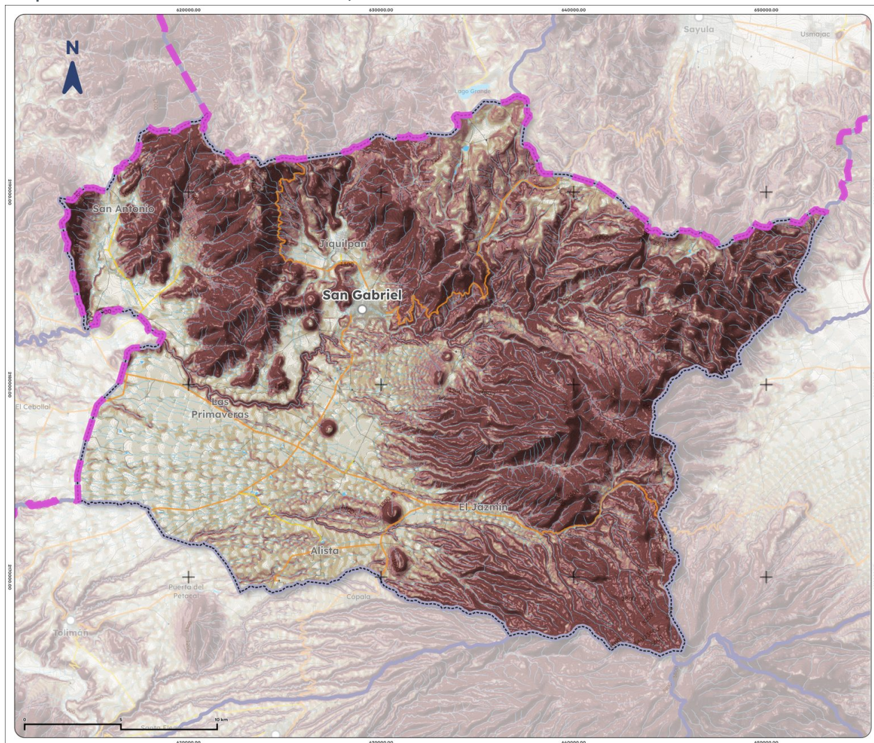
Mapa 5. Pendientes de San Gabriel, 2025
