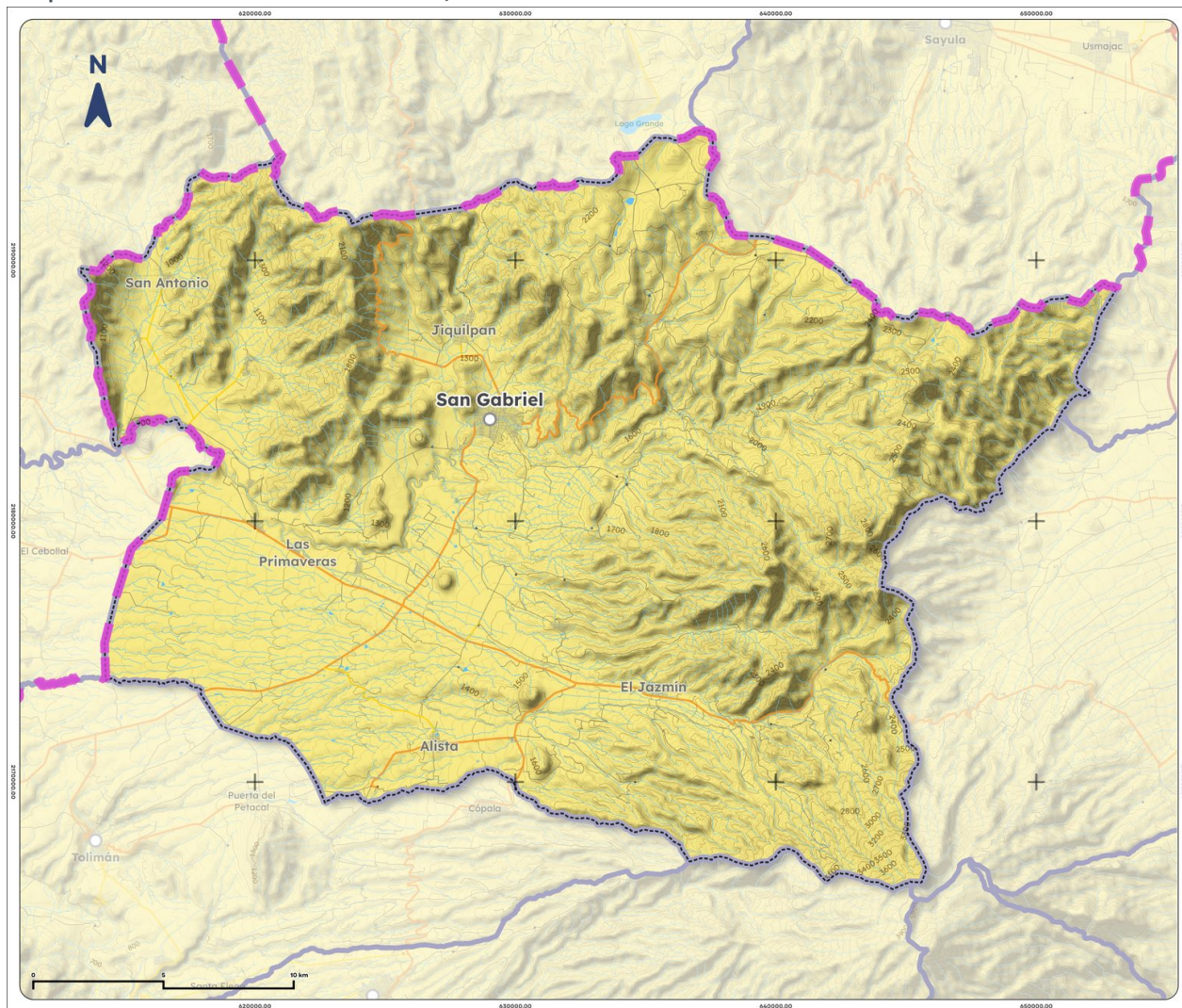
Mapa 7. Acuíferos de San Gabriel, 2023
