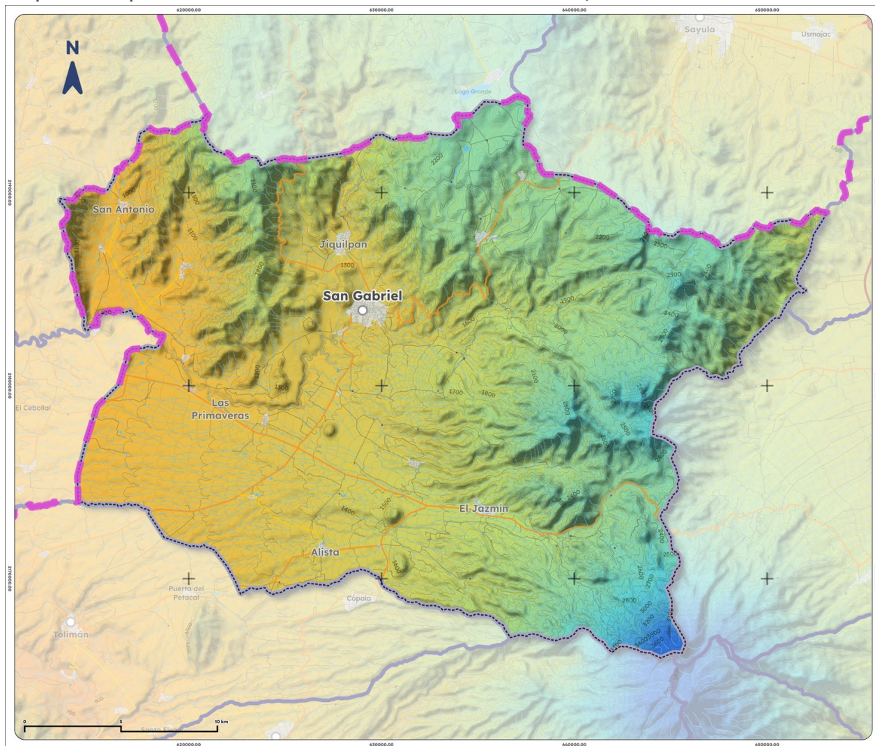
Mapa 8. Temperatura media anual histórica de San Gabriel, 1995-2025
