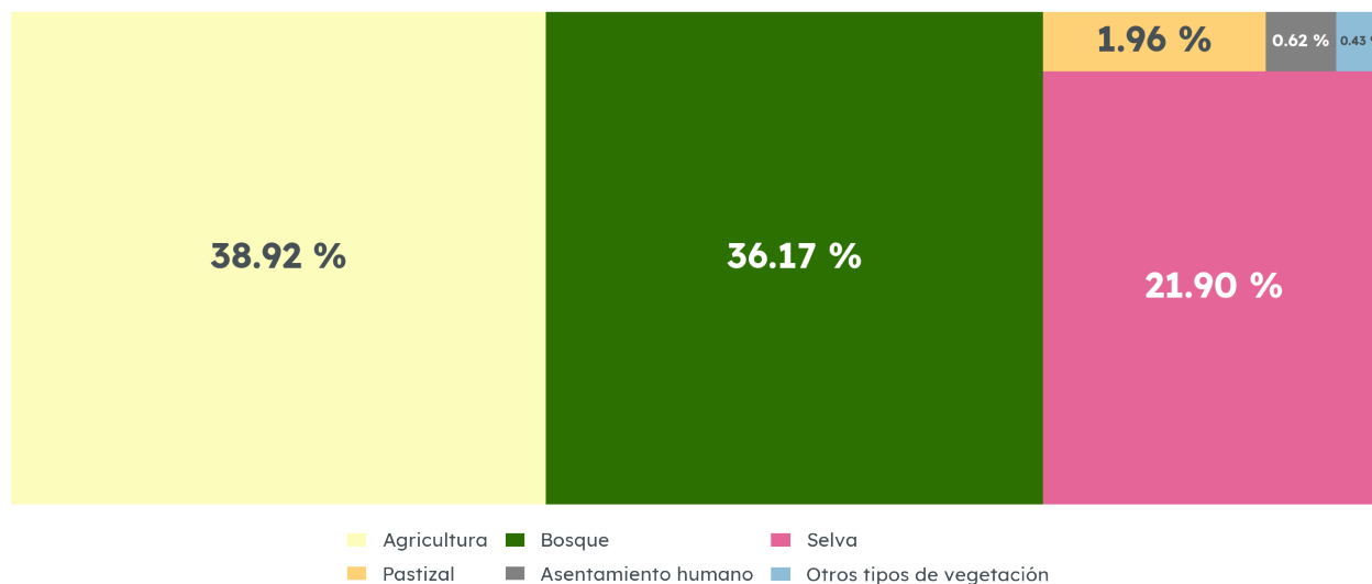
Uso de suelo y vegetación de San Gabriel, 2018
