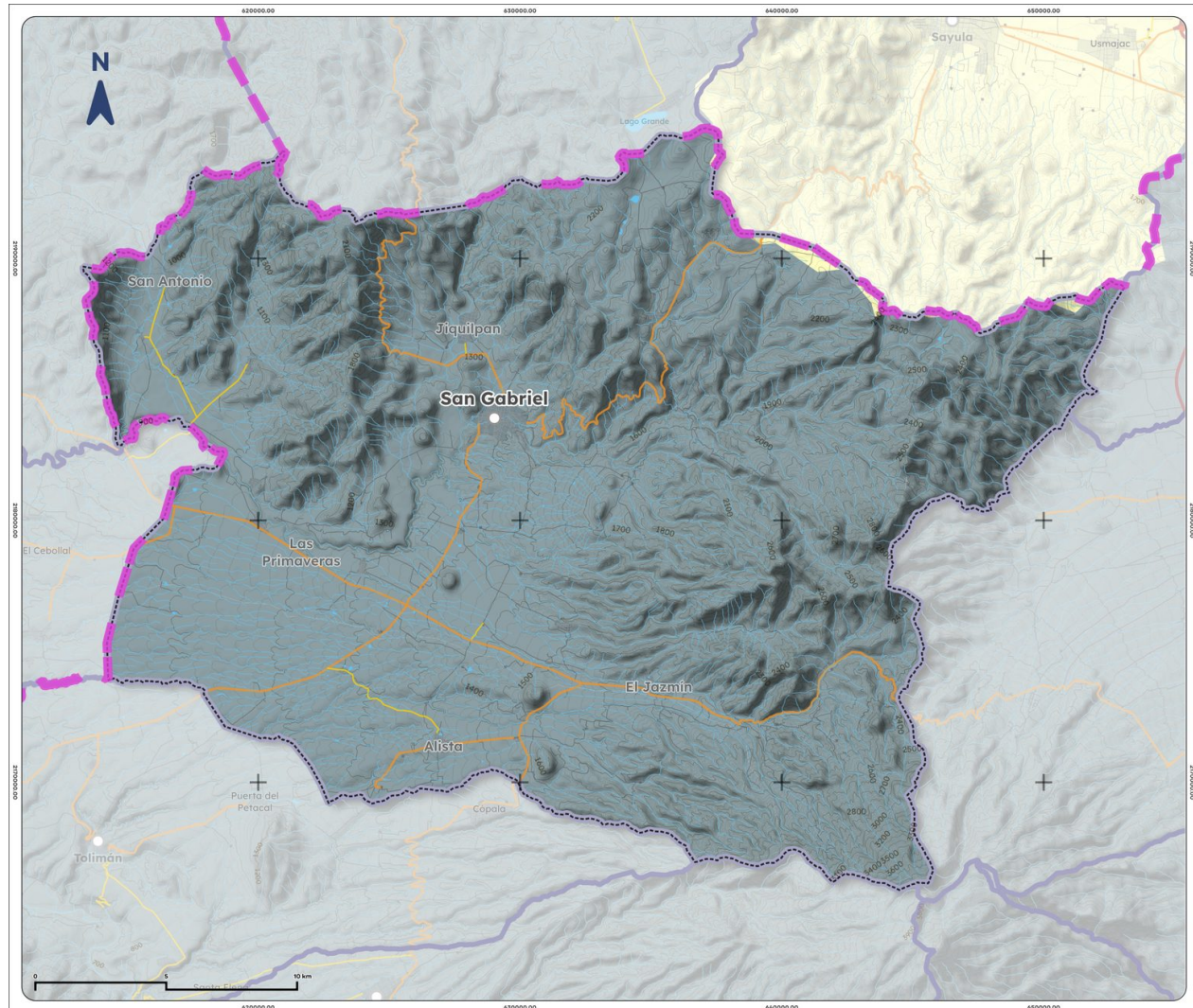
Mapa 6. Cuencas de San Gabriel, 2023
