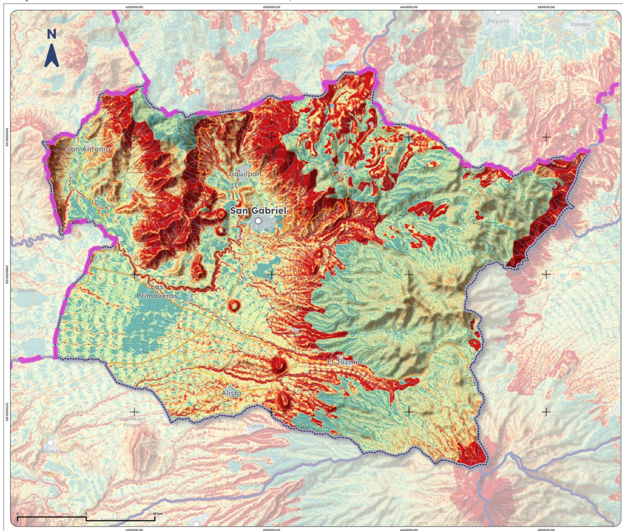
Mapa 17. Erosión efectiva de San Gabriel, 2025
