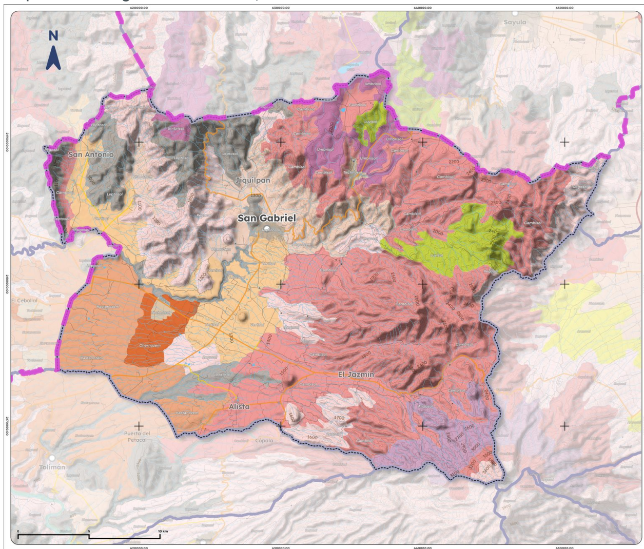
Mapa 4. Edafología de San Gabriel, 2025
