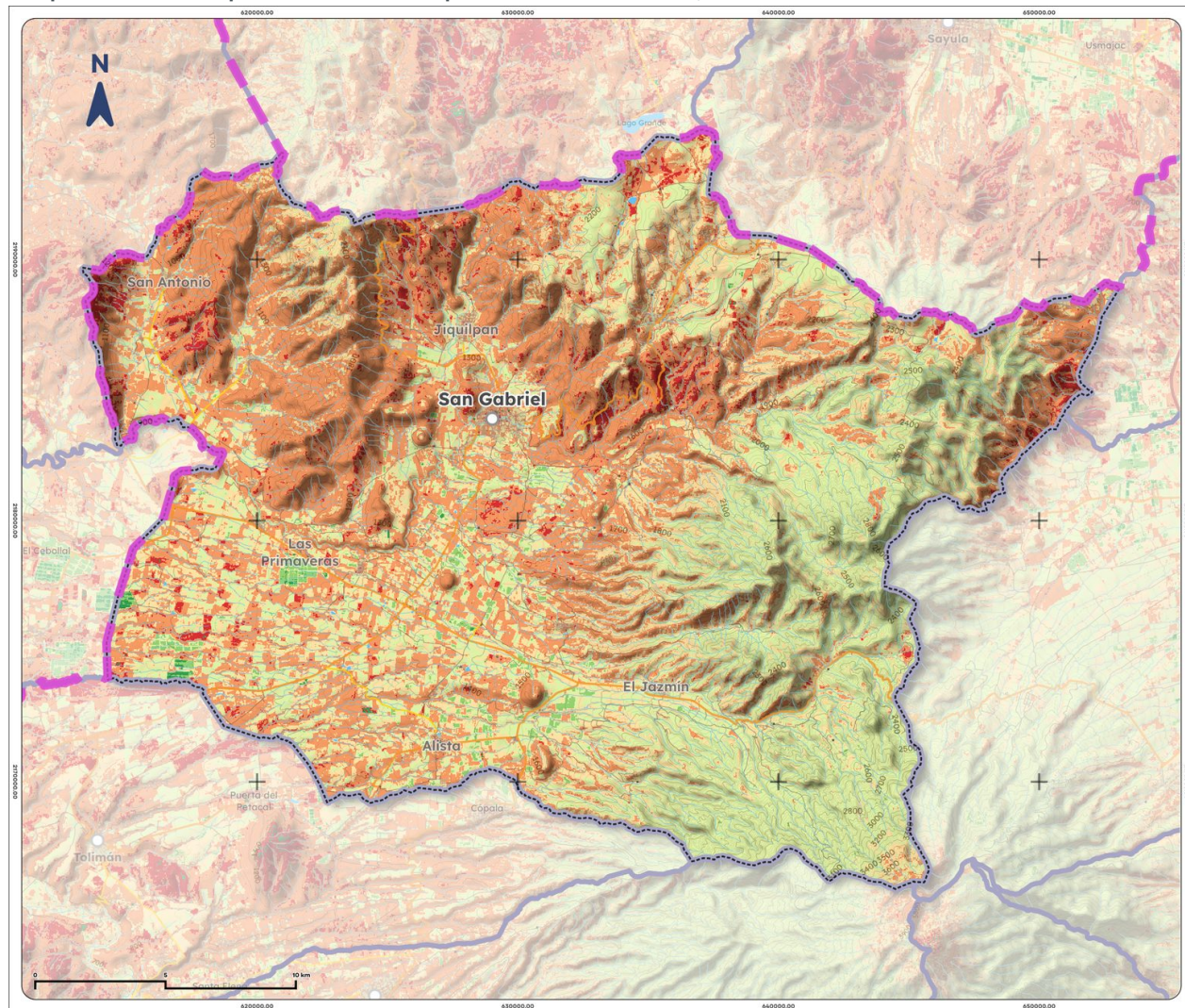
Mapa 15. Índice promedio de sequía de San Gabriel, 2025
