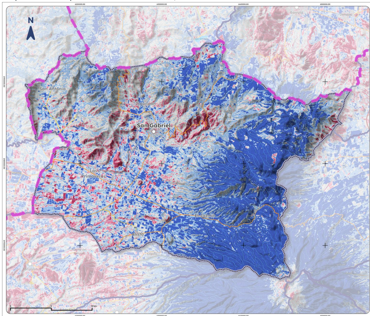
Mapa 13. NDWI promedio de San Gabriel, 2025
