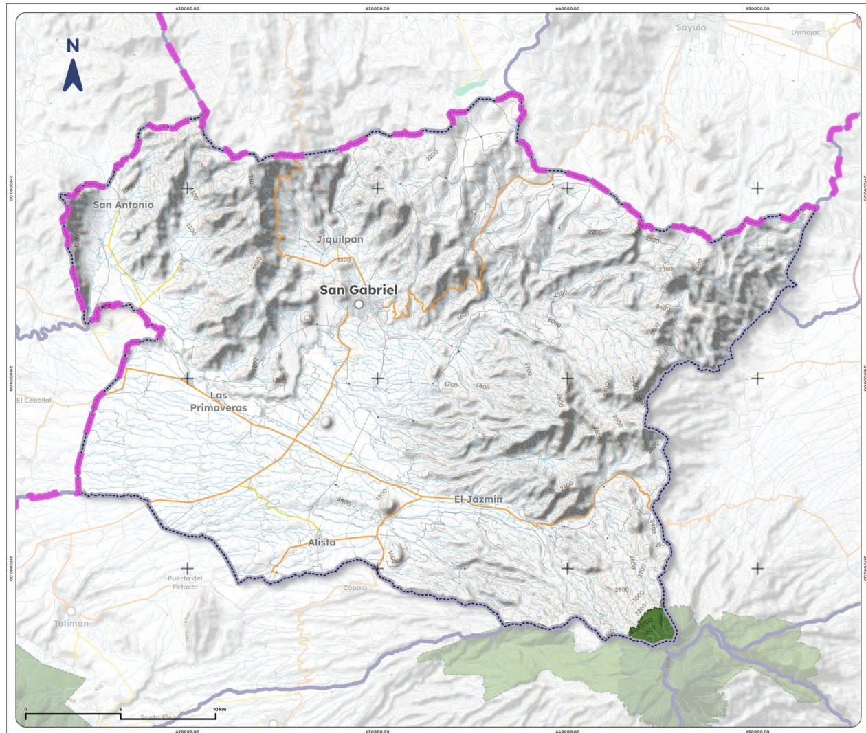
Mapa 14. Áreas naturales protegidas y humedales de San Gabriel, 2025
