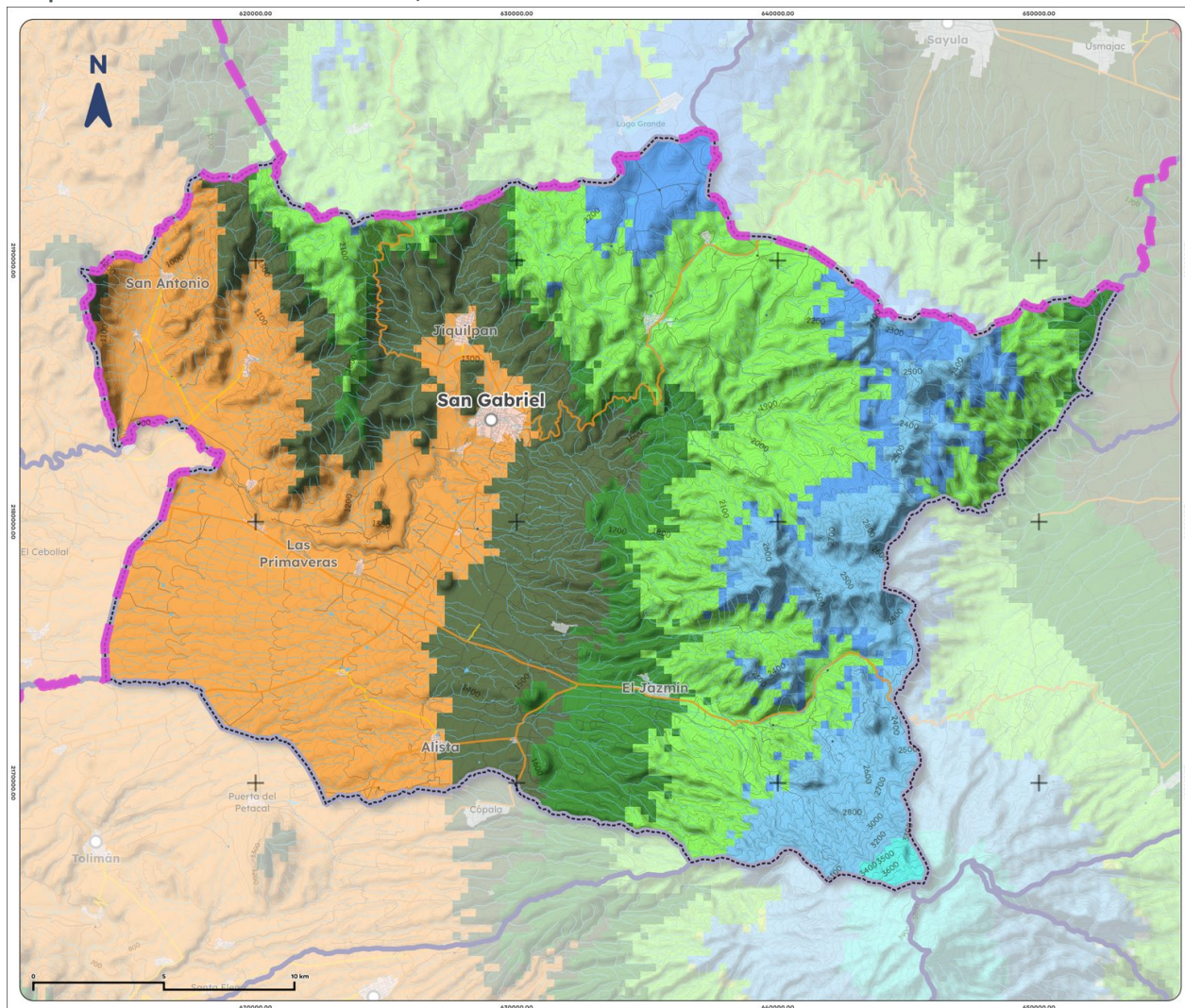
Mapa 10. Clima de San Gabriel, 1995-2025
