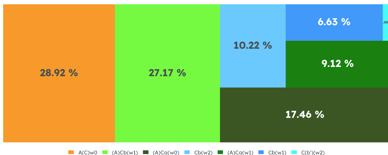
Clima de San Gabriel, 1995-2025
