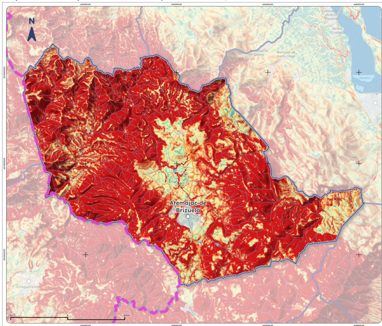
Mapa 16. Erosión potencial de Atemajac de Brizuela, 2025
