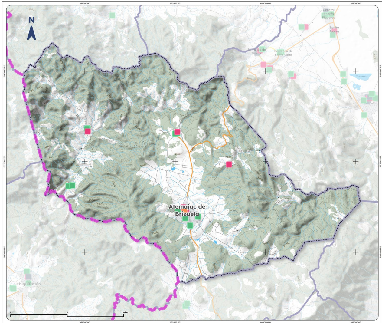
Mapa 21. Espacios públicos de Atemajac de Brizuela, 2025
