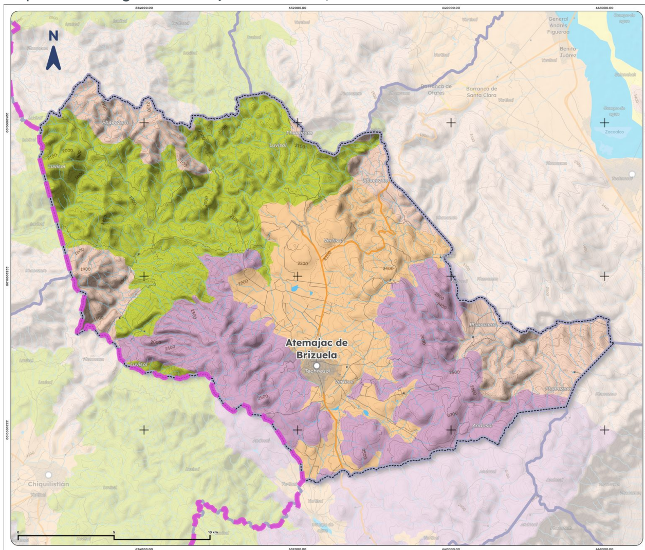
Mapa 4. Edafología de Atemajac de Brizuela, 2025
