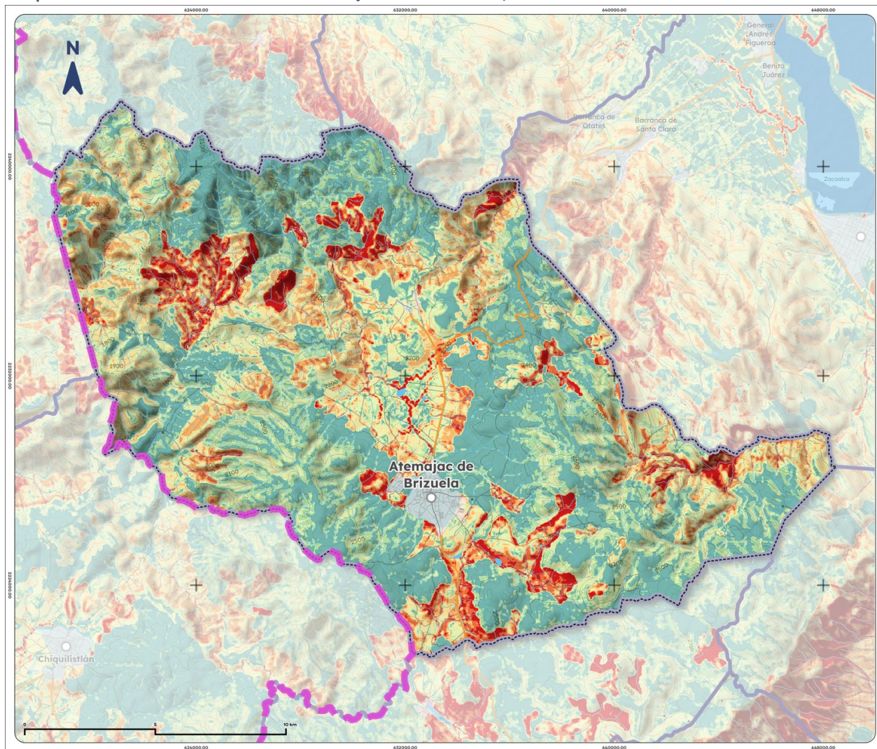
Mapa 17. Erosión efectiva de Atemajac de Brizuela, 2025
