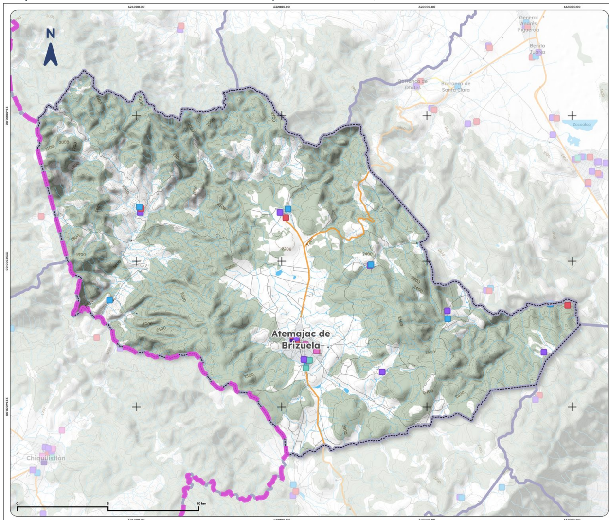
Mapa 20. Centros educativos de Atemajac de Brizuela, 2025
