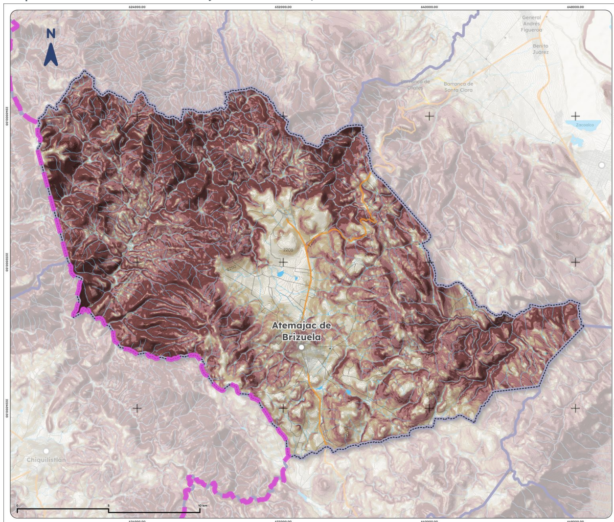
Mapa 5. Pendientes de Atemajac de Brizuela, 2025
