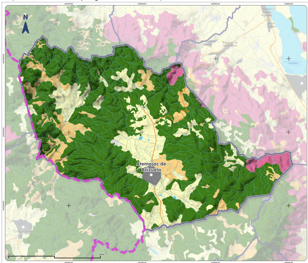
Mapa 11. Uso de suelo y vegetación de Atemajac de Brizuela, 2018
