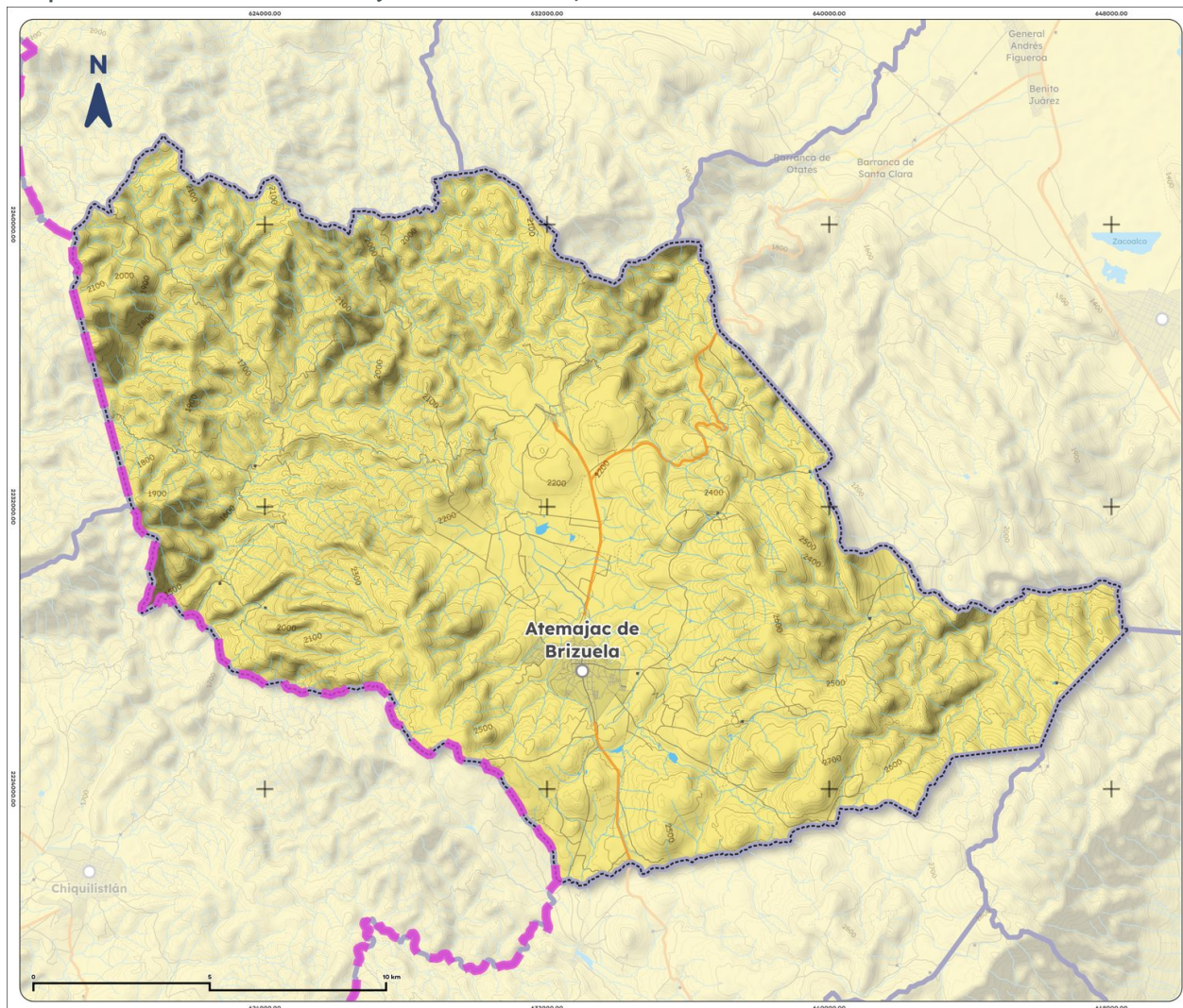
Mapa 7. Acuíferos de Atemajac de Brizuela, 2023
