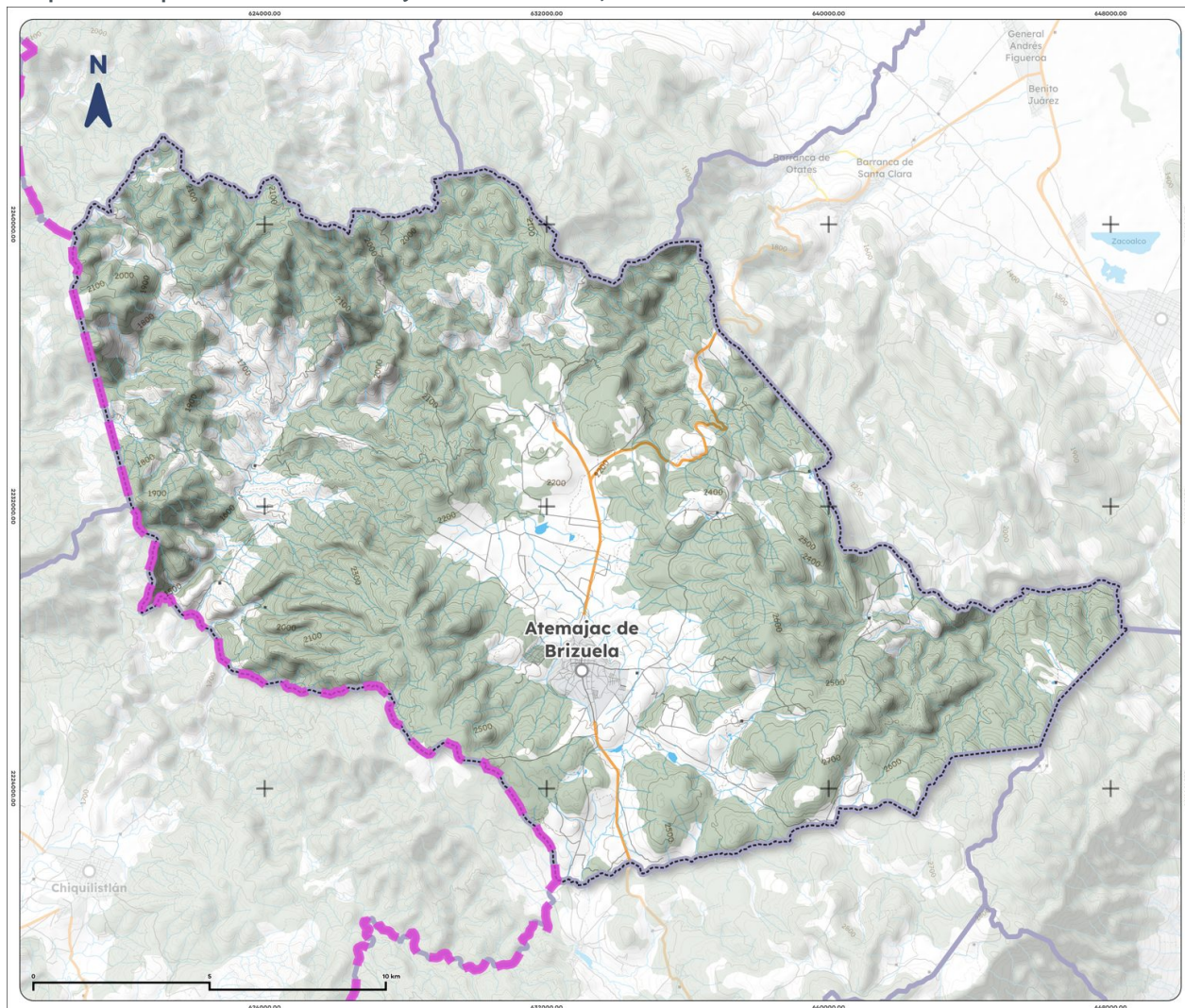
Mapa 2. Mapa base de Atemajac de Brizuela, 2025
