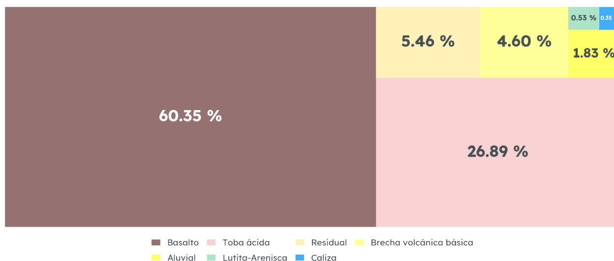
Geología de Atemajac de Brizuela, 1988
