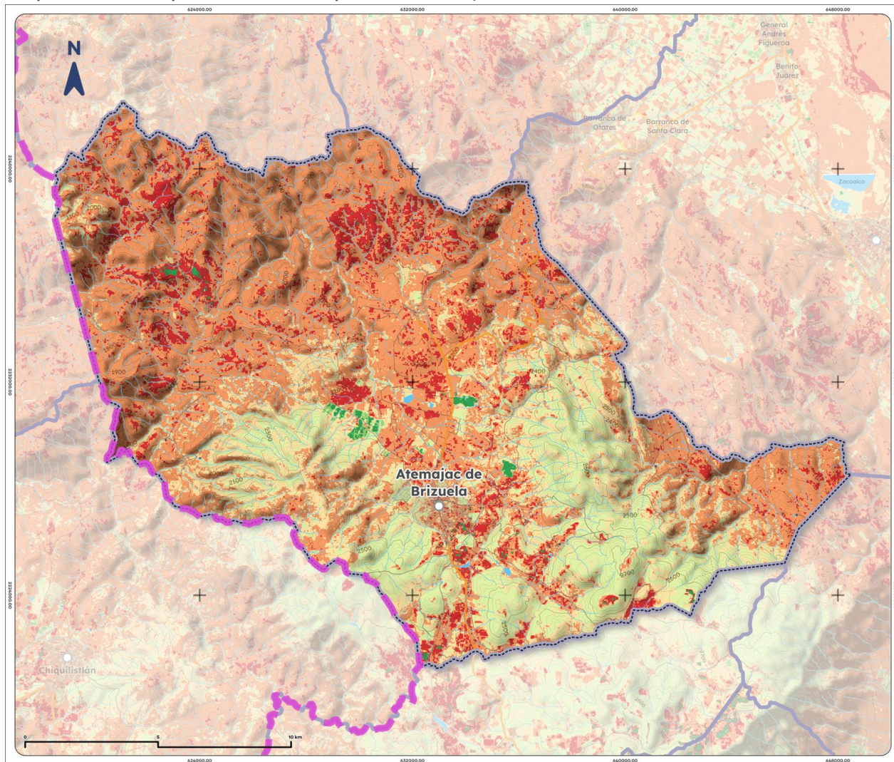
Mapa 15. Índice promedio de sequía de Atemajac de Brizuela, 2025
