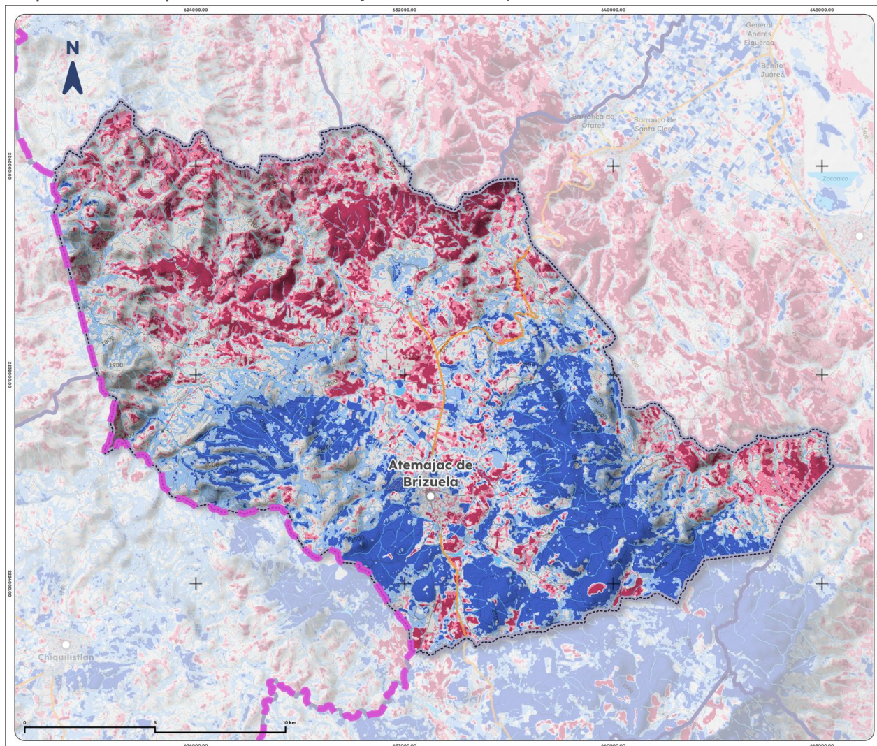
Mapa 13. NDWI promedio de Atemajac de Brizuela, 2025
