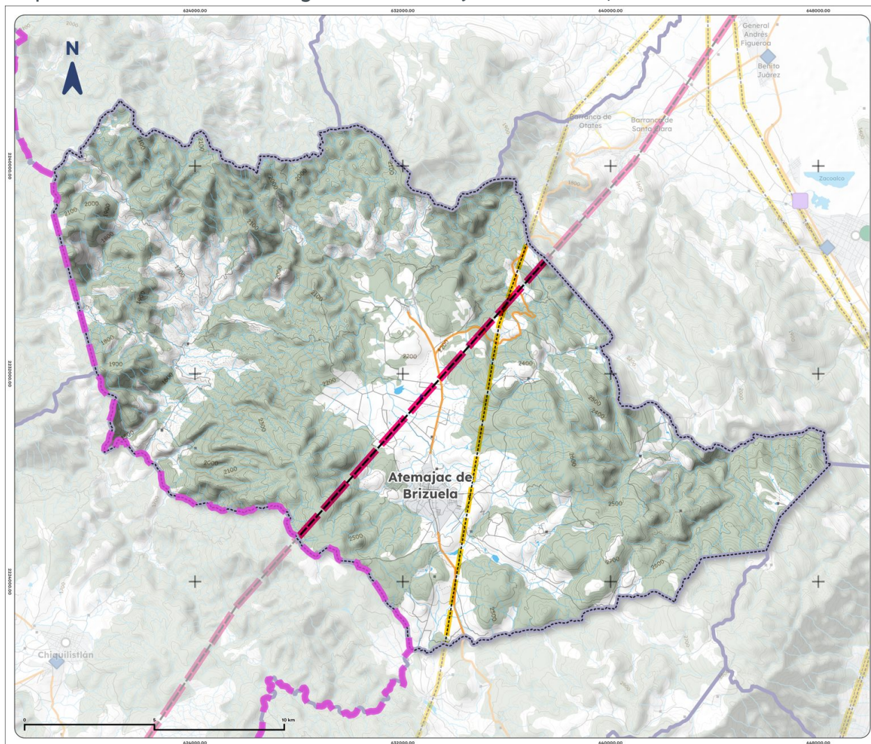
Mapa 22. Infraestructura energética de Atemajac de Brizuela, 2025
