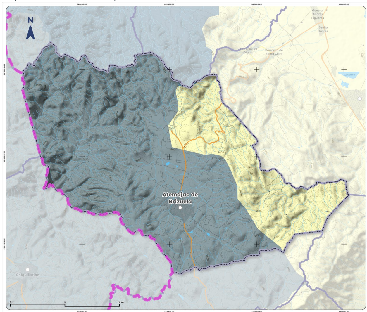
Mapa 6. Cuencas de Atemajac de Brizuela, 2023
