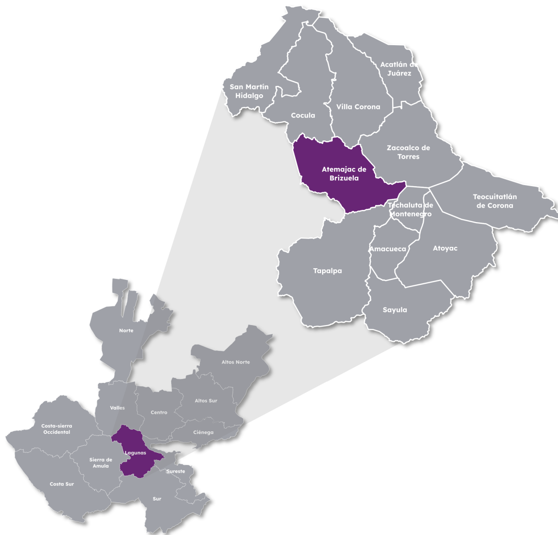
Mapa 1. Localización geográfica de Atemajac de Brizuela, Jalisco
