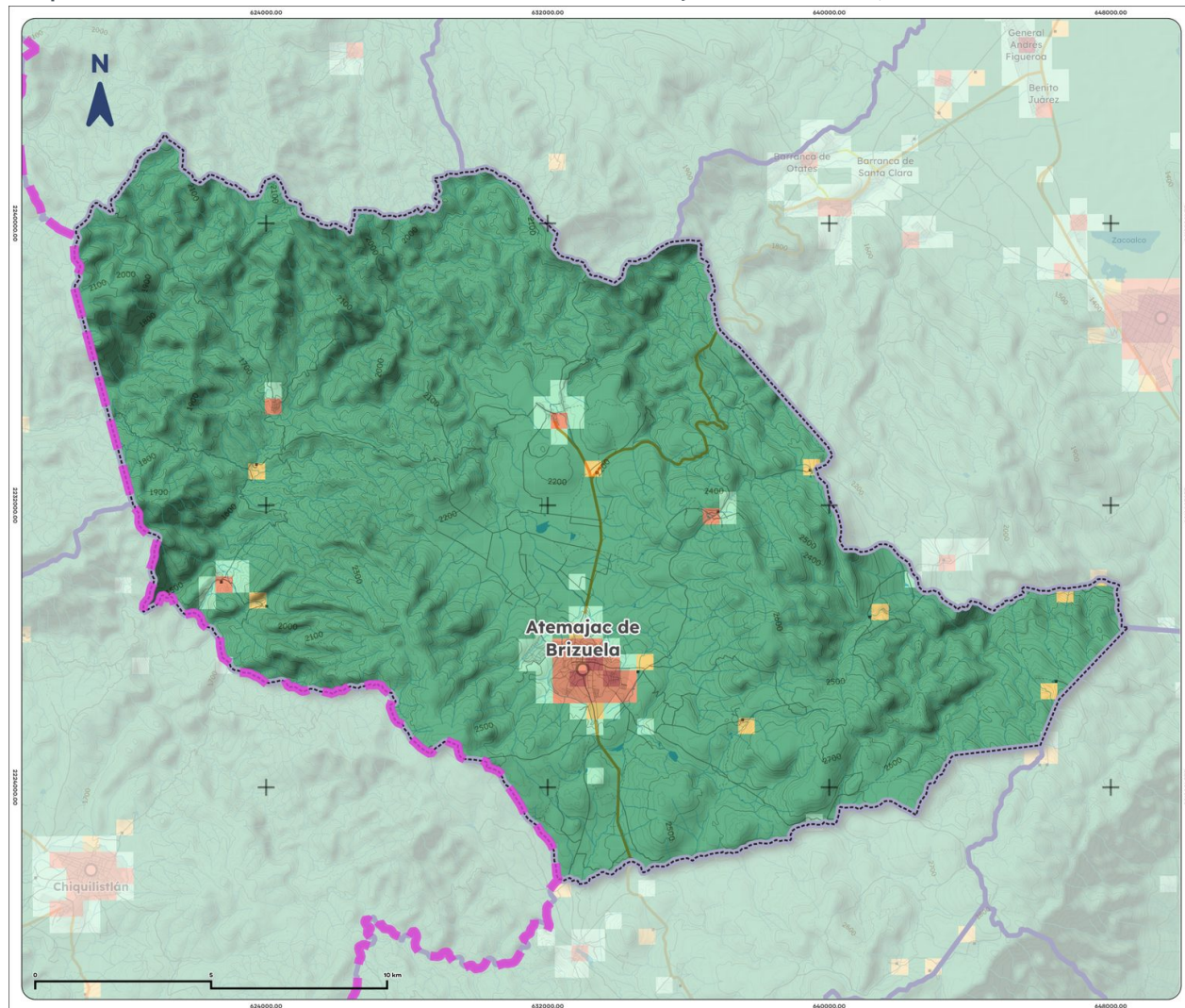
Mapa 18. Índice Territorial Urbano-Rural de Atemajac de Brizuela, 2025
