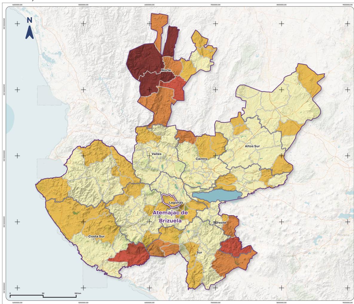
Mapa 25. Grado de marginación en Atemajac de Brizuela y el resto de municipios de Jalisco, 2020
