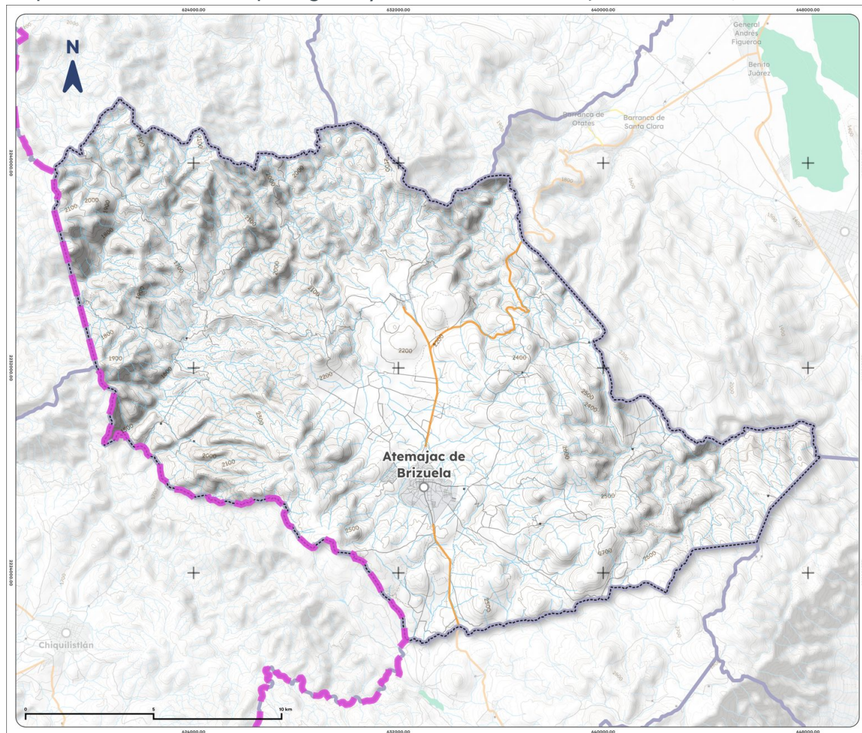
Mapa 14. Áreas naturales protegidas y humedales de Atemajac de Brizuela, 2025
