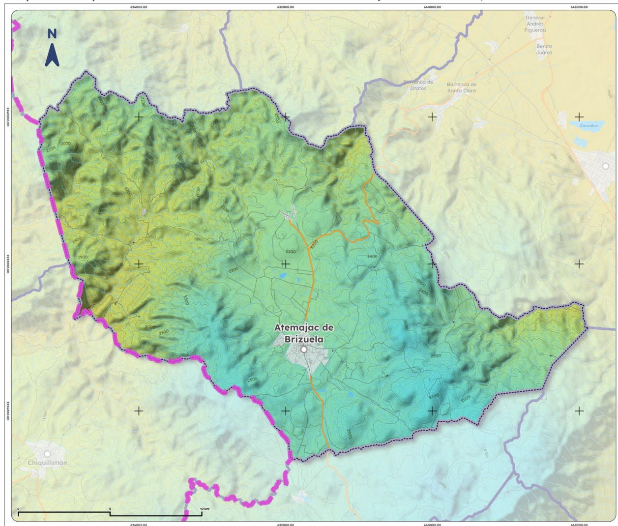
Mapa 8. Temperatura media anual histórica de Atemajac de Brizuela, 1995-2025
