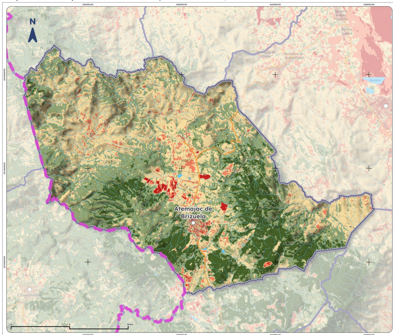
Mapa 12. NDVI promedio de Atemajac de Brizuela, 2025
