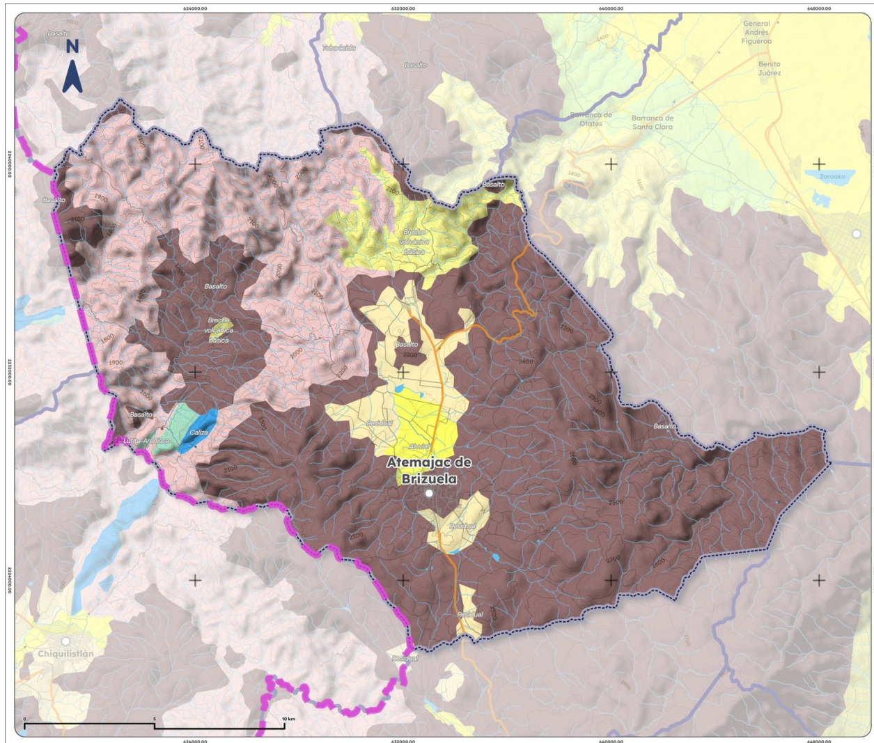
Mapa 3. Geología de Atemajac de Brizuela, 1988
