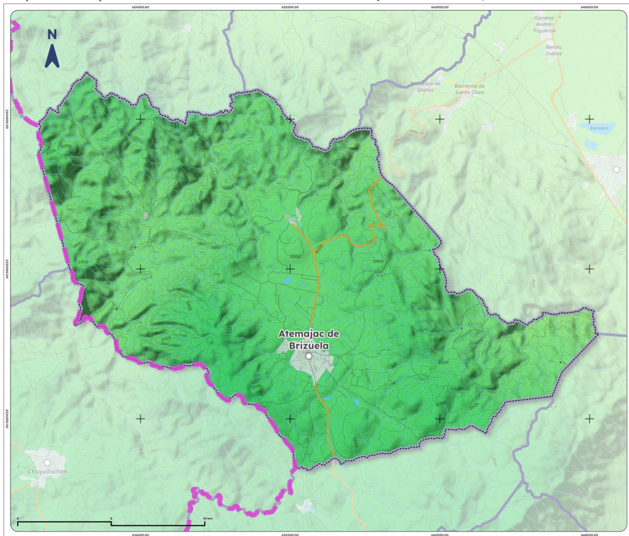
Mapa 9. Precipitación histórica acumulada de Atemajac de Brizuela, 1995-2025
