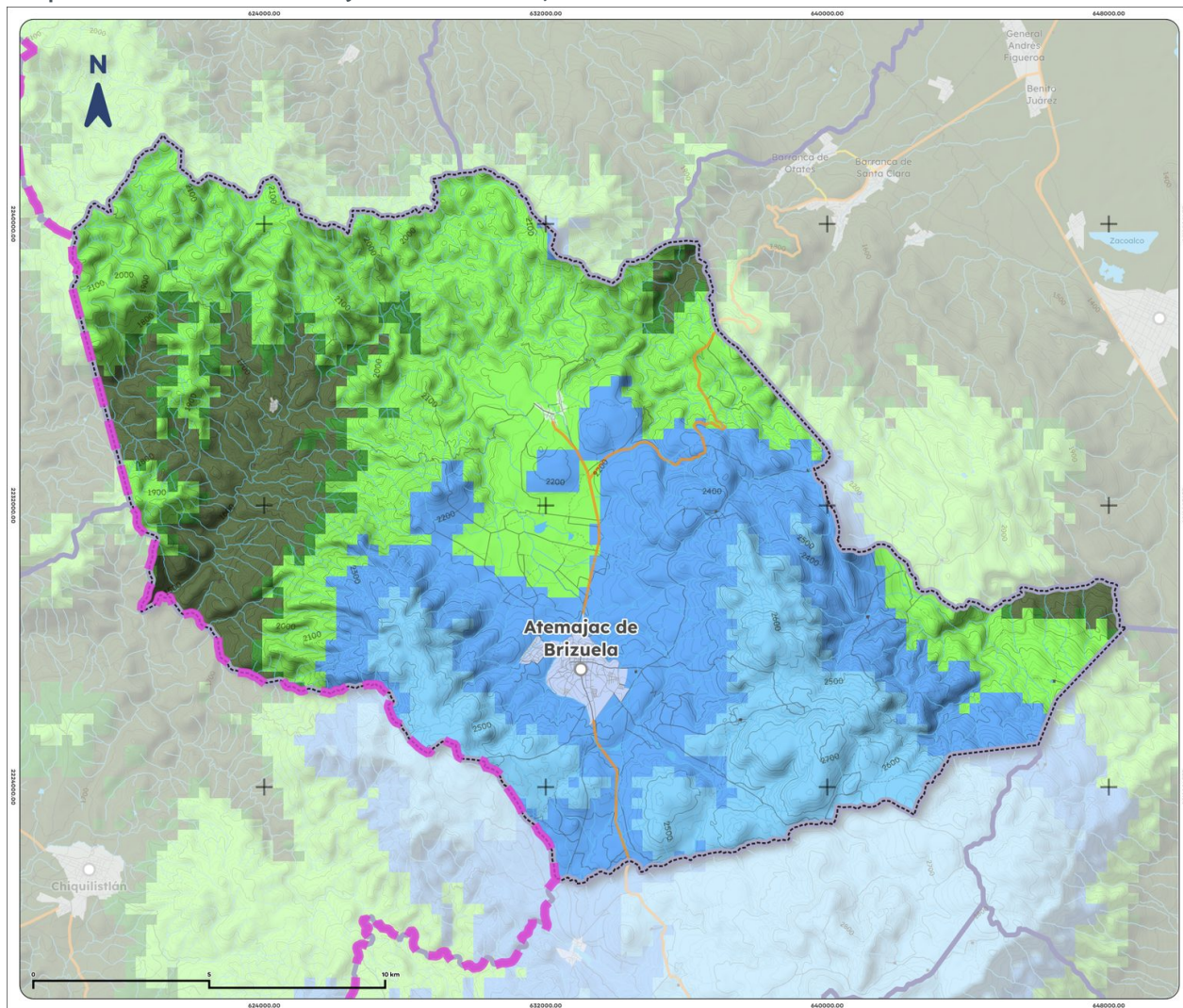
Mapa 10. Clima de Atemajac de Brizuela, 1995-2025
