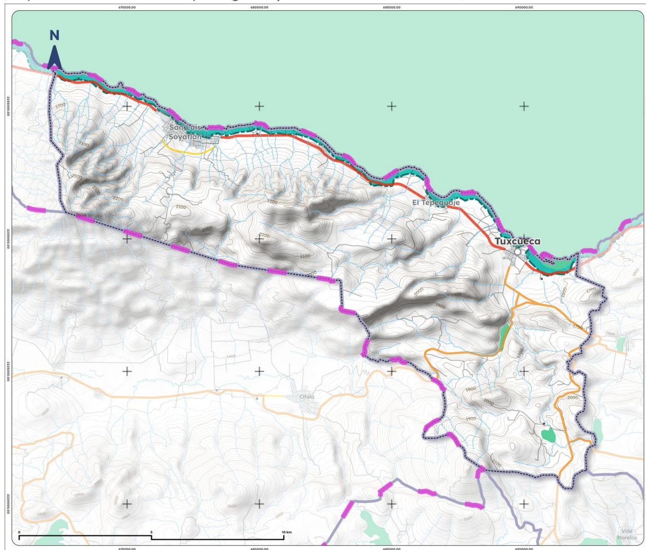
Mapa 14. Áreas naturales protegidas y humedales de Tuxcueca, 2025
