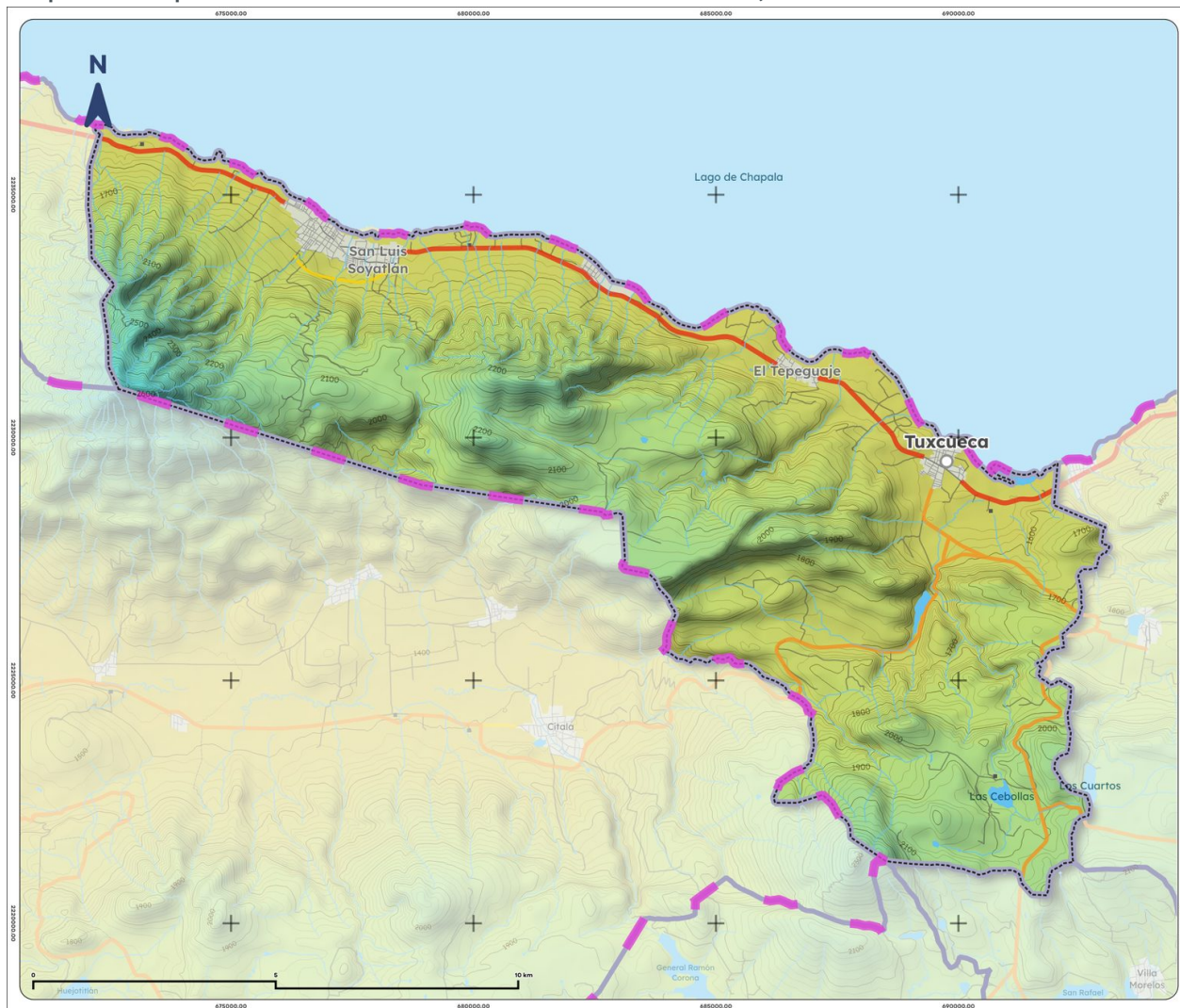
Mapa 8. Temperatura media anual histórica de Tuxcueca, 1995-2025
