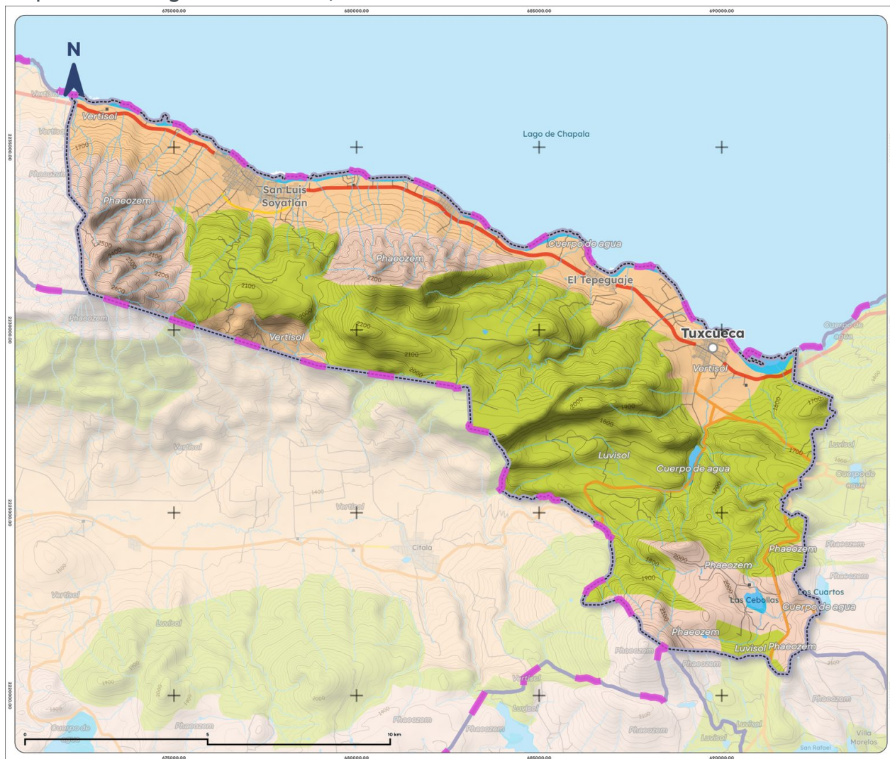
Mapa 4. Edafología de Tuxcueca, 2025
