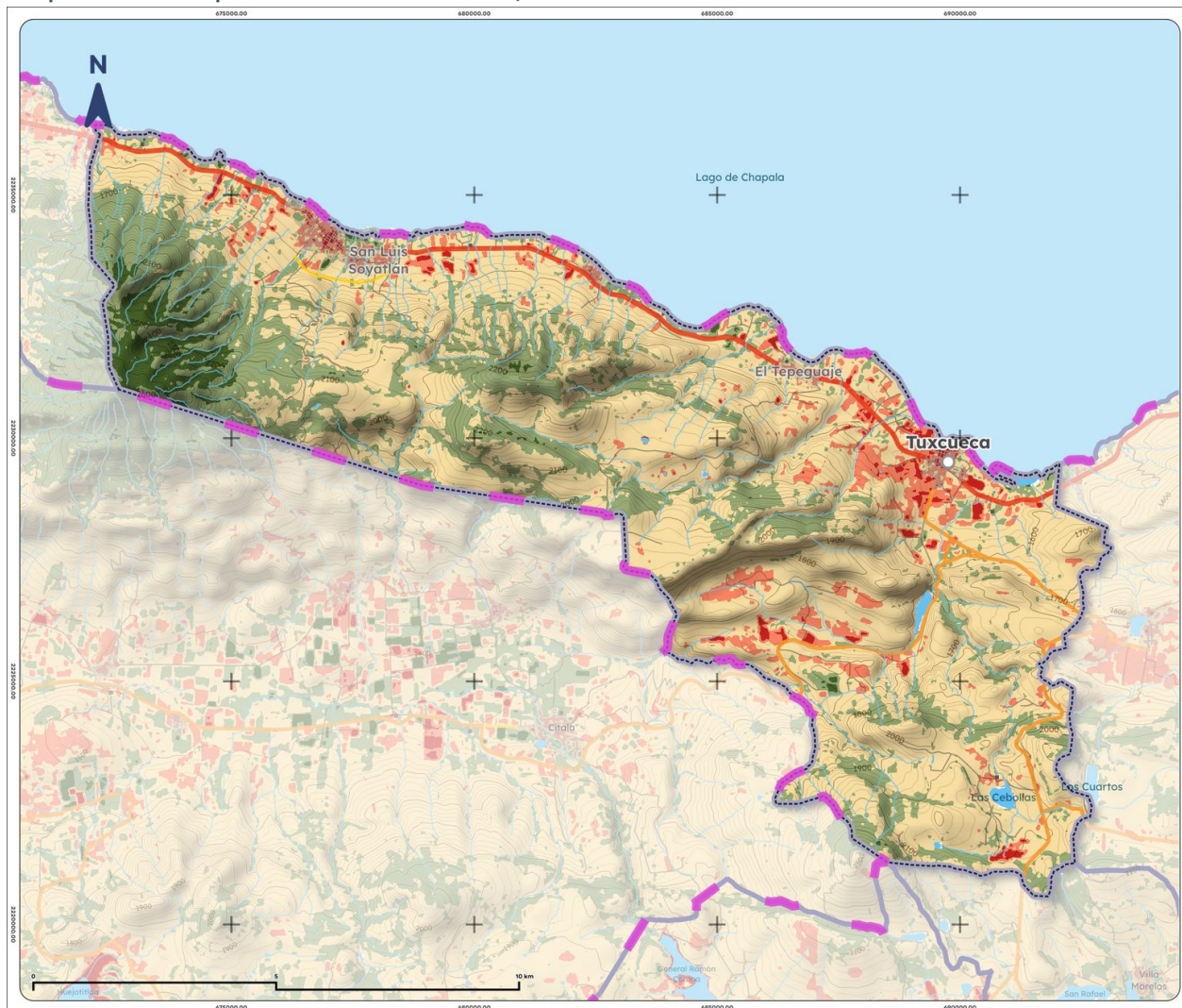
Mapa 12. NDVI promedio de Tuxcueca, 2025
