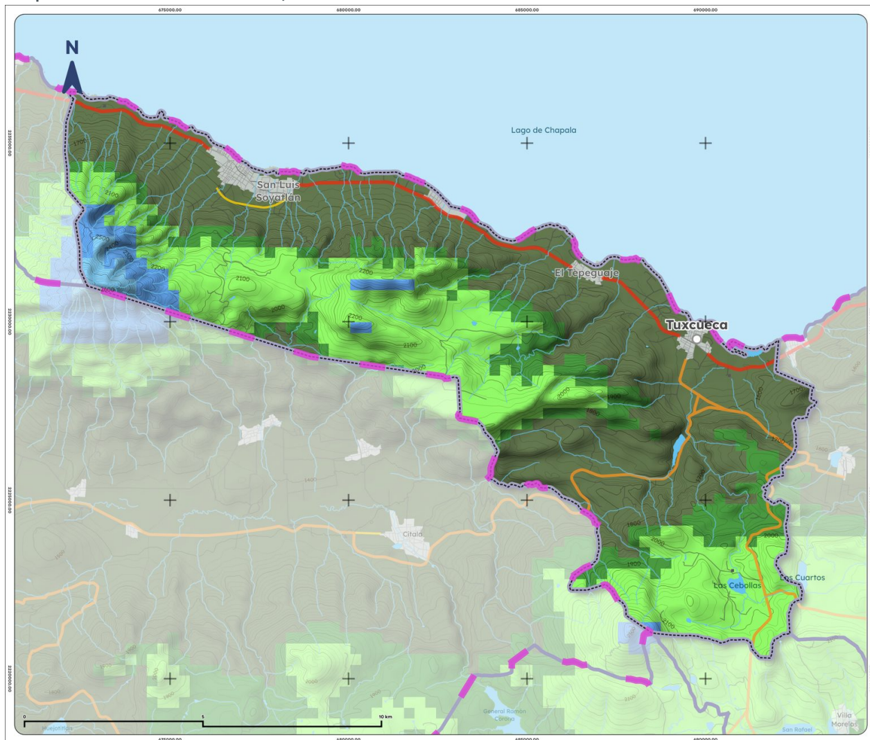
Mapa 10. Clima de Tuxcueca, 1995-2025
