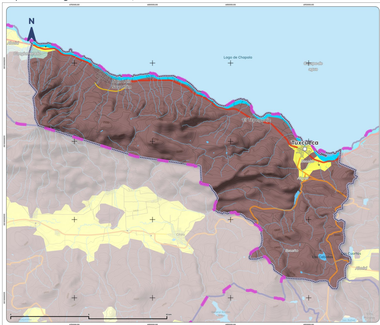
Mapa 3. Geología de Tuxcueca, 1988
