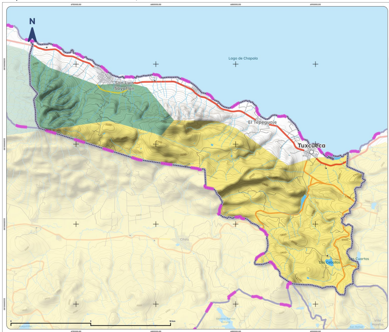
Mapa 7. Acuíferos de Tuxcueca, 2023
