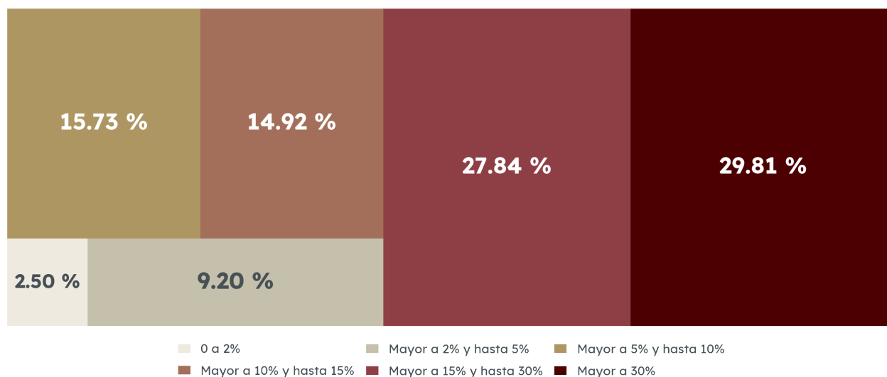
Topografía y pendientes de Tuxcueca, 2025
