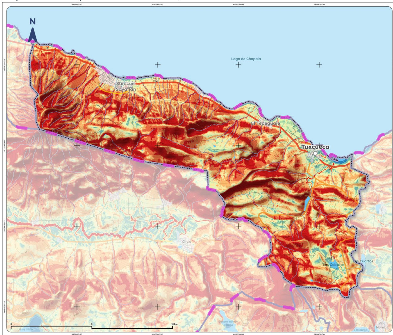
Mapa 16. Erosión potencial de Tuxcueca, 2025
