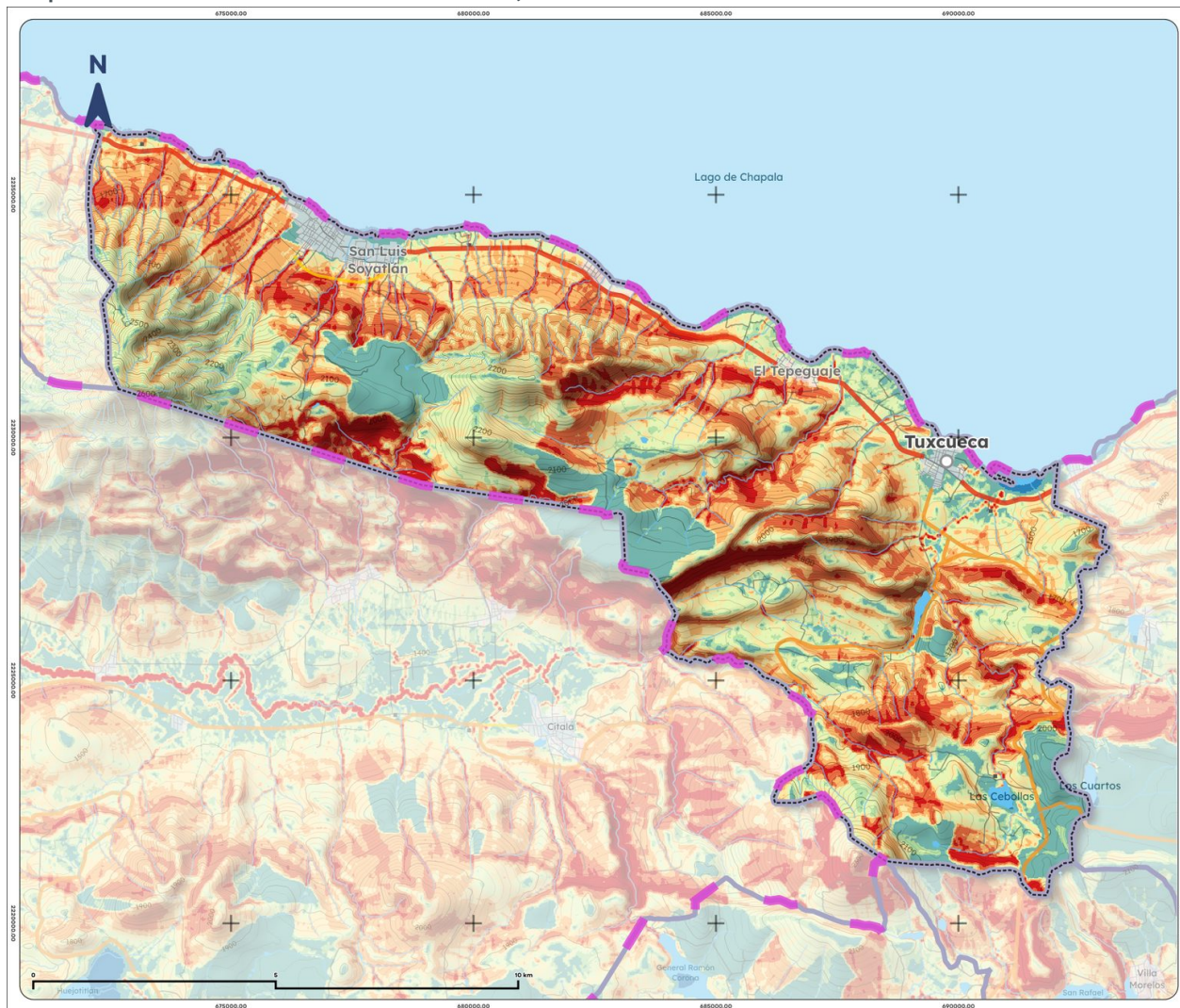
Mapa 17. Erosión efectiva de Tuxcueca, 2025
