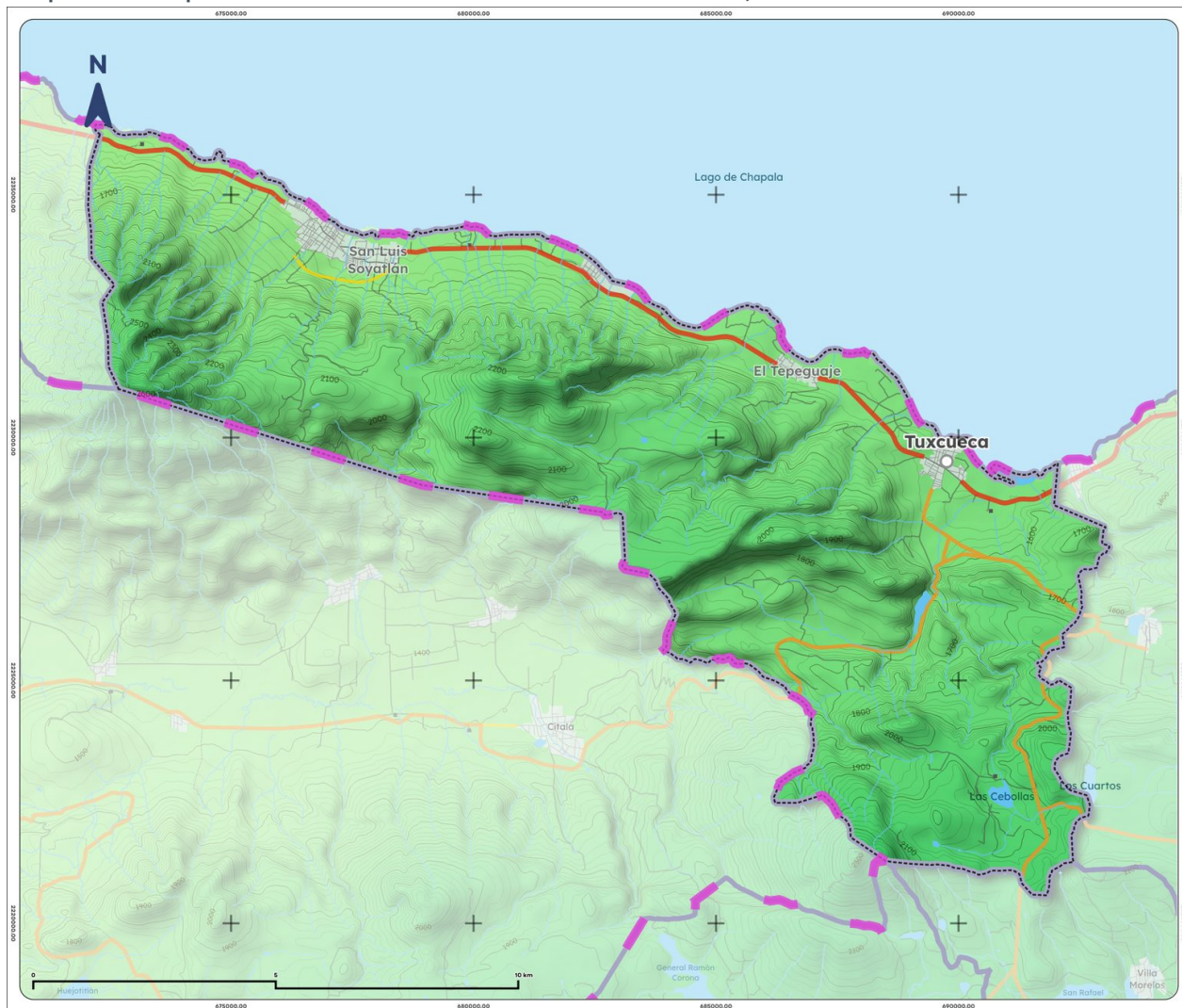
Mapa 9. Precipitación histórica acumulada de Tuxcueca, 1995-2025
