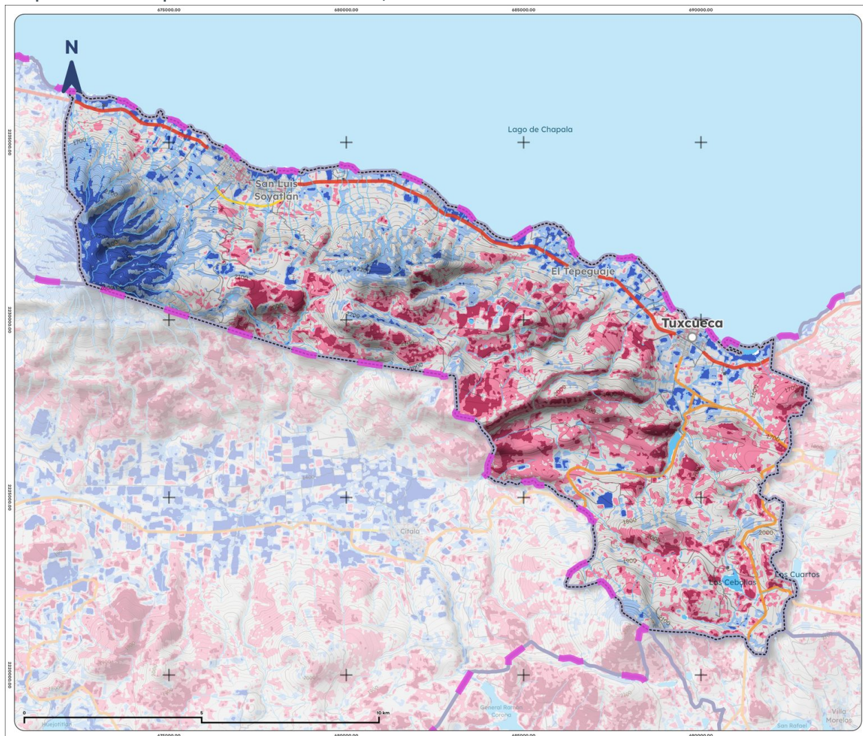
Mapa 13. NDWI promedio de Tuxcueca, 2025
