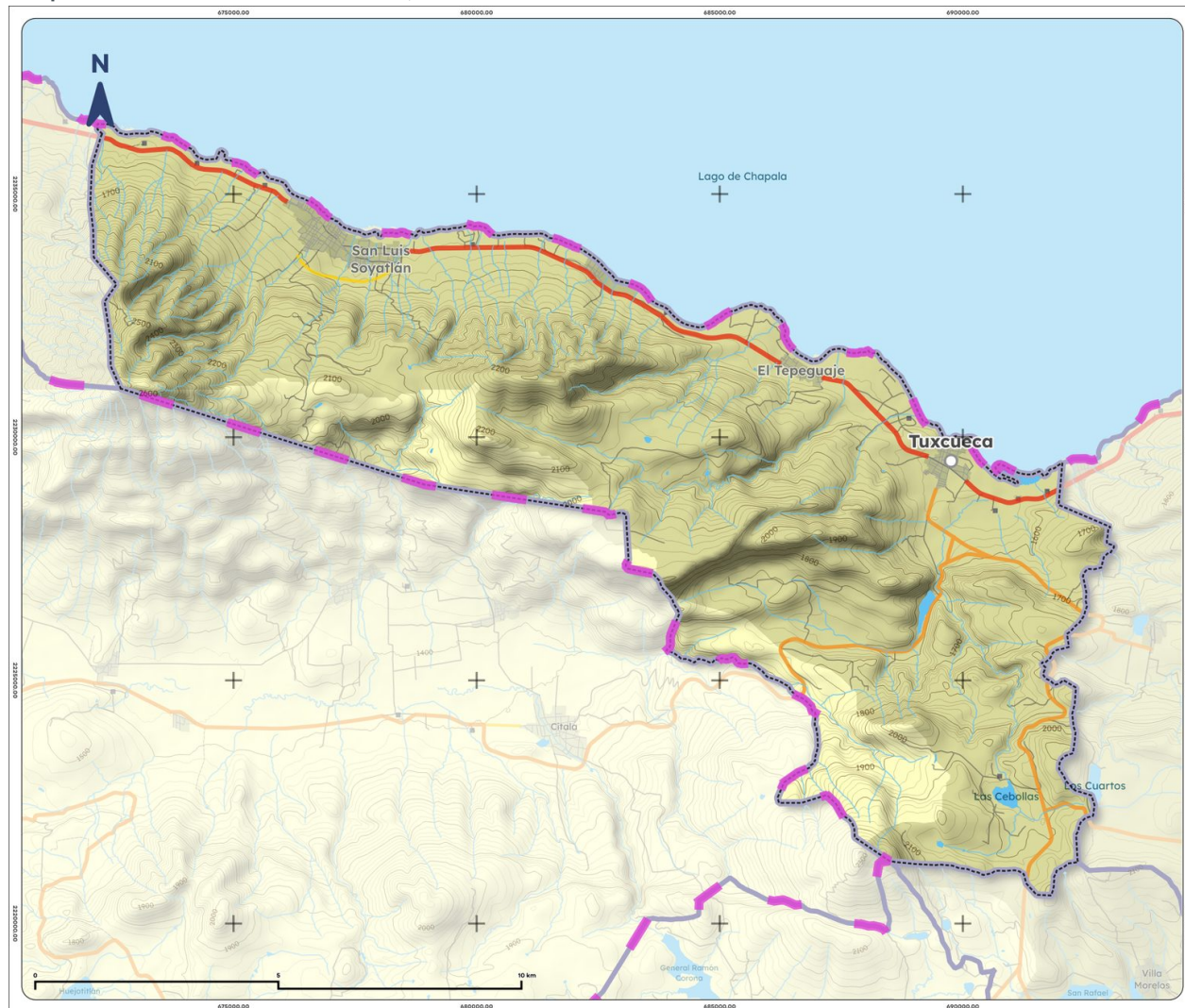
Mapa 6. Cuencas de Tuxcueca, 2023
