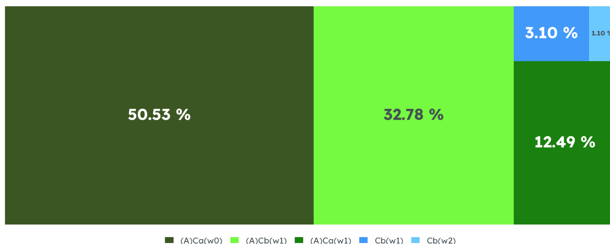
Clima de Tuxcueca, 1995-2025
