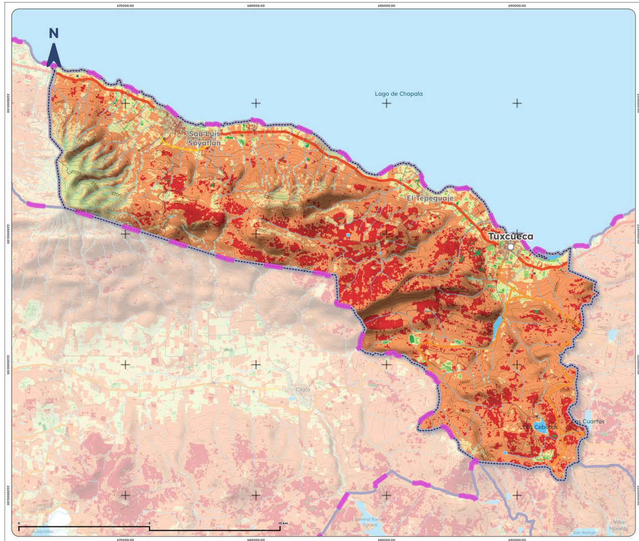
Mapa 15. Índice promedio de sequía de Tuxcueca, 2025
