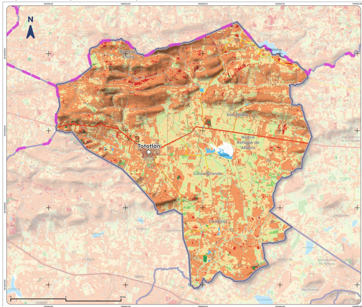
Mapa 15. Índice promedio de sequía de Tototlán, 2025
