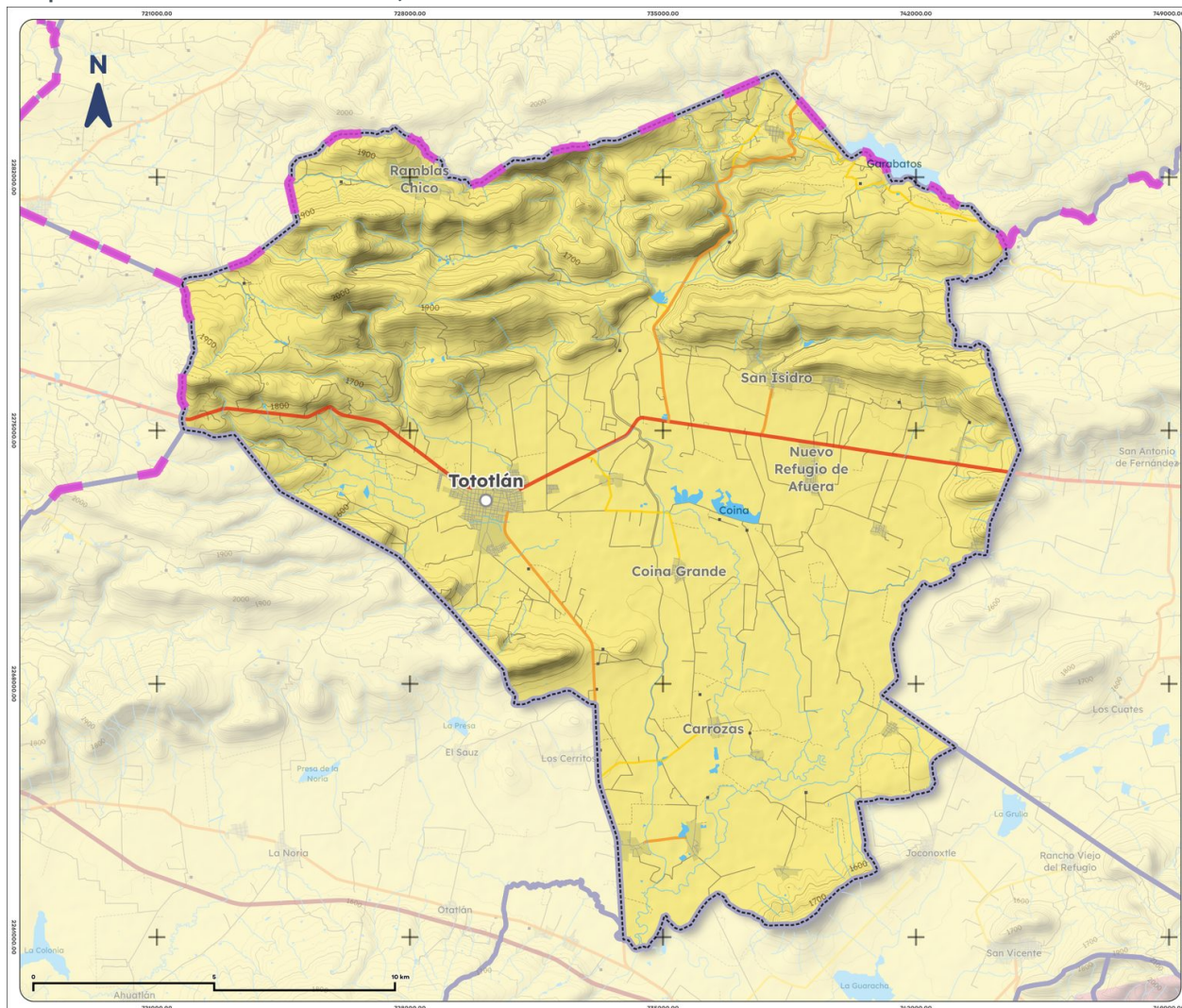
Mapa 7. Acuíferos de Tototlán, 2023
