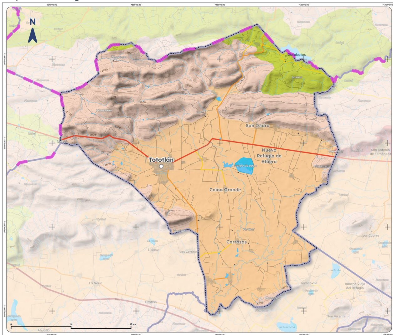
Mapa 4. Edafología de Tototlán, 2025
