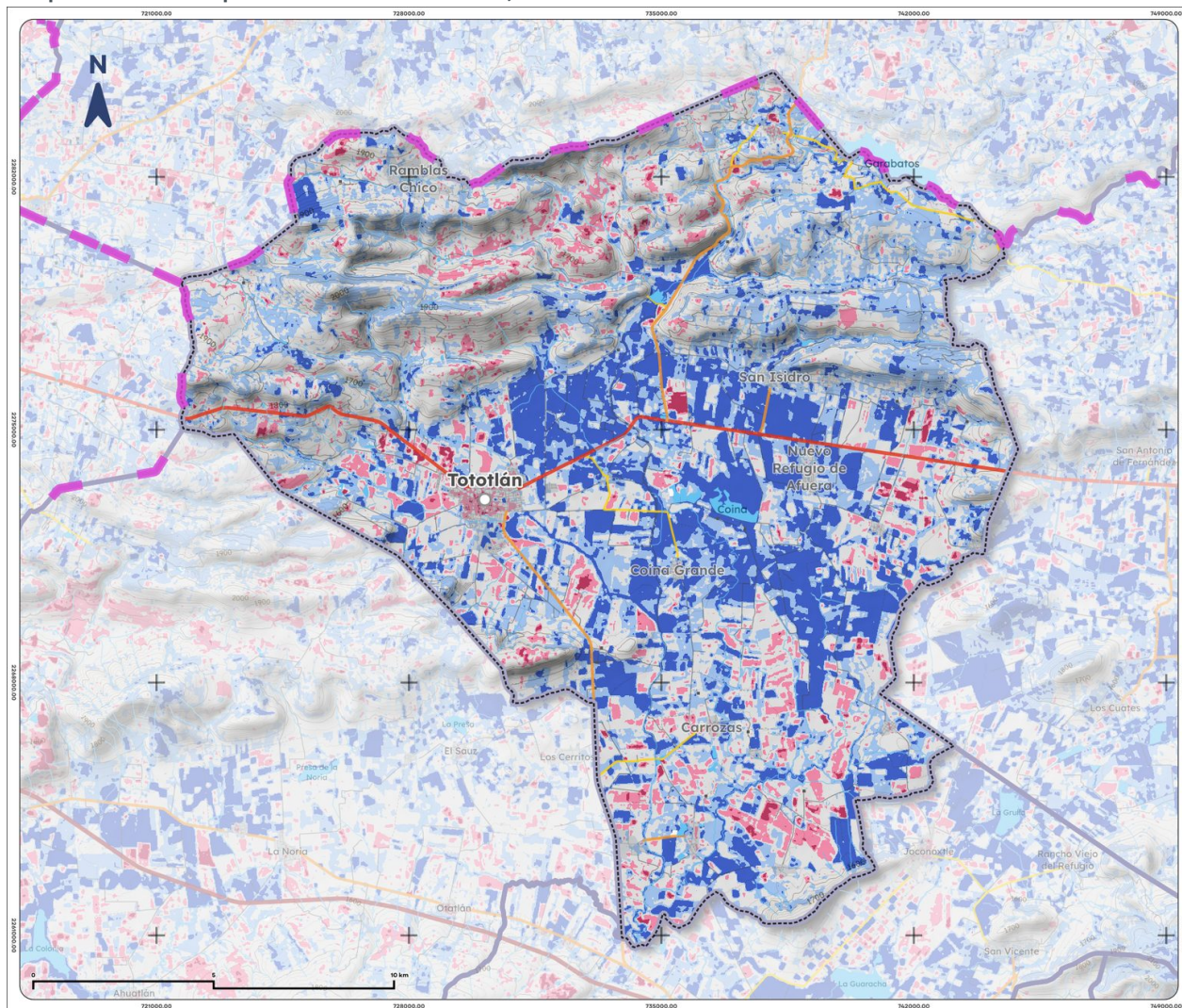
Mapa 13. NDWI promedio de Tototlán, 2025
