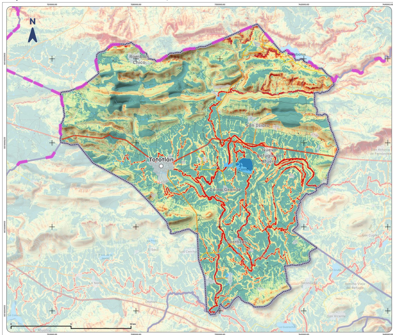
Mapa 17. Erosión efectiva de Tototlán, 2025
