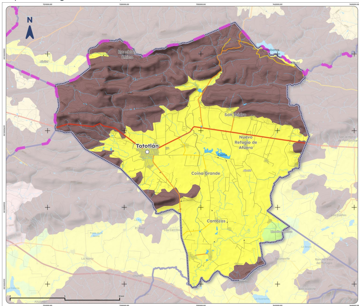
Mapa 3. Geología de Tototlán, 1988
