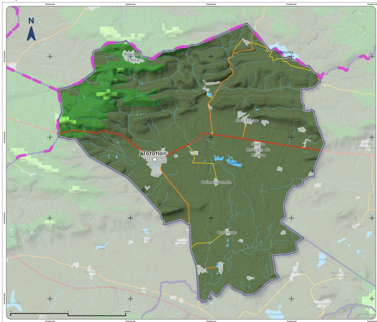
Mapa 10. Clima de Tototlán, 1995-2025
