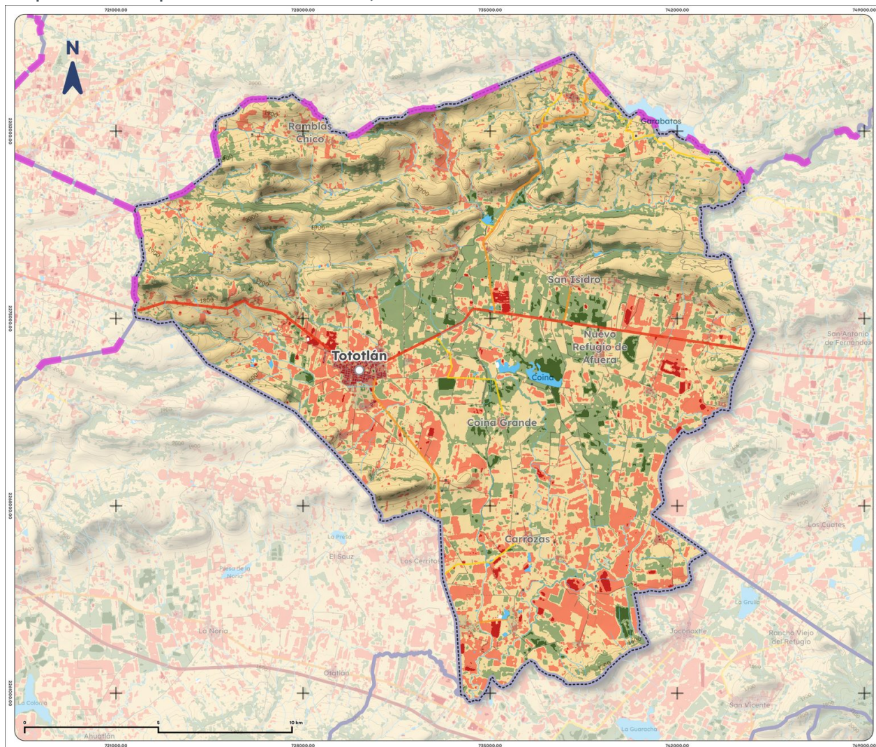
Mapa 12. NDVI promedio de Tototlán, 2025
