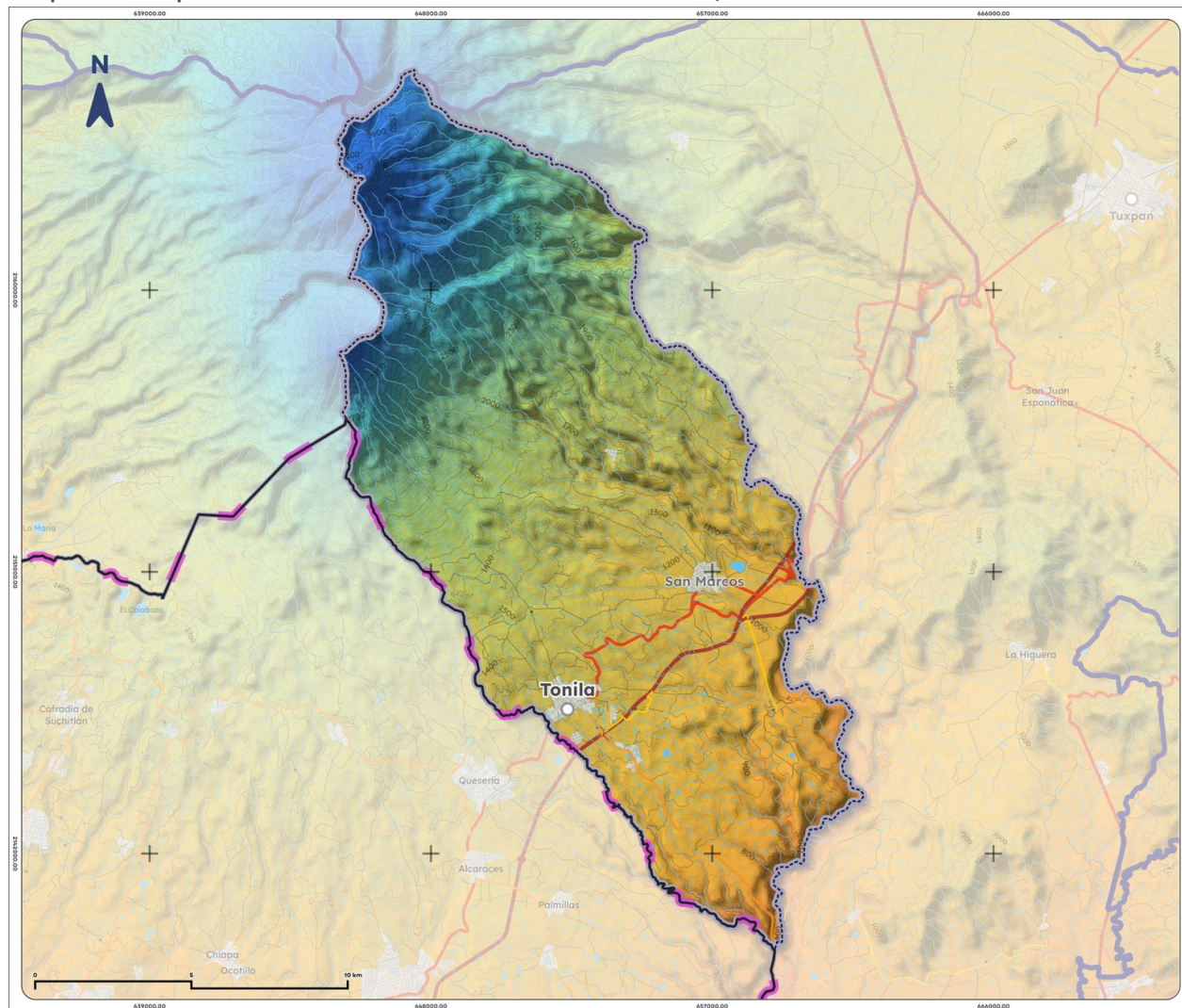
Mapa 8. Temperatura media anual histórica de Tonila, 1995-2025
