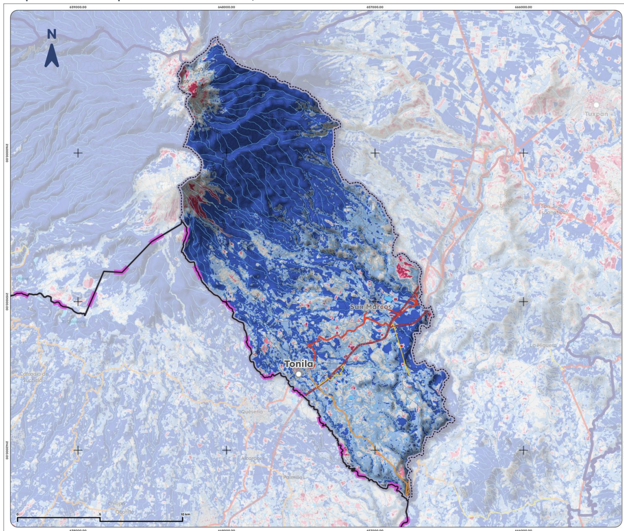
Mapa 13. NDWI promedio de Tonila, 2025
