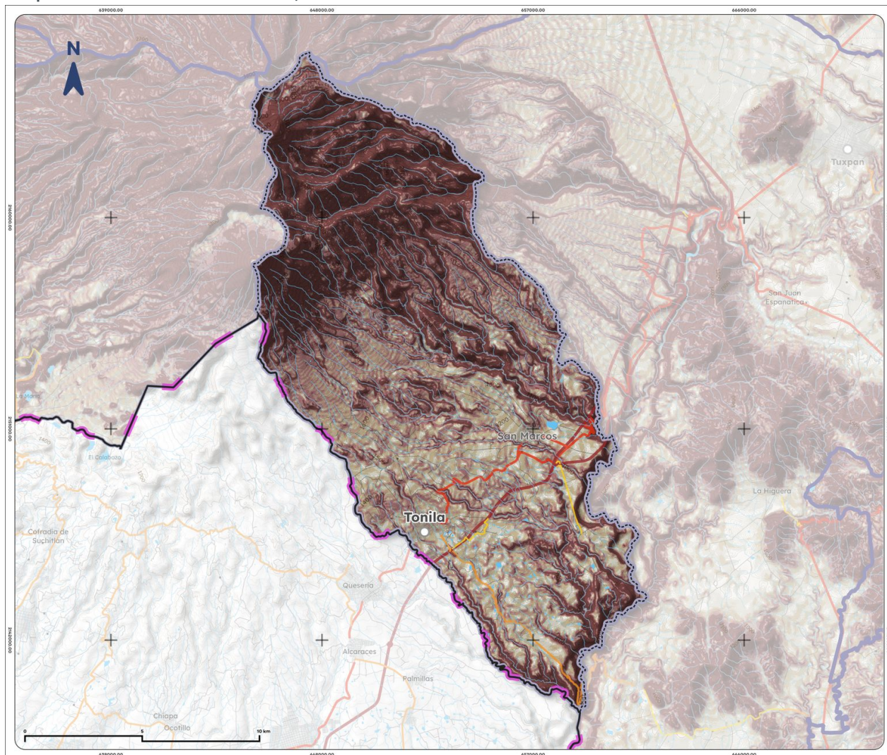
Mapa 5. Pendientes de Tonila, 2025
