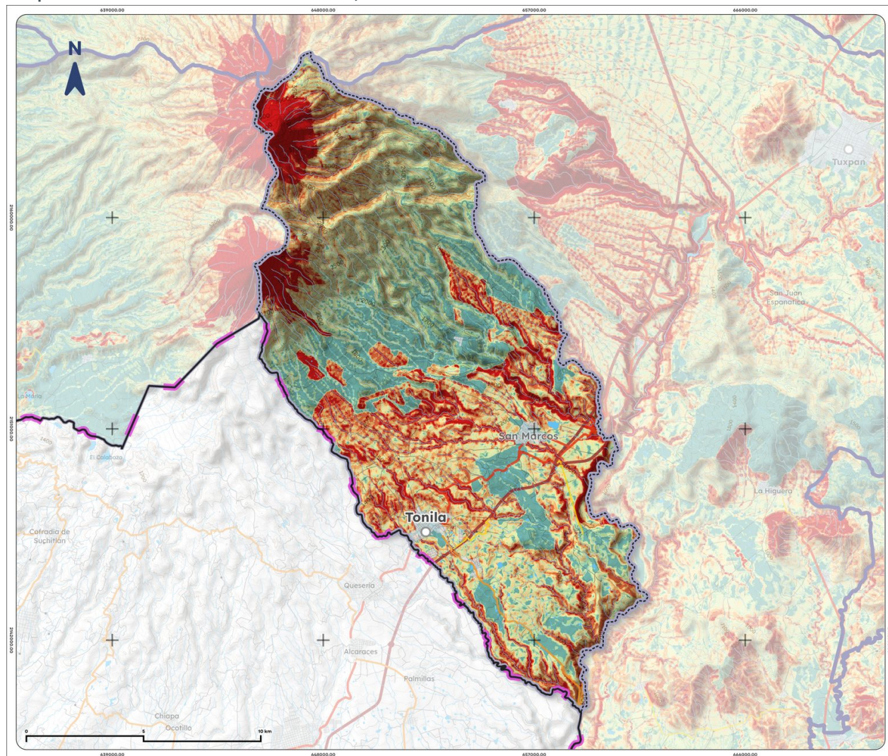
Mapa 17. Erosión efectiva de Tonila, 2025
