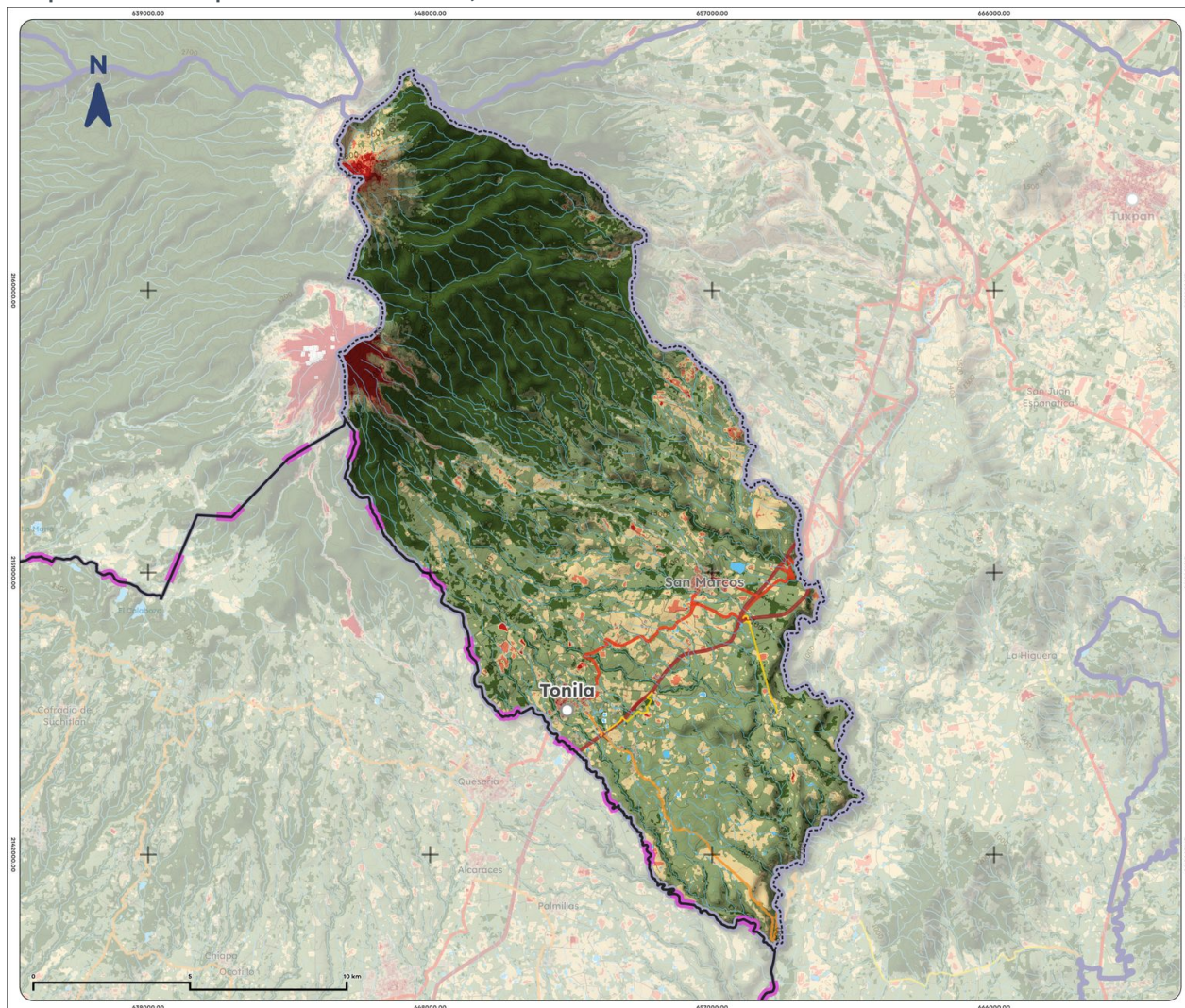
Mapa 12. NDVI promedio de Tonila, 2025
