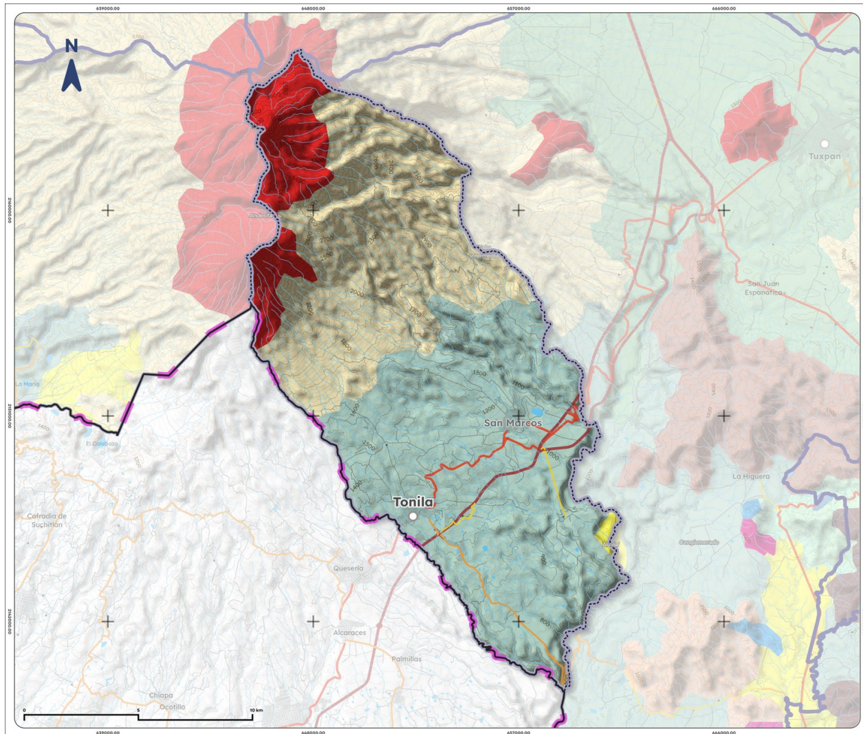
Mapa 3. Geología de Tonila, 1988
