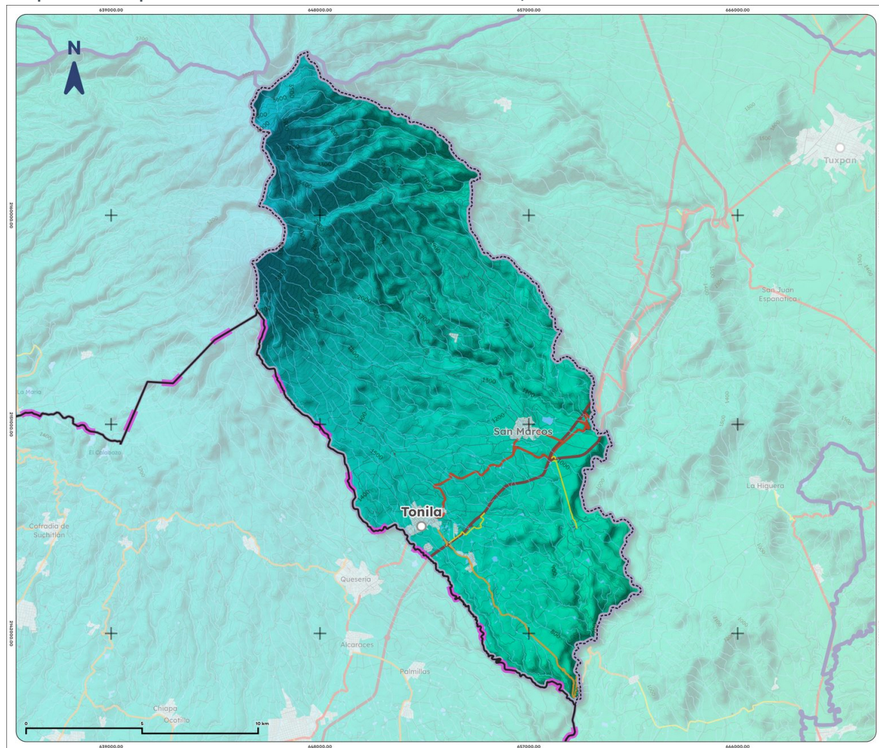
Mapa 9. Precipitación histórica acumulada de Tonila, 1995-2025
