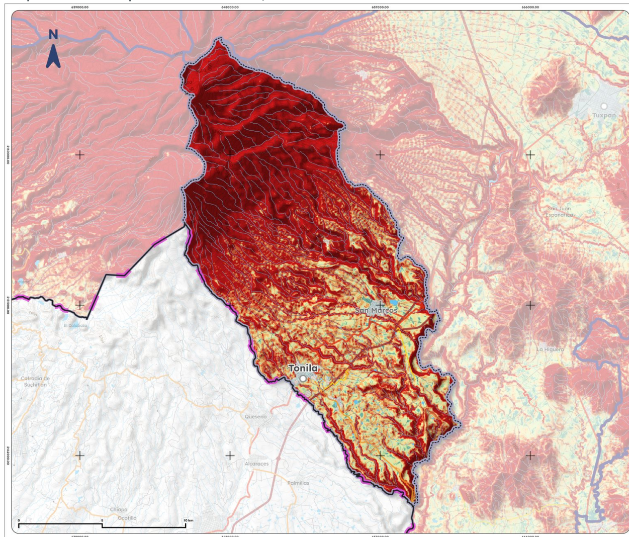
Mapa 16. Erosión potencial de Tonila, 2025
