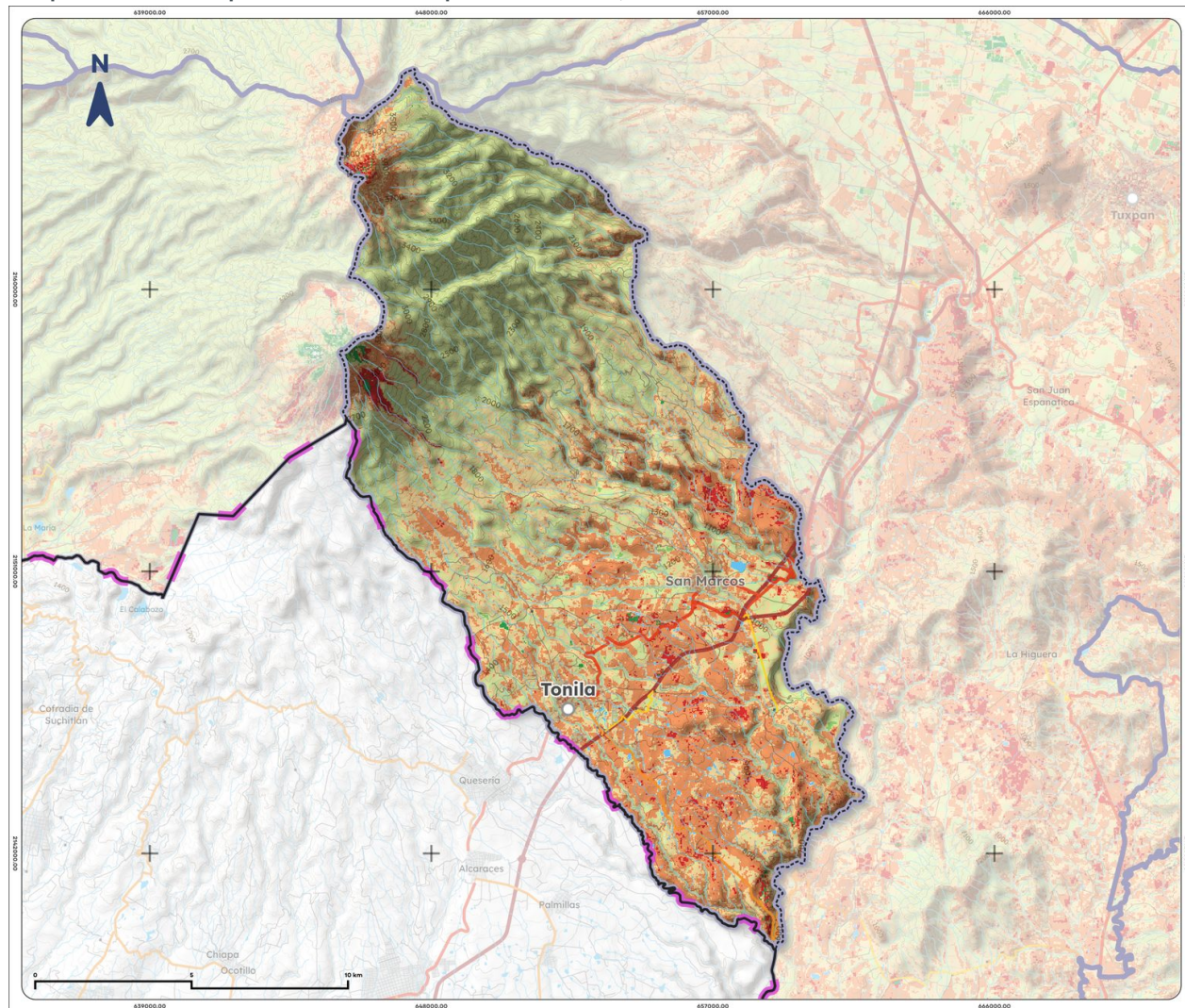
Mapa 15. Índice promedio de sequía de Tonila, 2025
