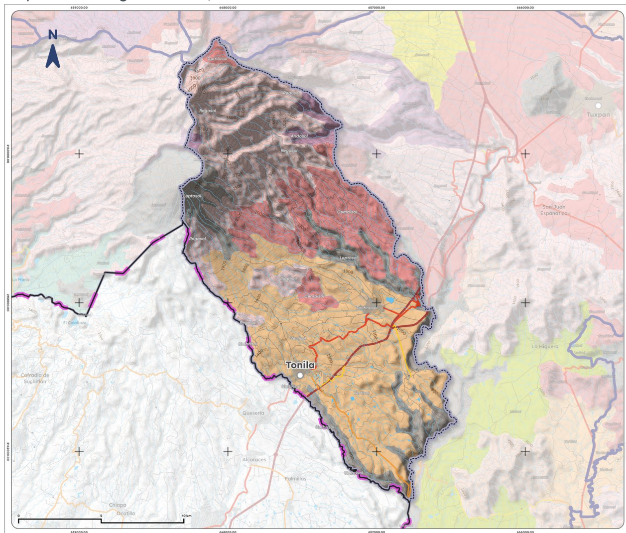
Mapa 4. Edafología de Tonila, 2025
