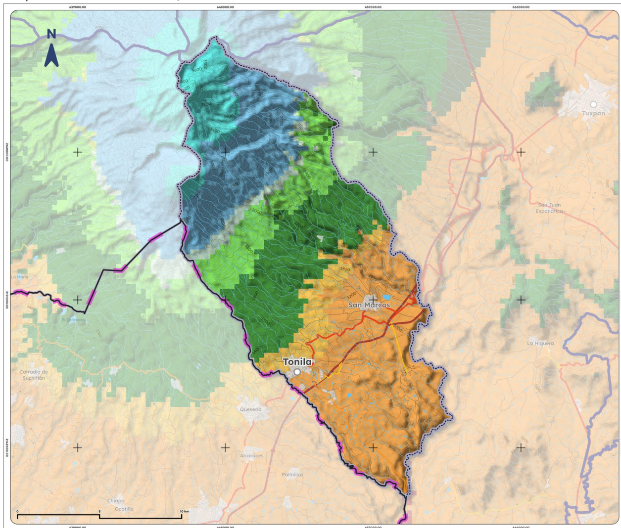
Mapa 10. Clima de Tonila, 1995-2025
