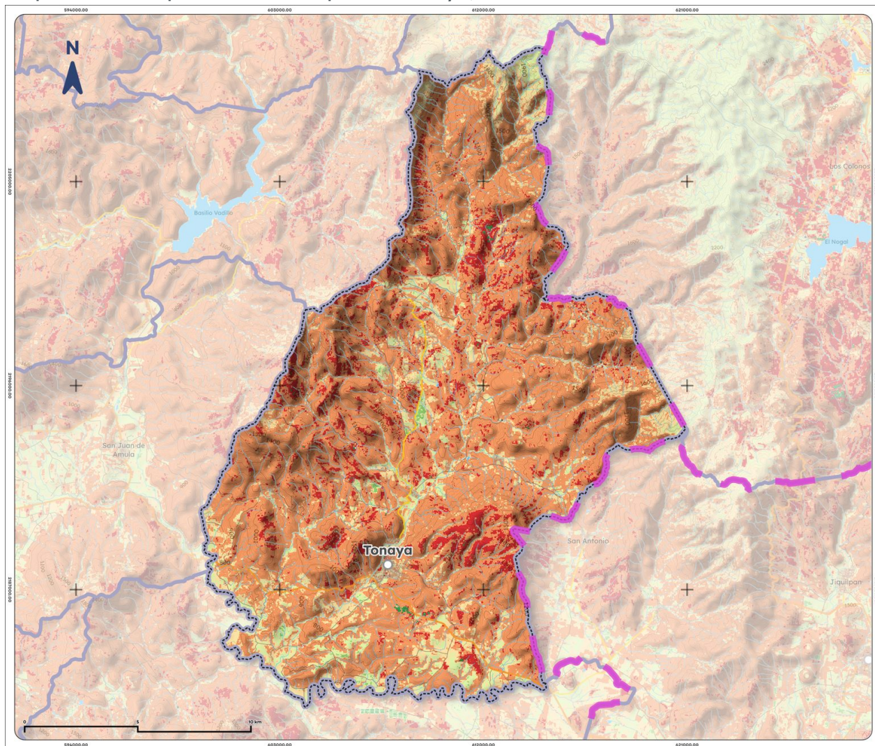
Mapa 15. Índice promedio de sequía de Tonaya, 2025
