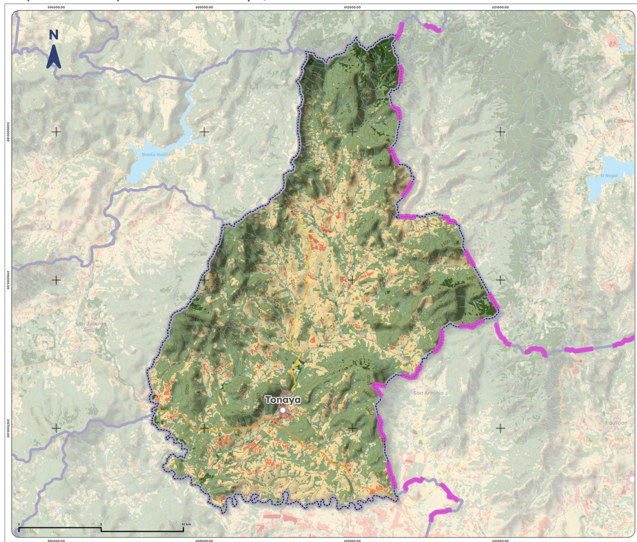
Mapa 12. NDVI promedio de Tonaya, 2025
