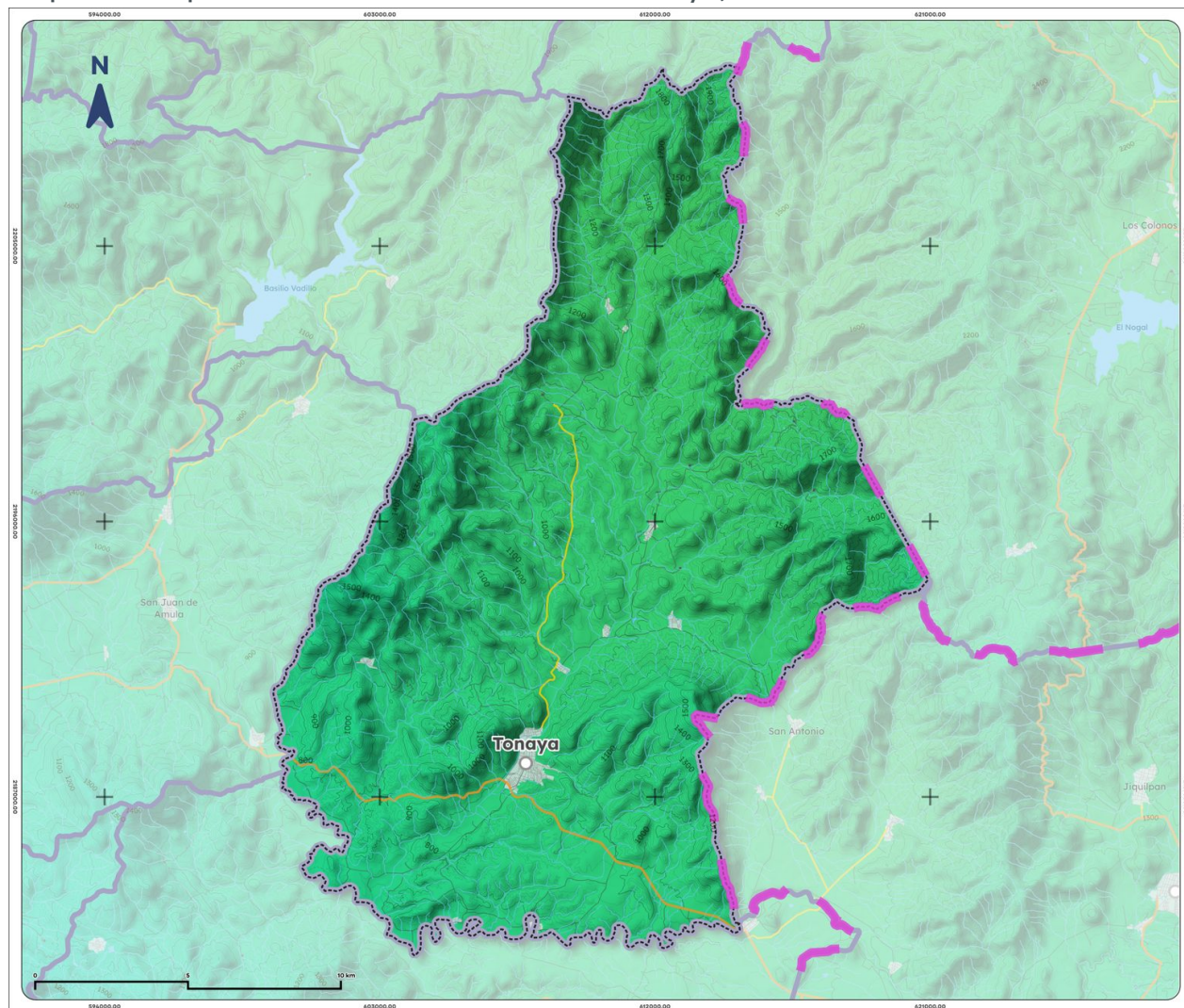
Mapa 9. Precipitación histórica acumulada de Tonaya, 1995-2025
