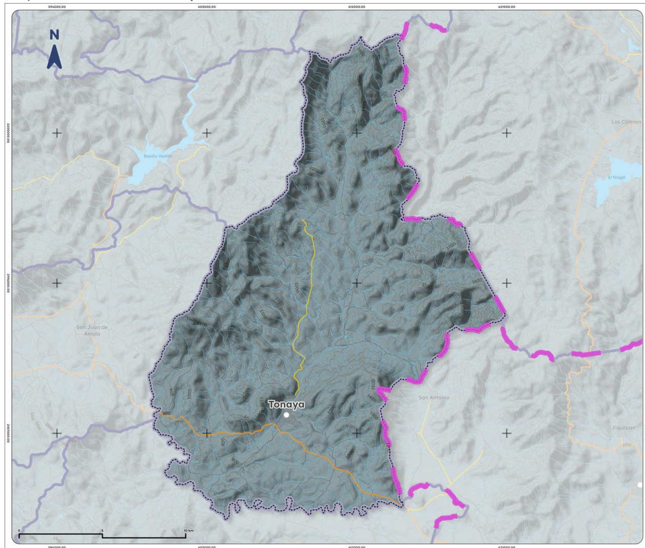
Mapa 6. Cuencas de Tonaya, 2023
