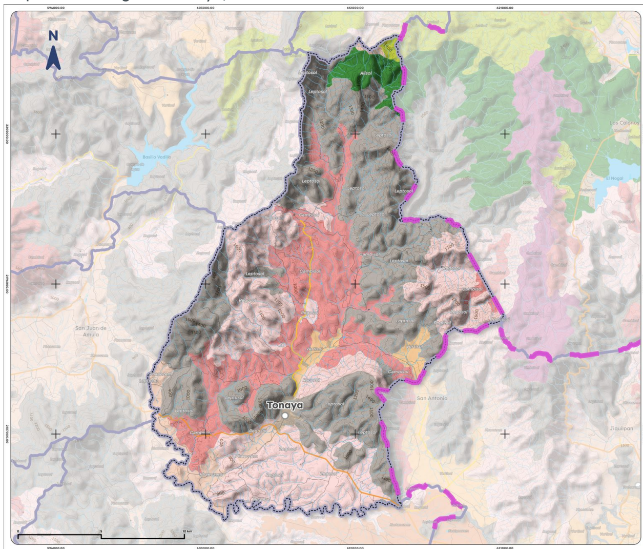
Mapa 4. Edafología de Tonaya, 2025
