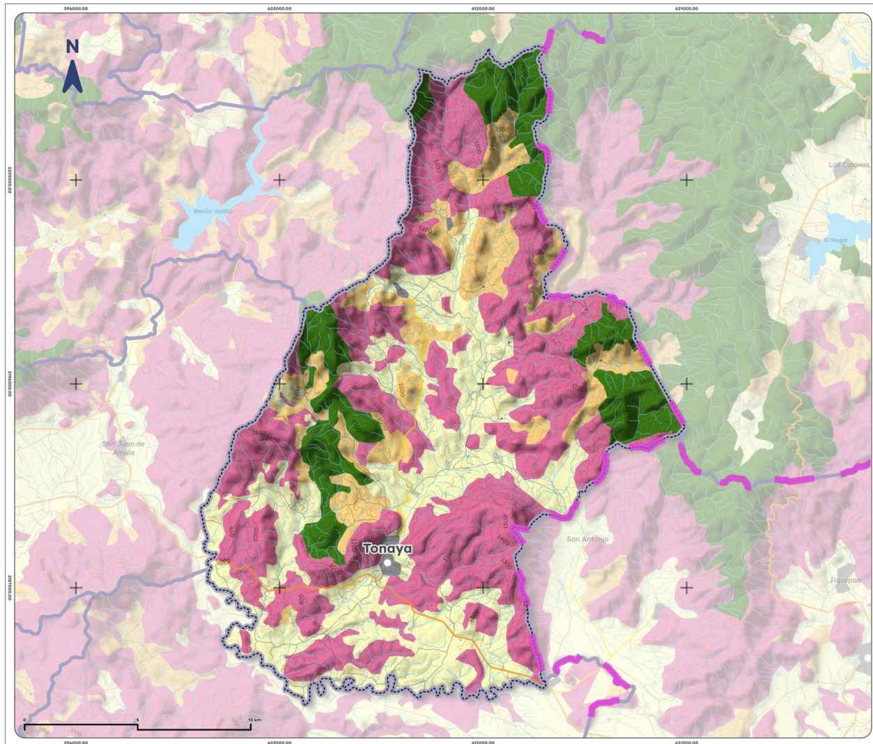
Mapa 11. Uso de suelo y vegetación de Tonaya, 2018
