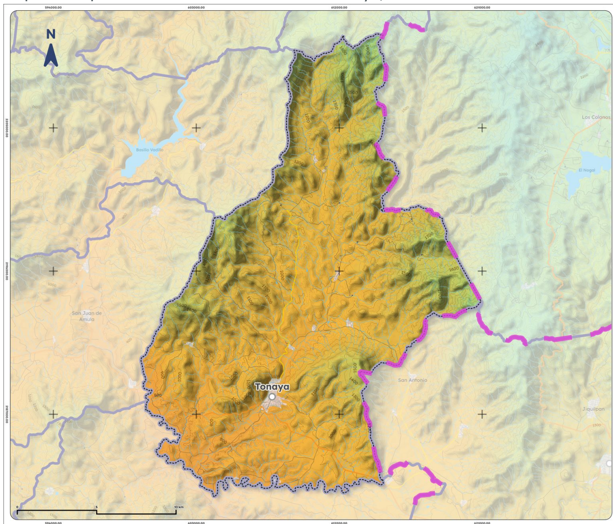
Mapa 8. Temperatura media anual histórica de Tonaya, 1995-2025
