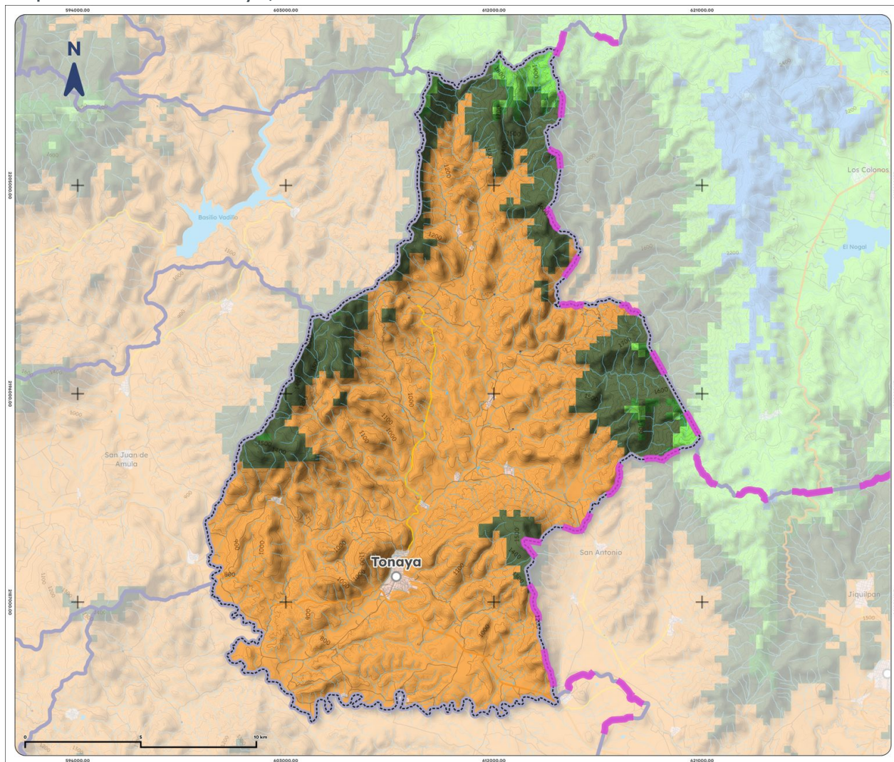
Mapa 10. Clima de Tonaya, 1995-2025
