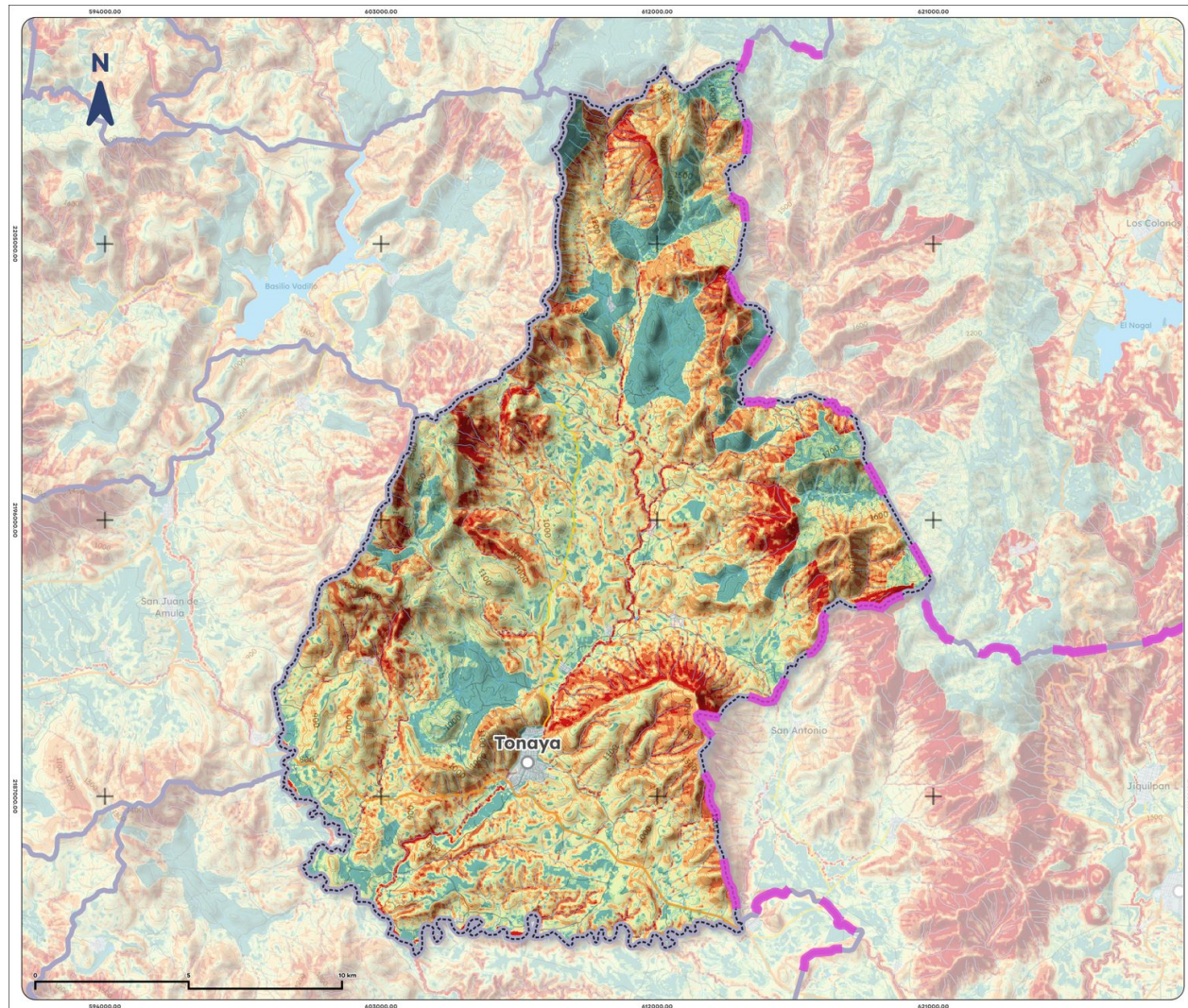
Mapa 17. Erosión efectiva de Tonaya, 2025
