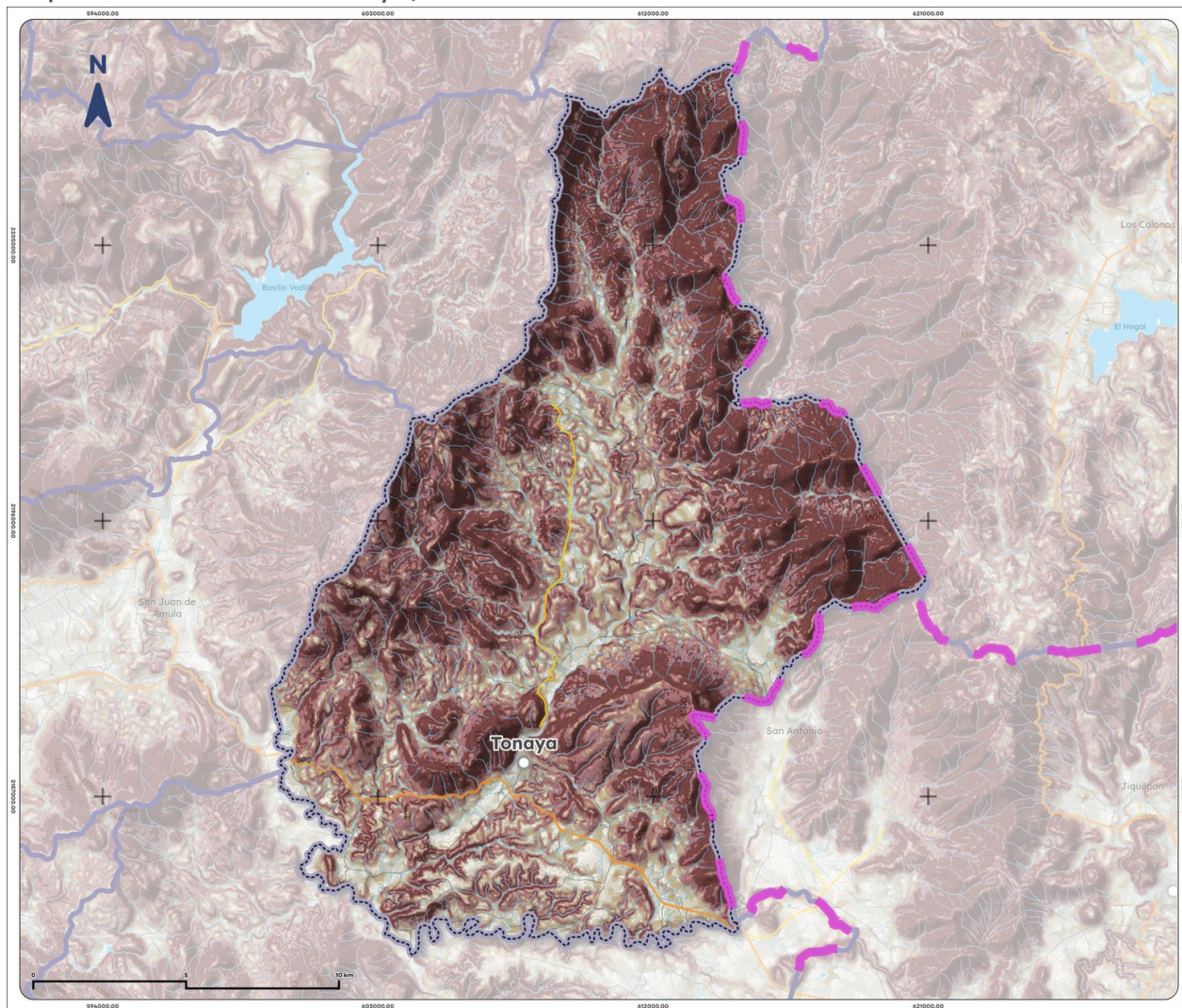
Mapa 5. Pendientes de Tonaya, 2025
