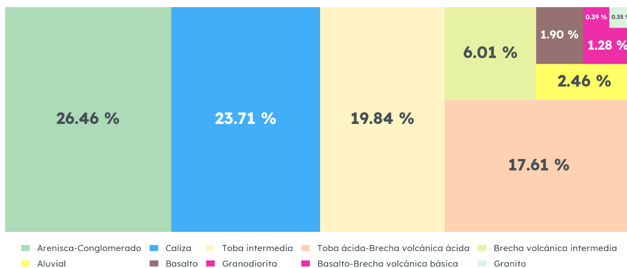
Geología de Tonaya, 1988
