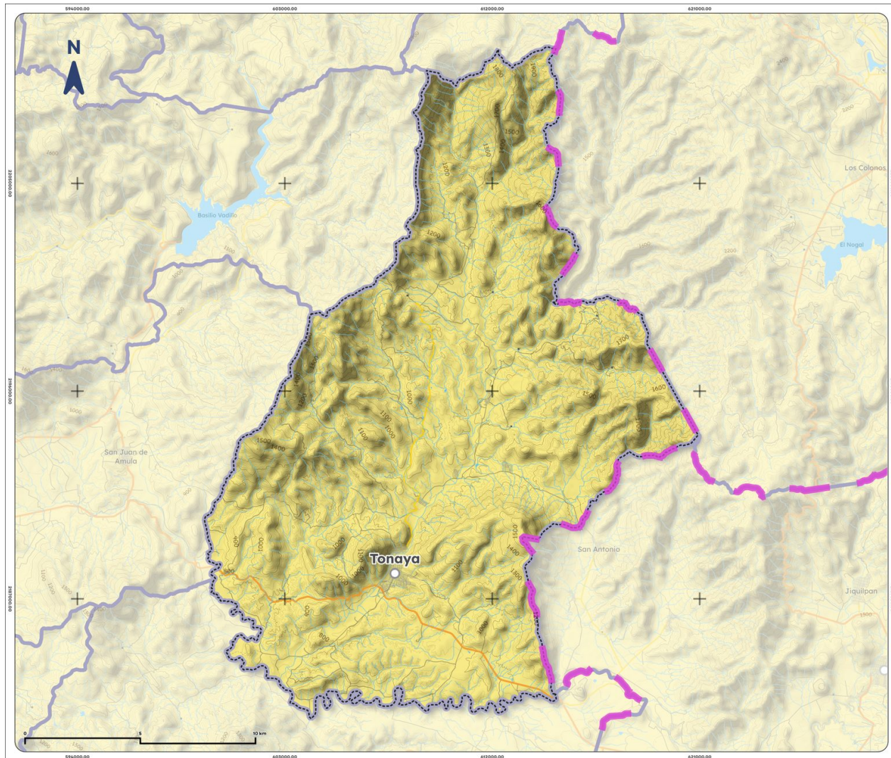
Mapa 7. Acuíferos de Tonaya, 2023
