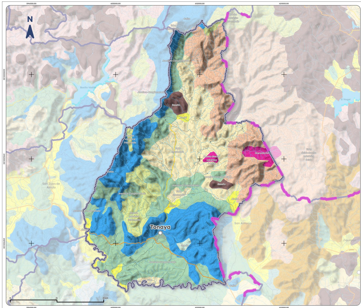
Mapa 3. Geología de Tonaya, 1988
