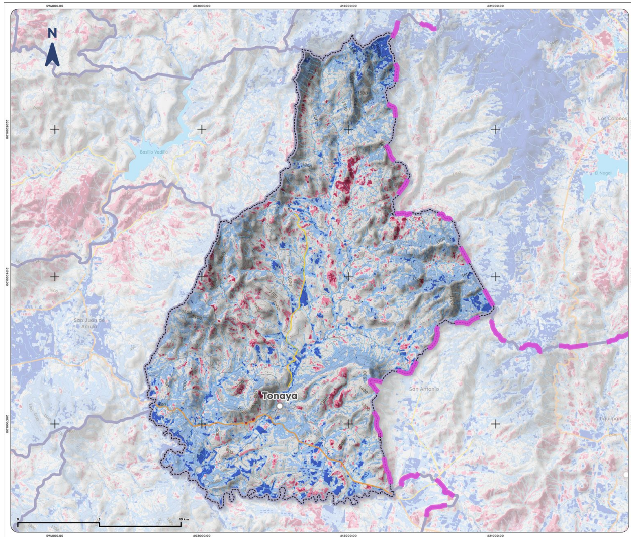
Mapa 13. NDWI promedio de Tonaya, 2025
