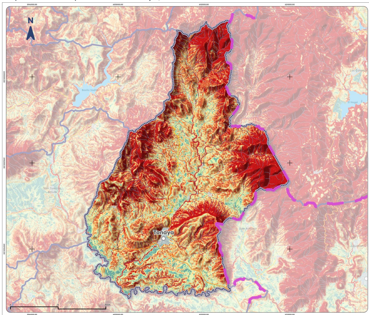
Mapa 16. Erosión potencial de Tonaya, 2025
